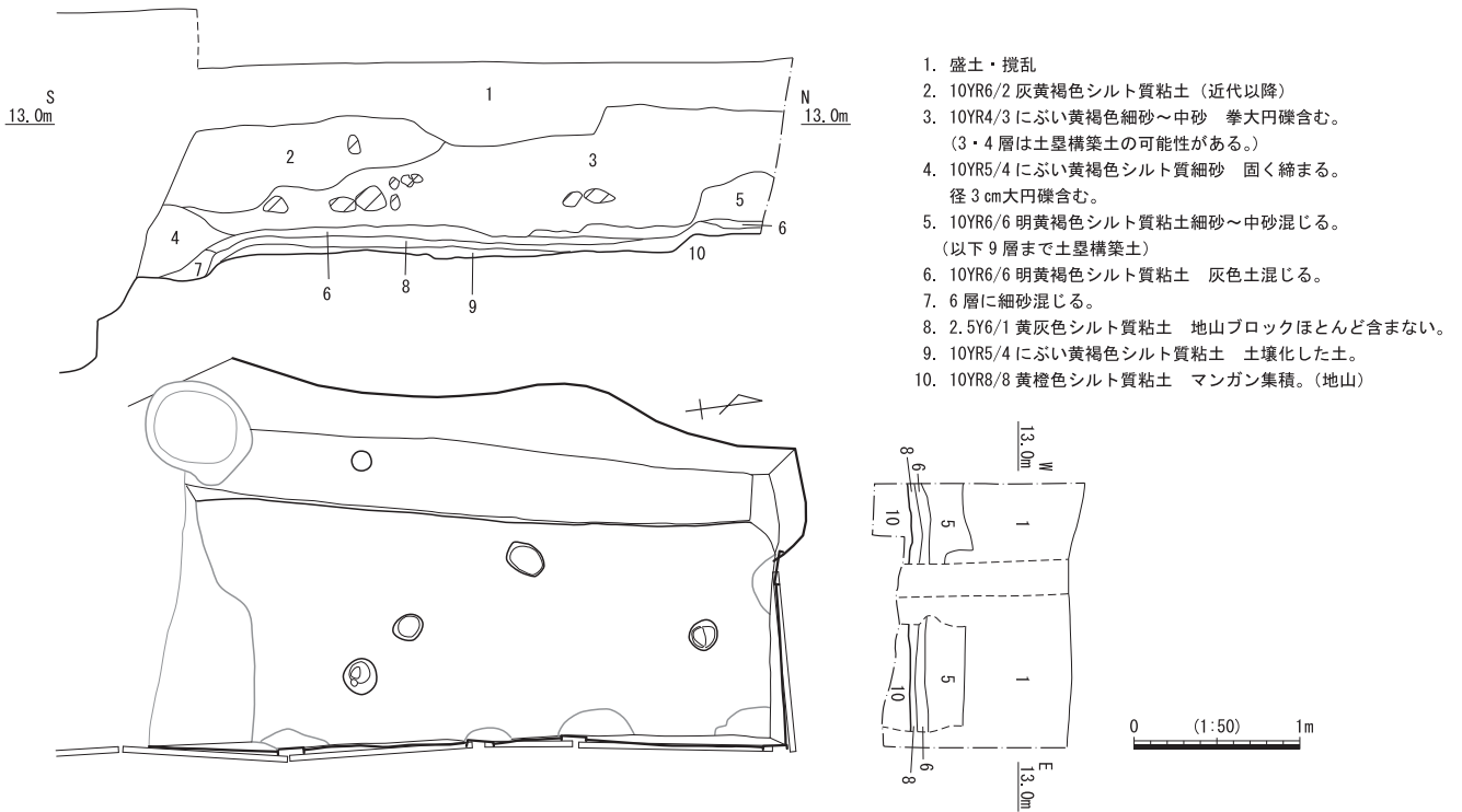
図17 土壘 平・断面図
