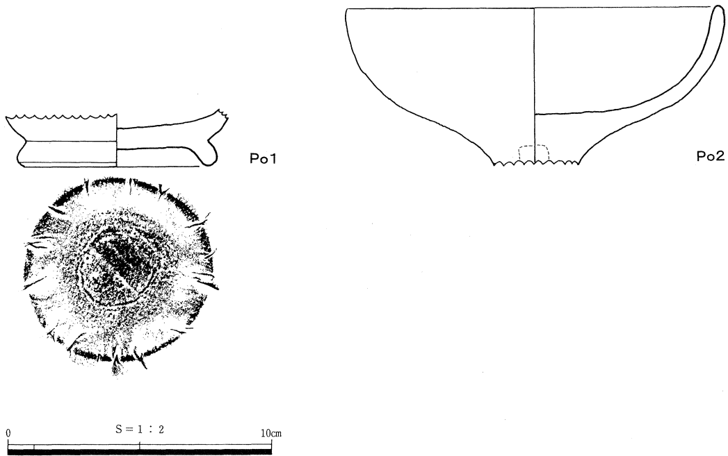
挿図13 出土遺物実測図
