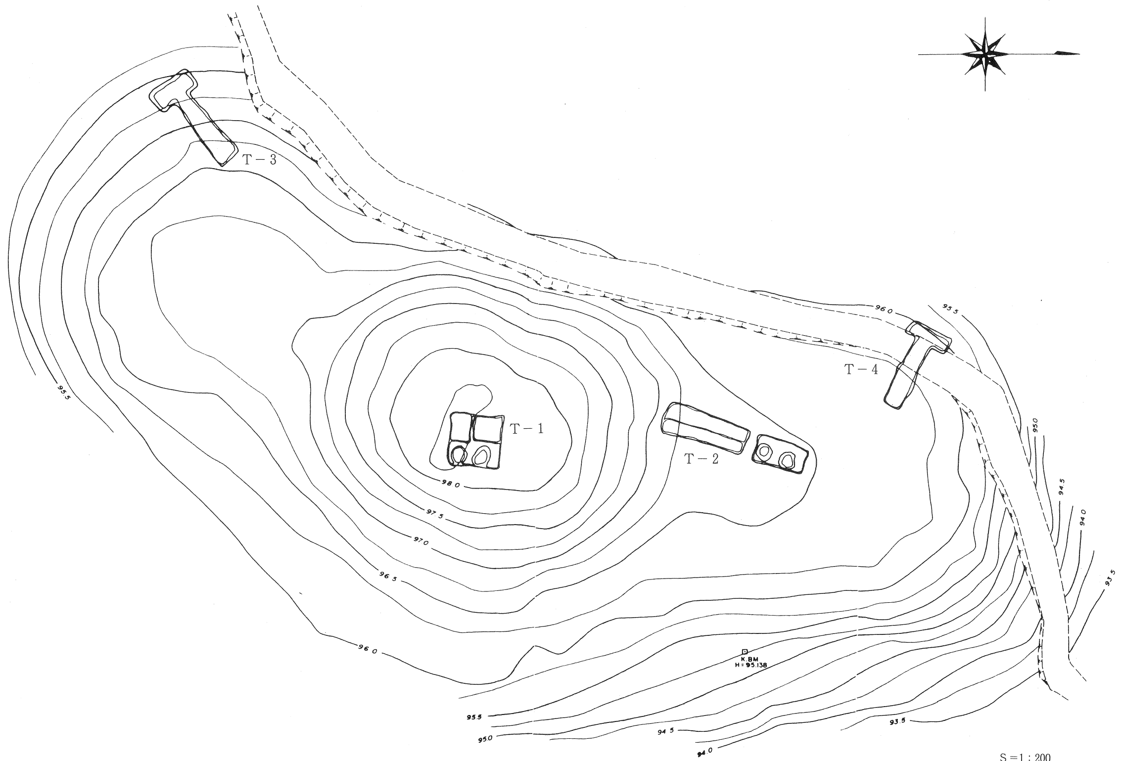
挿図2 渡一木6号墳トレンチ配置図
