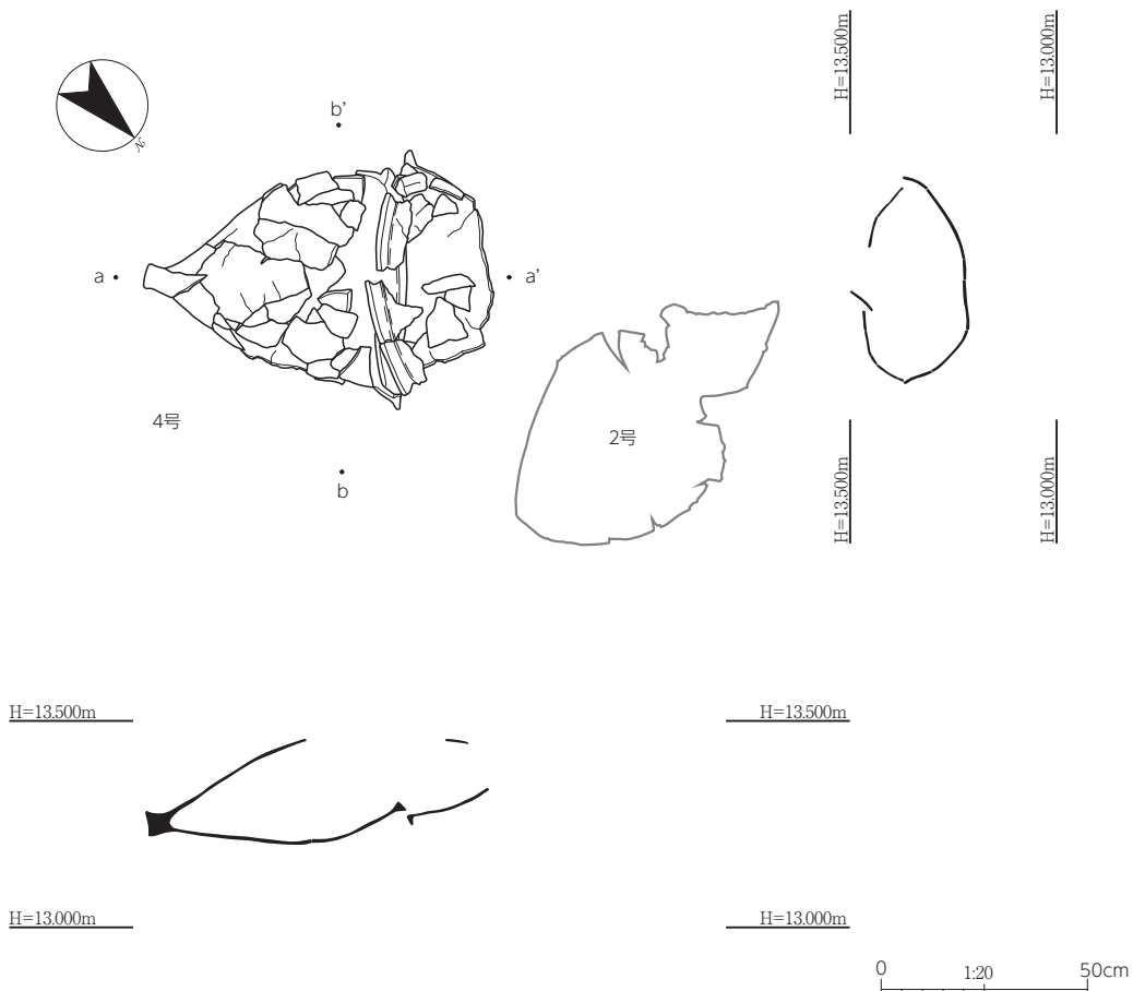
第 13 図 4号甕棺出土状況図
