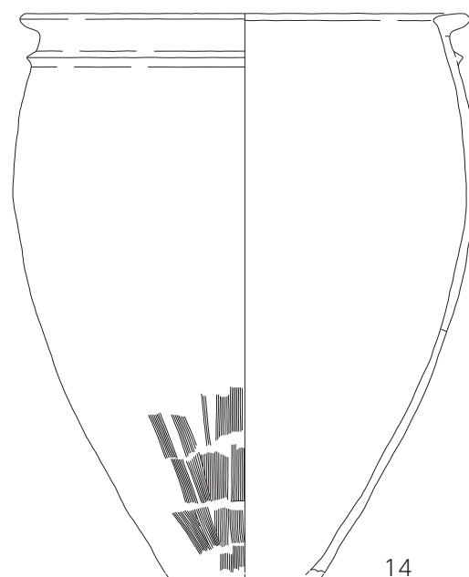
第12図 3号甕棺実測図
