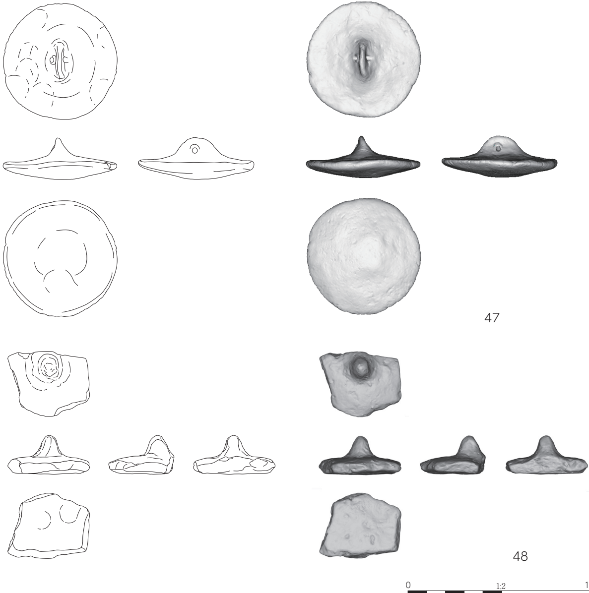
第24図 土製品実測図・オルソ展開図
