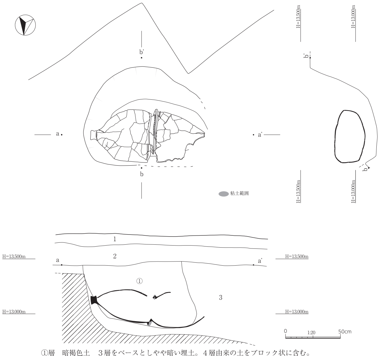
第11図 3号甕棺出土状況図
