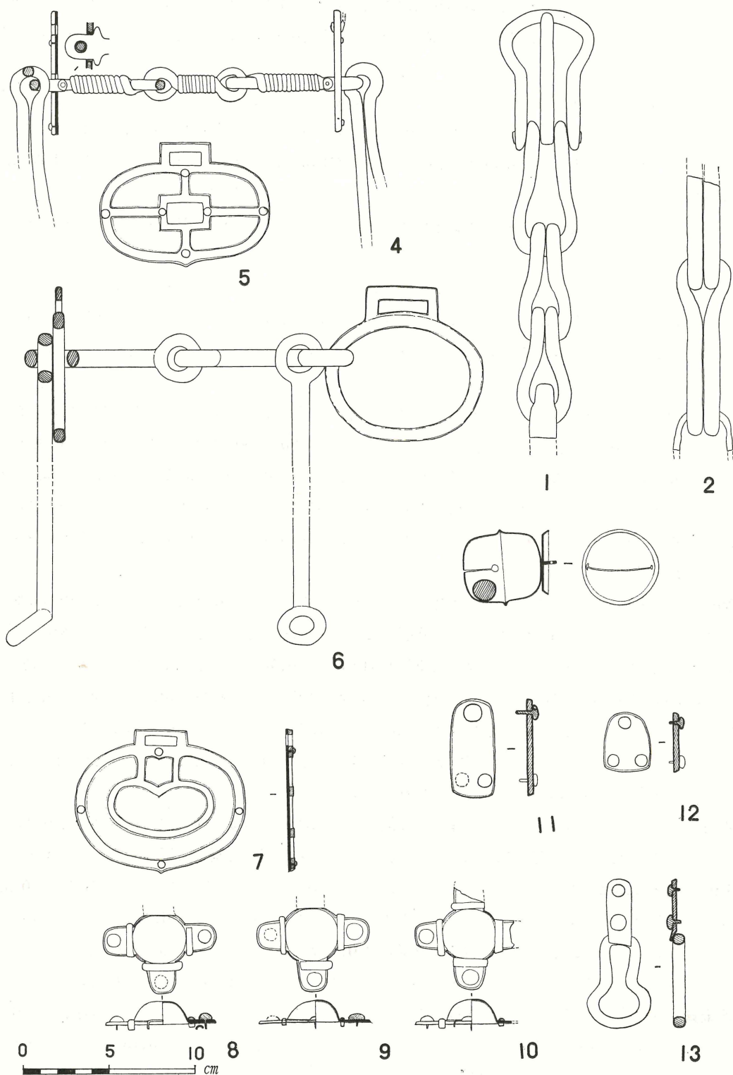
第11図 馬具類実測図 (その2)
