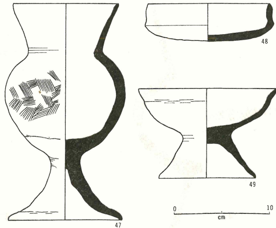
第9図 土師器実測図
