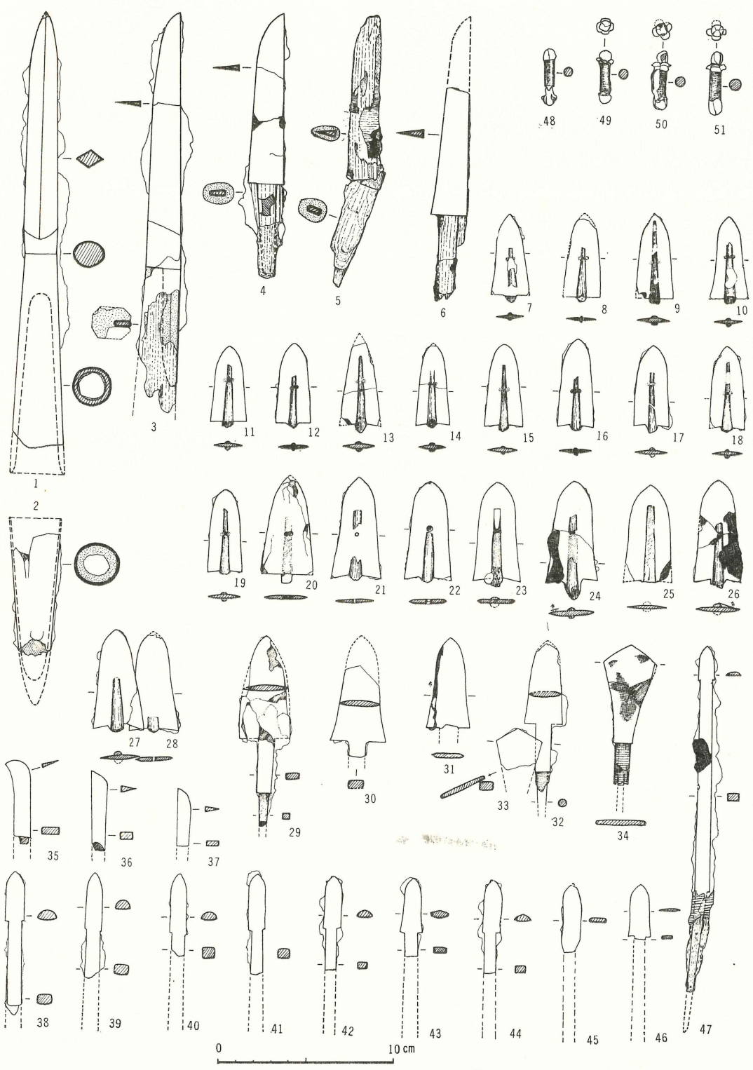
第13图 武器類 実測图
