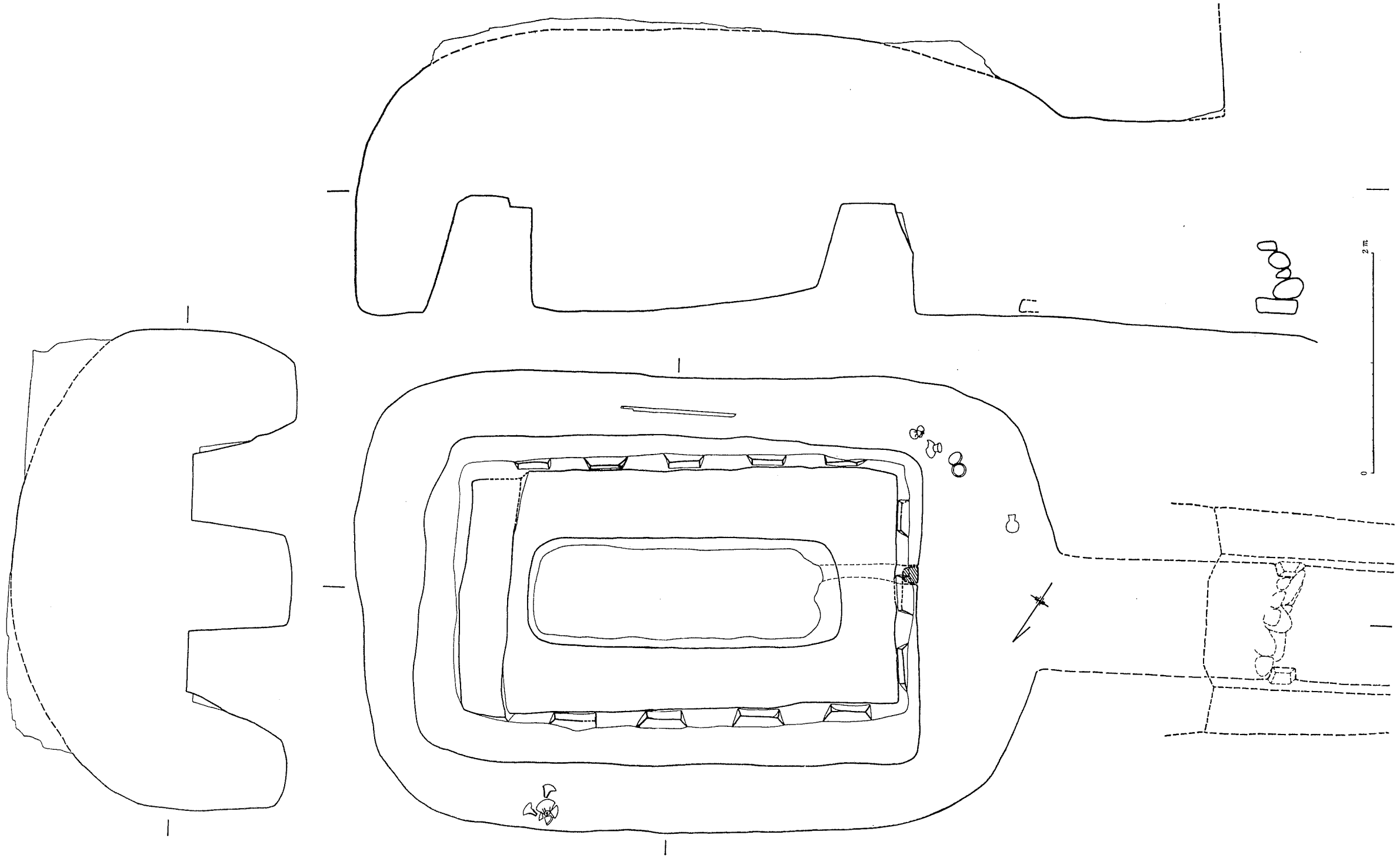
第2圖 橫穴墳構造圖
