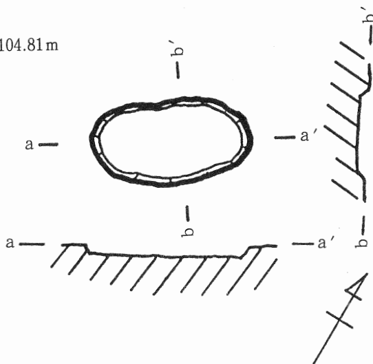
插图5 SK1遺構図
