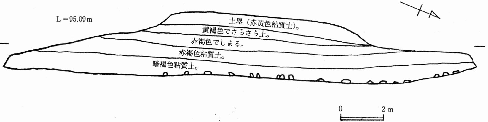
挿図7 水堀(濠)1・土塁1断面図
