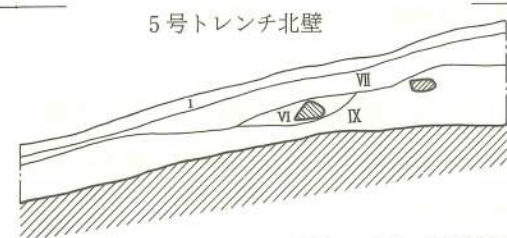
Fig. 17 船石遺跡基壇状遺構土層断面図
