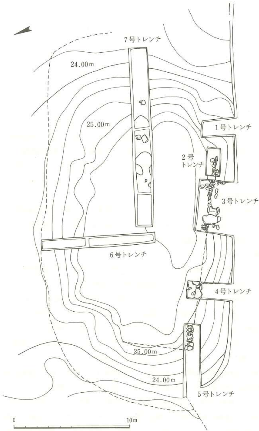
Fig. 15 船石遺跡基壇状遺構実測図
