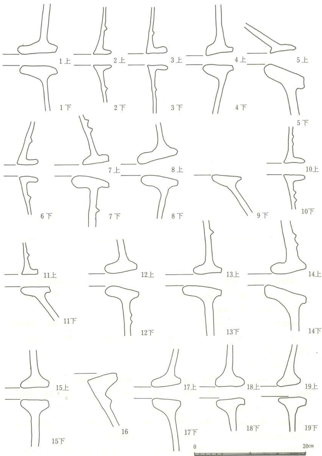
Fig. 18 船石遺跡北区出土甕棺口縁部実測図
