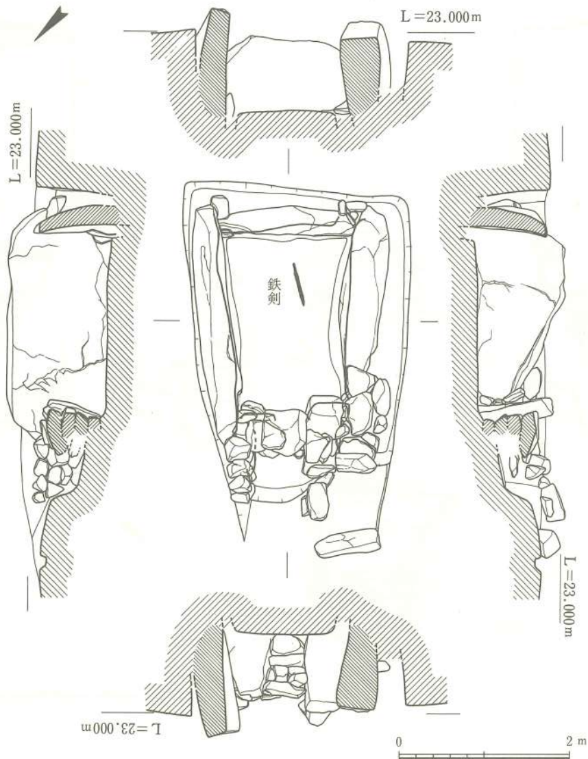
Fig. 14 船石遺跡3号墳石室実測図
