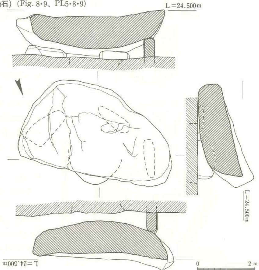
Fig. 8 船石遺跡 2号支石墓(船石) 実測図
