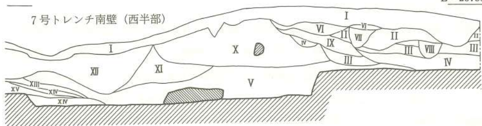
Fig. 16 船石遺跡基壇状遺構石列実測図
