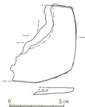
Fig. 5 11号土壇出土鉄製鋤先実測図
