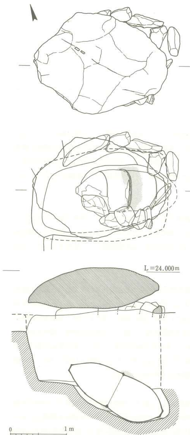
Fig. 7 船石遺跡 1号石墓(亀石)実測図
