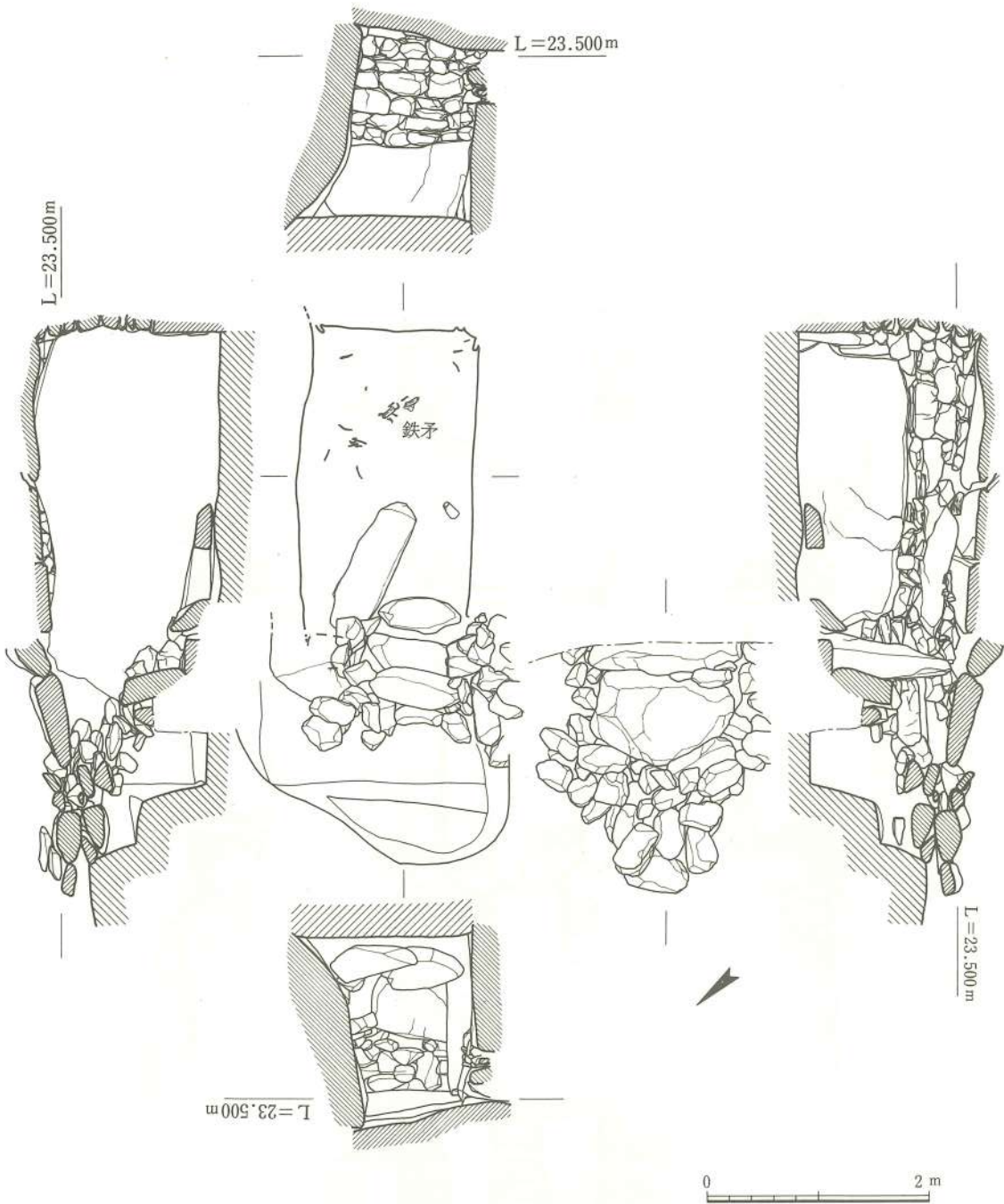
Fig. 13 船石遺跡 2号墳石室実測図
