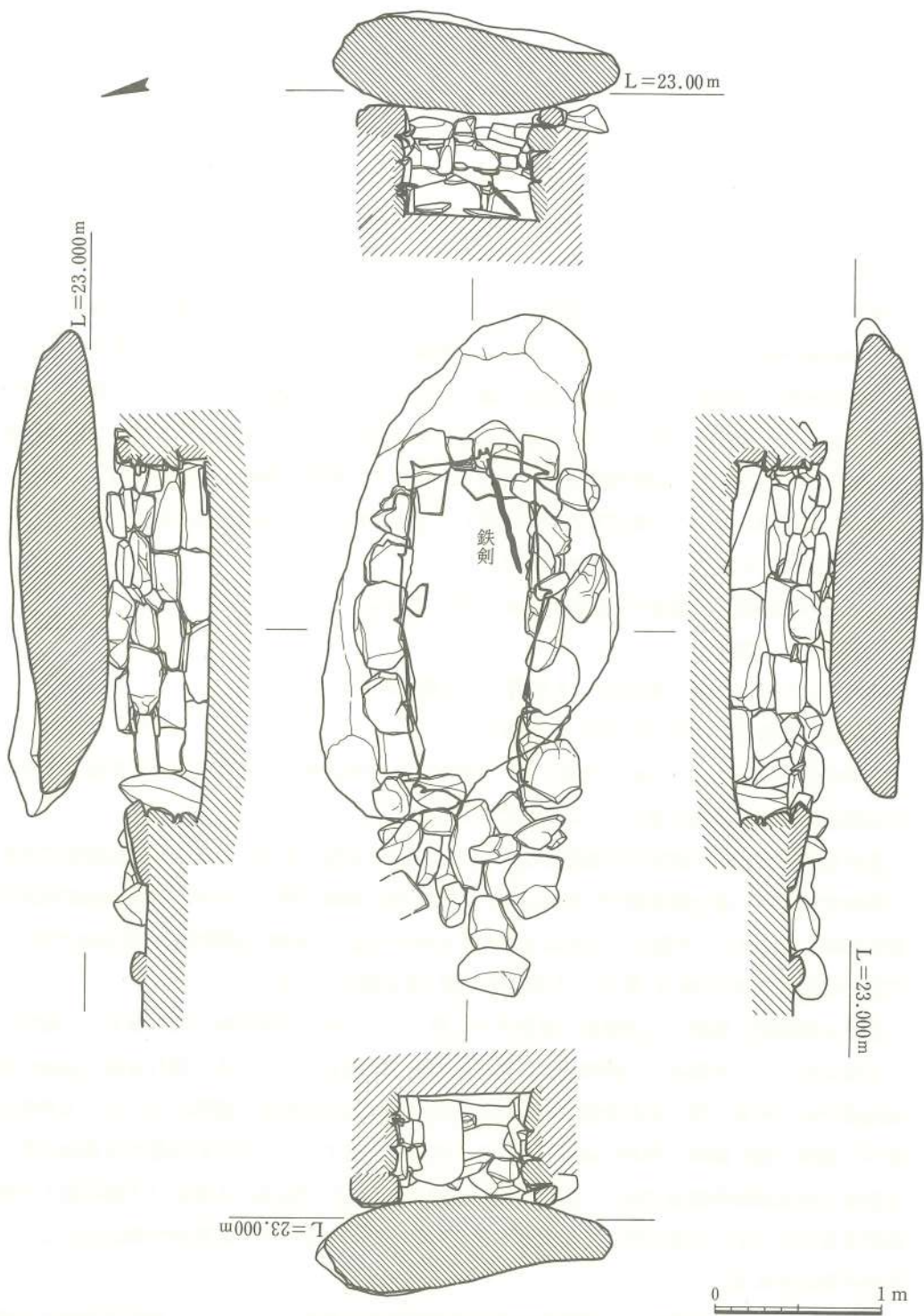
Fig. 10 船石遺跡1号墳(鼻血石)石室実測図
