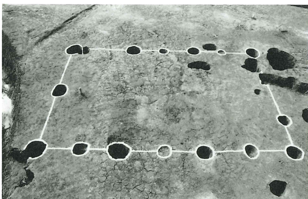
第31号掘立柱建物跡
