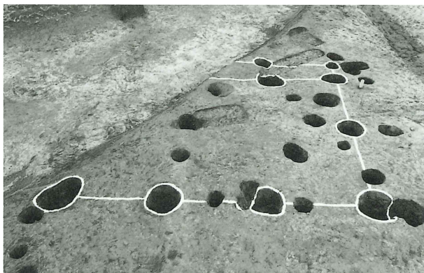
第28号掘立柱建物跡
