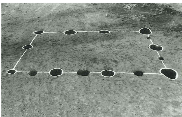
第29号掘立柱建物跡
