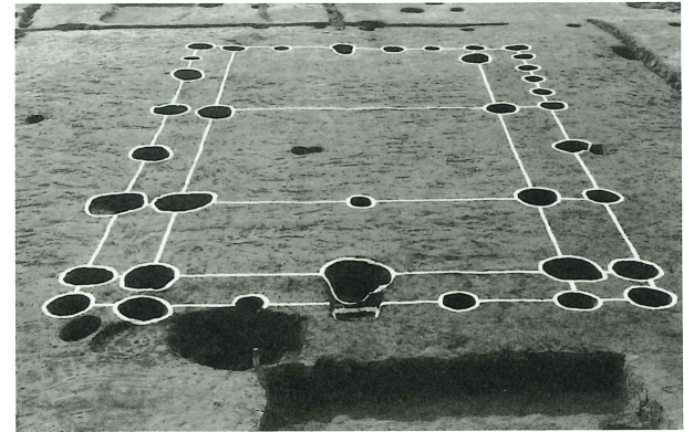
第21号掘立柱建物跡
