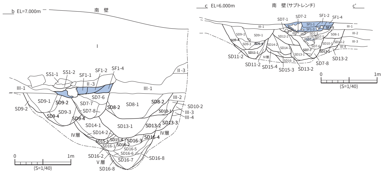
図 18 SF 1 土層断面図
