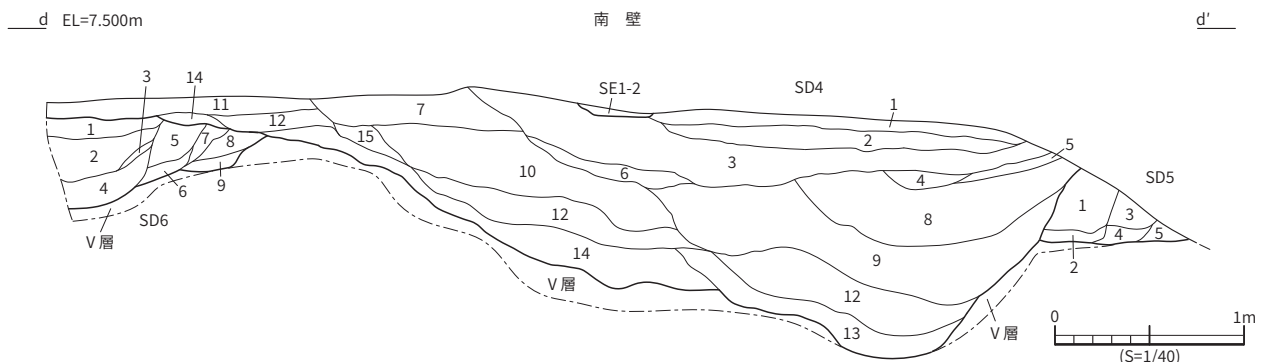
図 22 SD 4～6 土層断面図
