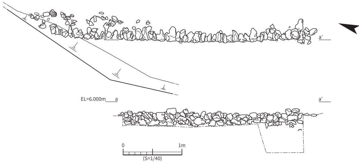
図 17 SF 1 平面・立面図
