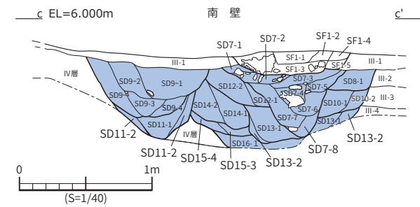
図26 SD 7～16サブトレンチ土層断面図
