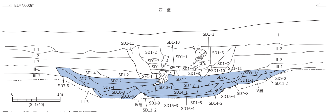
図27 SD 7・9～16土層断面図
