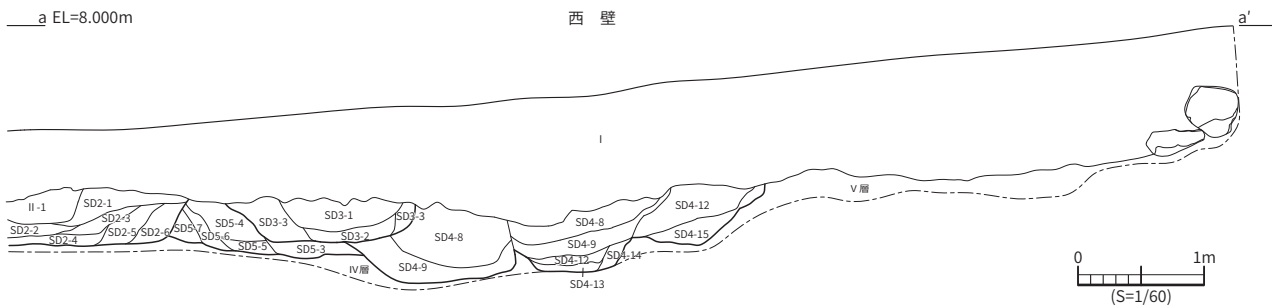
図 21 SD 2～5 土層断面図
