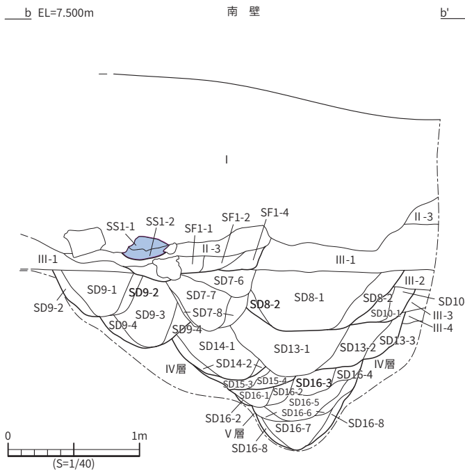
図15 SS 1土層断面図
