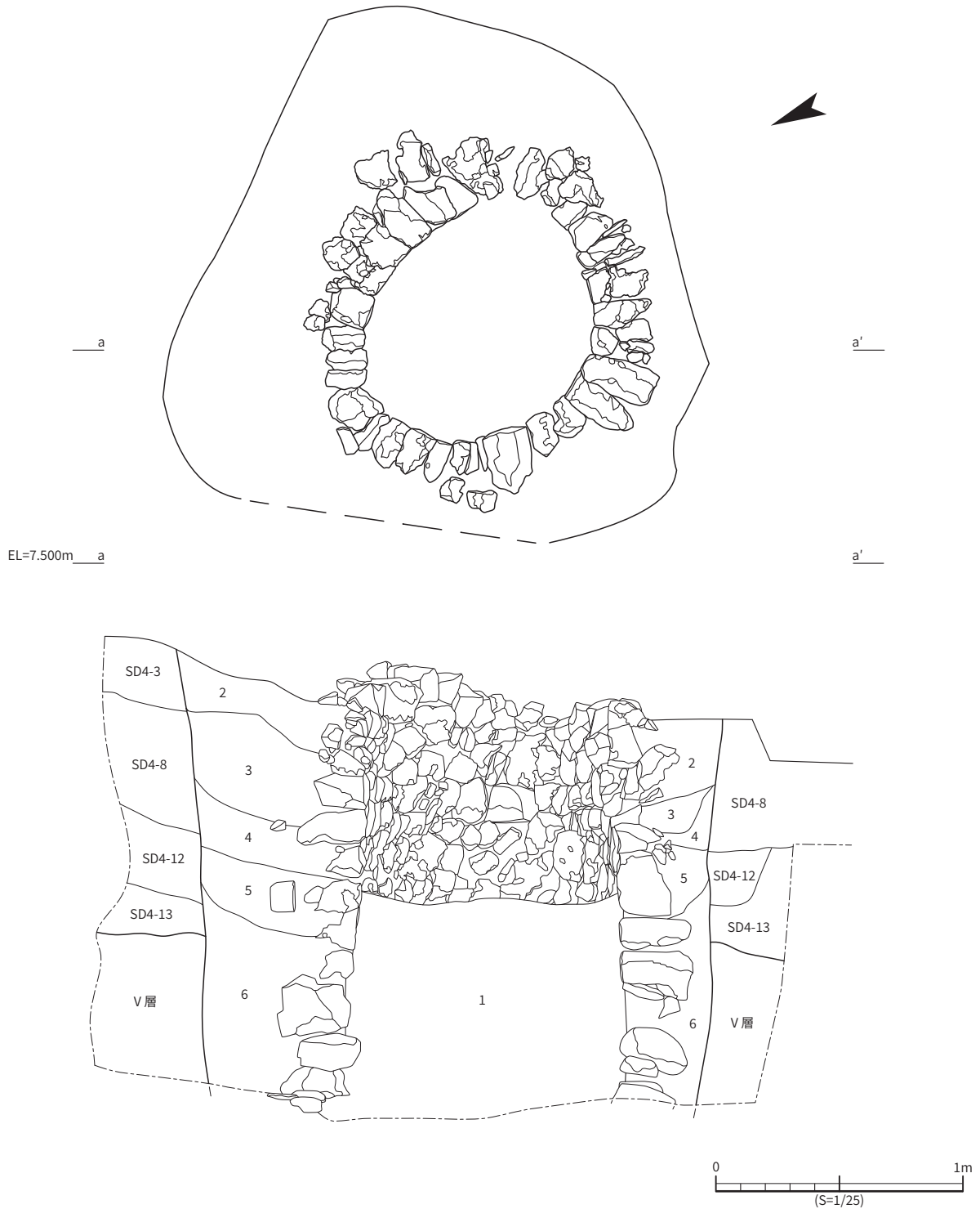
図 13 SE 1 平面・土層断面図
