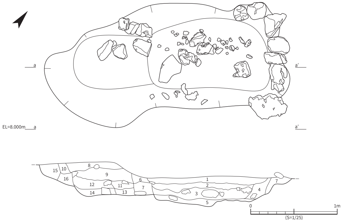
図10 SK 2 平面・土層断面図
