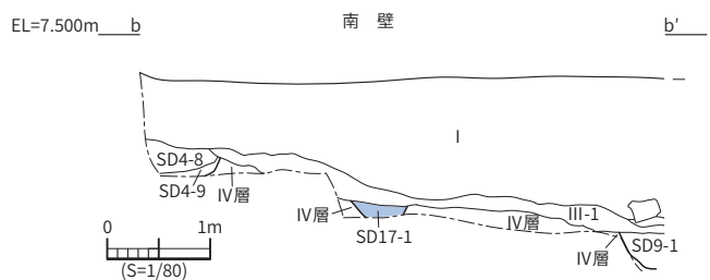
図34 SD17 土層断面図
