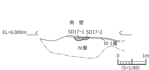
図33 SD17 サブトレンチ土層断面図
