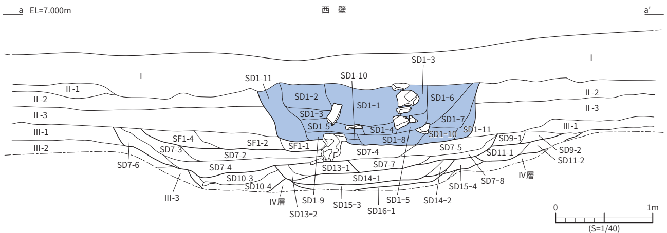
図 12 SD 1 土層断面図
