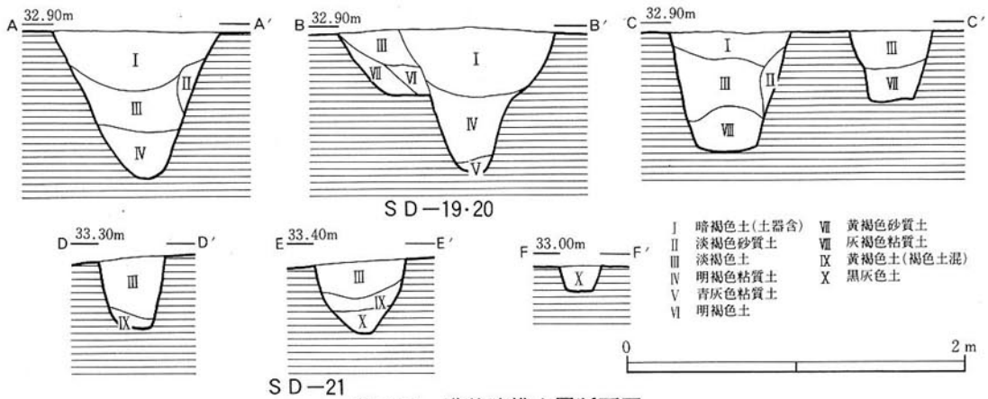
第10図 溝状遺構土層断面図
