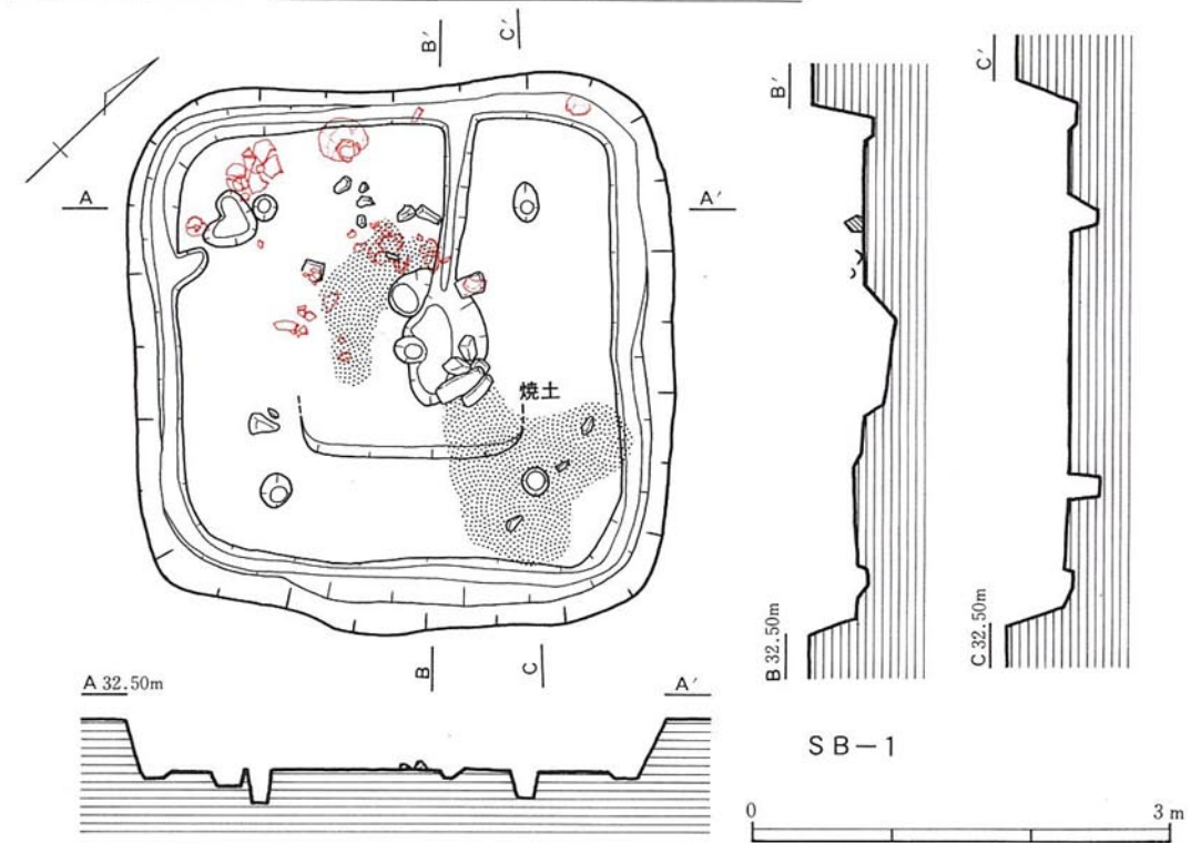
第5図 竪穴住居跡実測図(1)
