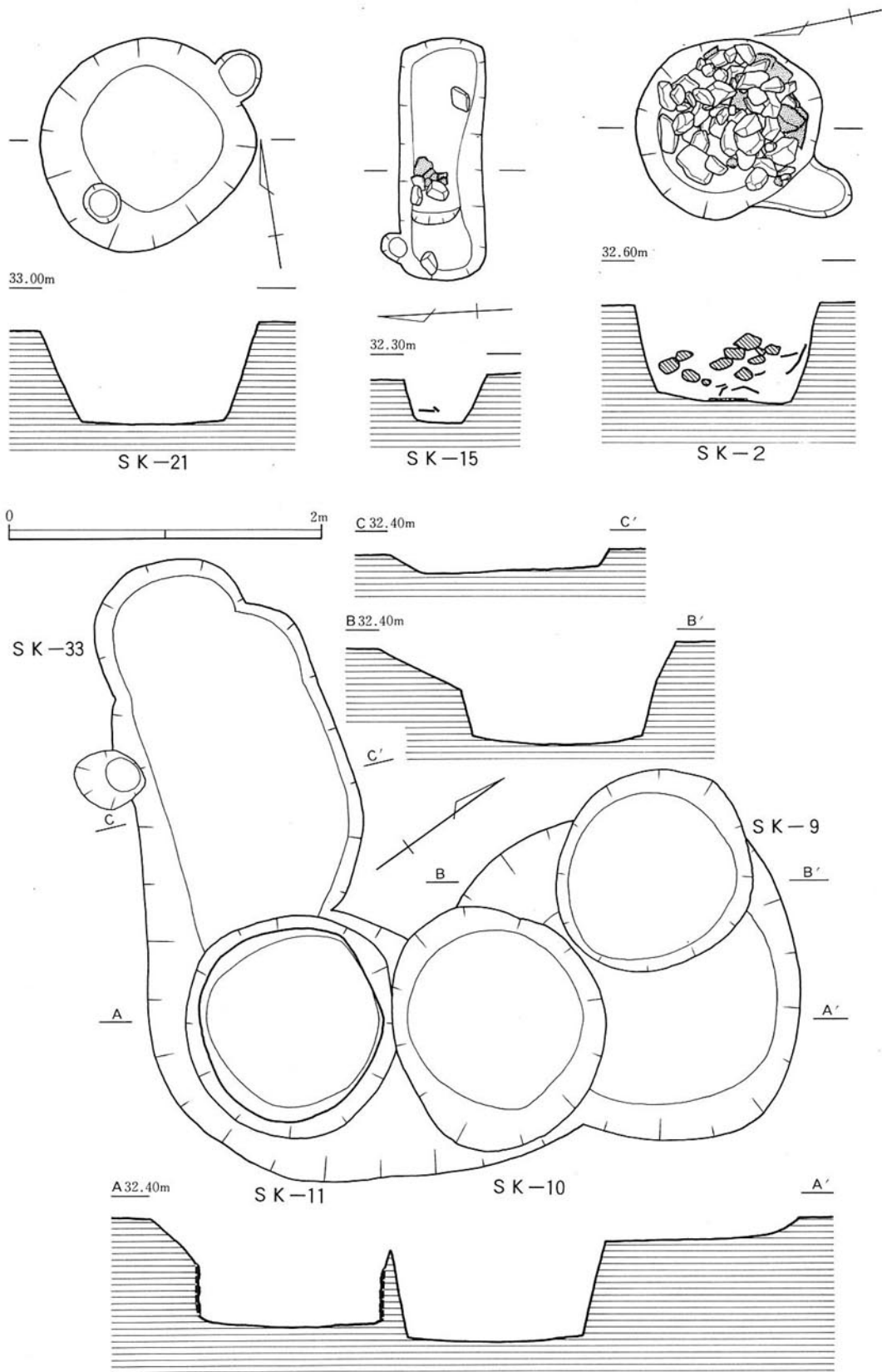
第9図 土坑実測図
