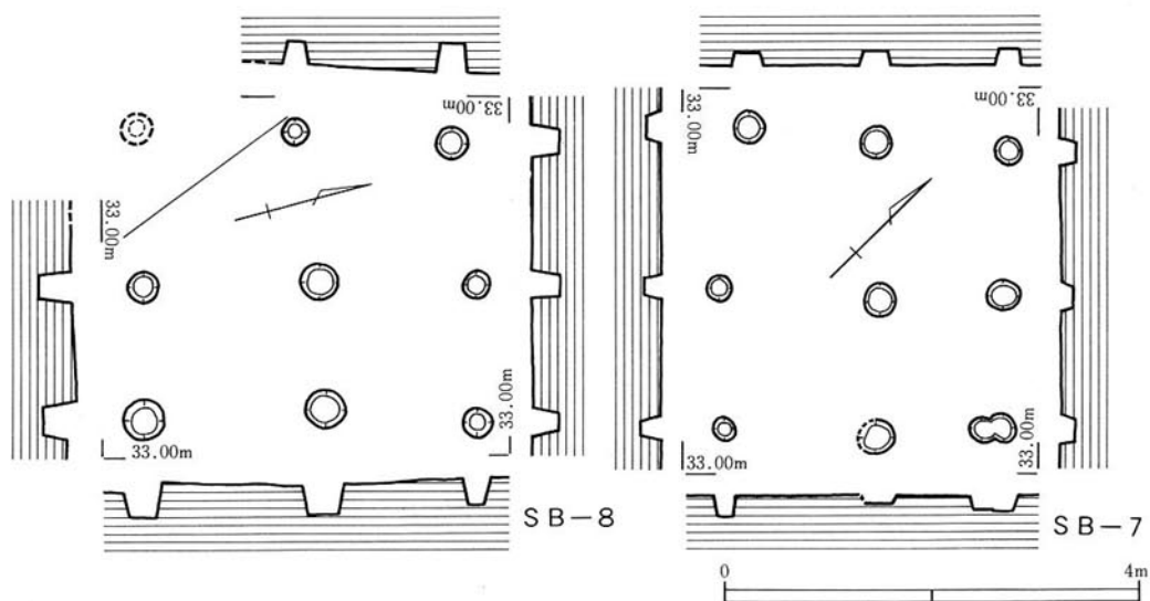
第8図 掘立柱建物跡実測図
