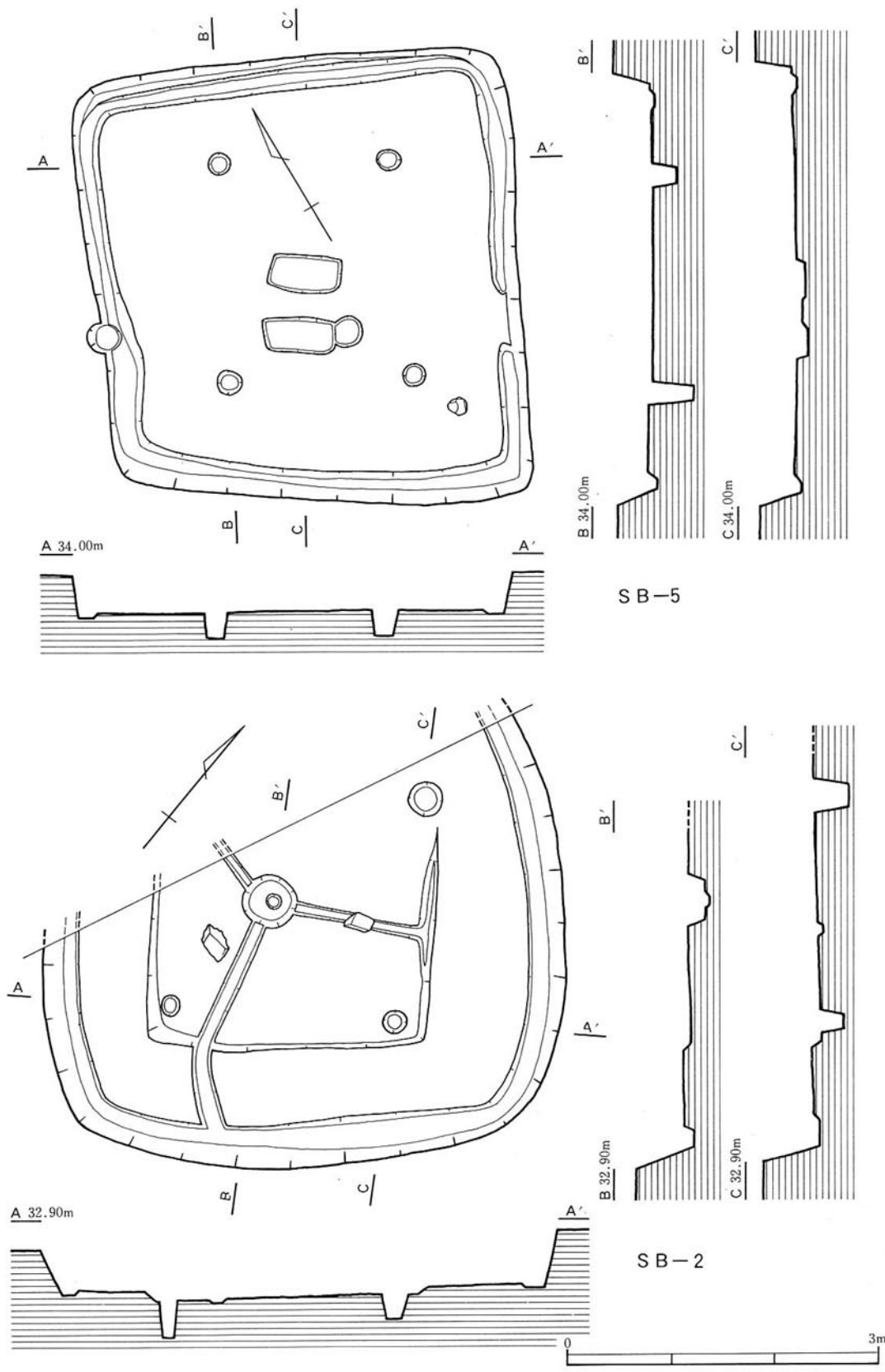
第6図 竖穴住居跡実測図(2)
