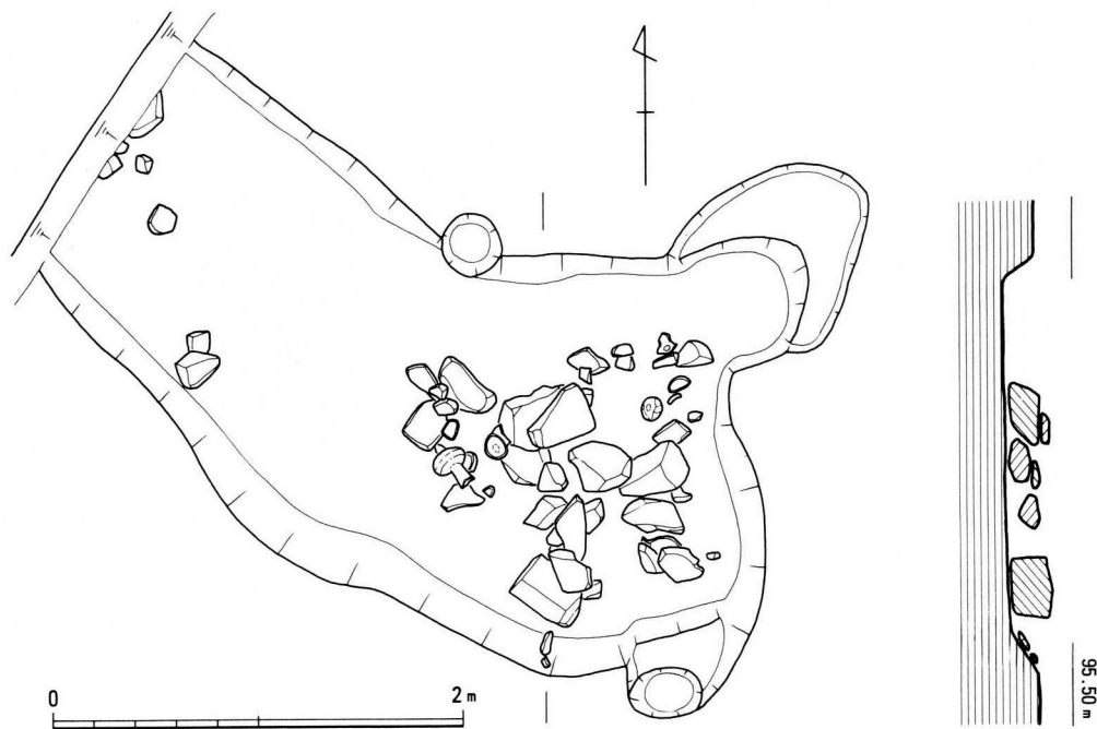
第8図 3号墳 S T-3 周濠部実測図
