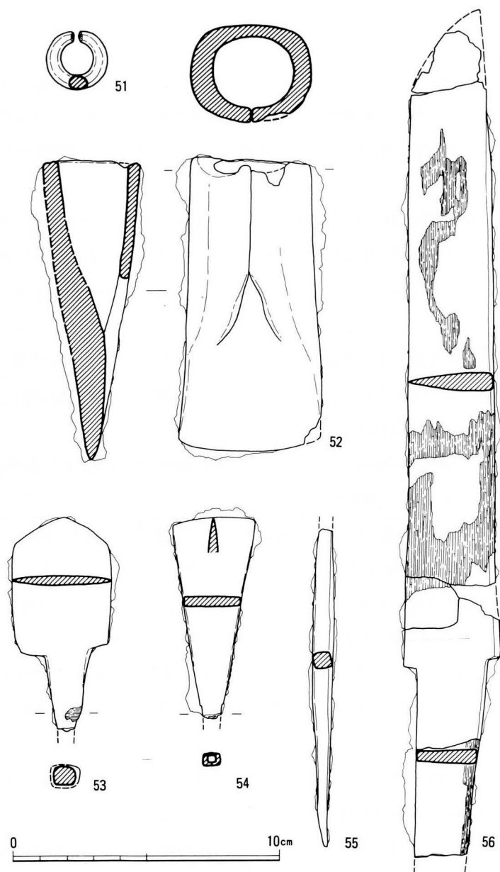
第12図 耳環・鉄器実測図
