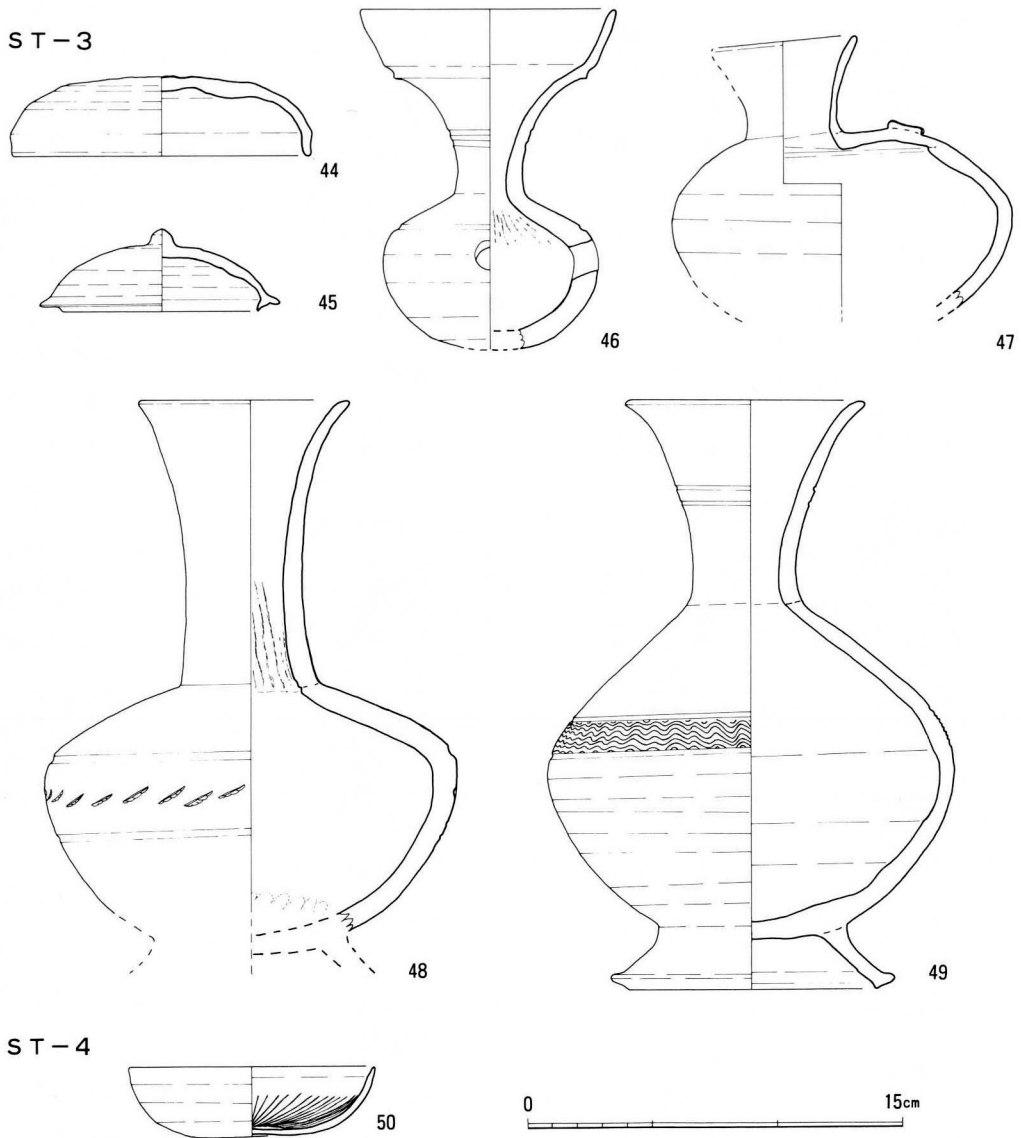
第11図 須恵器・土師器実測図
