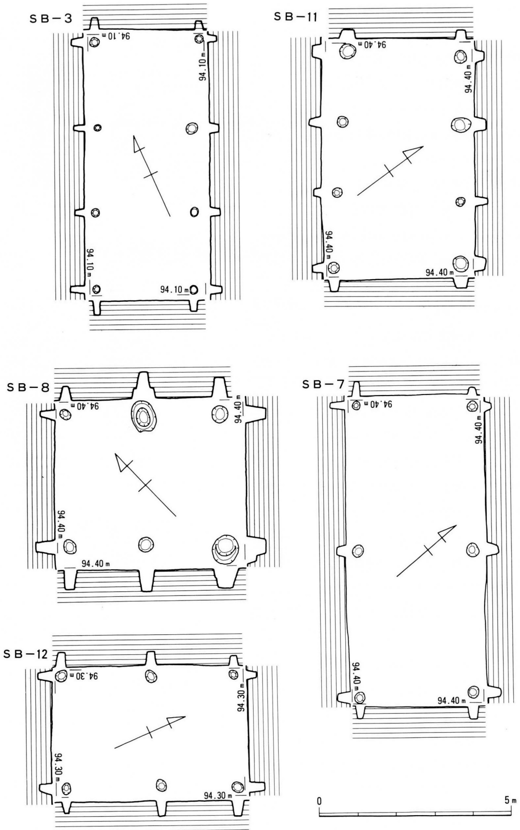
第15图 掘立柱建物实测图(3)
