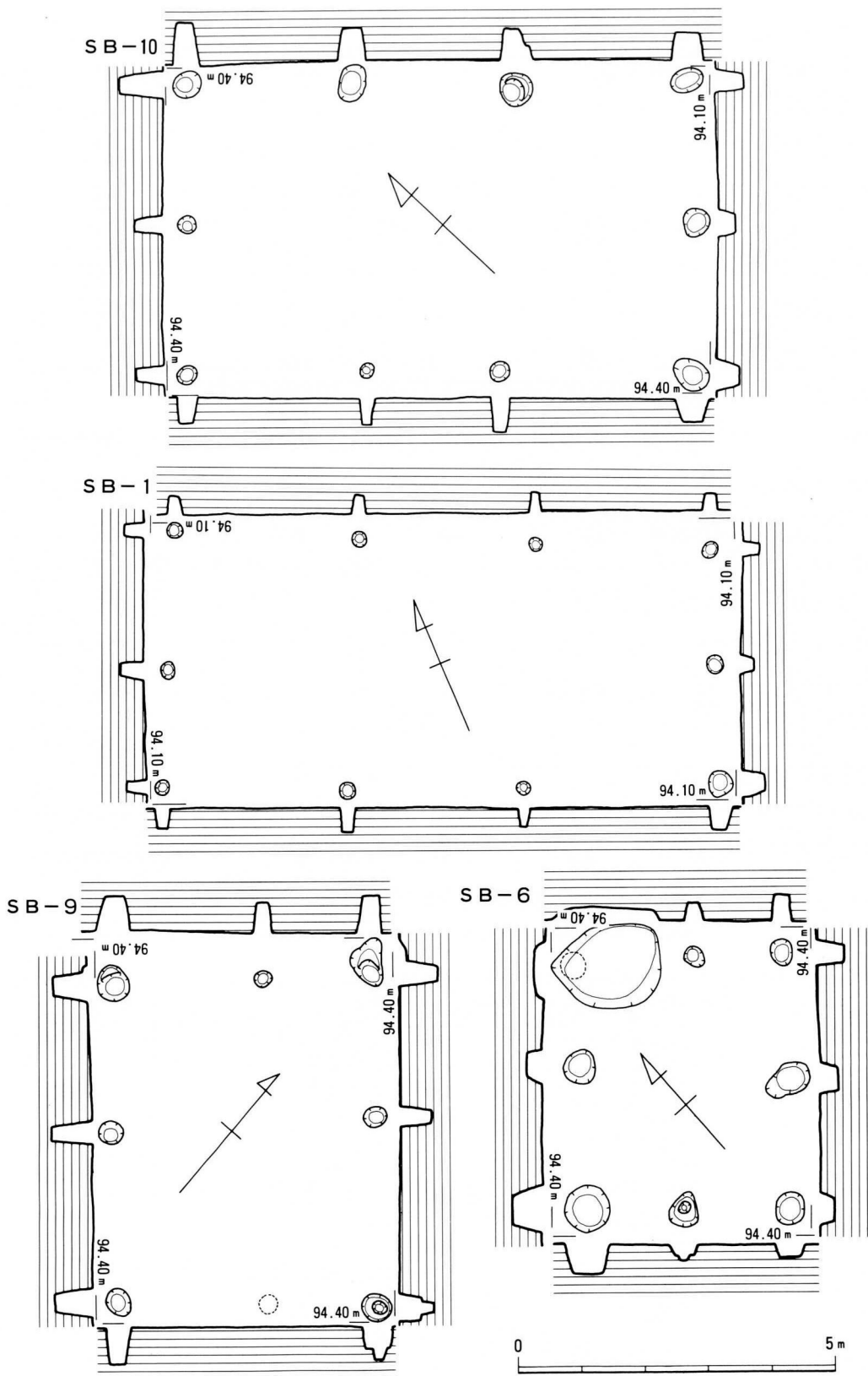
第13图 掘立柱建物实测图(1)
