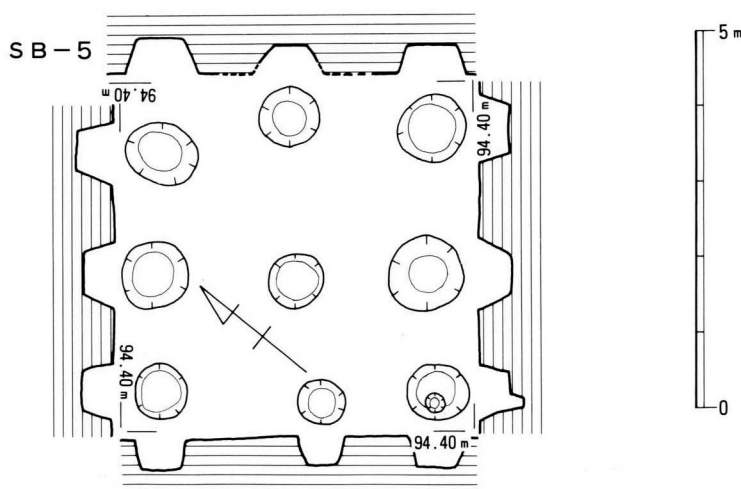
第14图 掘立柱建物实测图(2)
