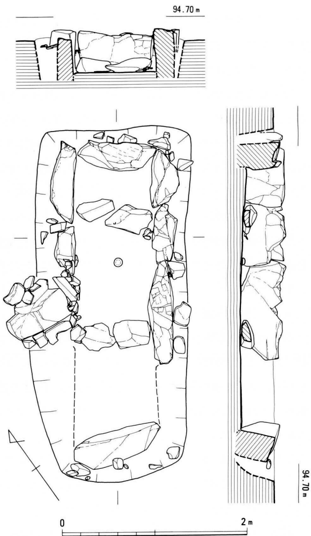
第9図 4号墳ST-4石室実測図
