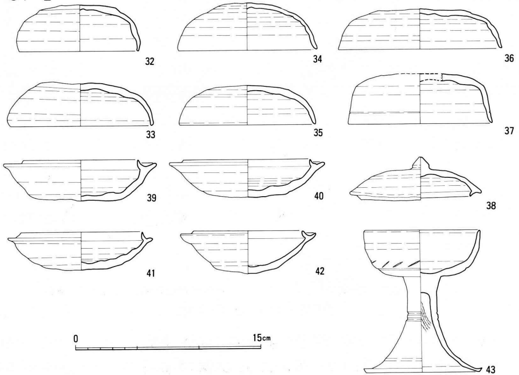
第10図 須恵器実測図
