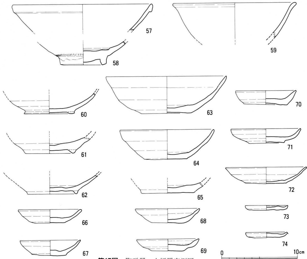
第17図 陶磁器・土師器実測図
