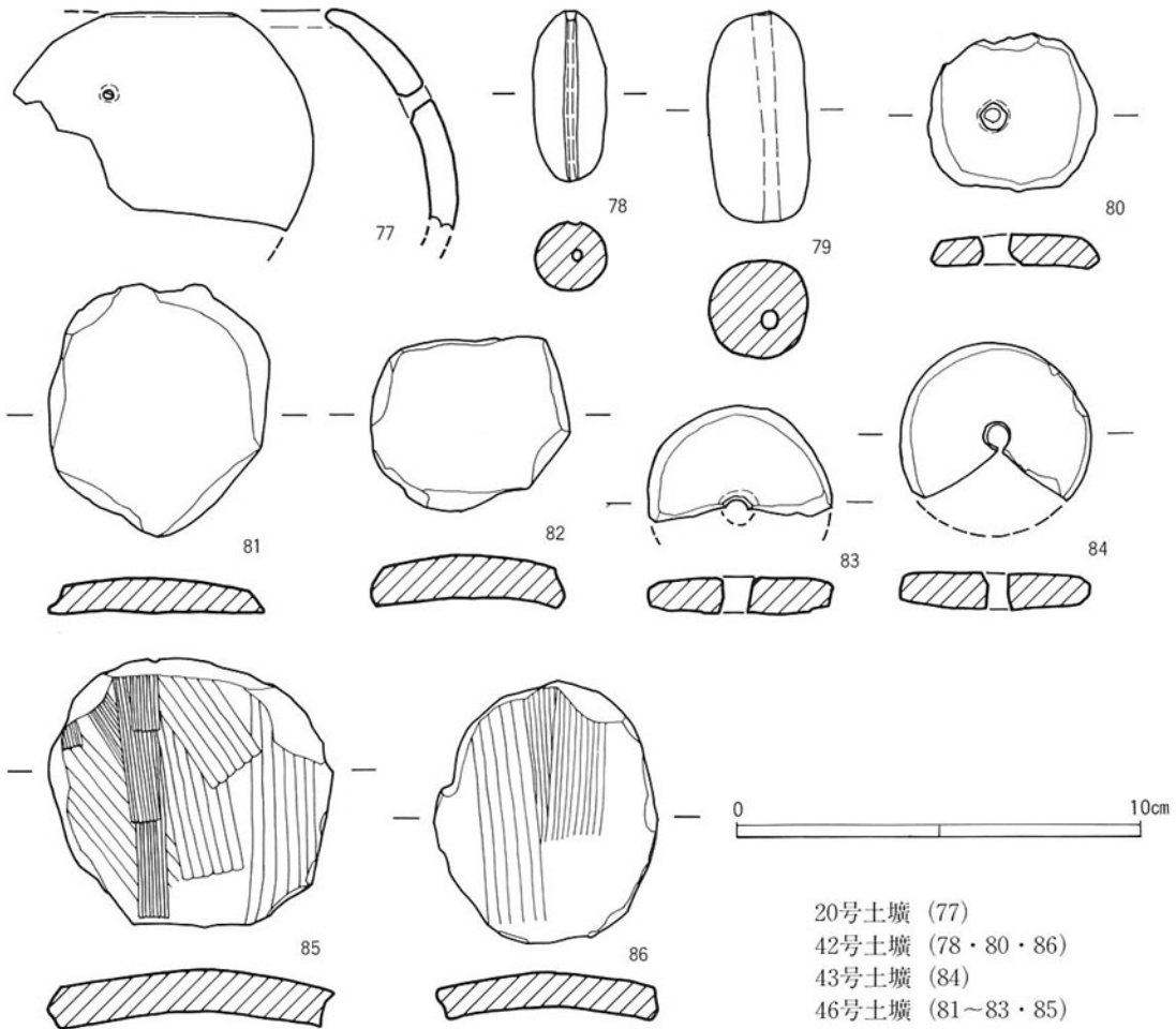
▲図14 出土土製品実測図
