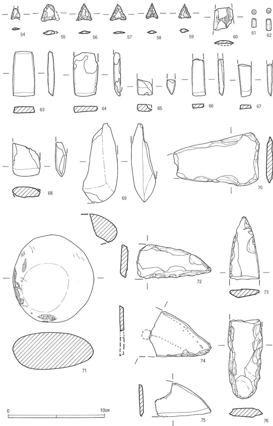
▲图13 出土石器实测图
