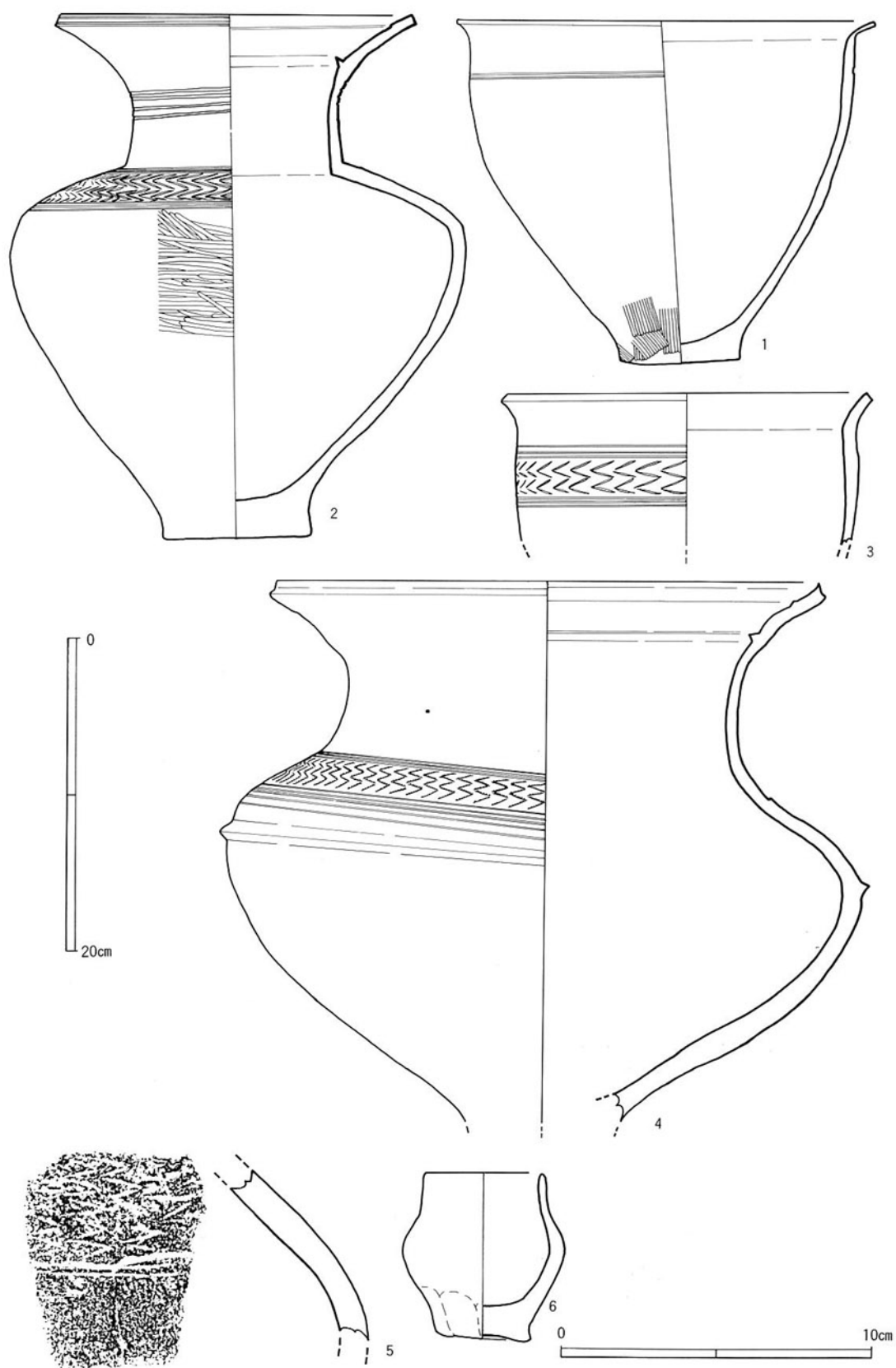
▲图8 出土土器实测图 (1) 1号土坑(2·5·6)、2号土坑(1·4)、37号土坑(3)
