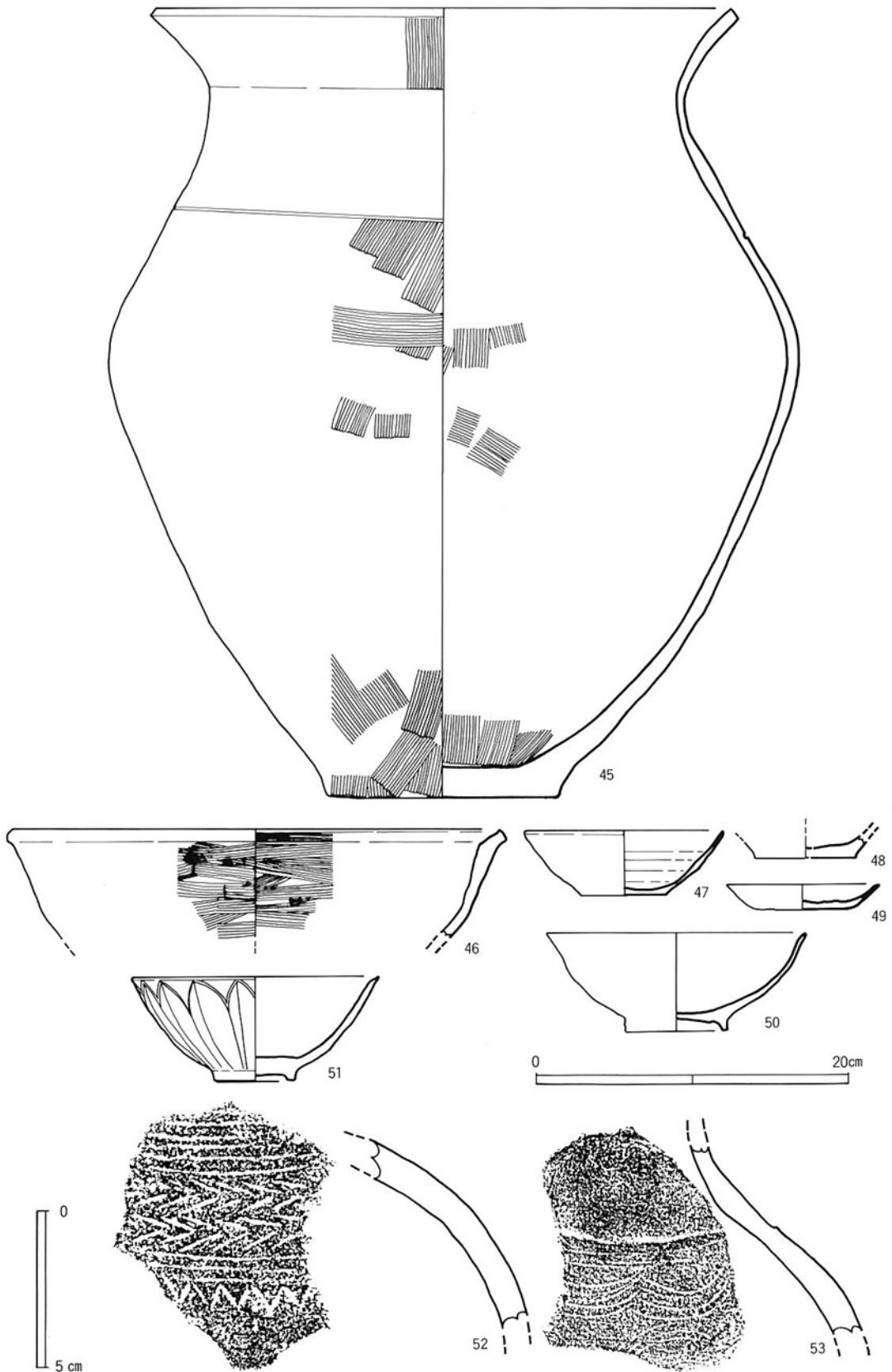
▲図12 出土土器実測図 (5) 3号土壙(51)、4号土壙(46~48)、74号土壙(45・52・53)、図3 矢印の柱穴(49・50)
