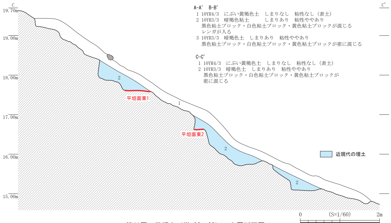
第11図 栄螺山（栄-02・03） 土層断面図
