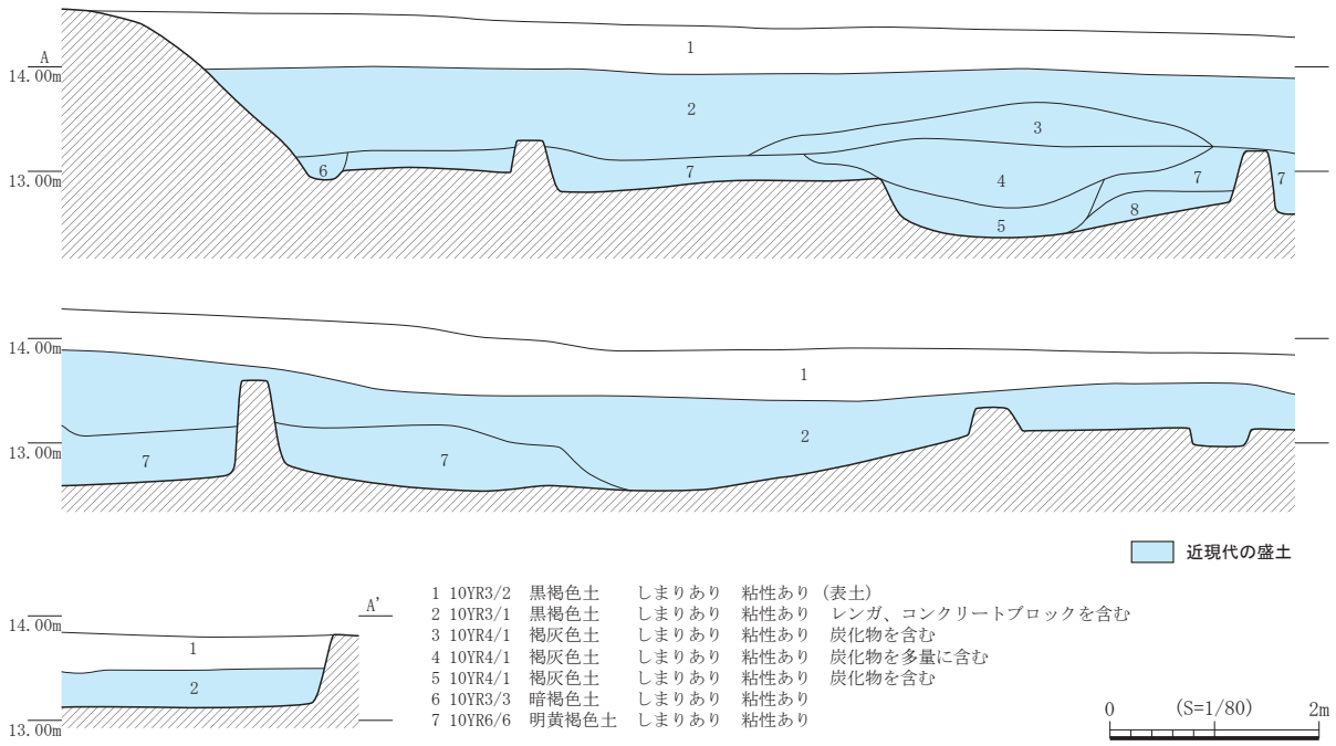
第47図 余芳 遺構平面・南壁面土層断面図
