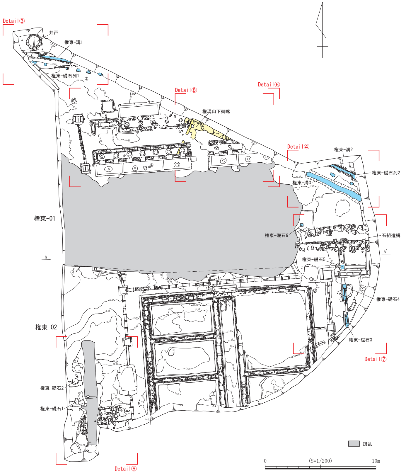
第34図 権現山東 遺構平面図
