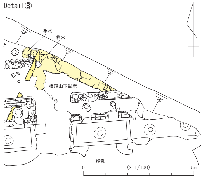
第43図 権現山東（権東-01） 権現山下御席 平面図 (Detail⑧)
