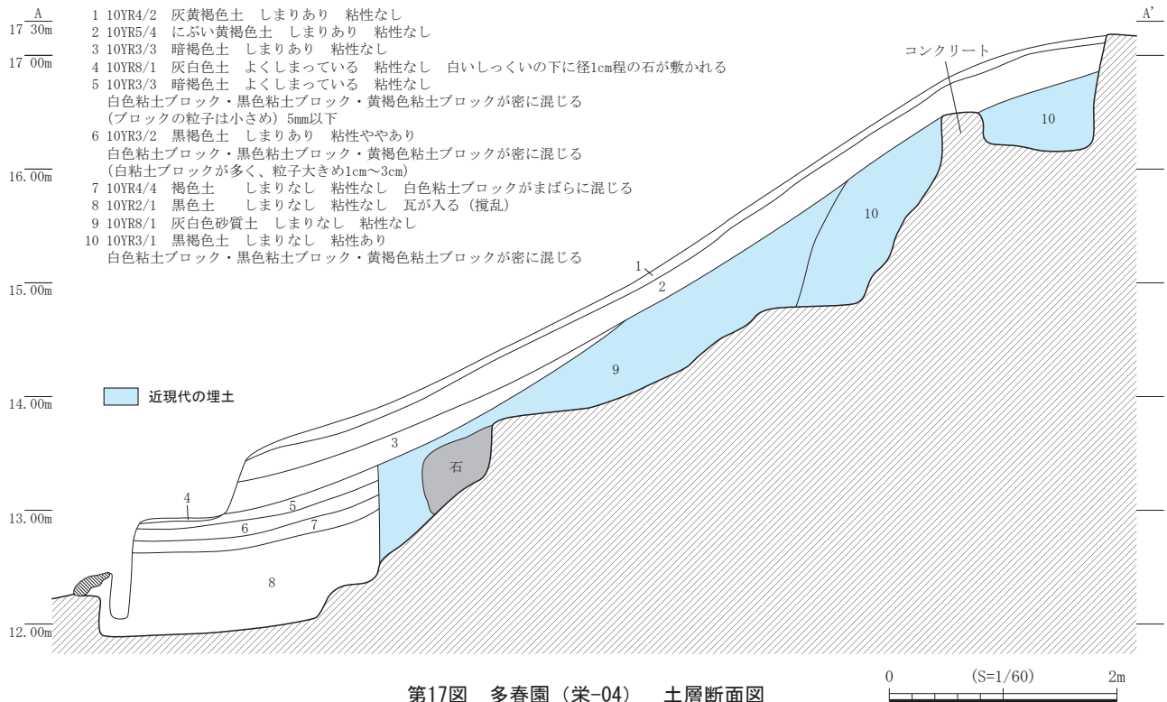
第17図 多春園(栄-04) 土層断面図
