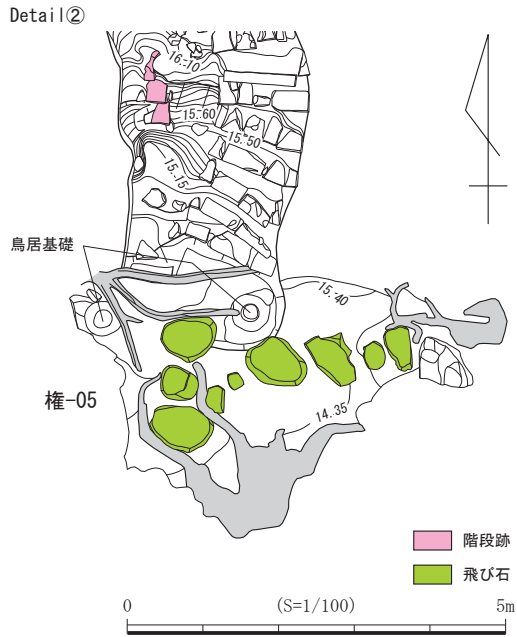
第32図 権現山（権-05）飛び石群平面図（Detail②）
