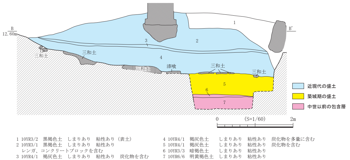
第49図 余芳 南西角壁面土層断面図
