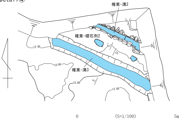
第42図 権現山東 (権東-01) 遺構平面・断面図 (Detail③・④)
