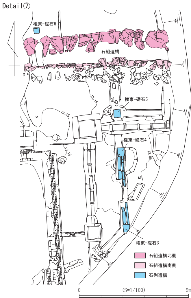
第44図 権現山東（権東-02）遺構平面図 (Detail⑦)
