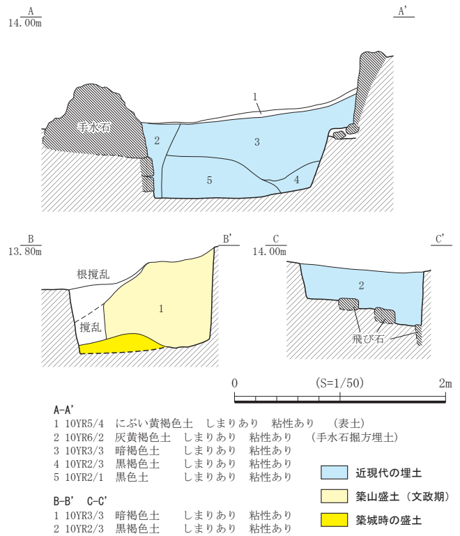
第25図 二子山（二-01・02・08） 土層断面図
