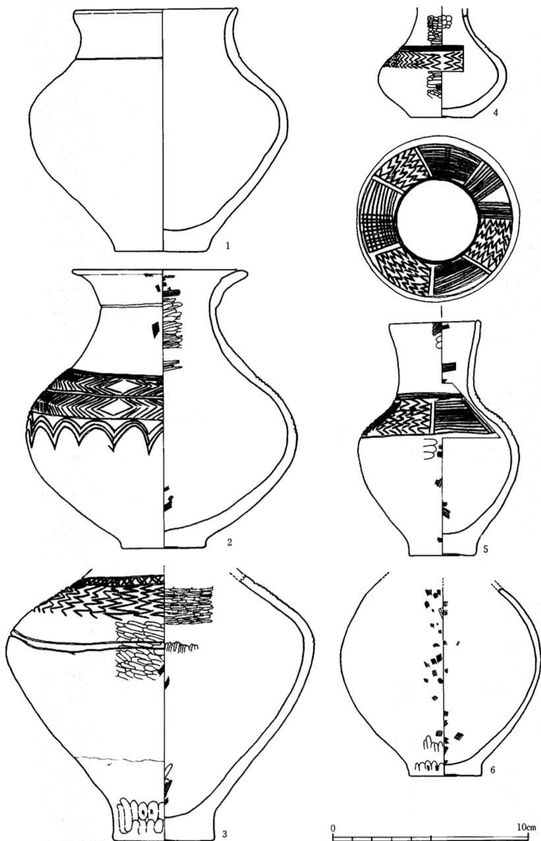
△出土遺物実測図（弥生土器）
