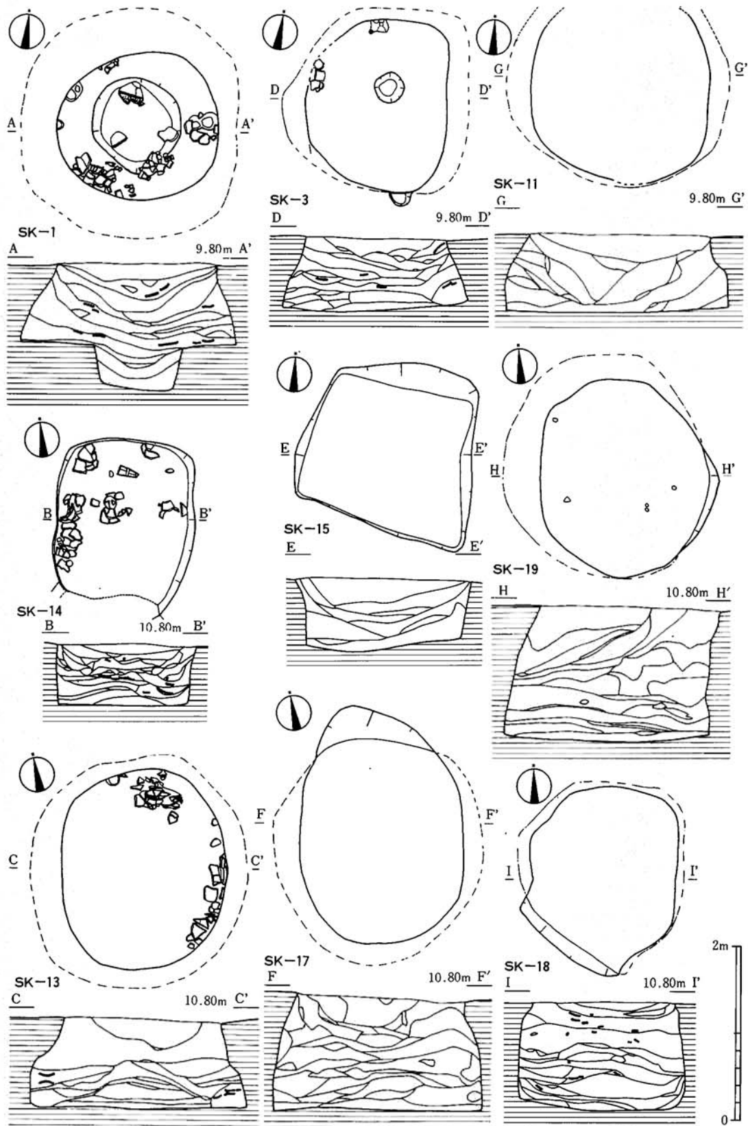
△貯蔵用竪穴実測図
