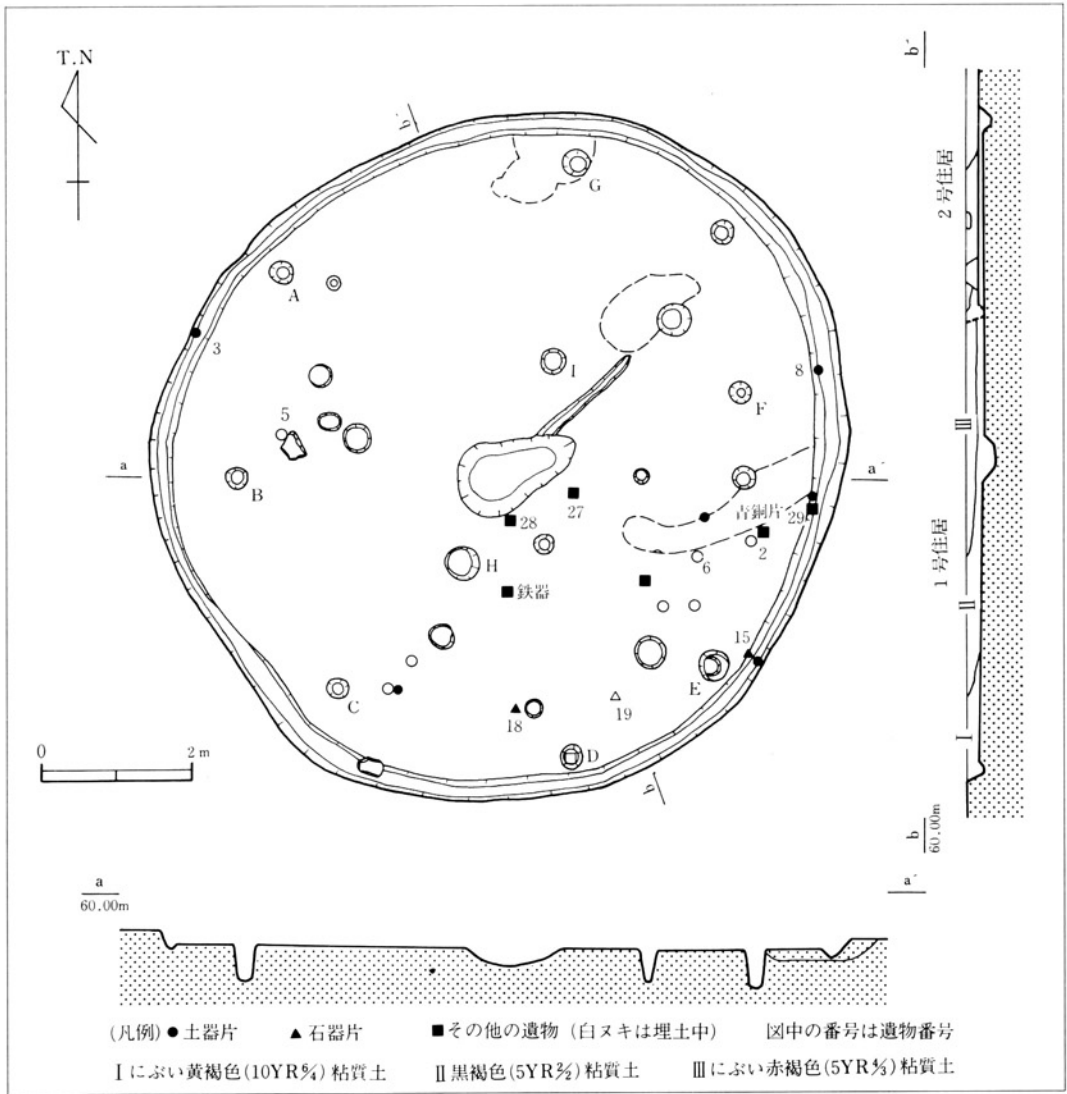
▲ 1号住居実測図
