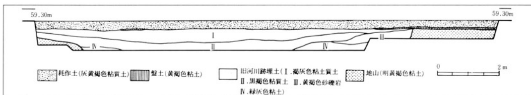
旧河川跡土層断面実測図
