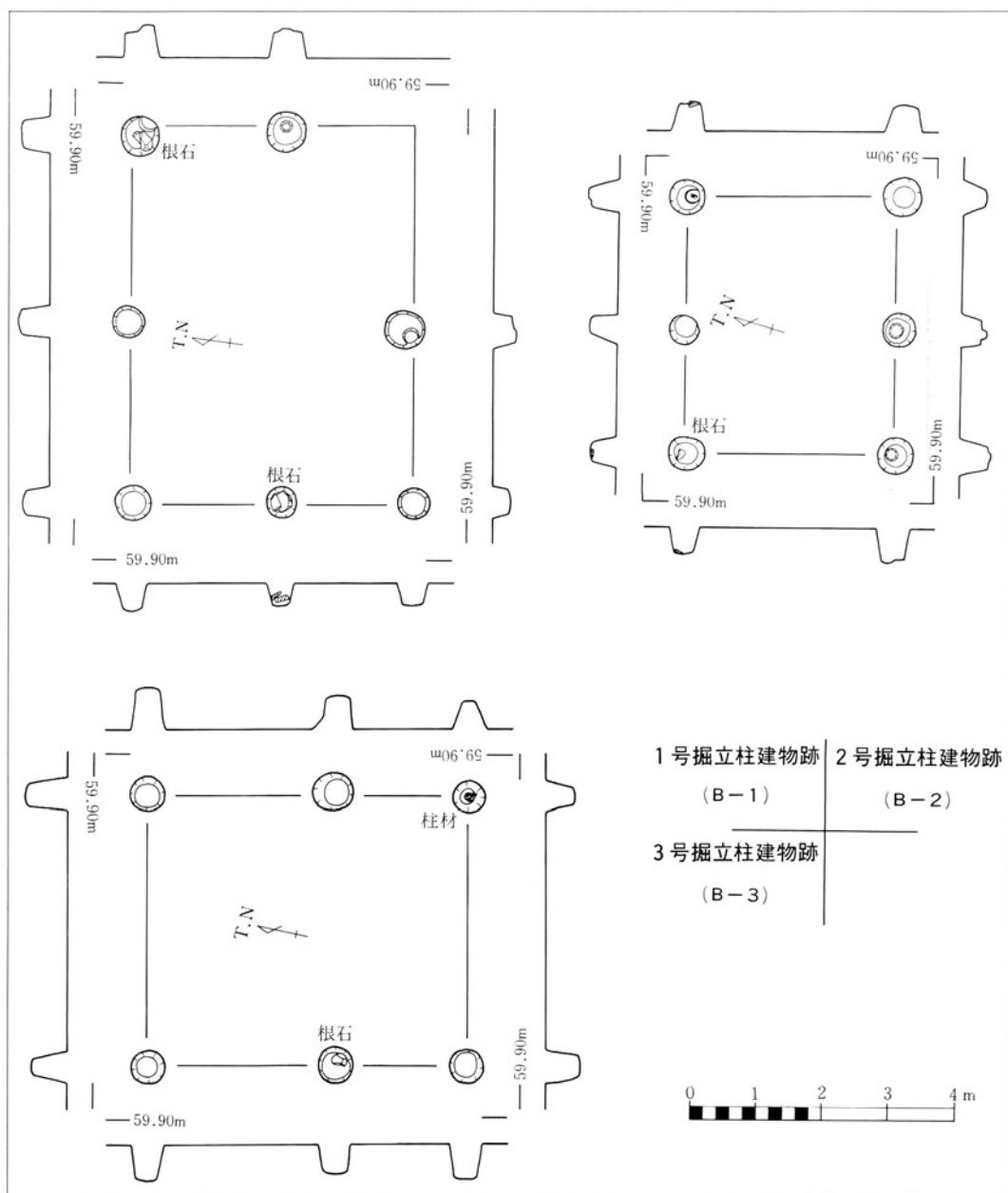
掘立柱建物実測図
