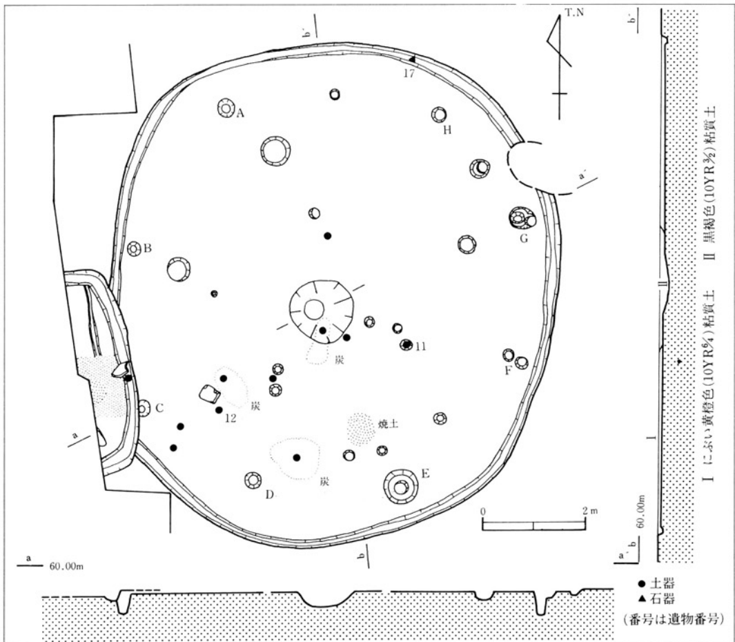
4号・7号 住居実測図
