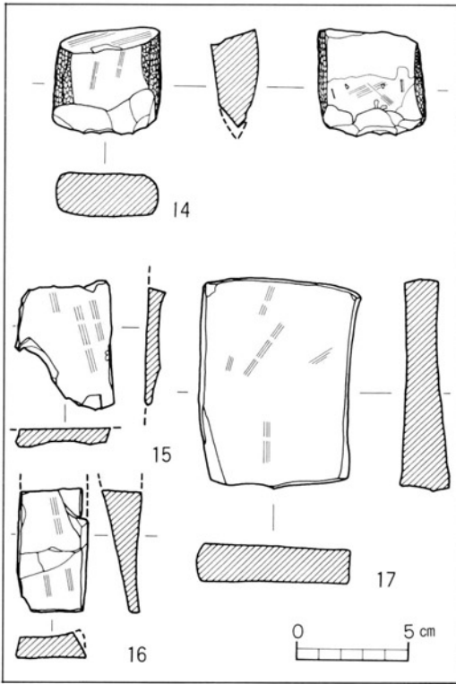
石斧・砥石実測図
