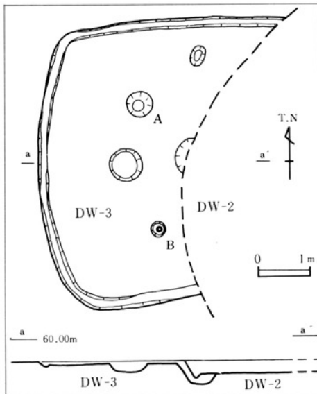
◀ 3号住居実測図
