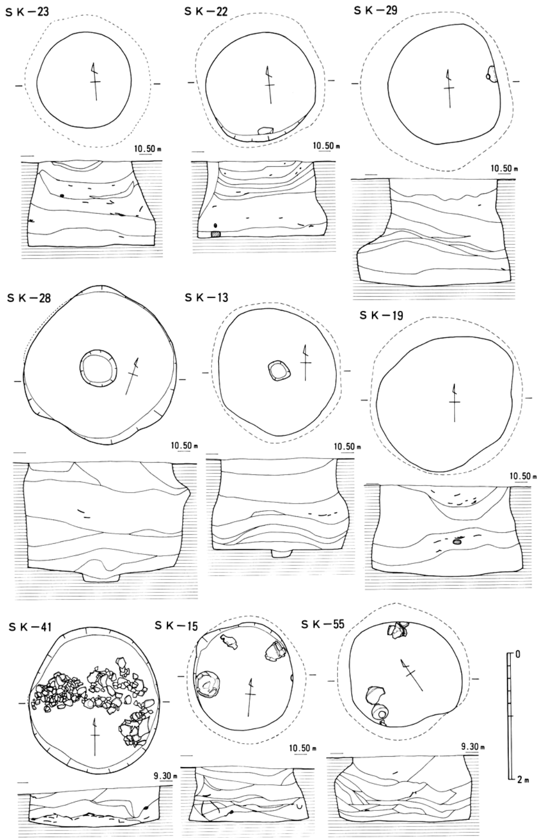
第8図 貯蔵用竪穴実測図(1)
