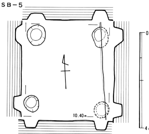
第7図 掘立柱建物SB-4・SB-5実測図
