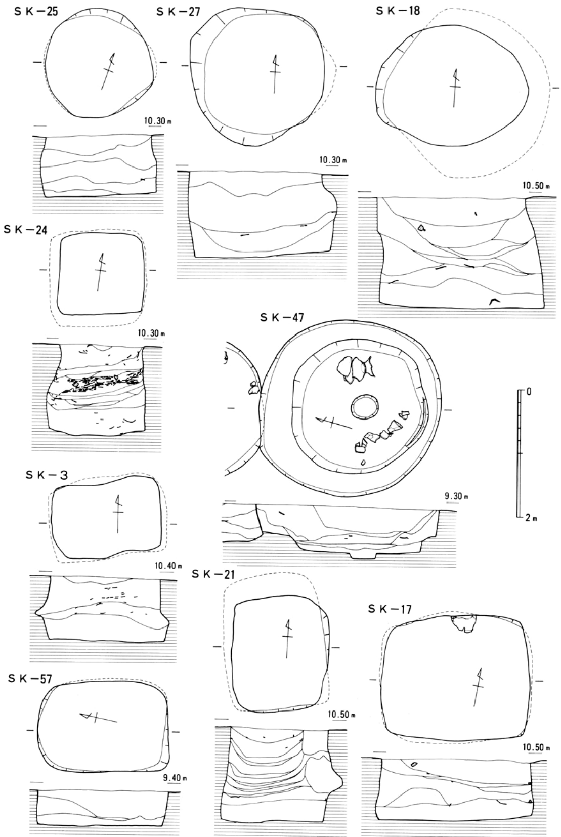
第9図 貯蔵用竪穴実測図(2)
