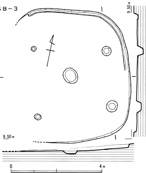
第6図 堅穴住居SB-1・SB-3実測図
