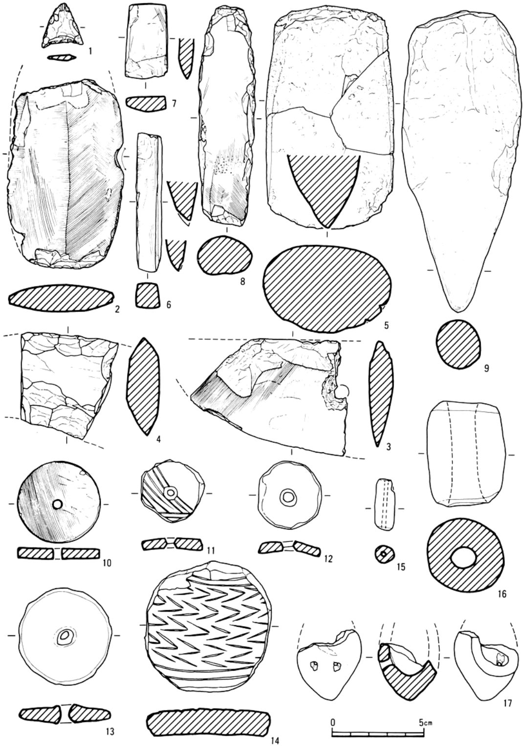
第15図 石器・土製品実測図
