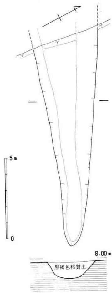
第10図 溝 S D - 1 実測図
