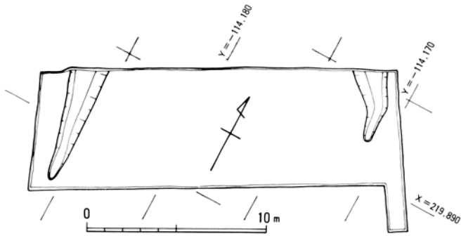
第4図 V地区北半部遺構配置図
