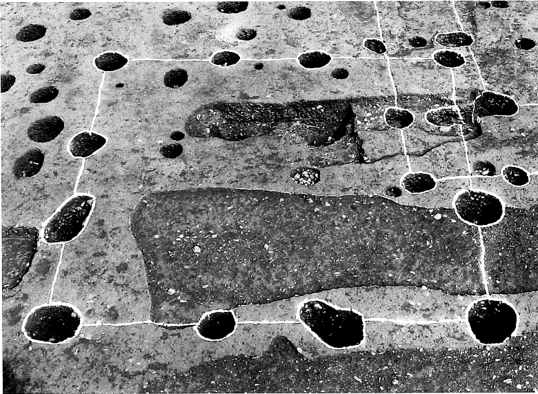
第36号掘立柱建物跡
