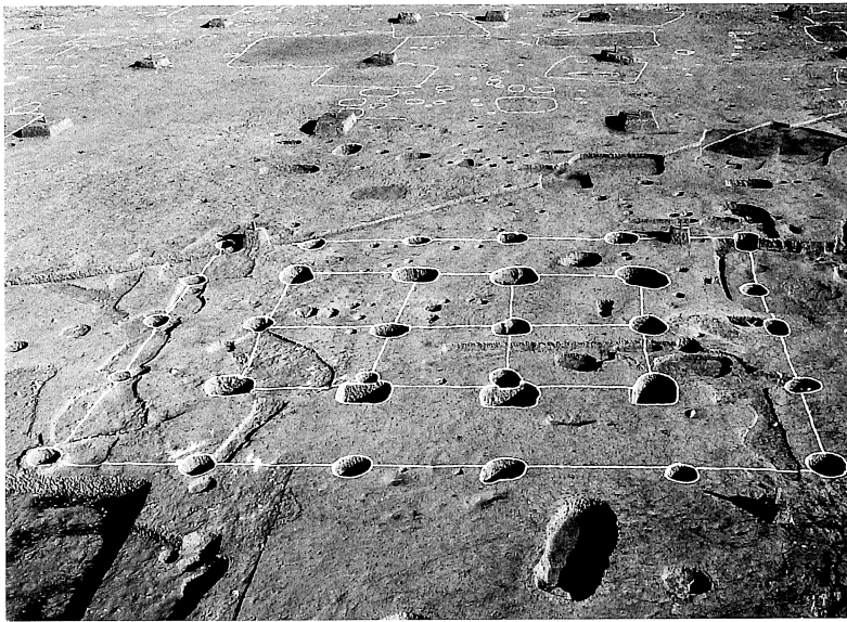
第42号掘立柱建物跡
