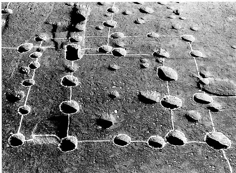
第44号掘立柱建物跡
