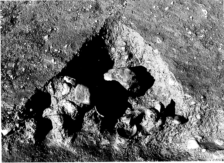
第202号住居跡カマド
