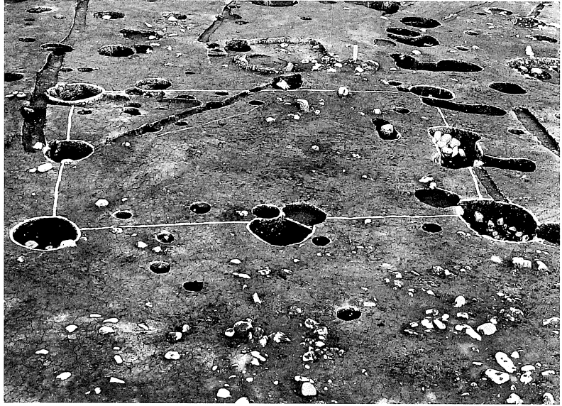
第38号掘立柱建物跡
