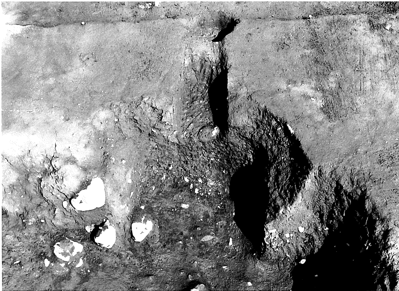
第55・56号住居跡カマド
