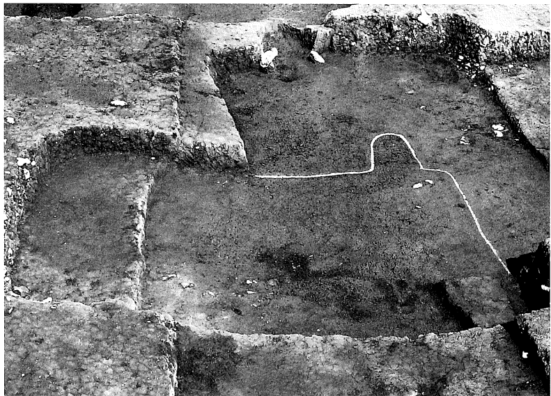
第106・109号住居跡
