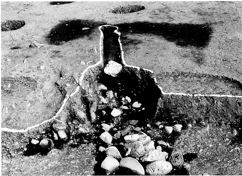
第100号住居跡カマド
