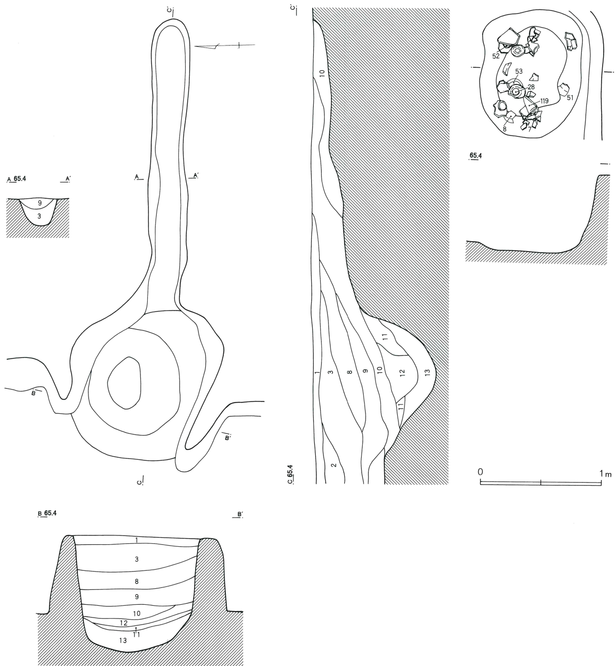
第390図 第223号住居跡カマド・貯蔵穴
