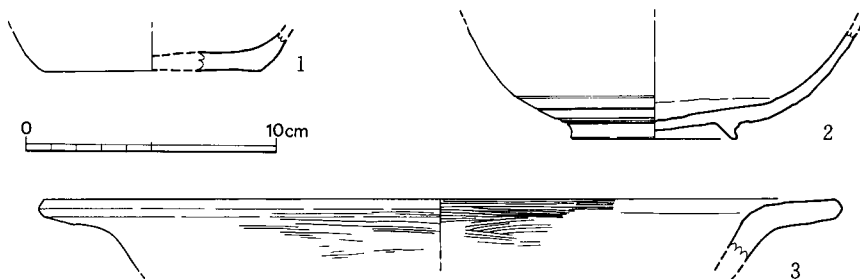
第 10 図 34号土塚出土土器実測図 (1/3)
