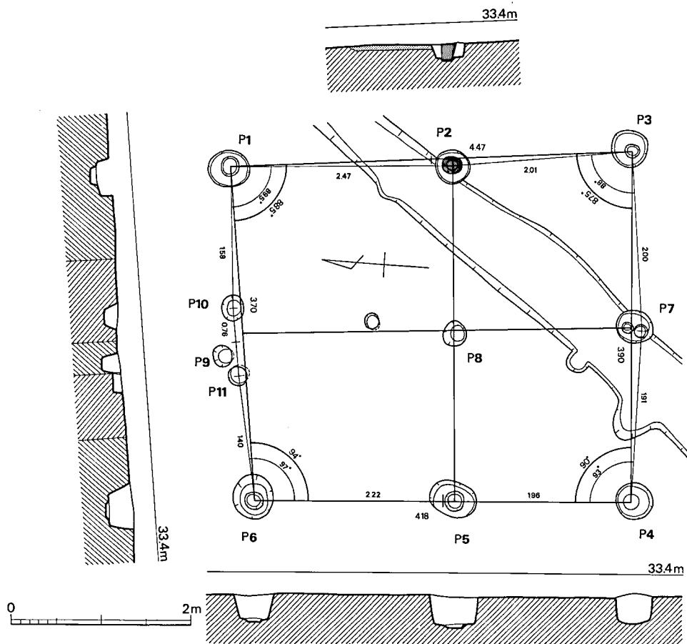
第 17 図 21号掘立柱建物実測図 (1/60)
