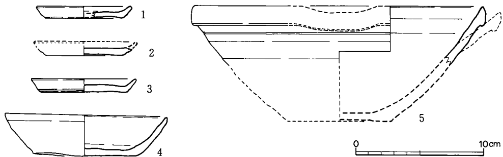
第 9 図 32・33号土塚出土土器実測図 (1/3)
