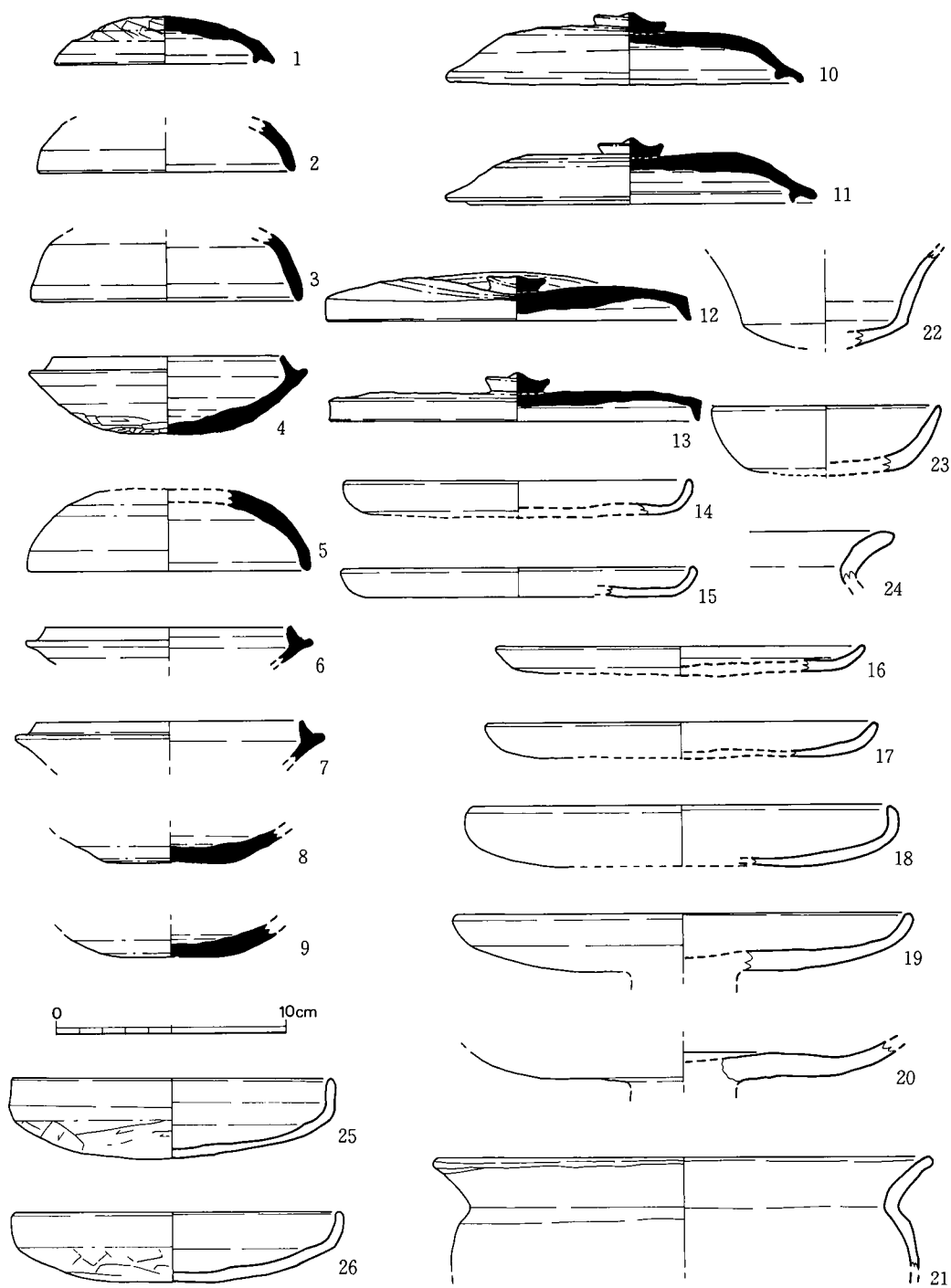
第 31 图 22号溝状遺構出土土器実測図 (1/3)
