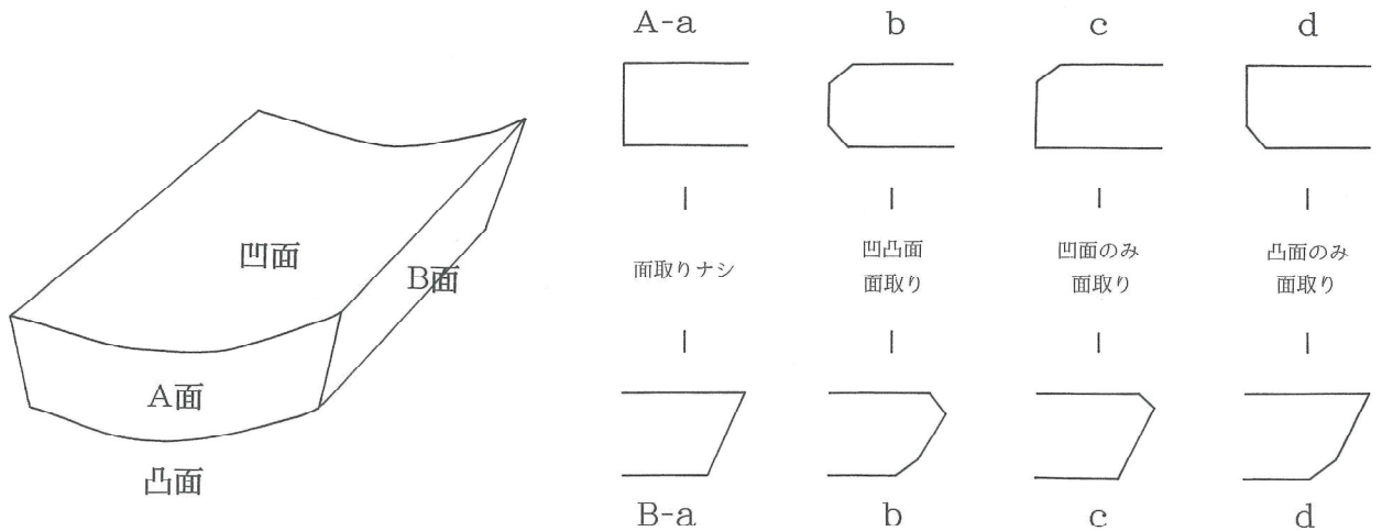
図14 平瓦模式図
