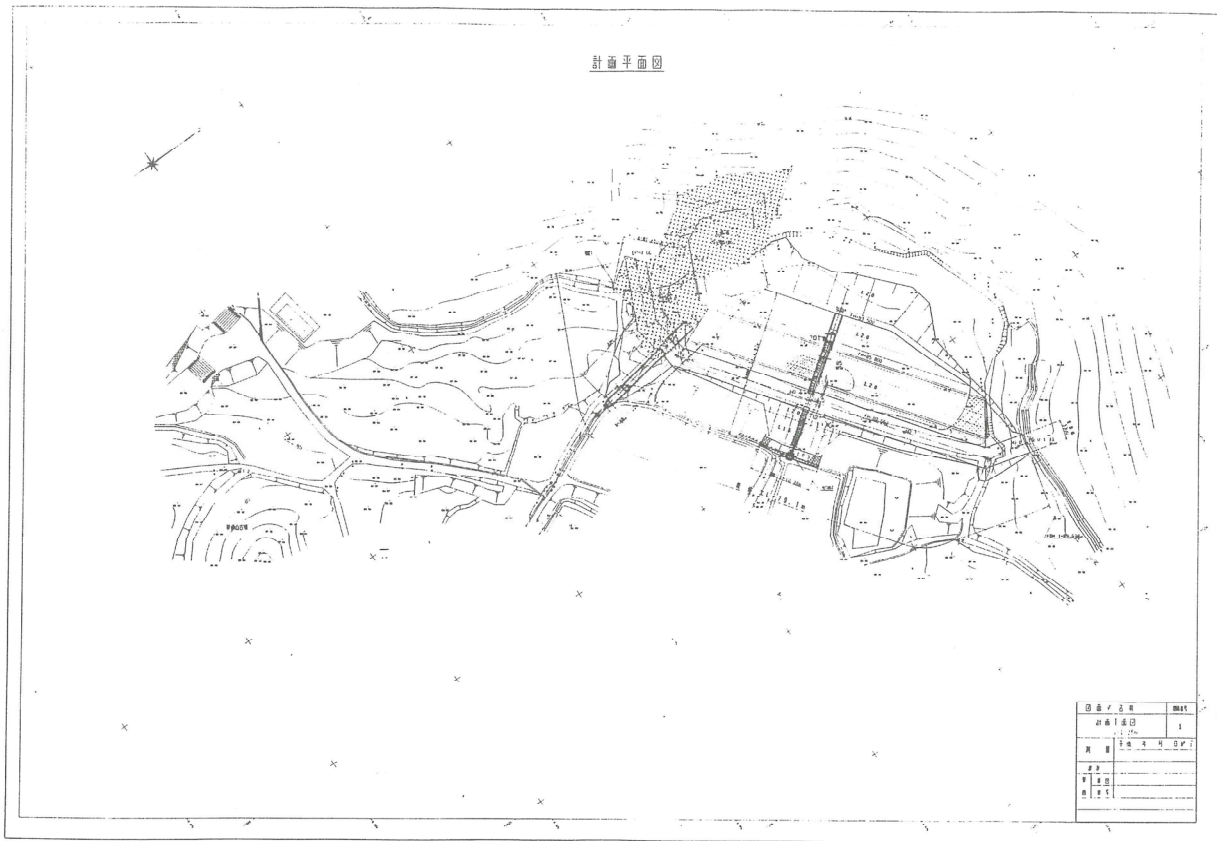
図6 土取り場配置図
