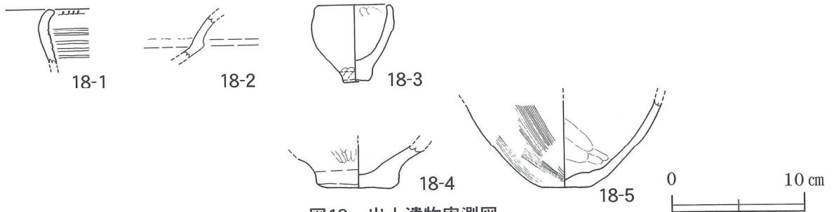
図18 出土遺物実測図
