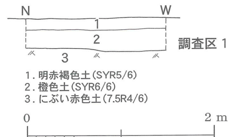
図14 土層図
