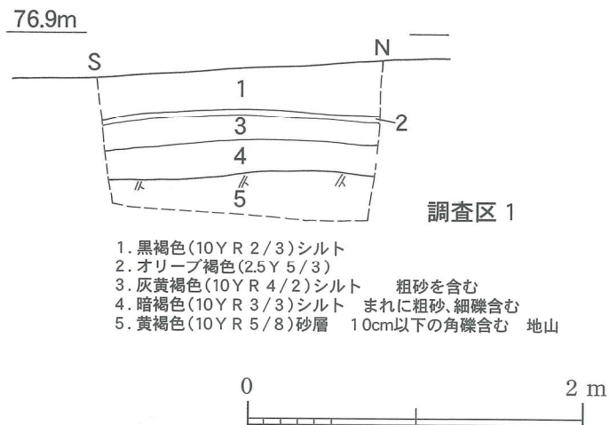
図37 土層図
