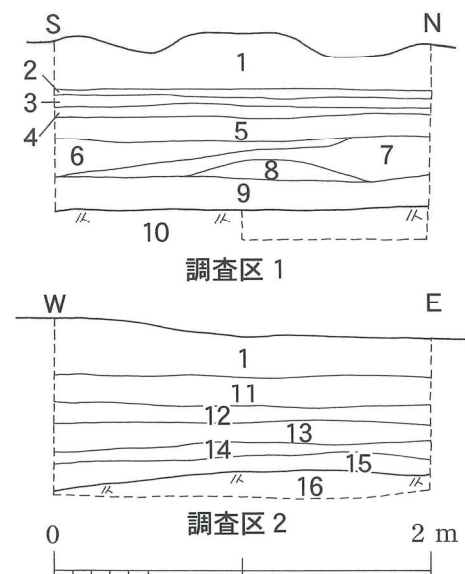
図3 土層図
