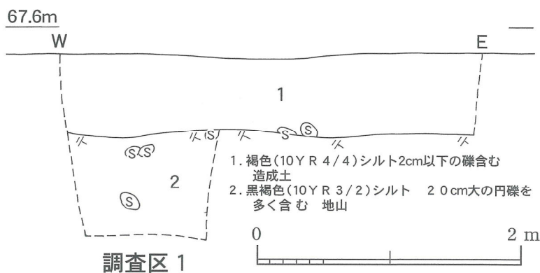
図31 土層図
