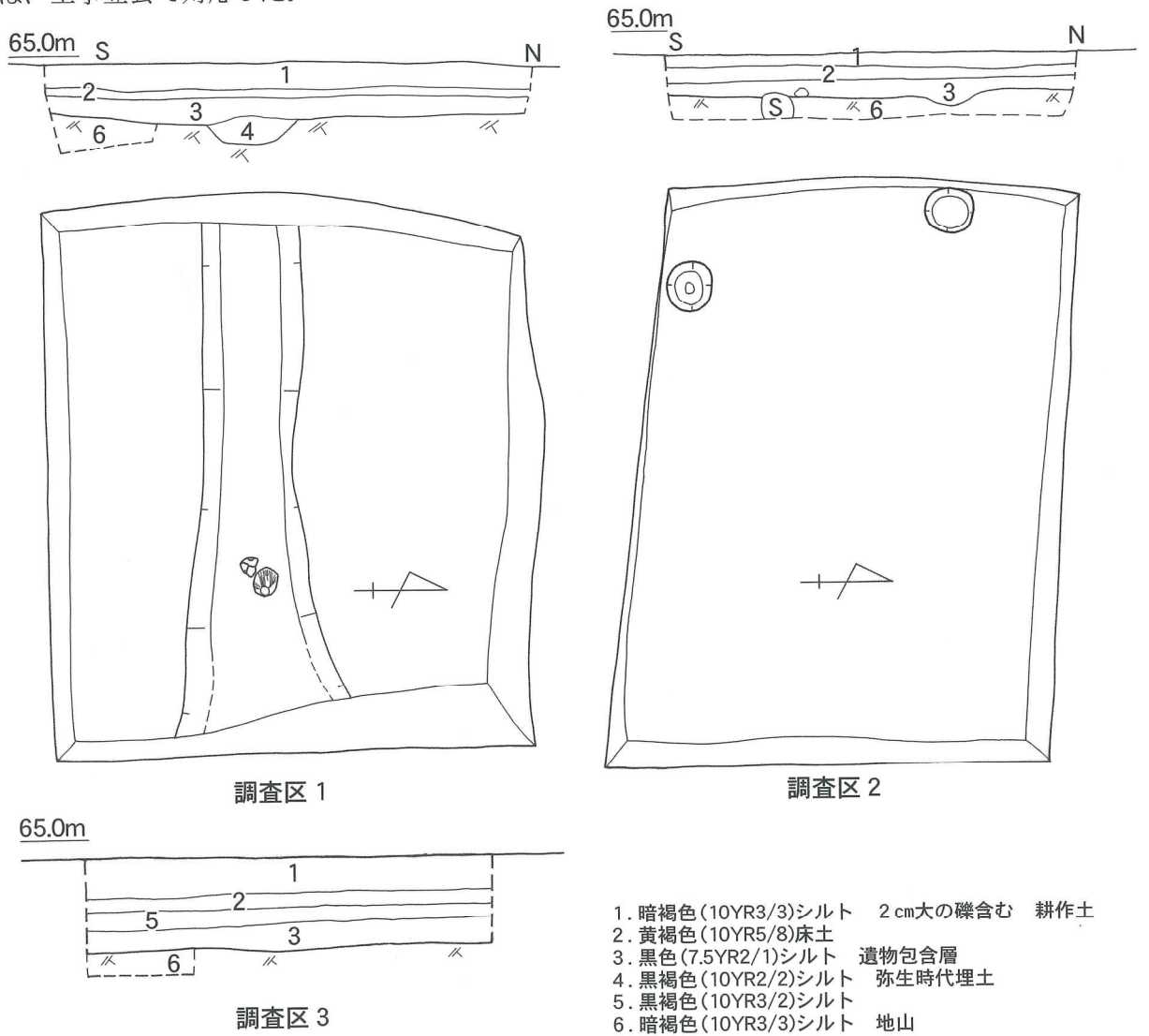
図17 土層図
