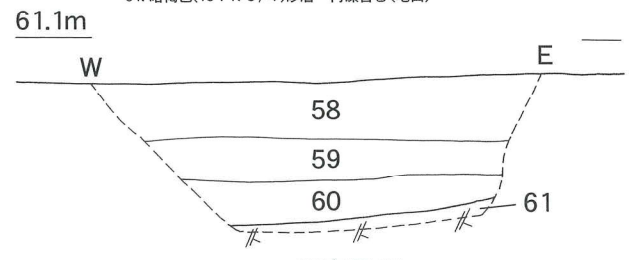
図41 土層図
