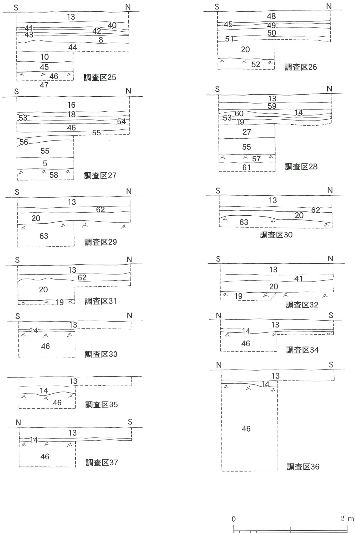
图9 土層図
