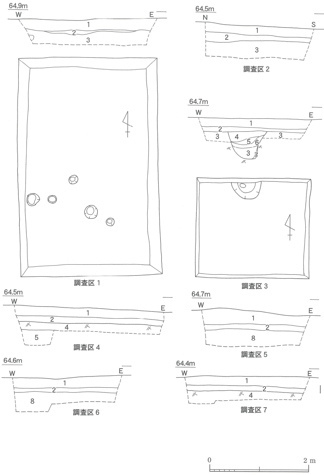
図25 土層図
