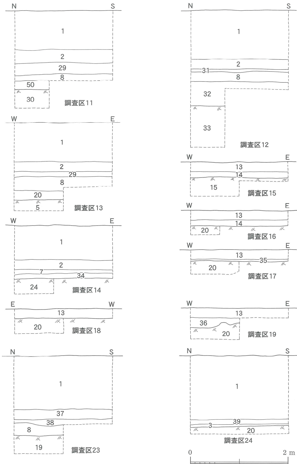
图 8 土層図
