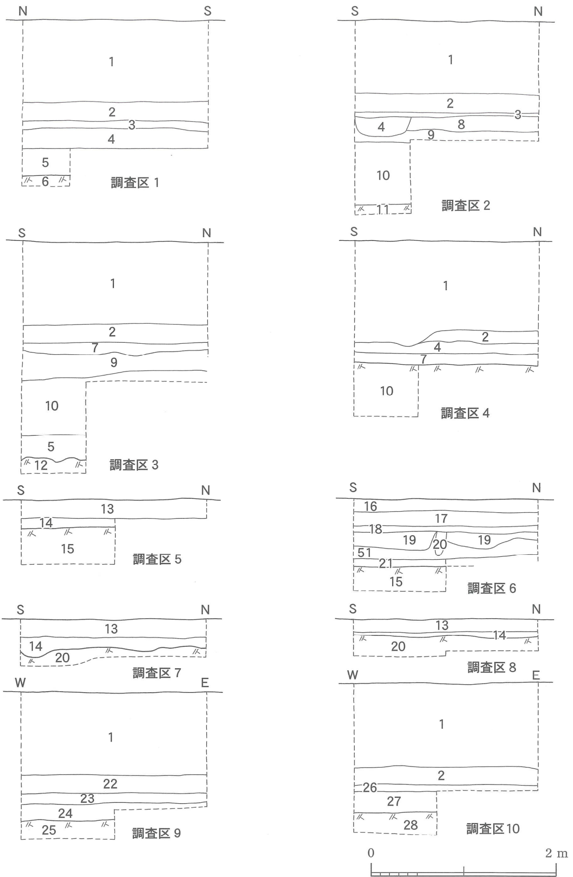
图7 土層図
