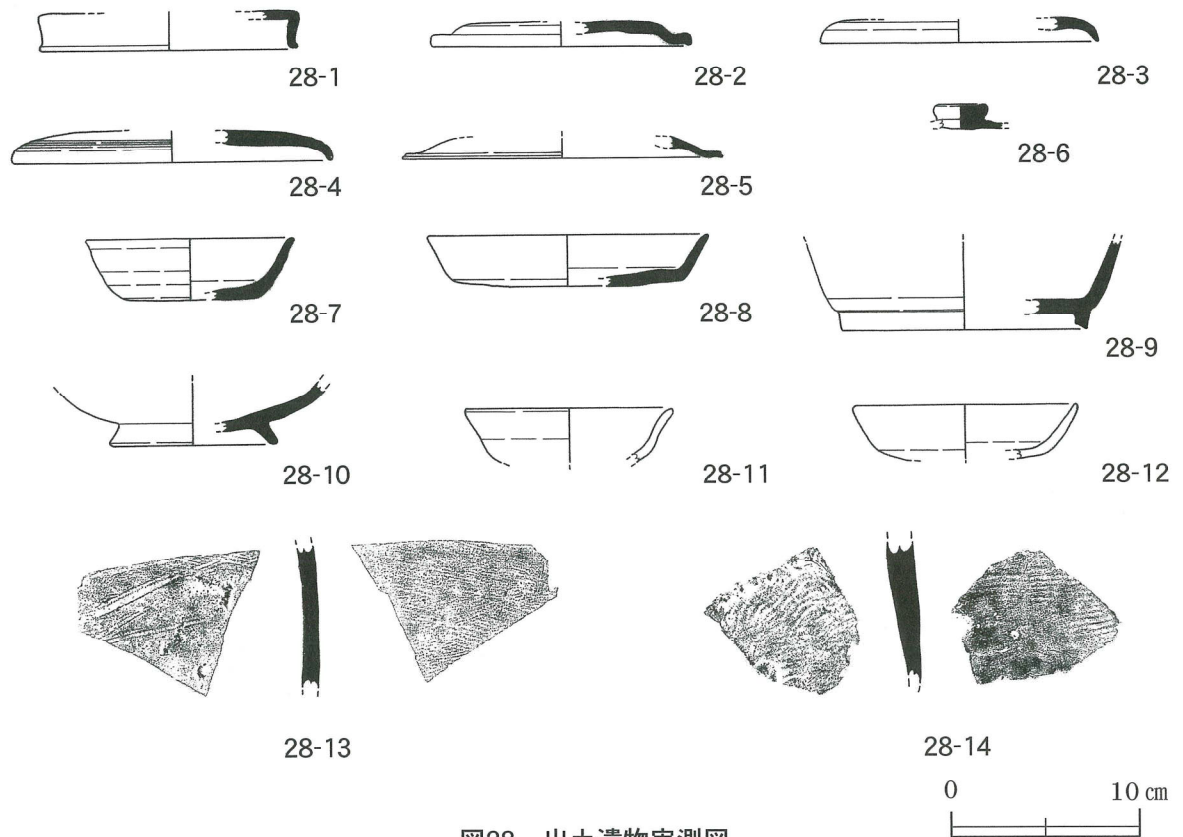
図28 出土遺物実測図
