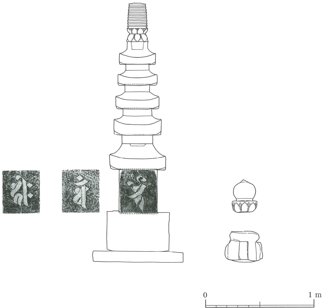
图45 石造五重塔 实测图
