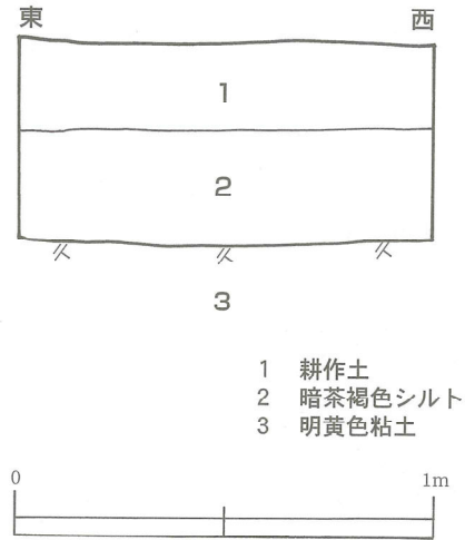
図18 土層図
