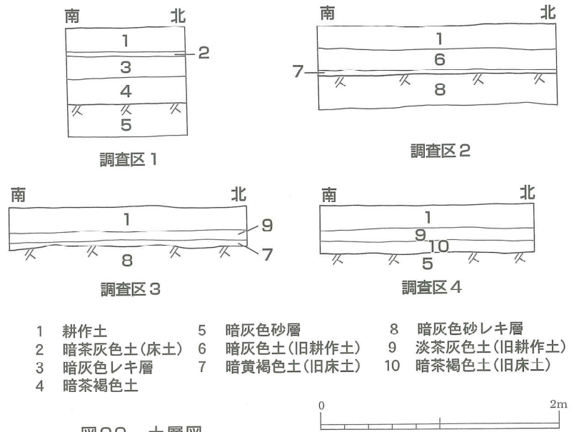
図29 土層図
