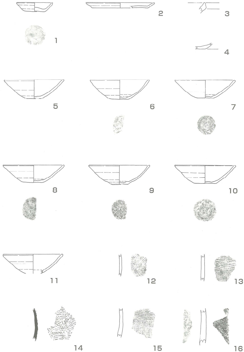
図56 出土遺物
