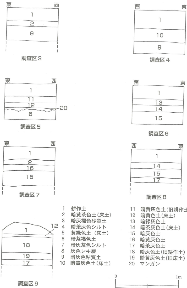
図44 土層図
