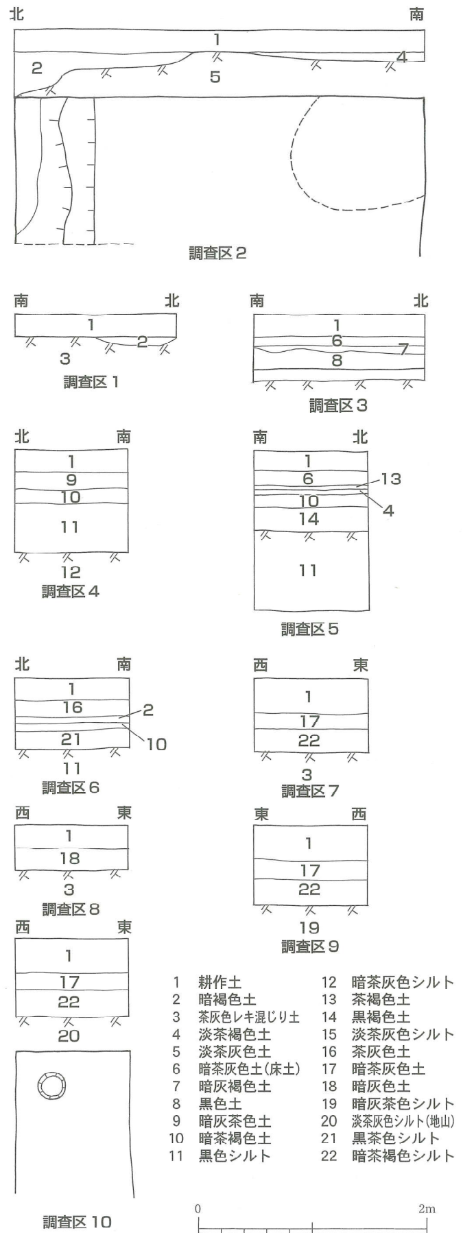
図10 土層図
