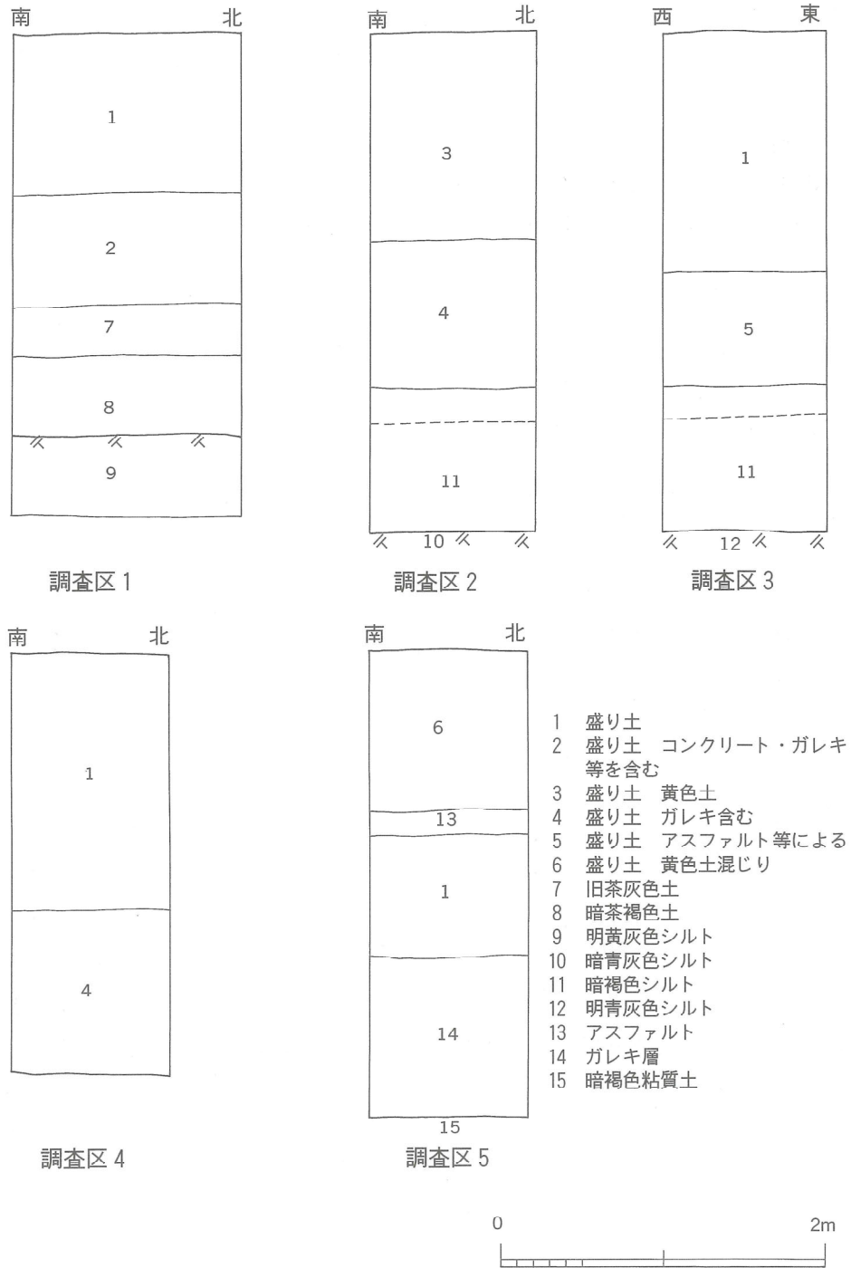
図 1 1 南田原中島地区土層図
