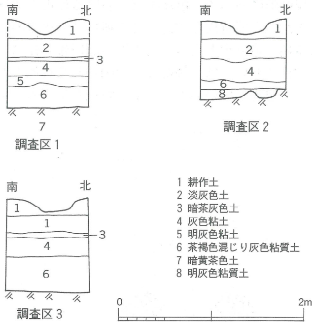
図 3 2 調査区土層図
