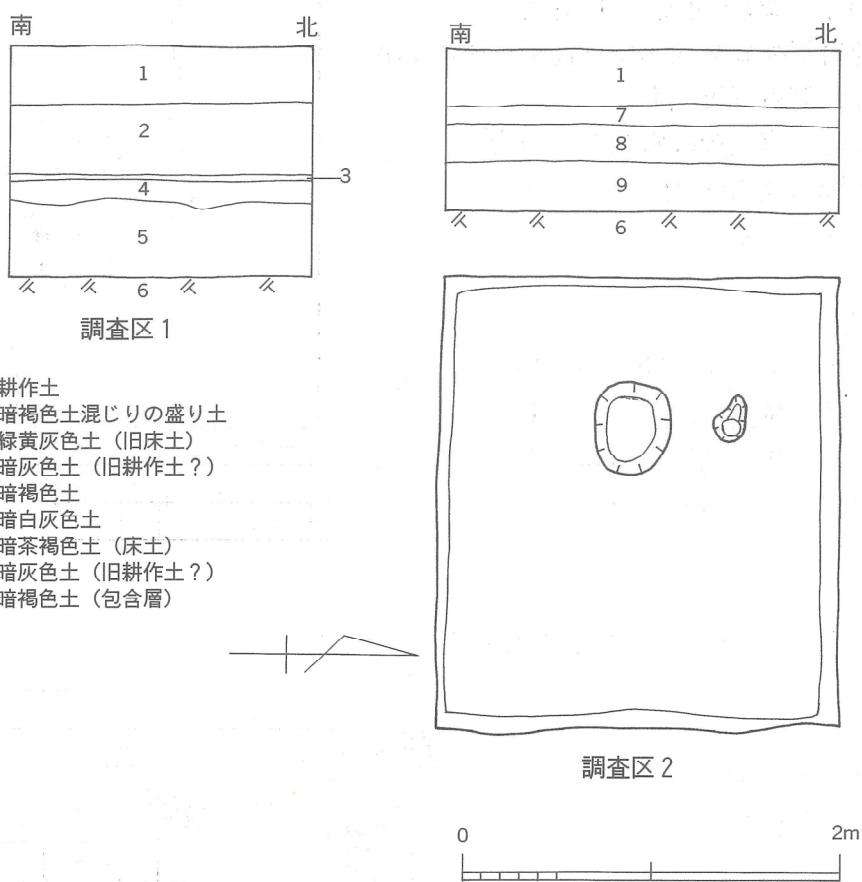
図24 西広畑遺跡土層図・平面図
