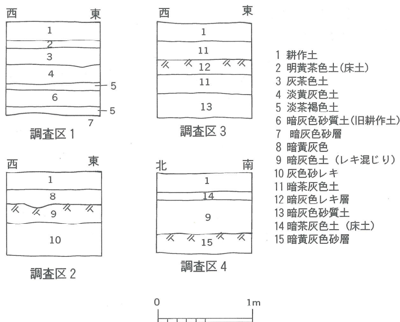
図4.3 調査区土層図
