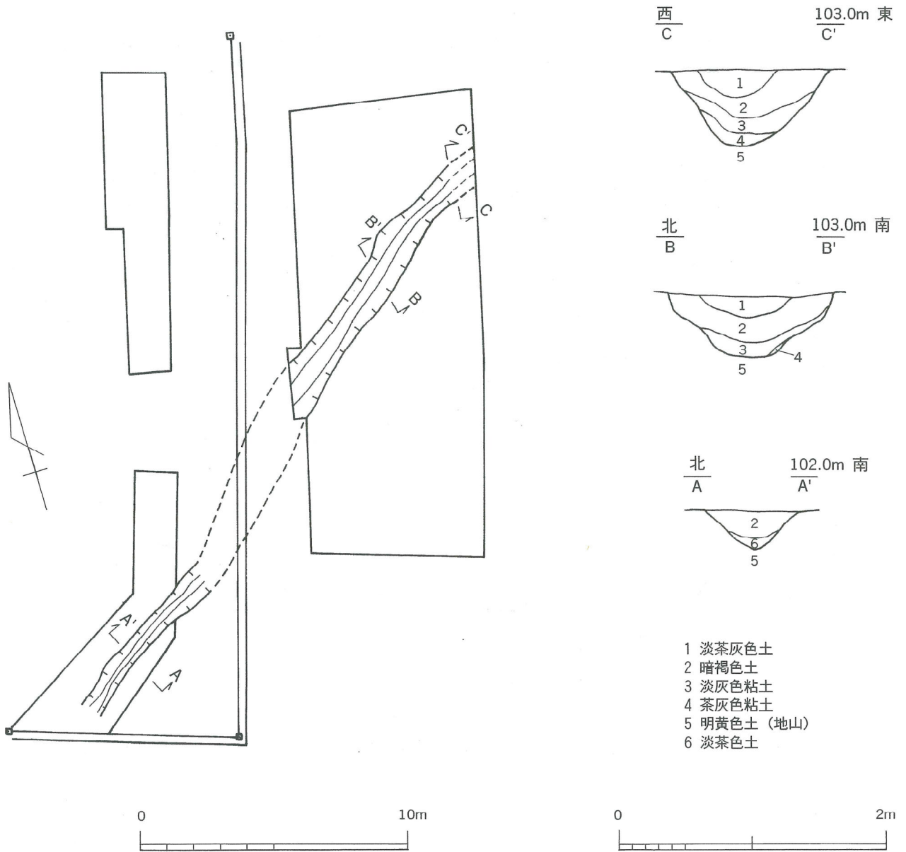
図28 遺構平面図・土層図
