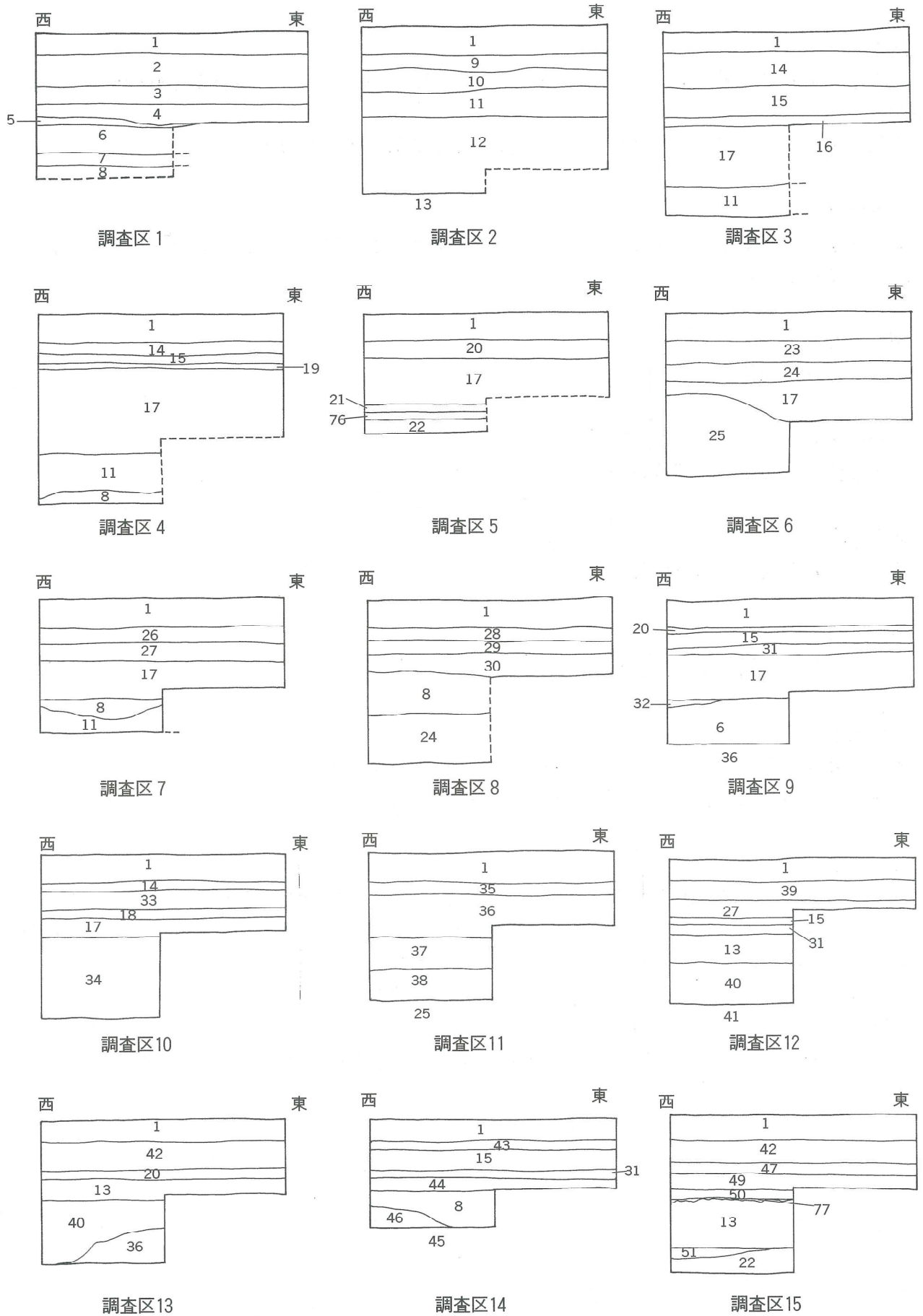
図 17 山崎地区調査区土層図
