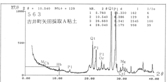
第21図 県内各地採取の粘土のX線回析図(第四紀分析)
