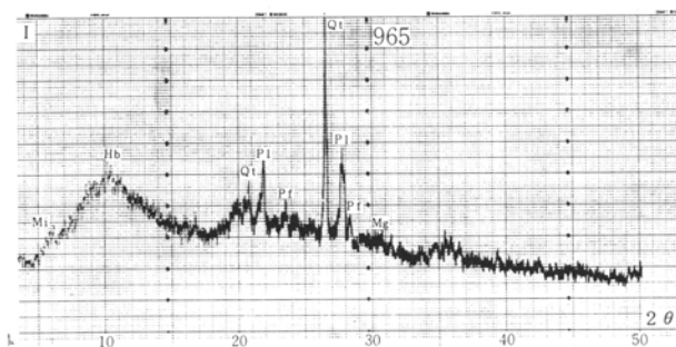
第17図 工試分析・土器（土師器）・粘土X線回折図
