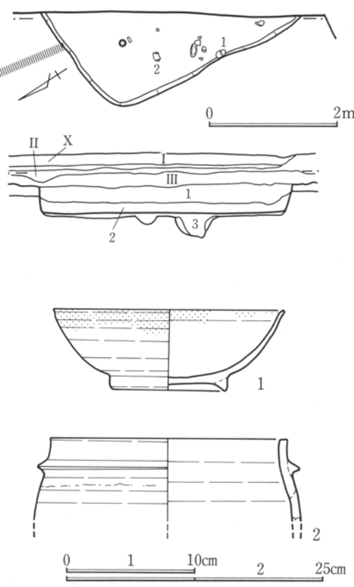
第3図 14号住居跡平面図・出土遺物図
