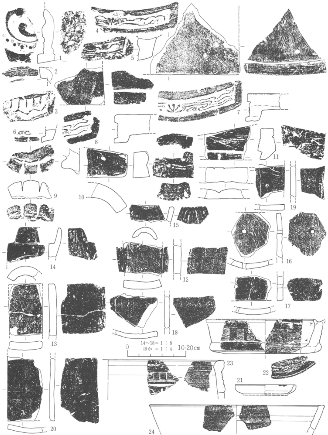
1・2 鍍瓦、3～8 字瓦、9 飾部瓦、10・11 道具瓦、12・13 同熨斗瓦、14・15 男瓦、16・17 女瓦（釘穴あり）、18～20 女瓦、21 土質土器皿。22 軟質陶器鉢（中性焰）、23 軟質陶器火鉢（燻焼）、24 軟質陶器内耳鍋形。22・23 乗附か、21・24 胎土製作地不明。3 は14世紀前半頃、4～8 は14～15世紀頃。12・16～18 は13世紀前半頃。21 は13世紀頃。22・23 は14世紀頃。14 は15・16世紀頃。中世遺物は鎌倉時代から中世後半まで通して存在し、その法燈は現在に続く。
