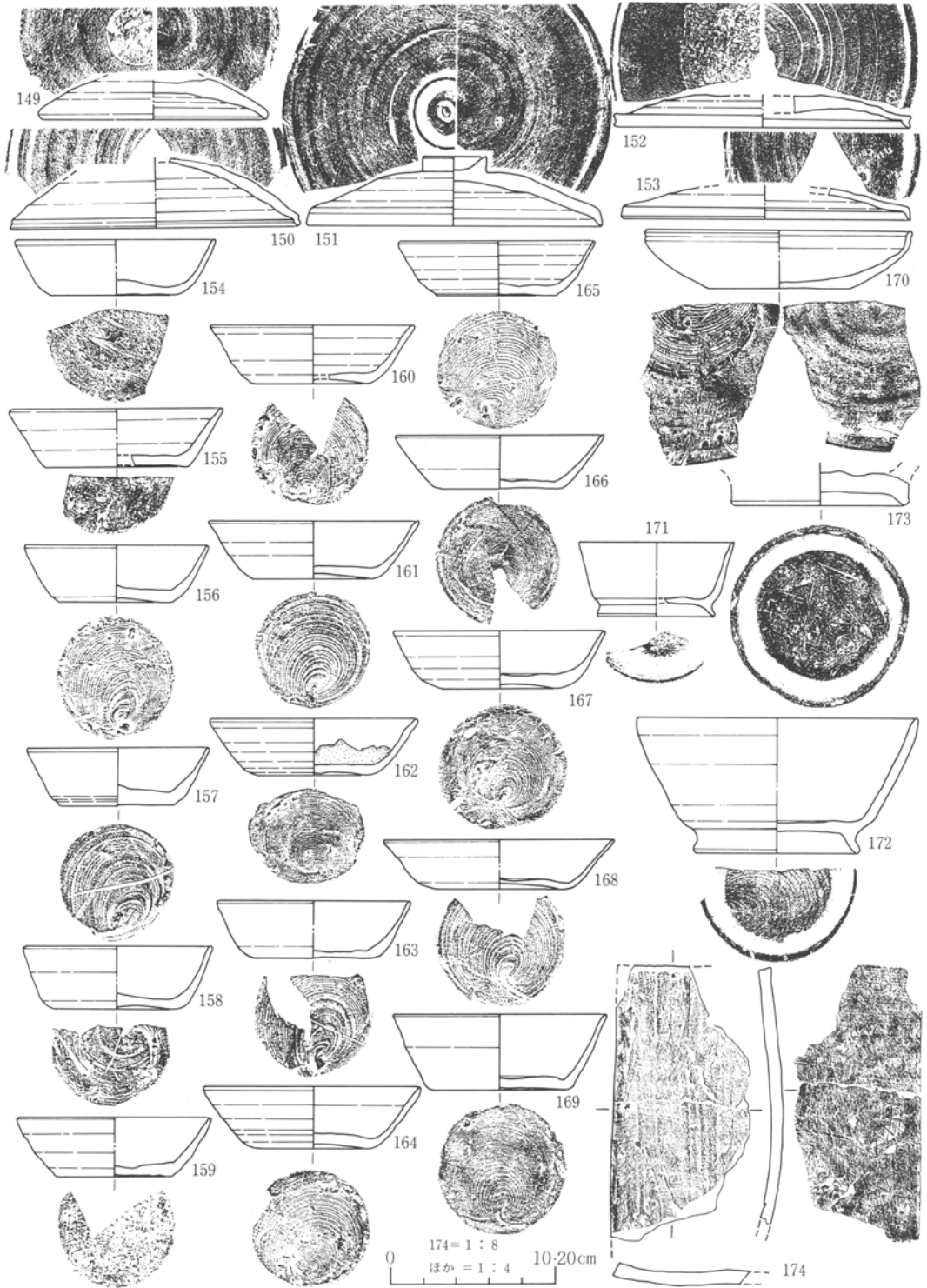
149～153 須恵器蓋、154～169同環、170同異形環、171同小形碗、172同碗、173同不明、174女瓦。154・155は底面手持篋削、環類の底面切りはなしに、轆轤右・左回転の両例があり注意を要す。174に斜格子、寄木圧痕あり桶巻作。
