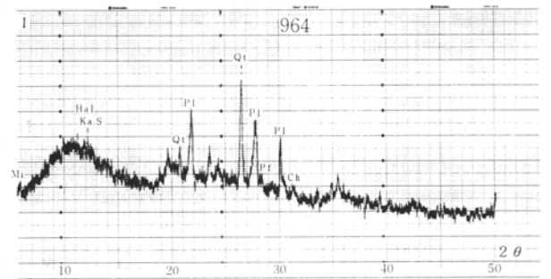
第17図 工試分析・土器（土師器）・粘土X線回折図
