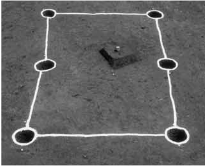
1号掘立柱建物 (南)
