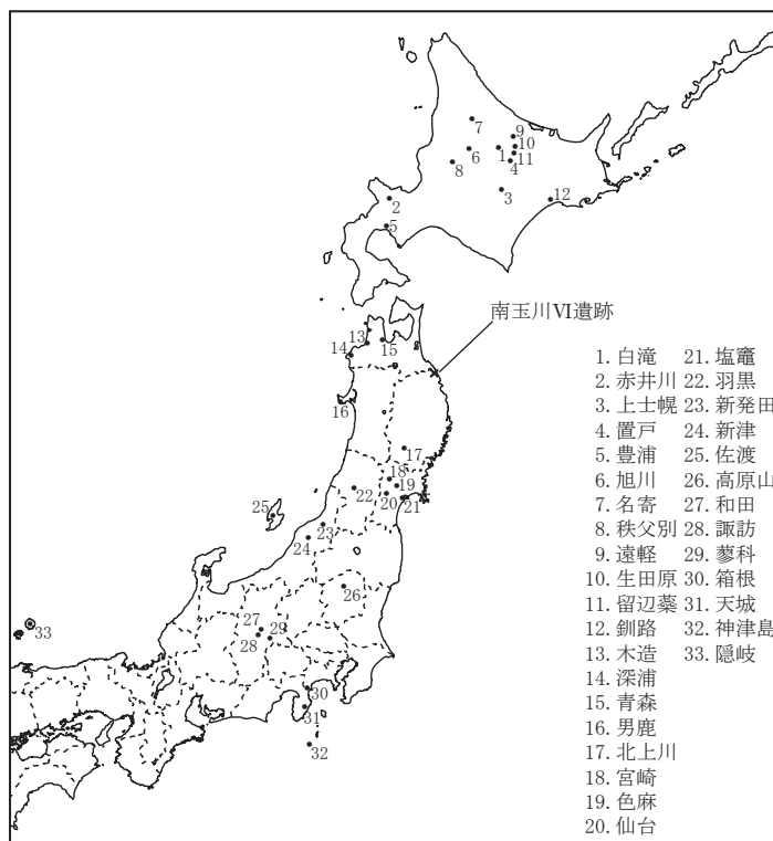
第C図 黒曜石産地分布図
