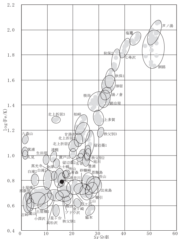
第 E 図 黒曜石産地推定判別図 (2)
