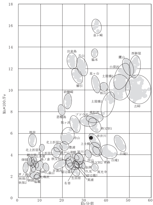
第 D 図 黒曜石産地推定判別図 (1)
