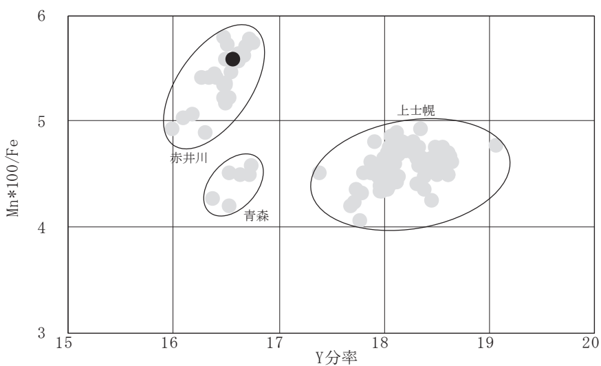
第 F 図 黒曜石産地推定判別図 (3)
