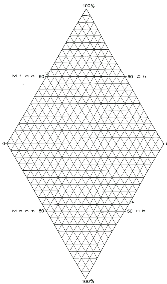
第4図 Mo-Ch, Mi-Hb菱角ダイヤグラム
