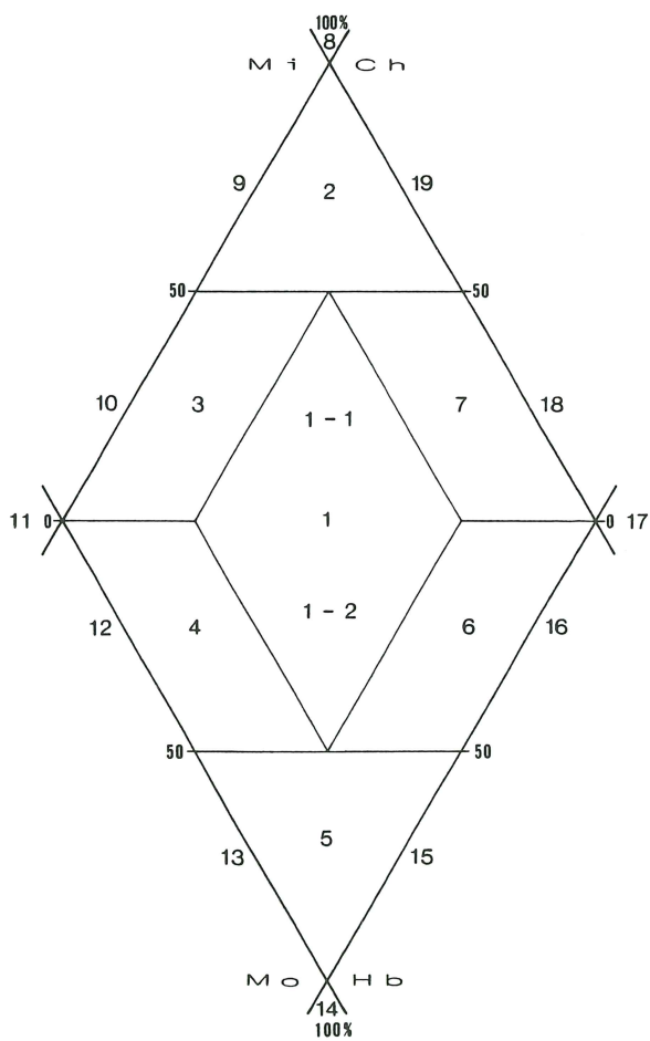
第2図 菱形ダイヤグラム位置分類図
