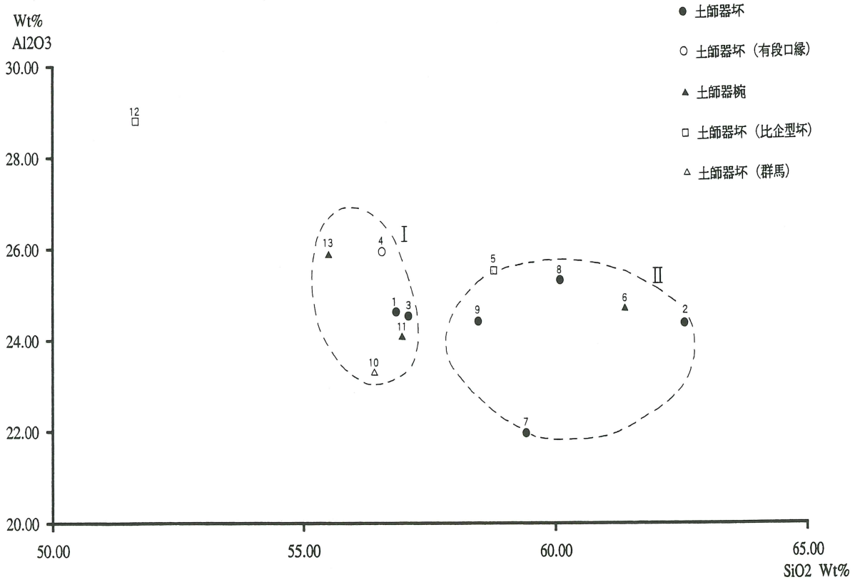
第6図 SiO 2 - Al 2 O 3 図
