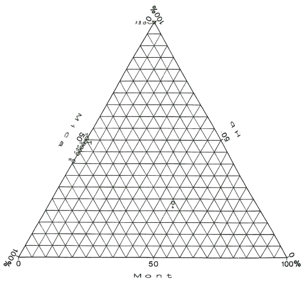
第3図 Mo-Mi-Hb三角ダイヤグラム
