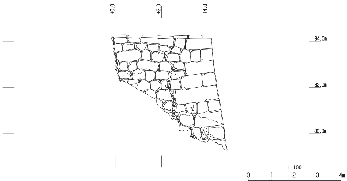
第2図 石垣立面图2
