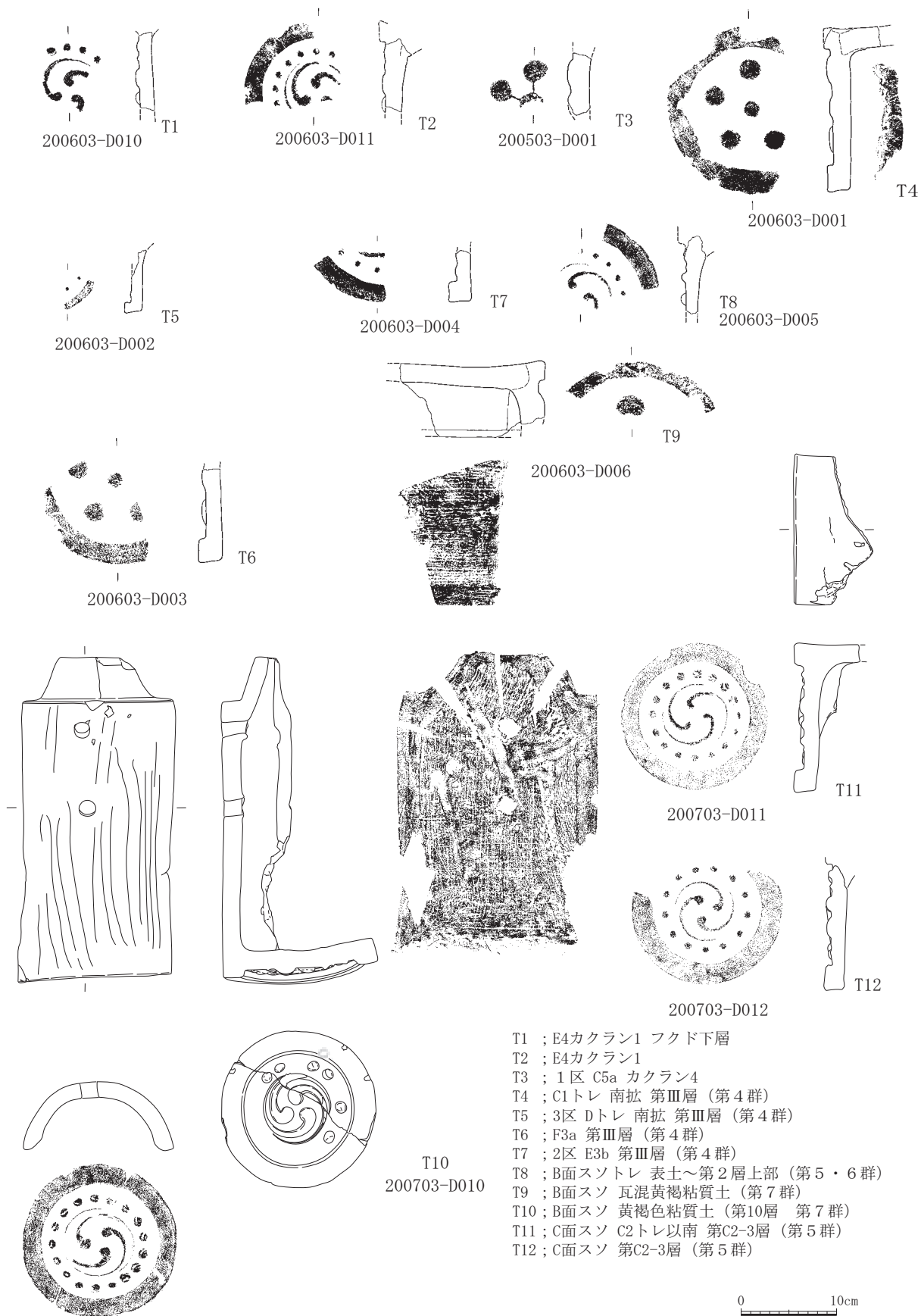
第146図 出土遺物実測図 瓦 1 (いぶし, S=1/6)
