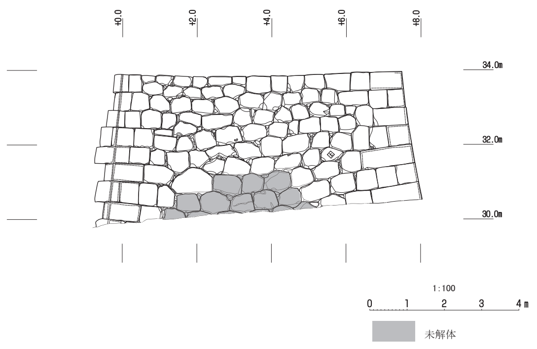
第198図 修復後石垣立面図 1
