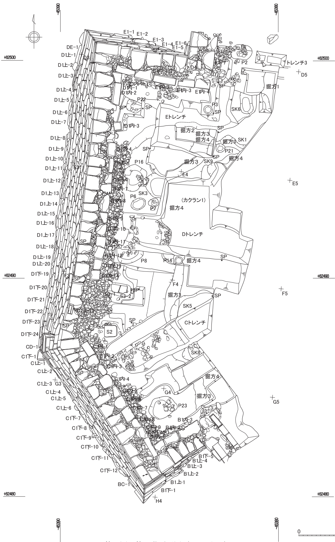
第26図 第1段平面図 (S=1/100)
