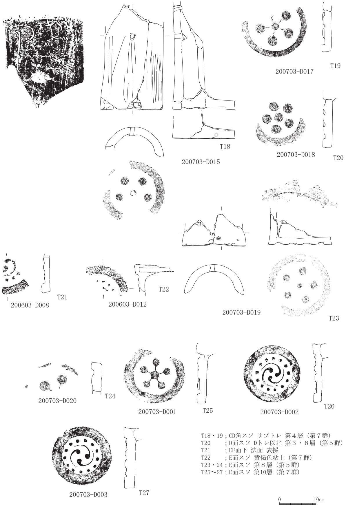
第148図 出土遺物実測図 瓦 3 (いぶし, S=1/6)
