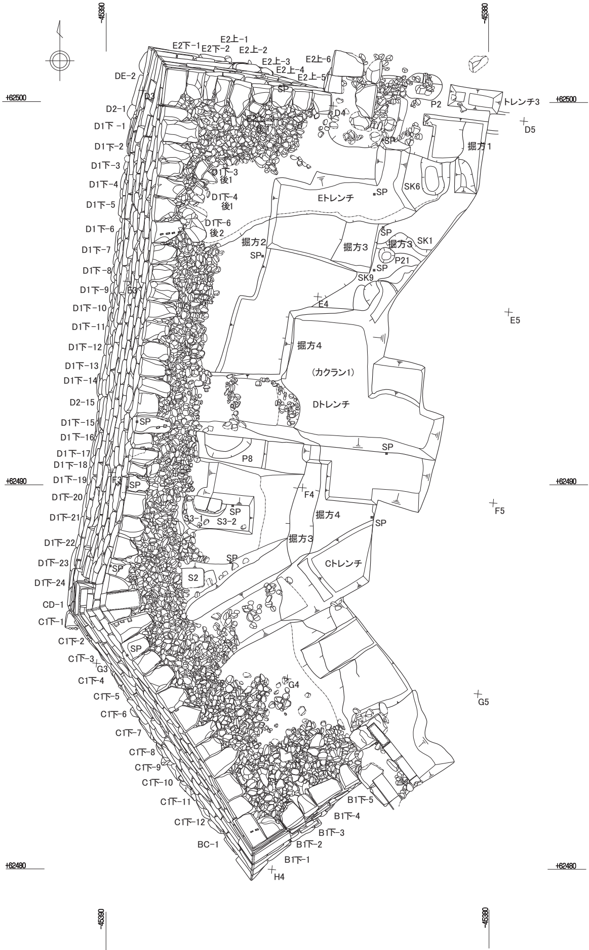
第28図 第2段平面図 (S=1/100)
