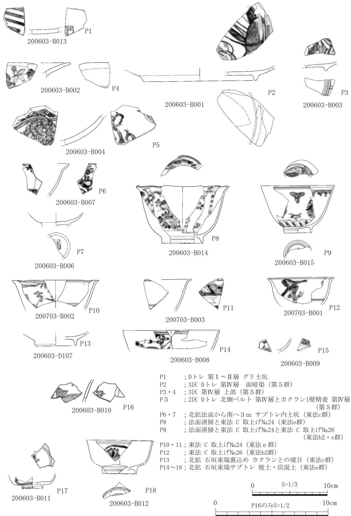
第170図 出土遺物実測図 陶磁器 1 (S=1/2、1/3)
