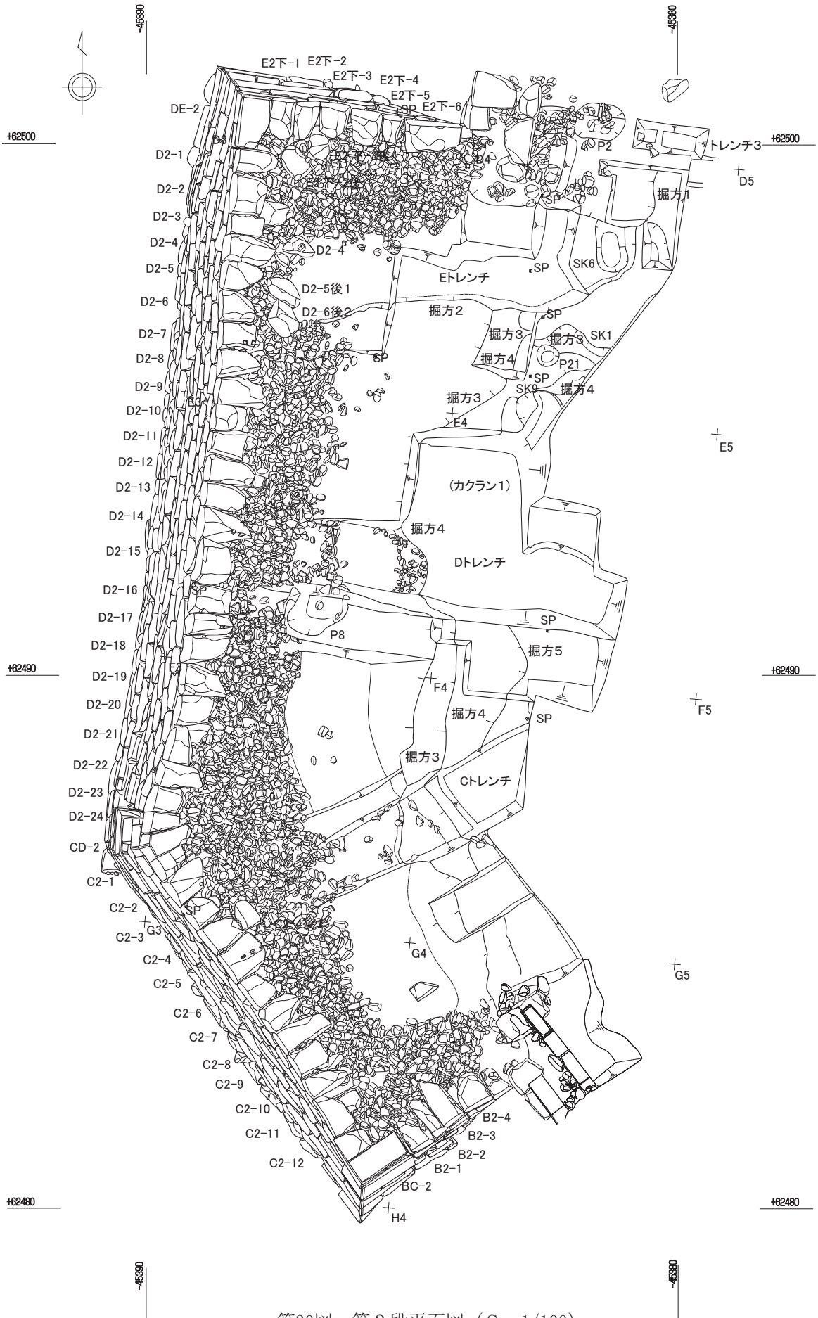
第30図 第3段平面図 (S = 1/100)
