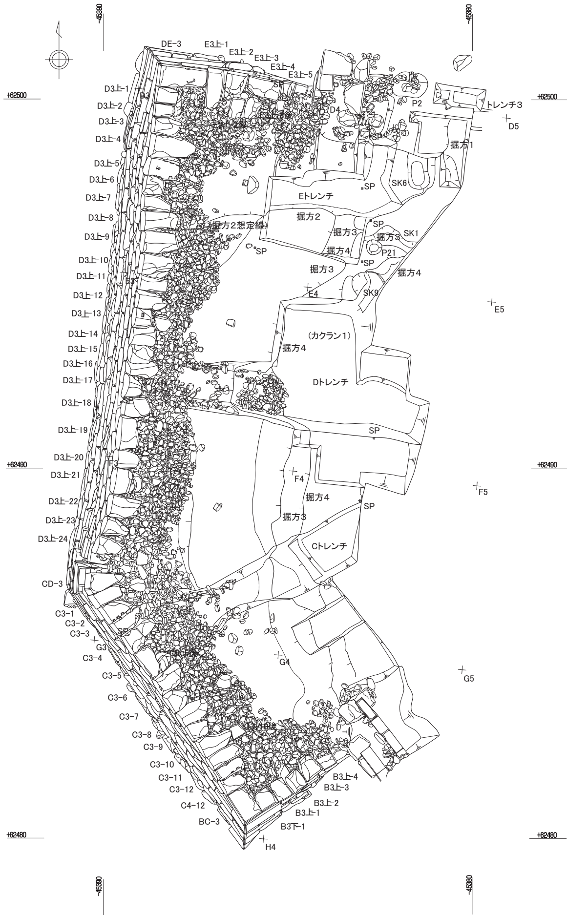
第32図 第4段平面図 (S = 1/100)
