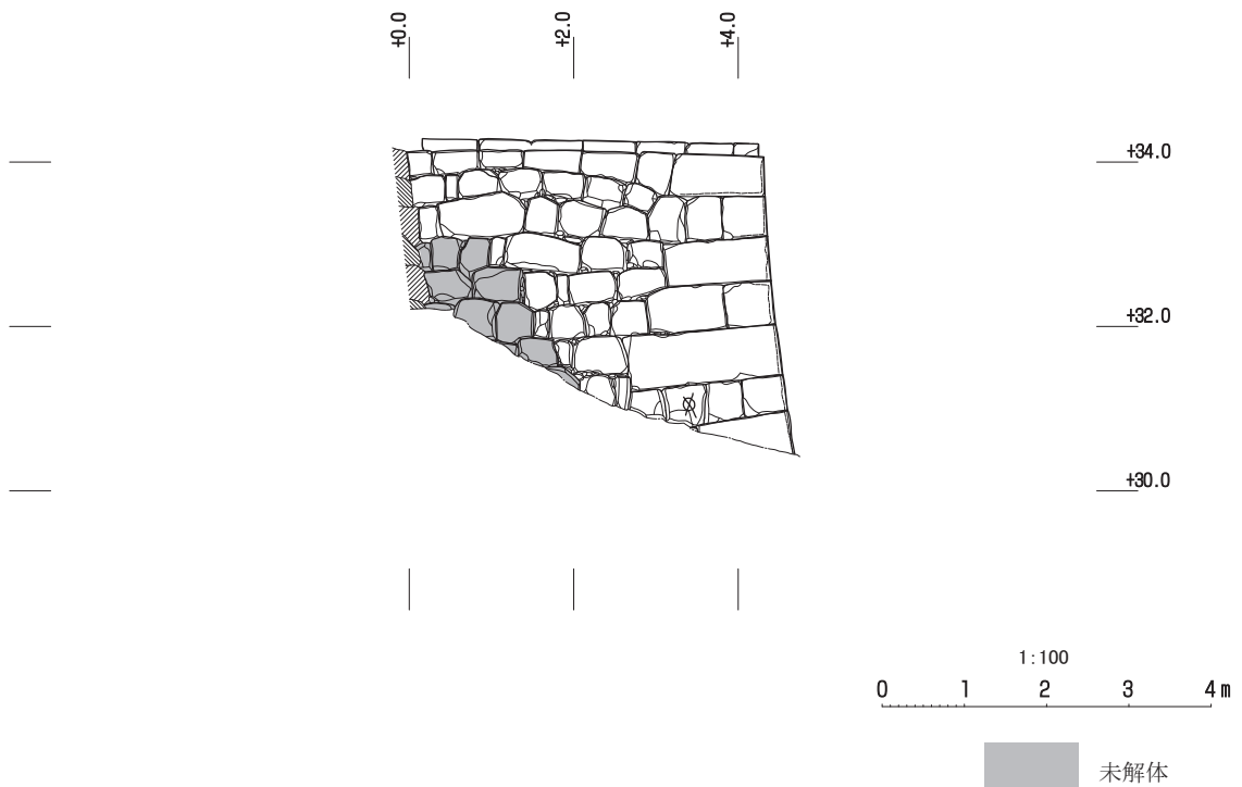
第199図 修復後石垣立面図 2
