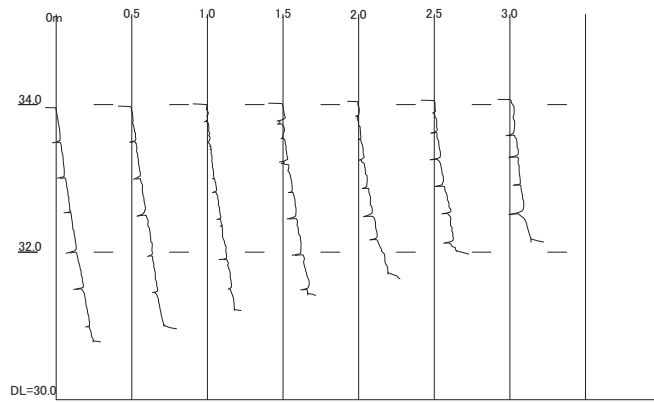
玉泉院丸南西石垣 解体修復後 断面図(垂直) (B面)
