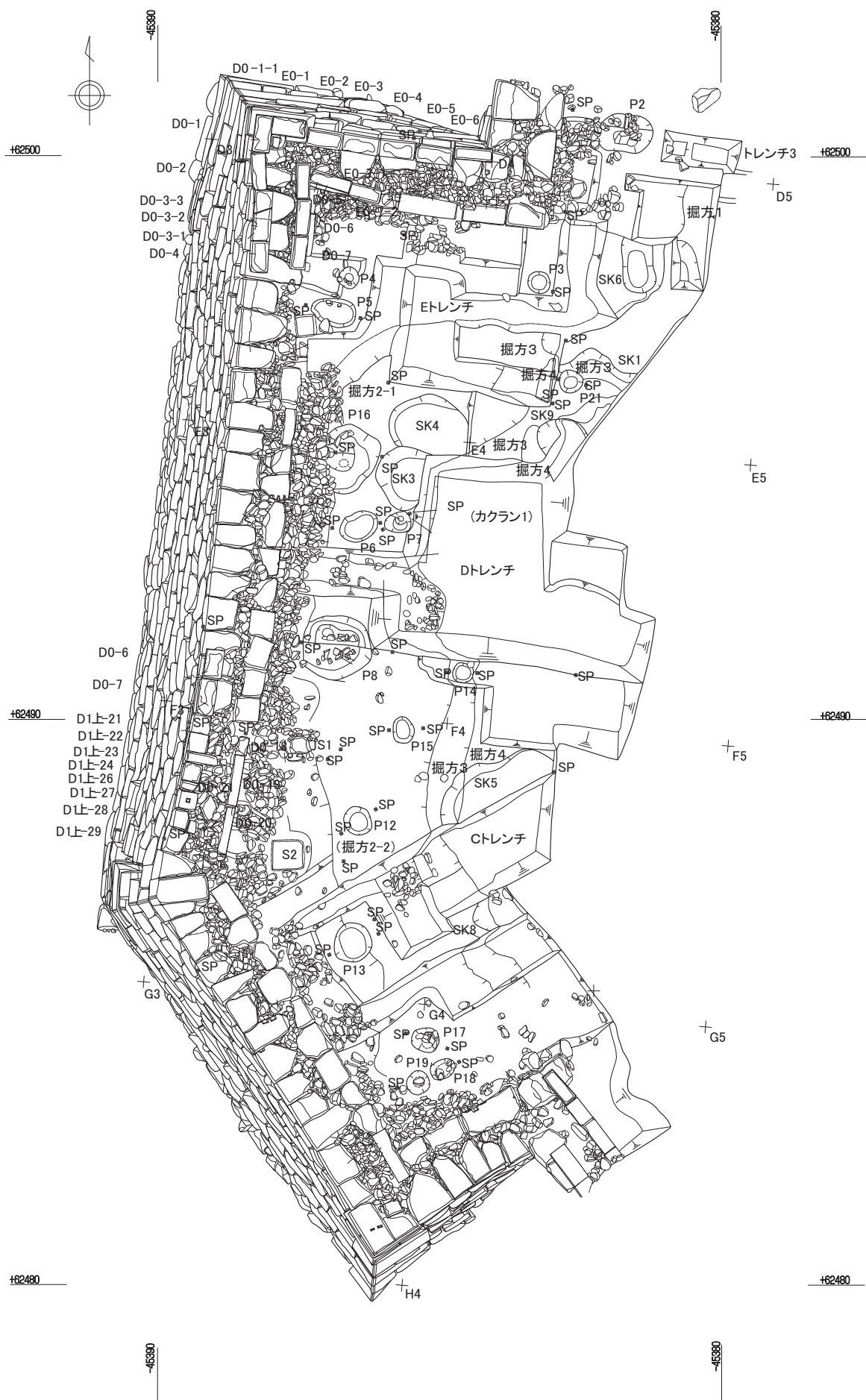
第22図 第0段平面図 (S=1/100)
