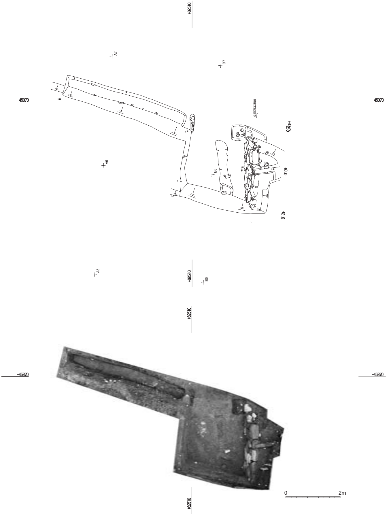
第74図 北拡張区平面図・平面写真 (S=1/80)
