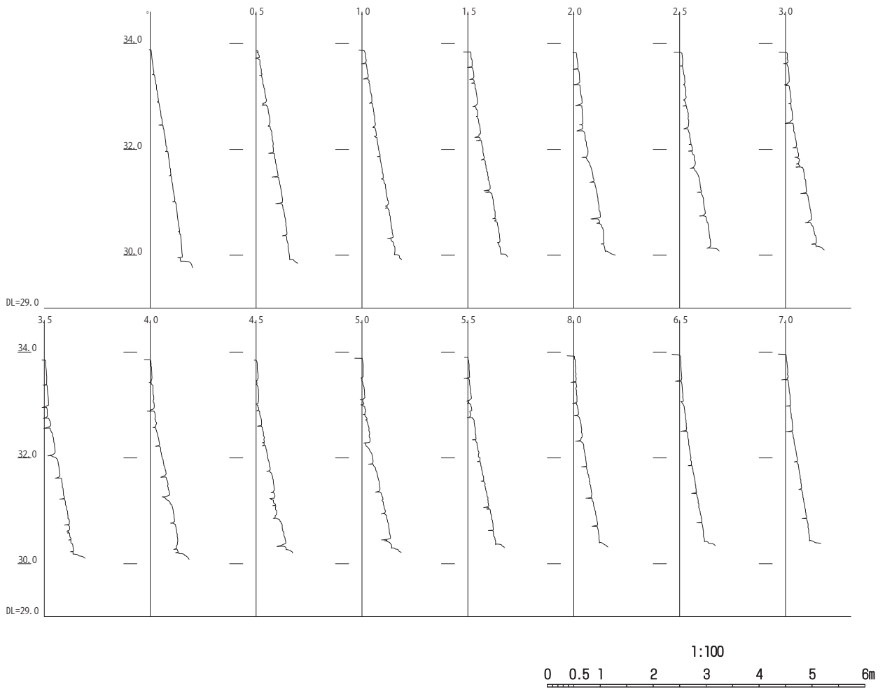
第206図 修復後石垣垂直断面図 1
