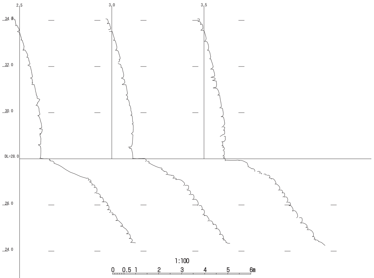
第17图 石垣垂直断面图3
