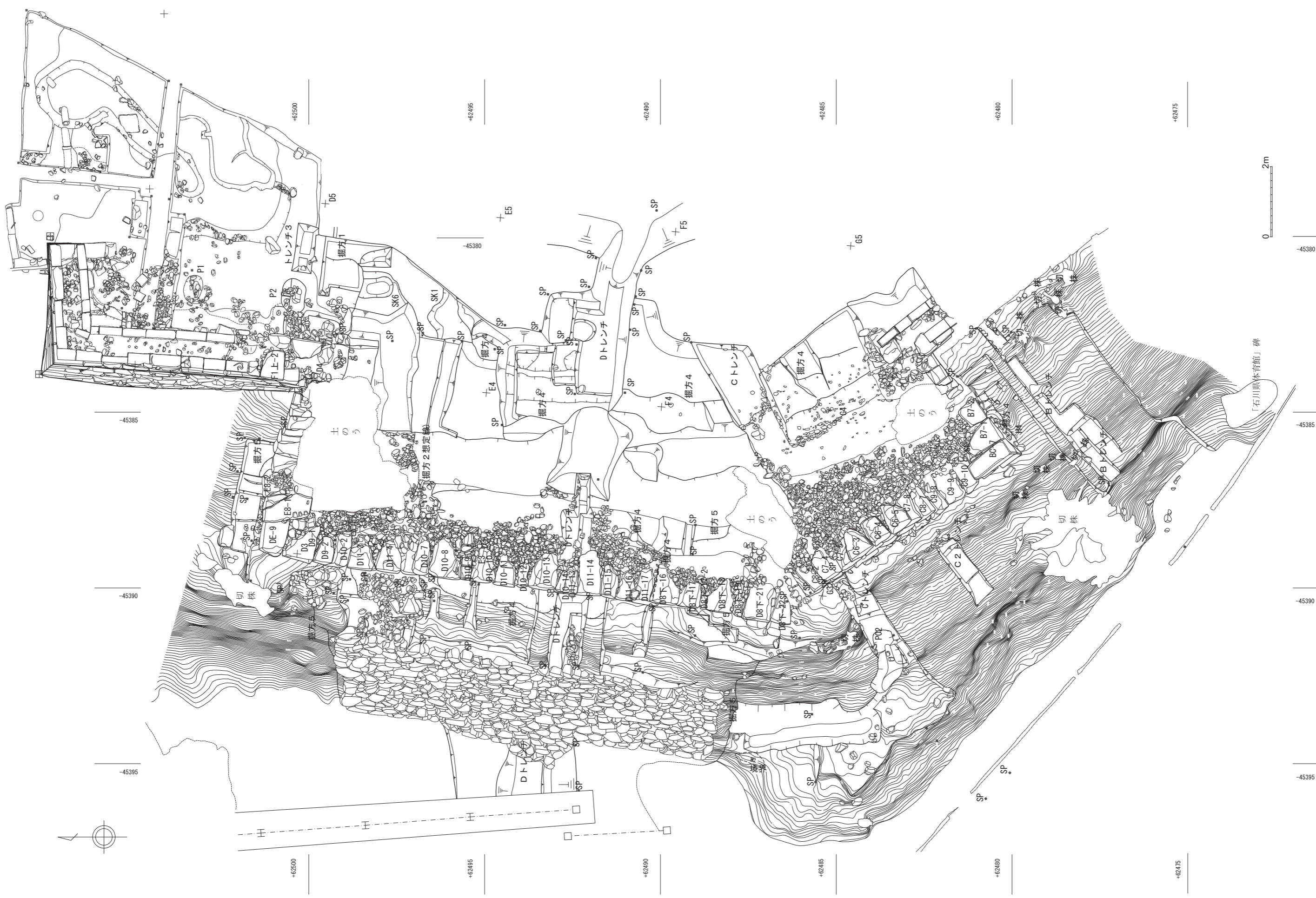
第63図 スノ部平面図 (S=1/100)
