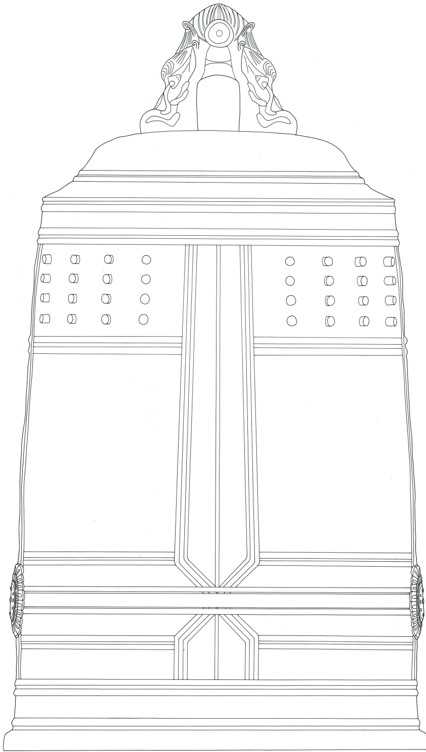
第474图 第10群第7号铸造土壙出土梵钟复原图
