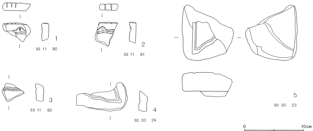
第460図 磬鑄型集成
