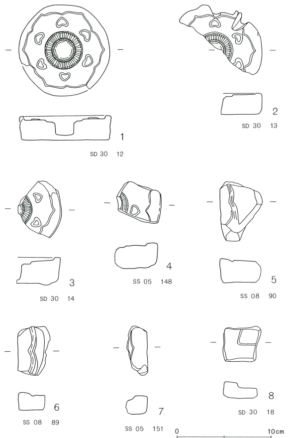
第459図 飾り金具鑄型集成
