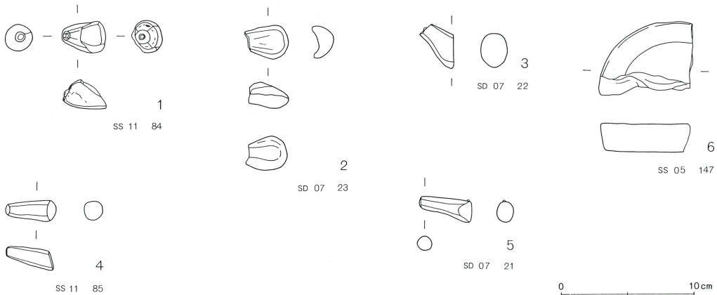
第462図 注ぎ口・鏡鑄型集成
