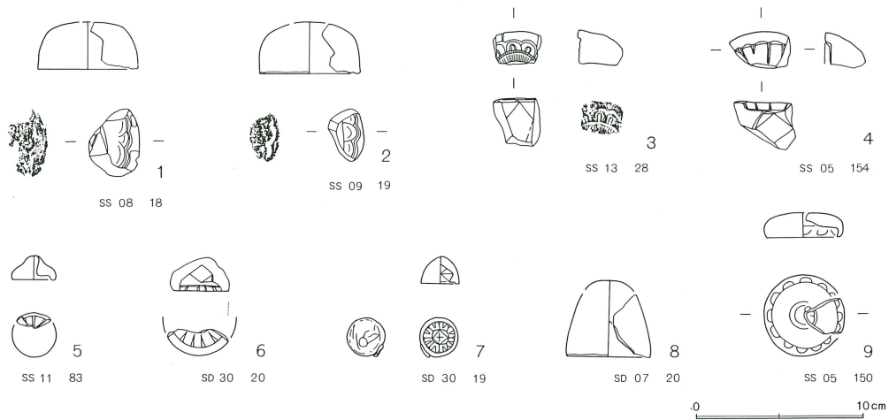
第461図 つまみ鑄型集成
