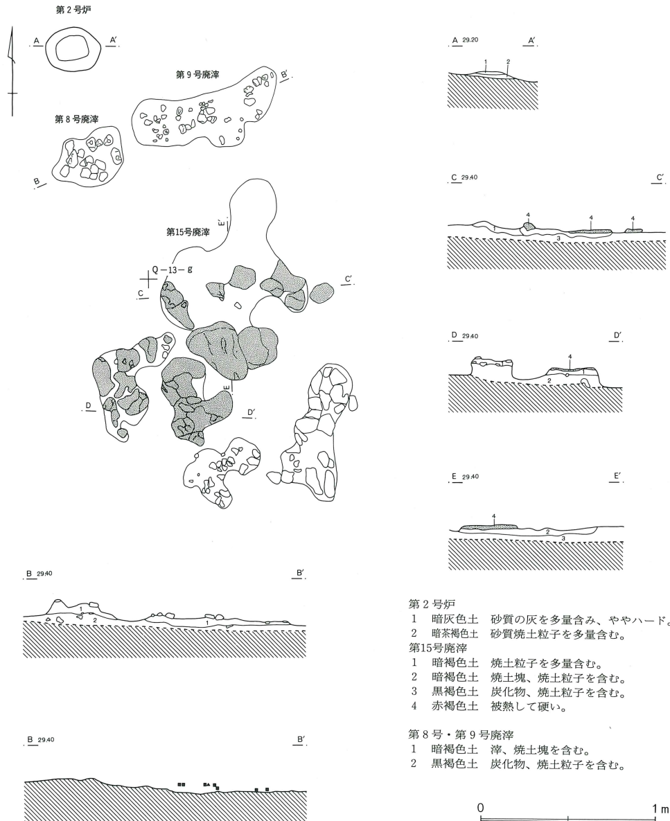
第272図 第8群第2号炉跡・第8・9・15号廃滓
