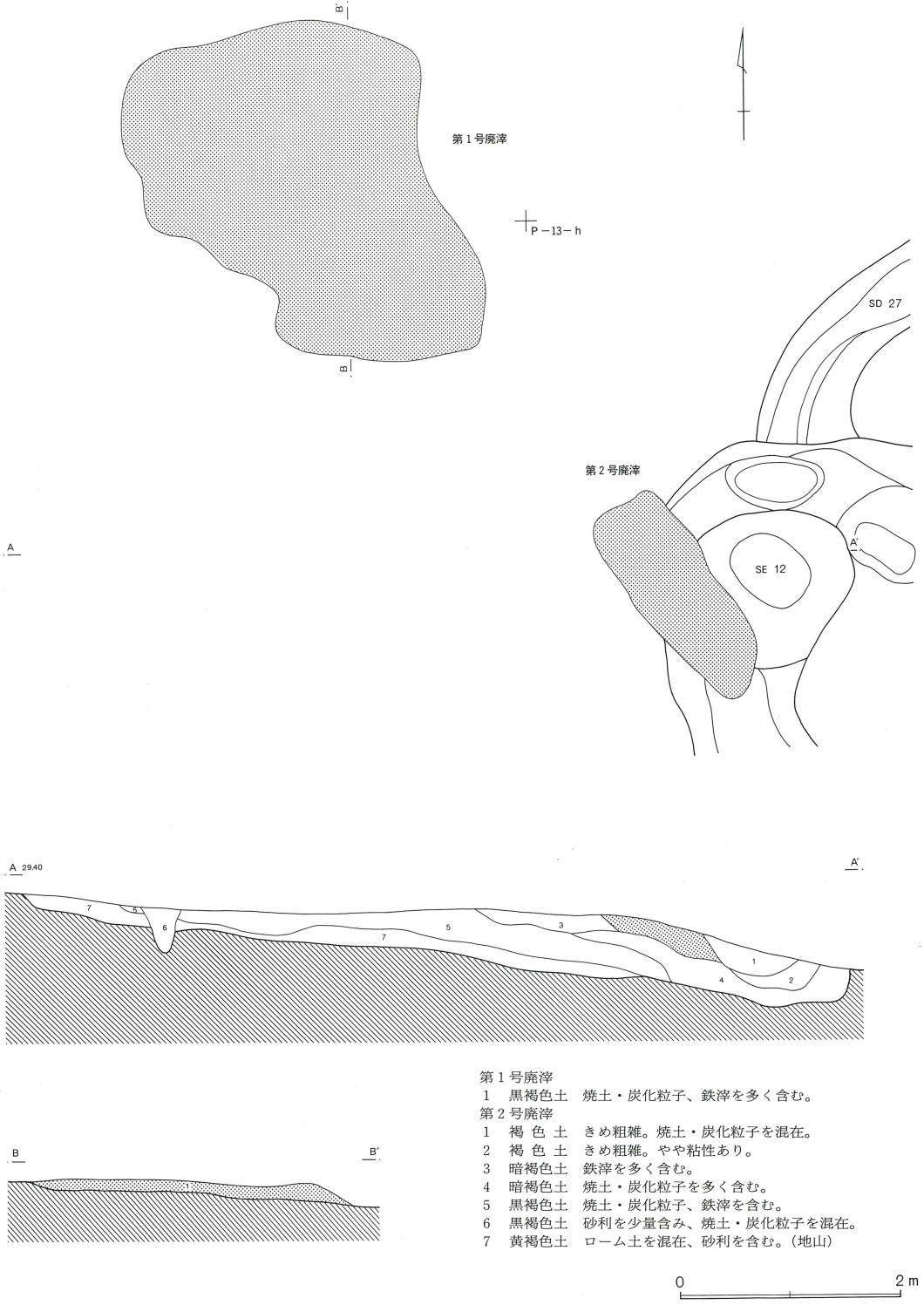
第289図 第9 铸造遺構群全体図
