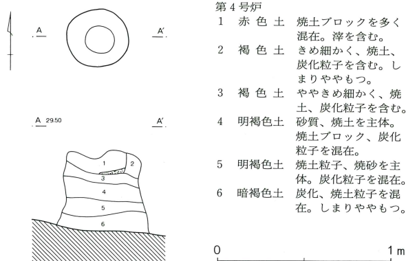
第299図 第10群第4号炉跡
