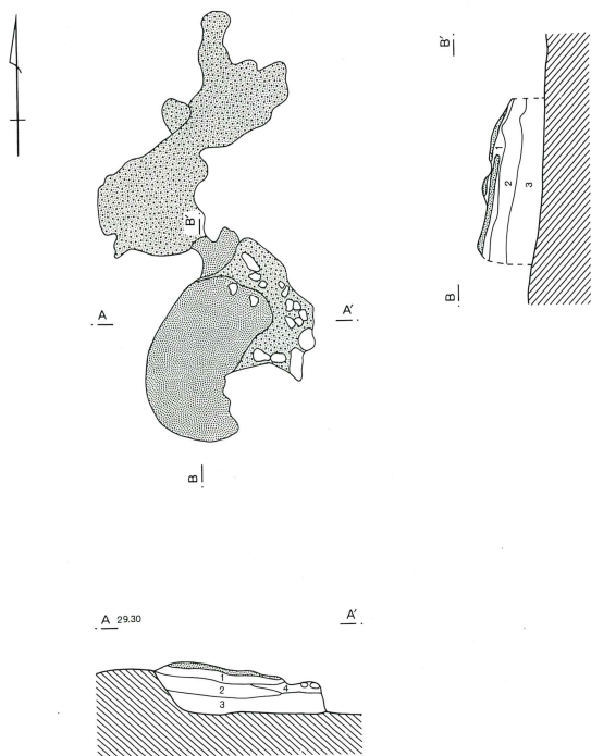
第271図 第8群炉体1号
