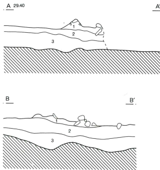
第274図 第8群第11・12号廃滓
