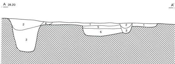
第295図 第10群第2・6・8・9号鑄造土壇
