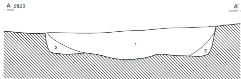
第296図 第10群第3・4号鑄造土壇
