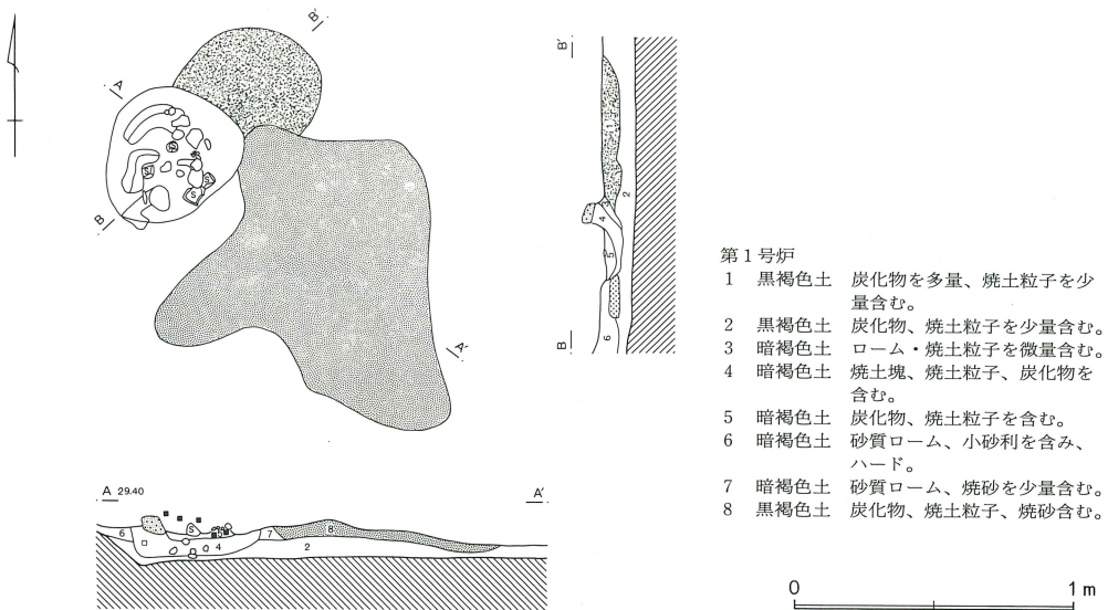
第269図 第8群第1号炉跡
