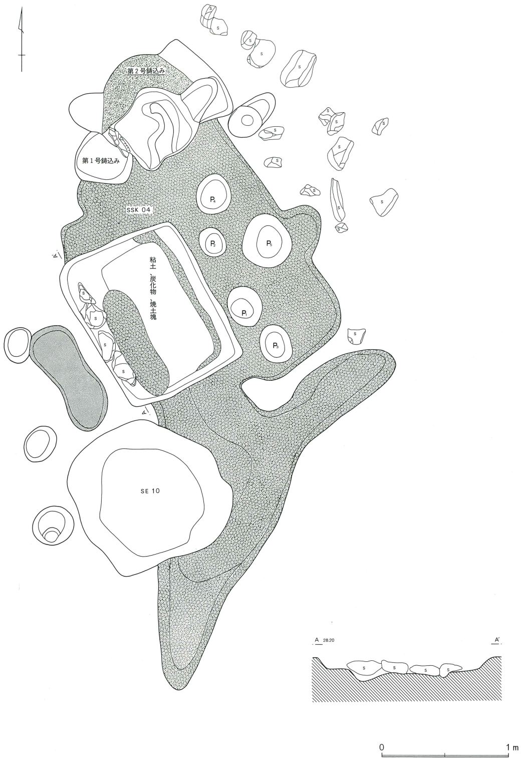
第312図 第11群第1・2号鋤込み跡・第4号鋤造土壇(1)
