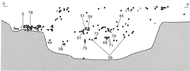
第267図 第8群第1号鑄造土壌
