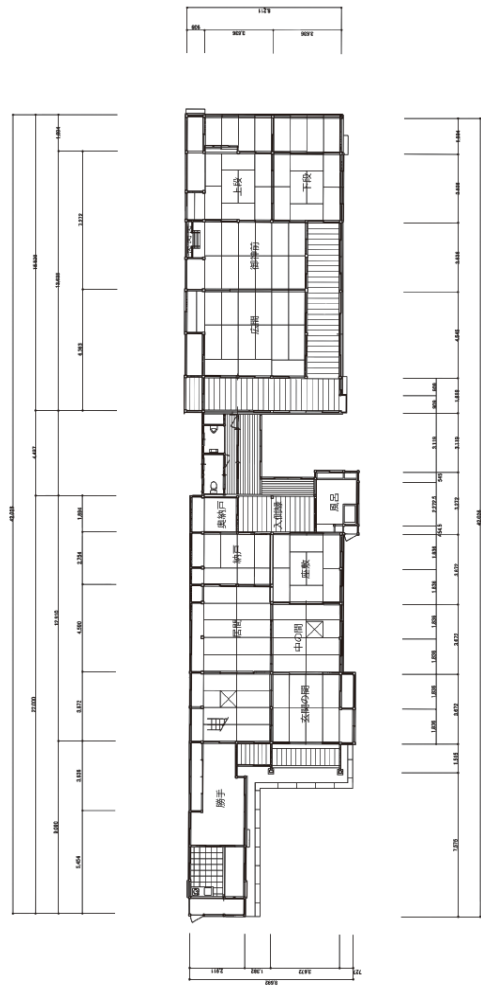
図 2-2 旧外川家住宅平面図(しほや)
