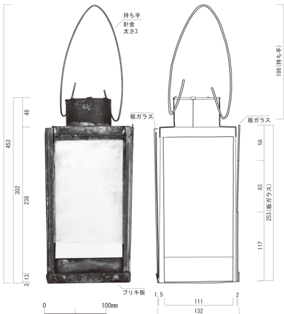
1709 (17-011-008-1、2) 井上小屋 角灯
