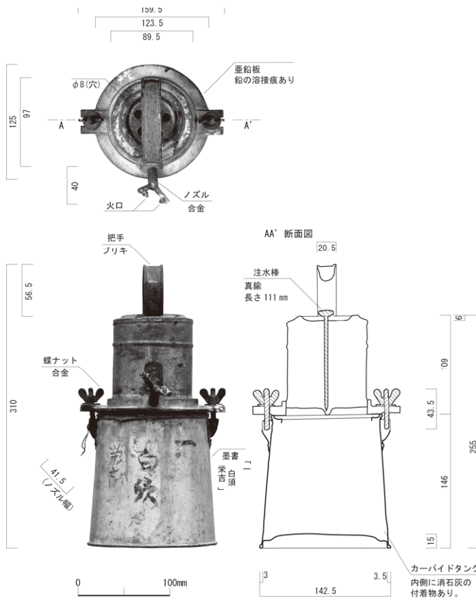
1707 (18-016-258) はちみつ屋 カーバイドランプ 垣内律子 (昭和測量)
