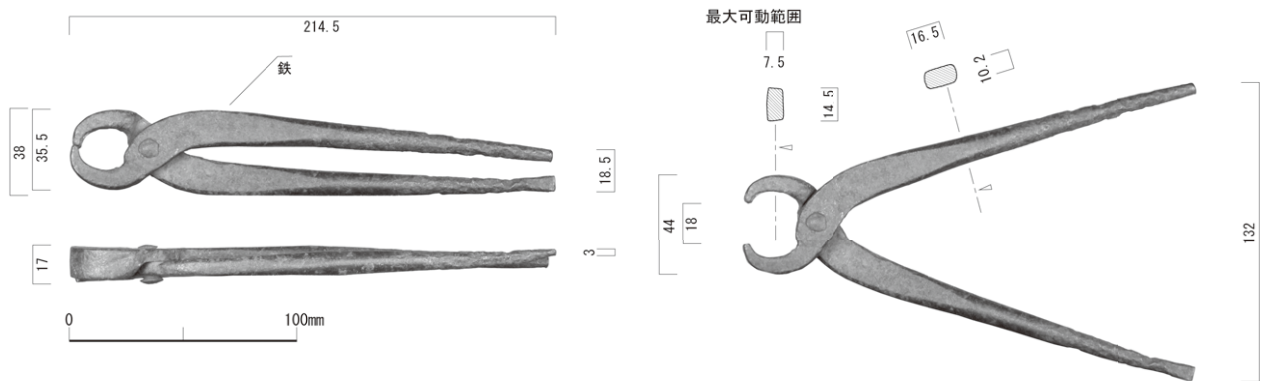
1978 (91-004-079-26) 富士山禊所 ヤットコ 尾川正美 (昭和測量)
