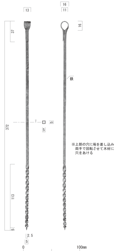
1982 (91-004-079-2) 富士山禊所 ボルト錐 藤原由香 (昭和測量)
