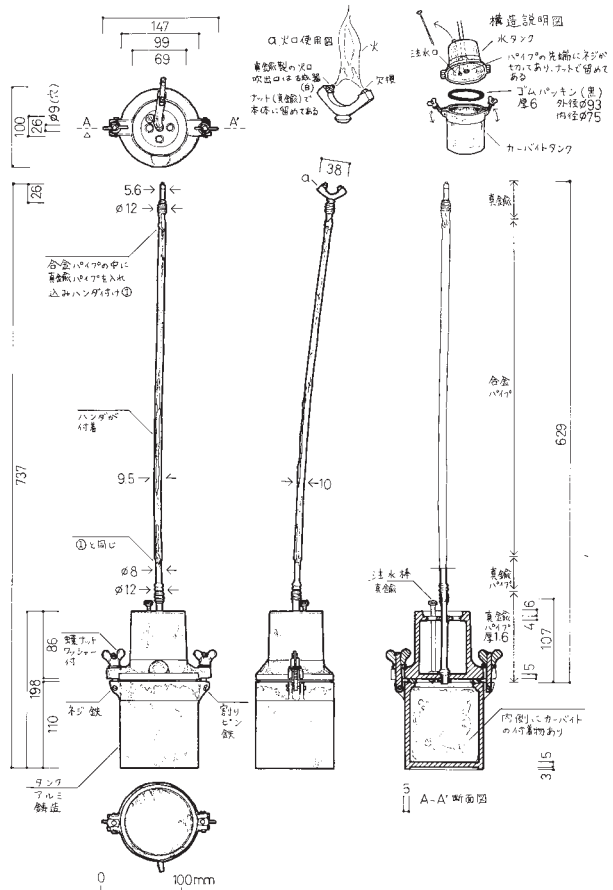
1712 (17-011-004) 井上小屋 カーバイドランプ 金井佐和子
