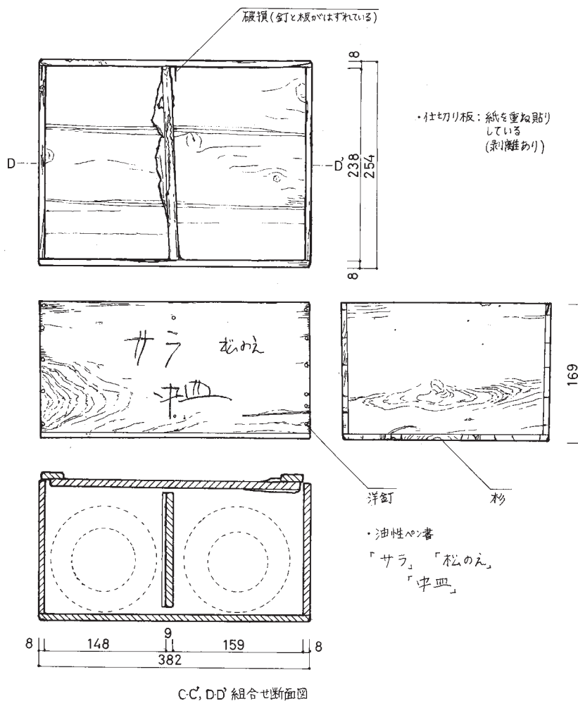
C-C', D-D' 組合せ断面図
