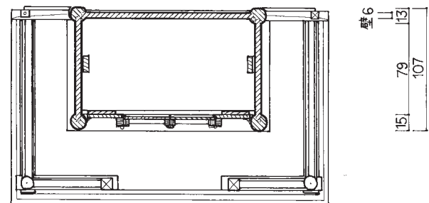
・A-A'断面図
