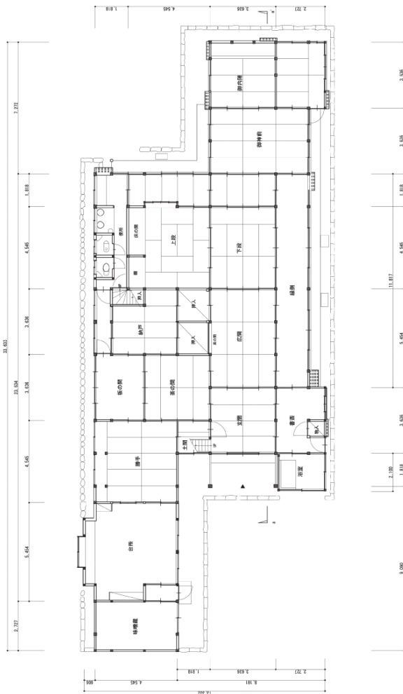
図 2-1 小佐野家住宅平面図(堀端屋)
