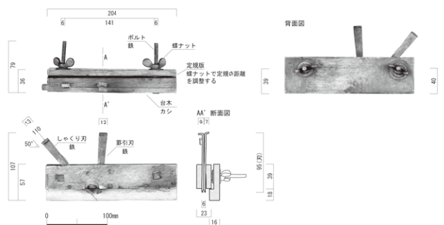
1976 (91-004-079-12) 富士山禊所 溝鉋 藤原由香 (昭和測量)
