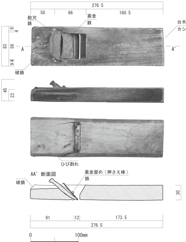
1994 (17-011-020) 井上小屋 台鉋 藤原由香 (昭和測量)
