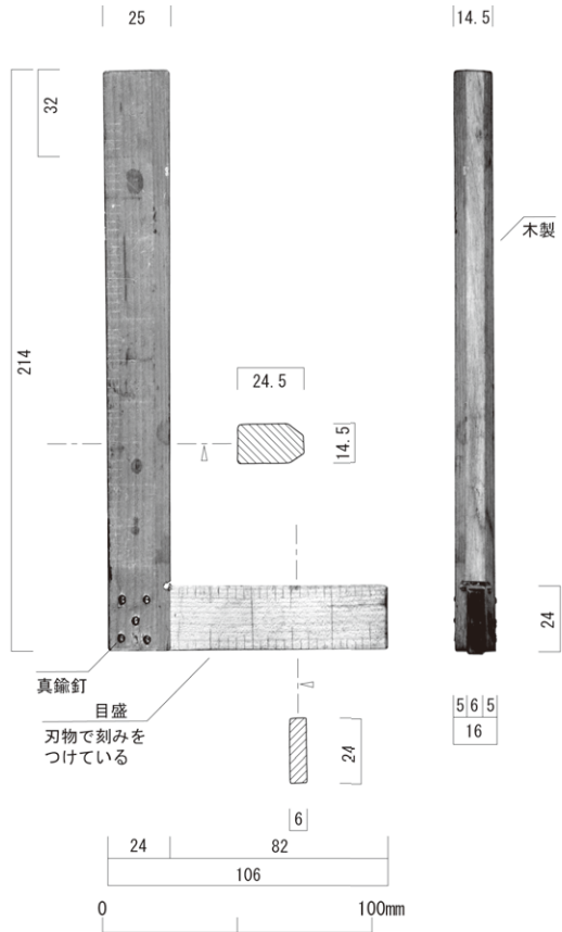
1977 (91-004-079-15) 富士山禊所 スコヤ 尾川正美 (昭和測量)
