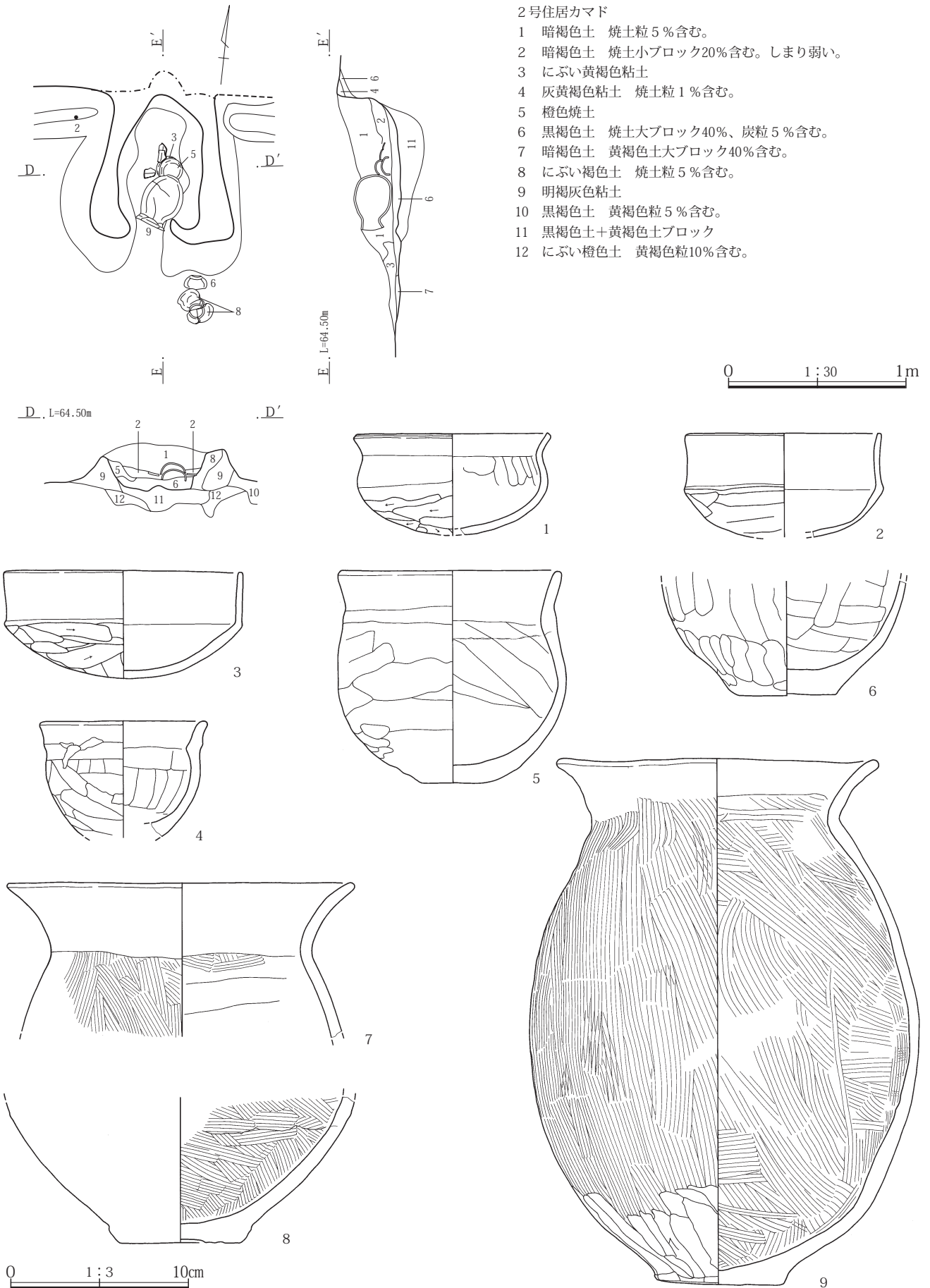
第11図 2号住居カマドと出土遺物
