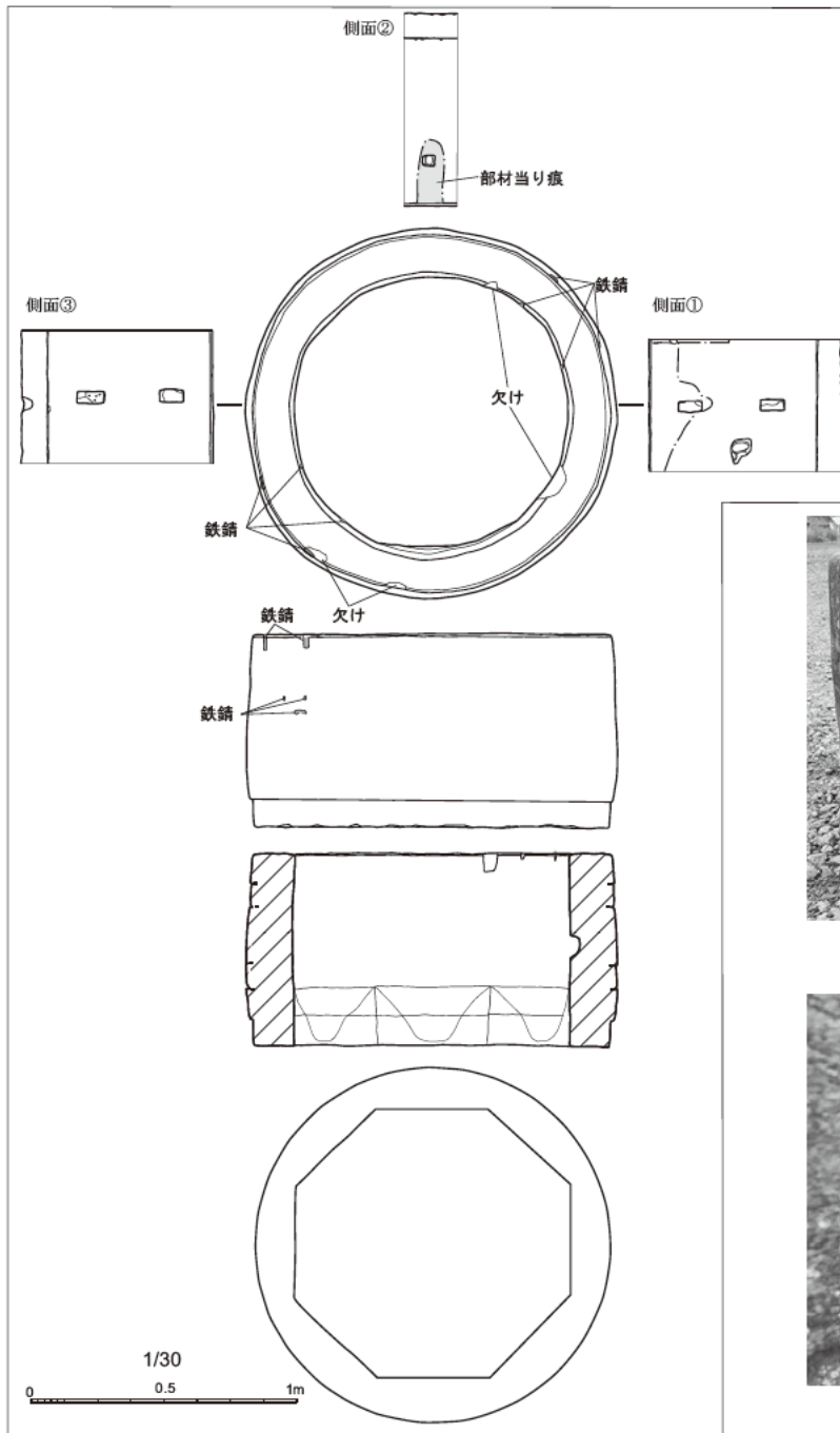
2 井戸杵実測図
