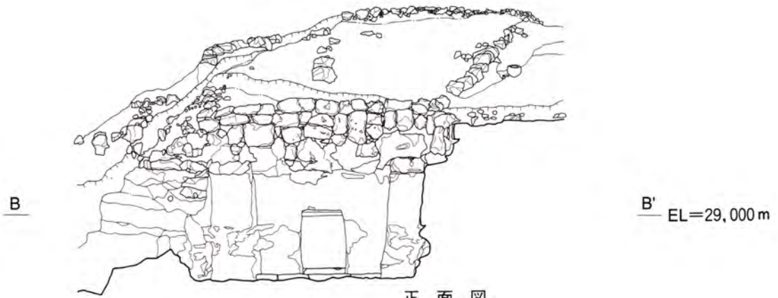
正面図 (Bライン)
