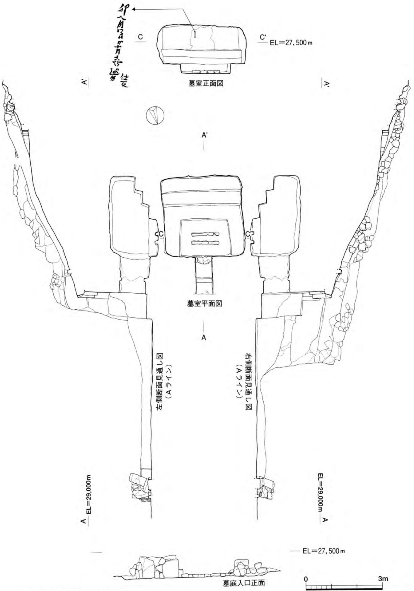
第25図 9号墓実測図 ②
