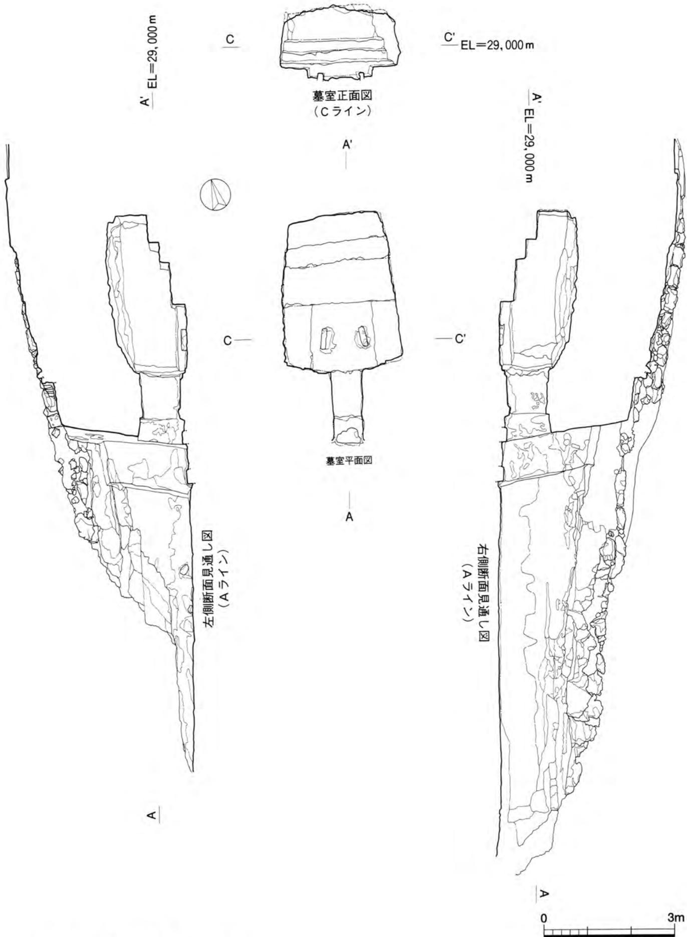
第10図 2号墓実測図②
