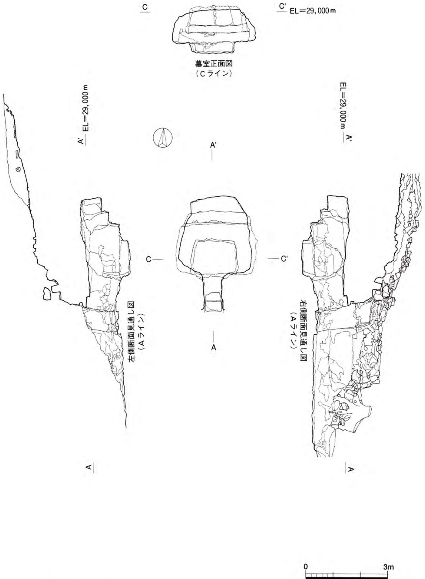
第12図 3号墓実測図②
