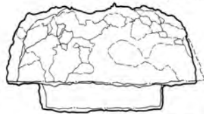
墓室正面図 (Cライン)
