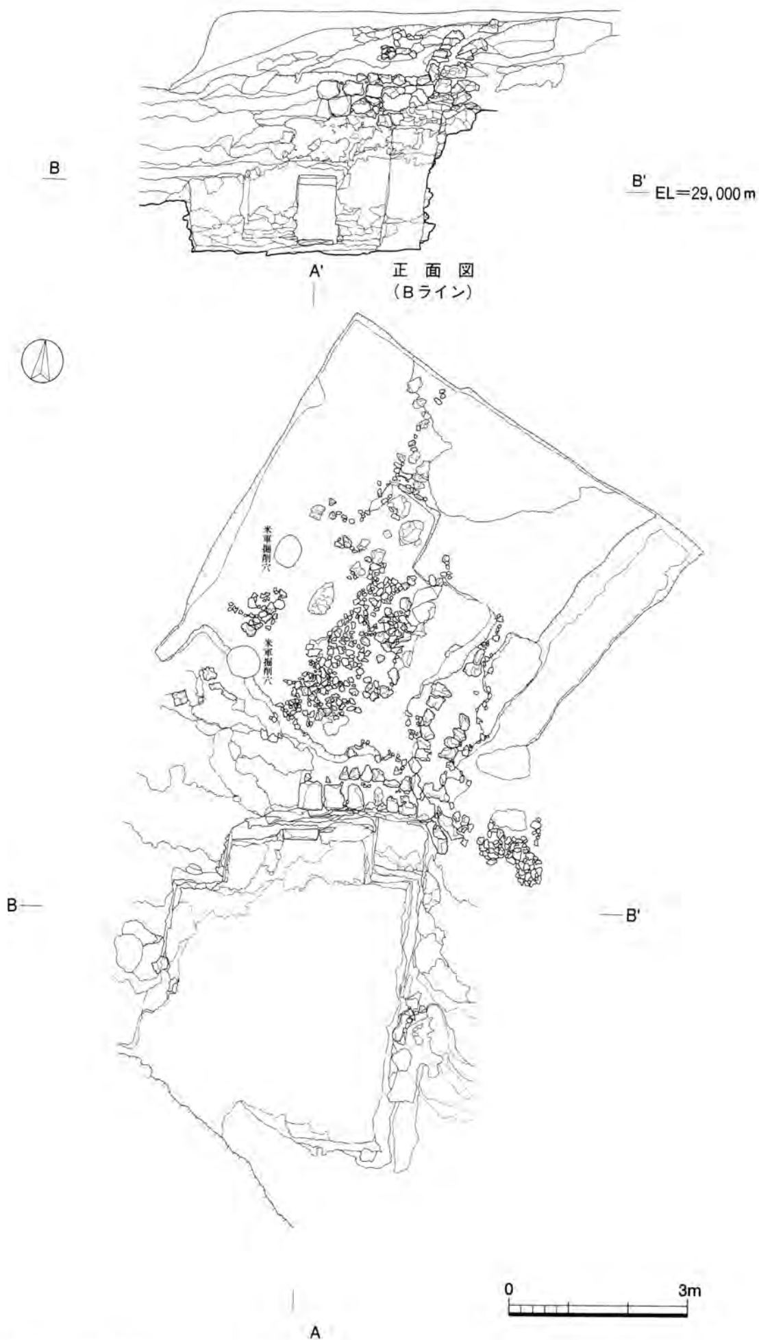
第11図 3号墓実測図①
