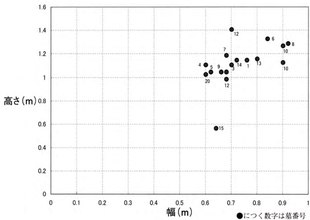
第5図 墓口の高さと幅の散布図
