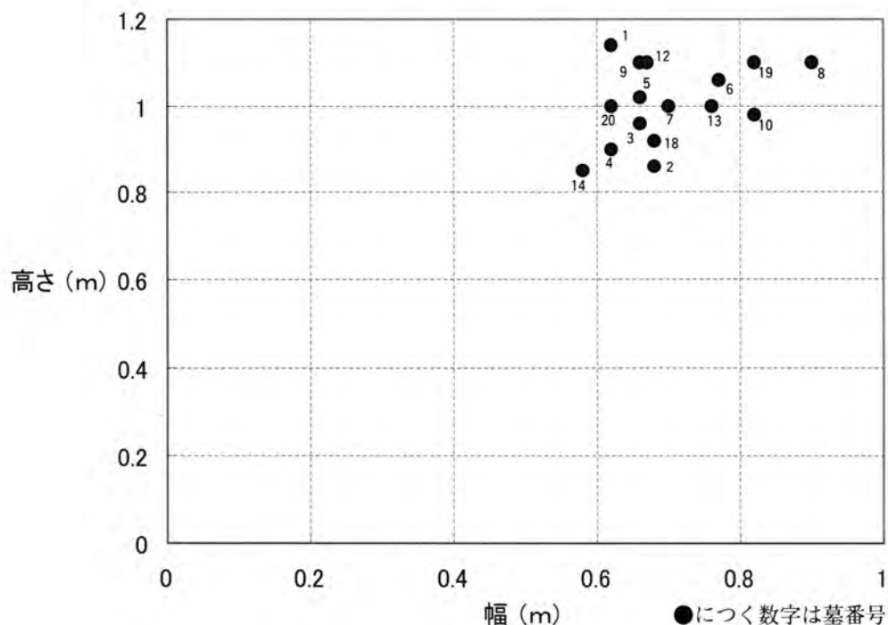
第6図 羨道の高さと幅の散布図
