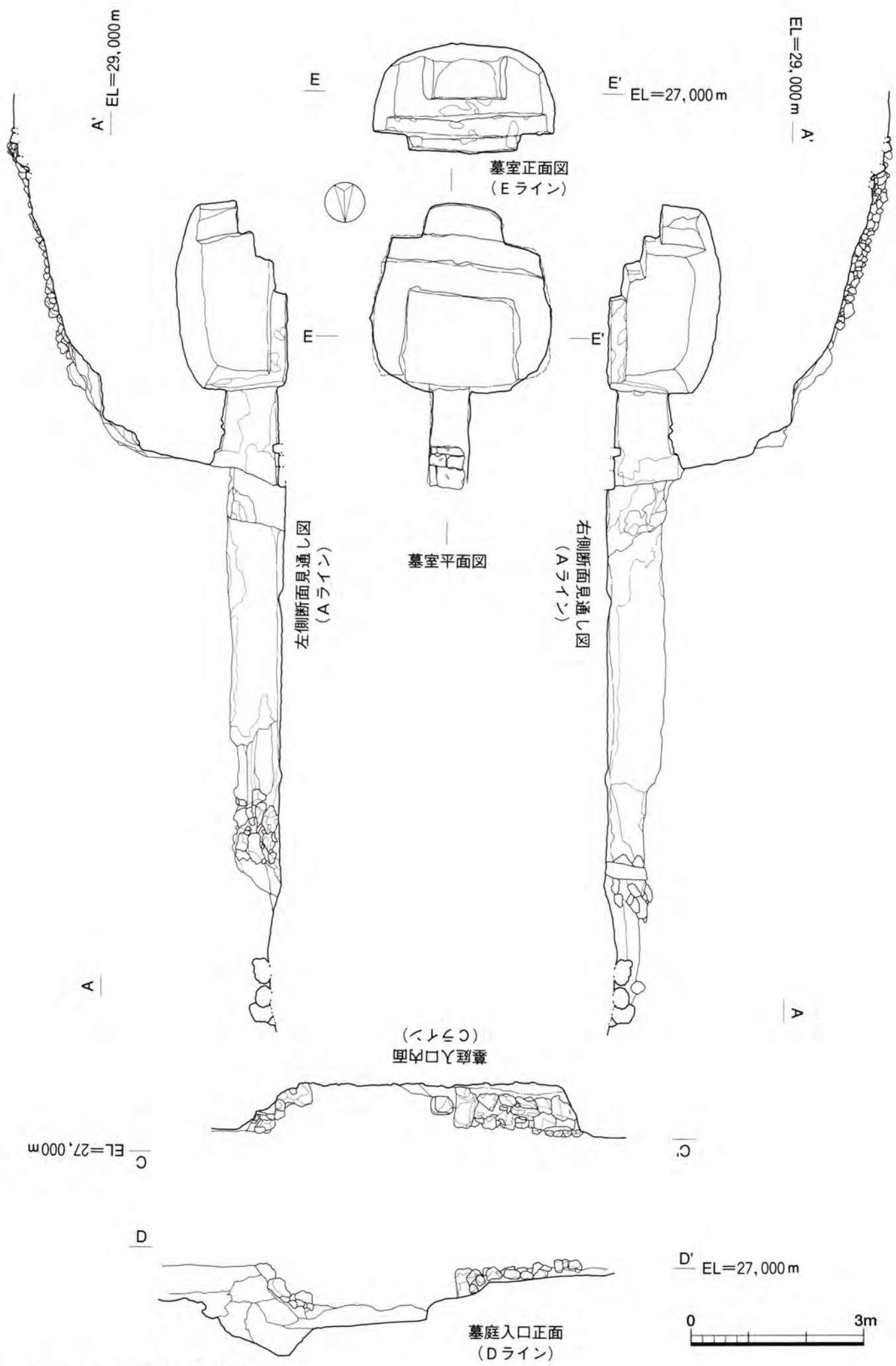
第21図 7号墓実測図②
