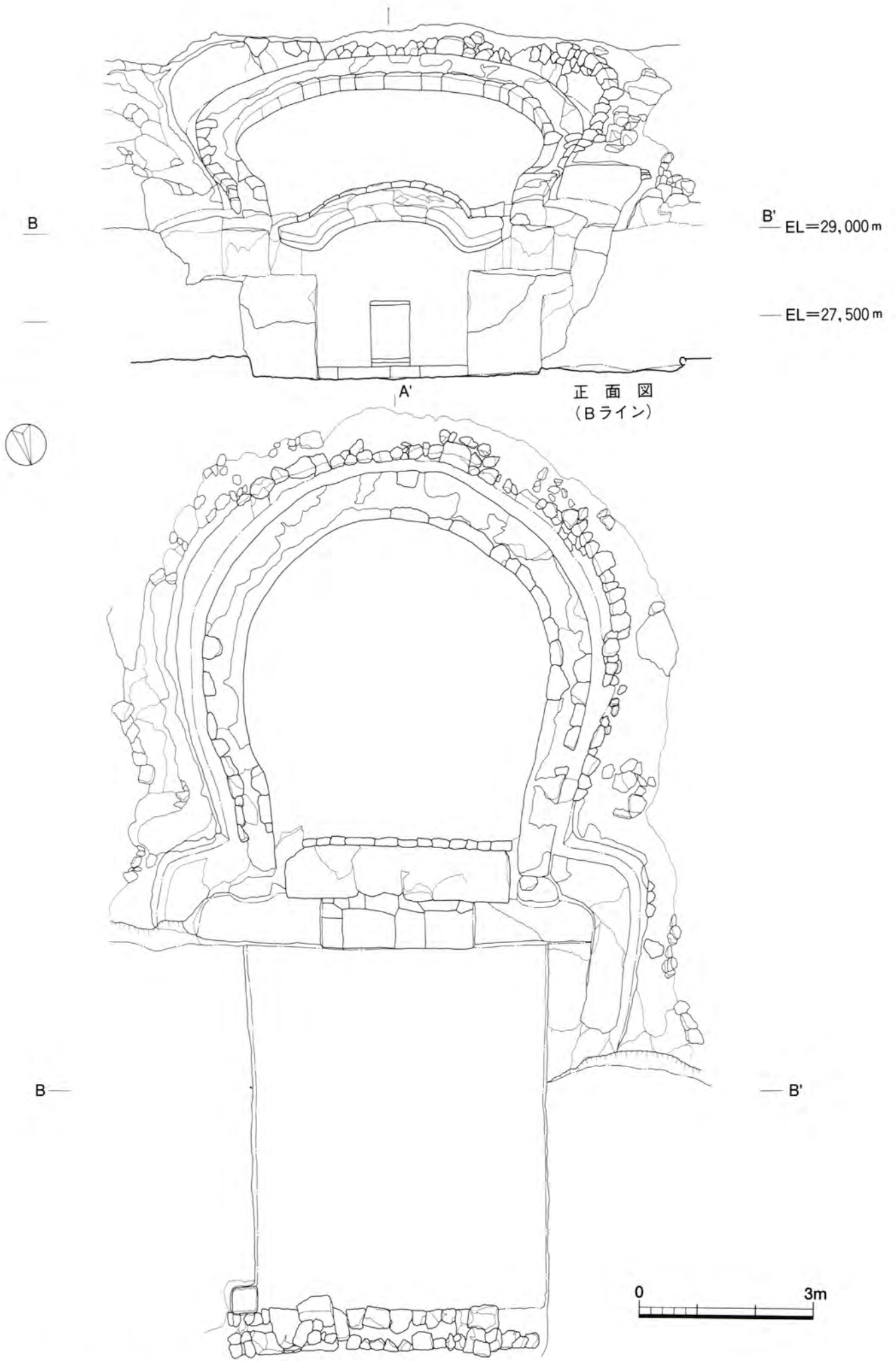
第24図 9号墓実測図①
