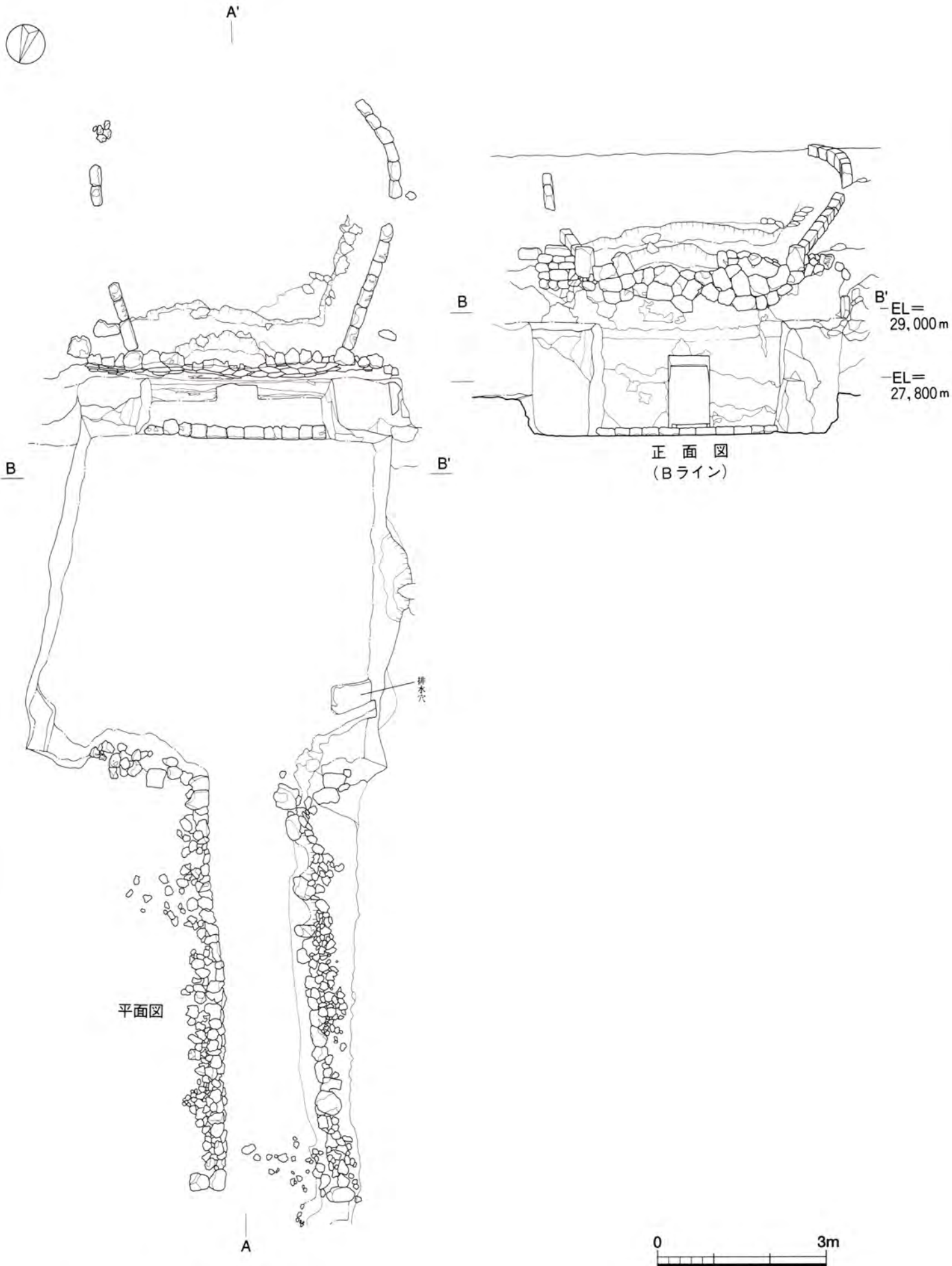
第18図 6号墓実測図①
