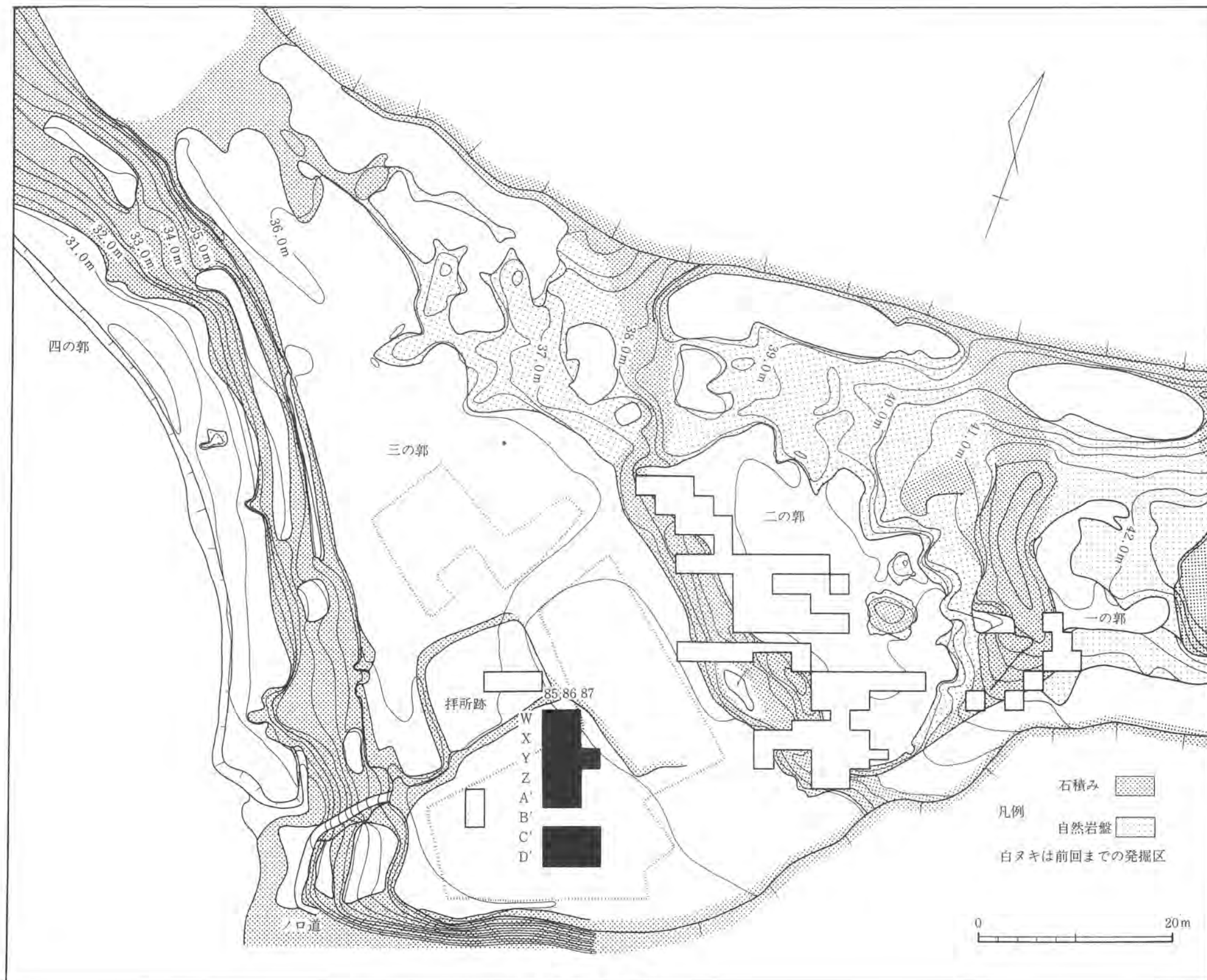
第2図 地形測量図
