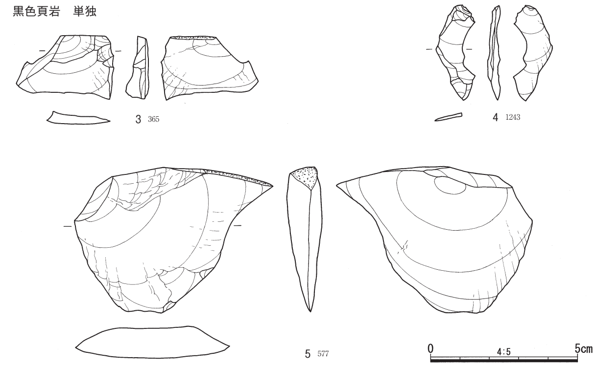
第103図 母岩別資料・接合資料
