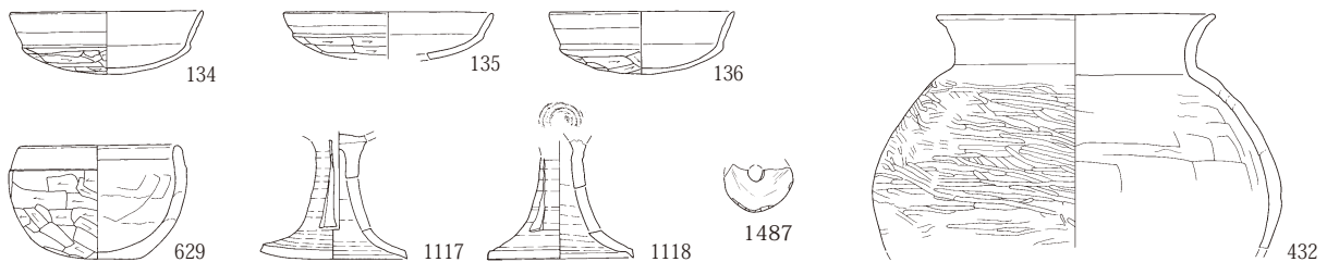
第205図 530号住居掘り方・カマド 531号住居出土遺物
