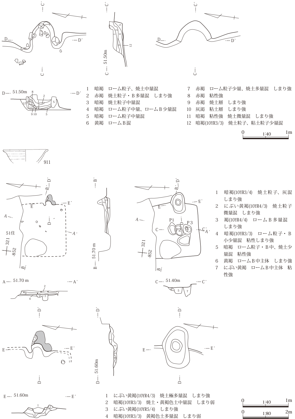
第196図 507号住居カマド 508号住居
