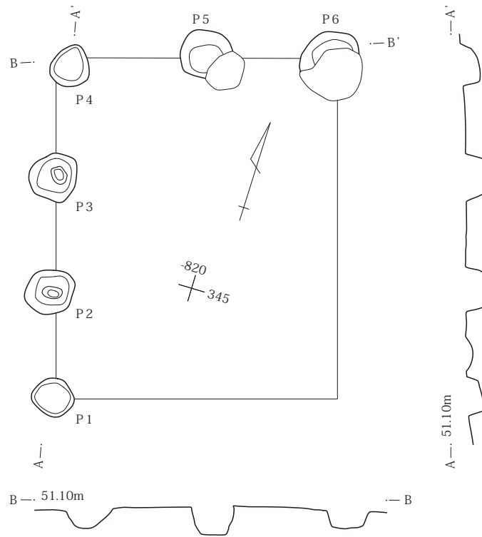
第223図 10号掘立柱建物 11号掘立柱建物
