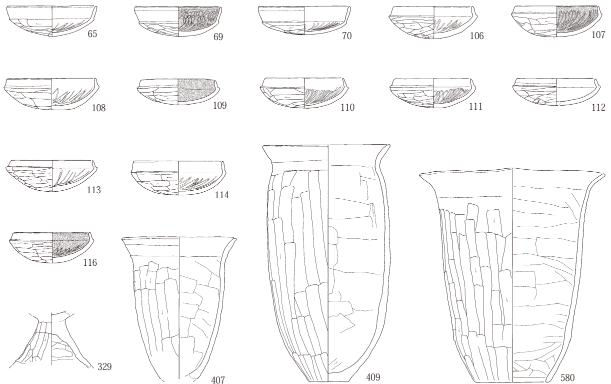
第211図 534号住居カマド 538号住居出土遺物
