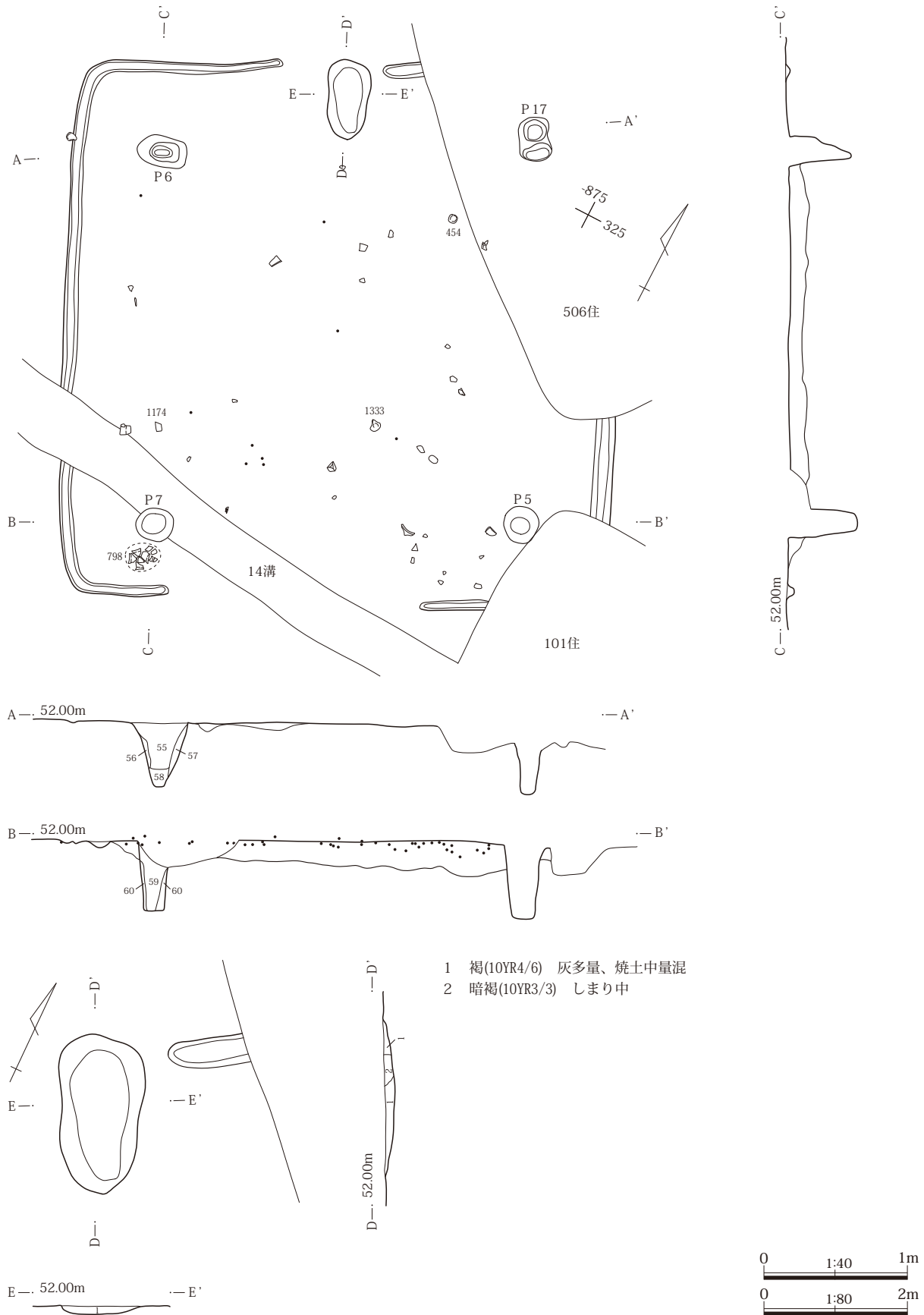
第192図 505B号住居使用面・カマド
