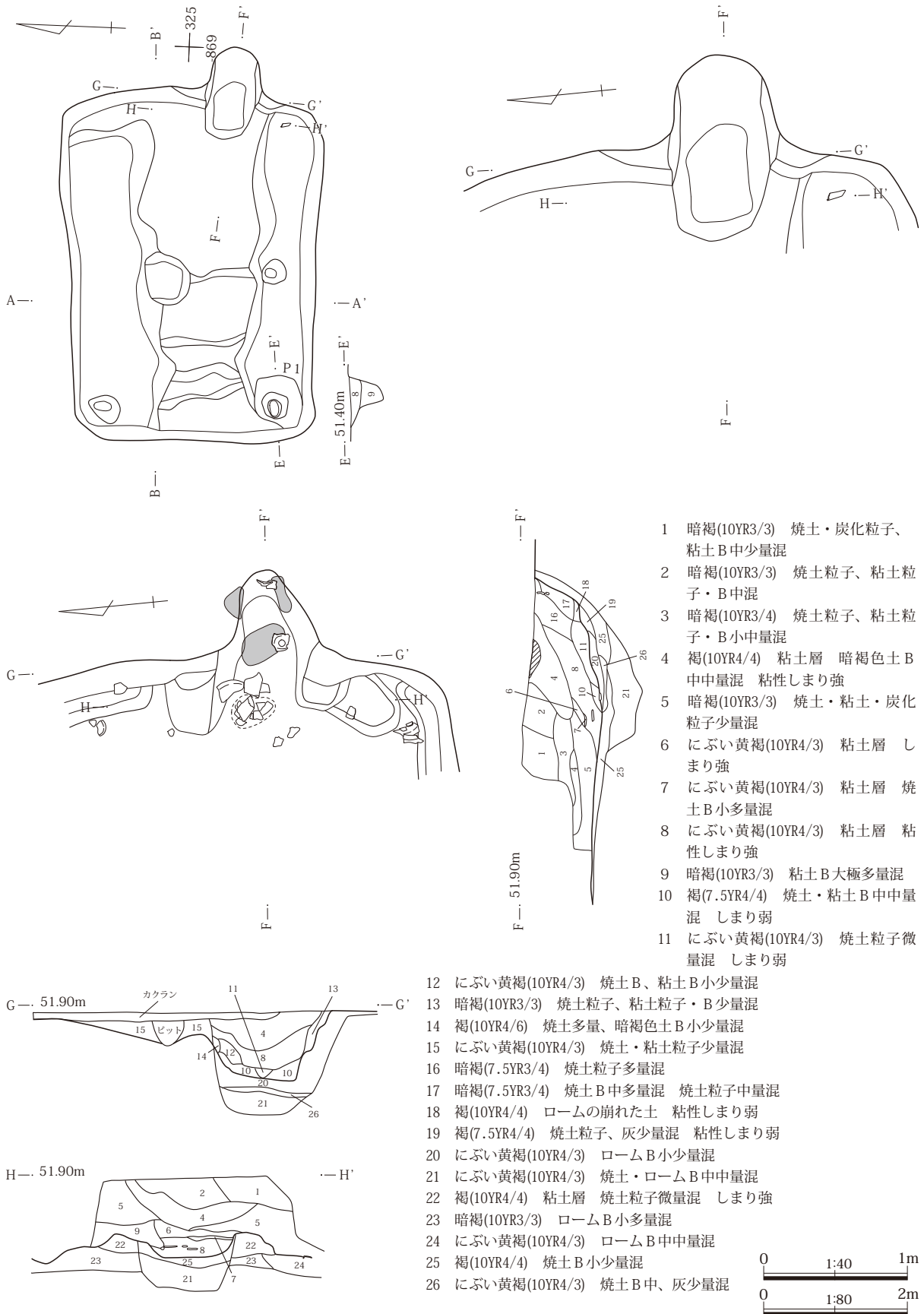
第163図 105号住居掘り方・カマド
