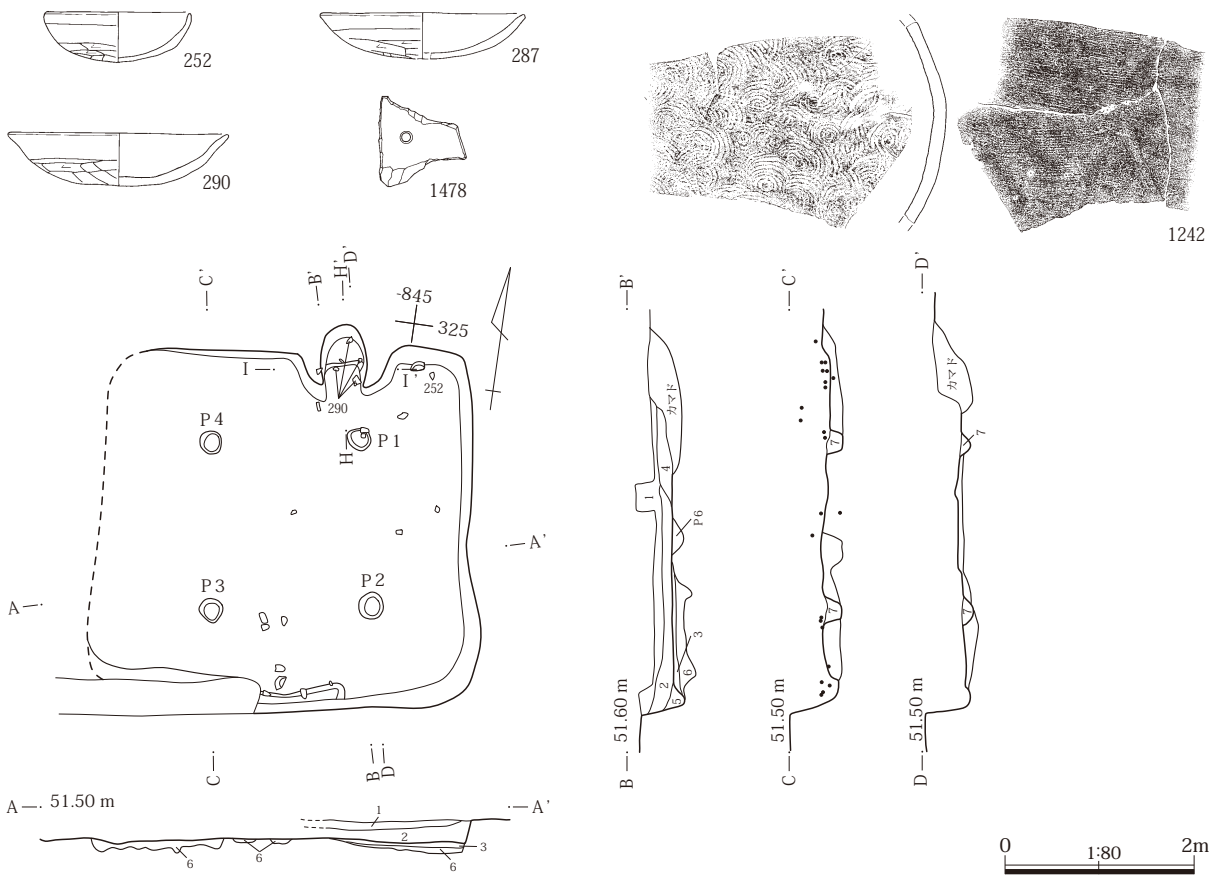
第198図 510号住居カマド 511号住居出土遺物・使用面
