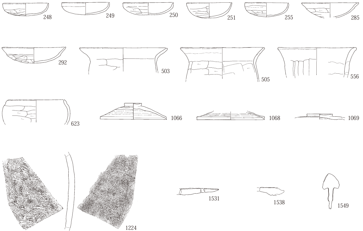
第179図 462号住居掘り方 484号住居出土遺物
