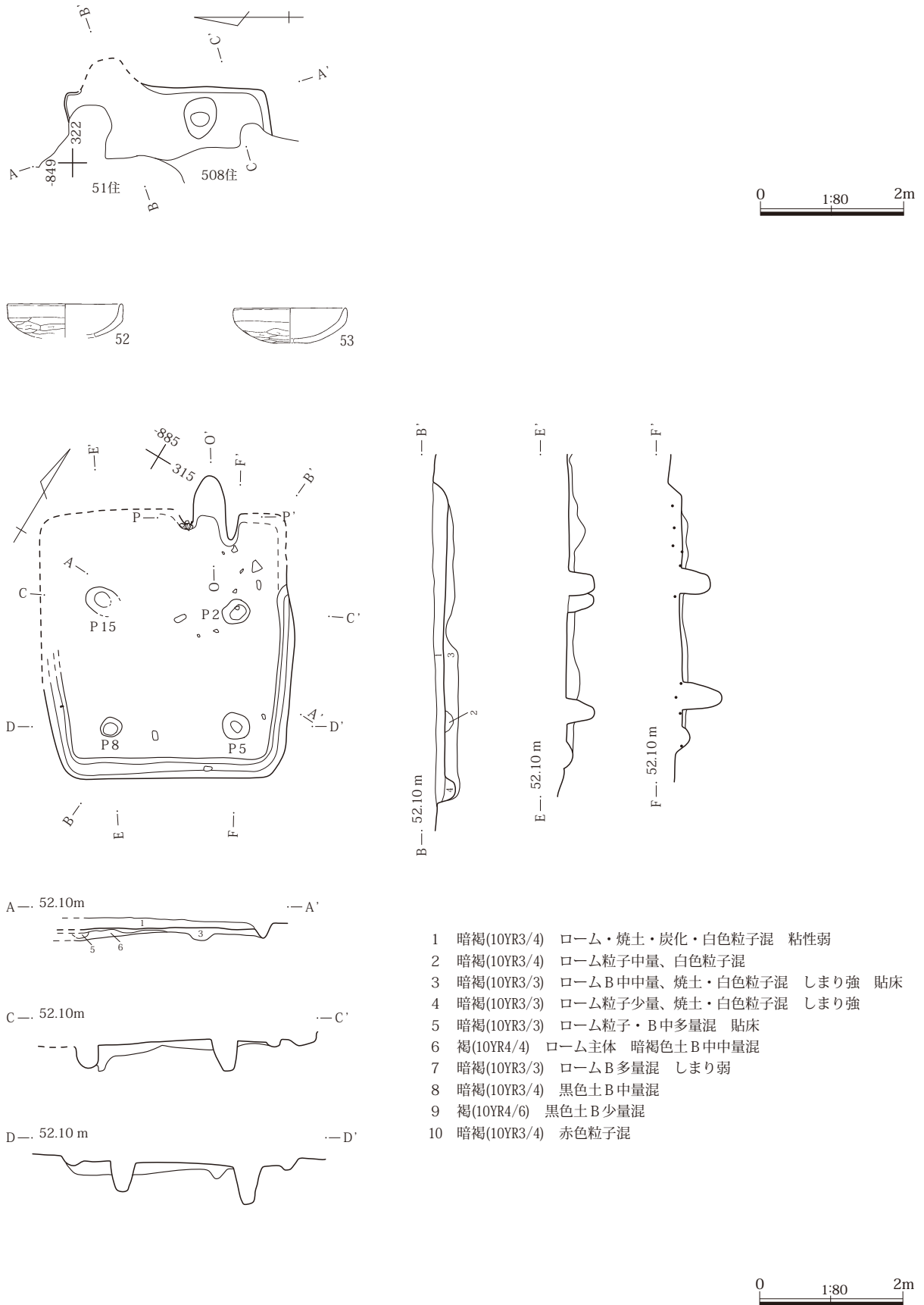
第182図 486号住居掘り方 488号住居出土遺物・使用面
