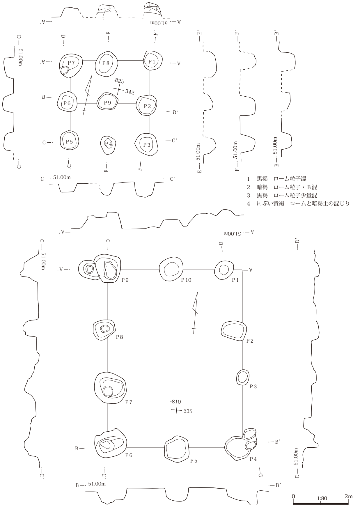
第222図 6号掘立柱建物 7号掘立柱建物
