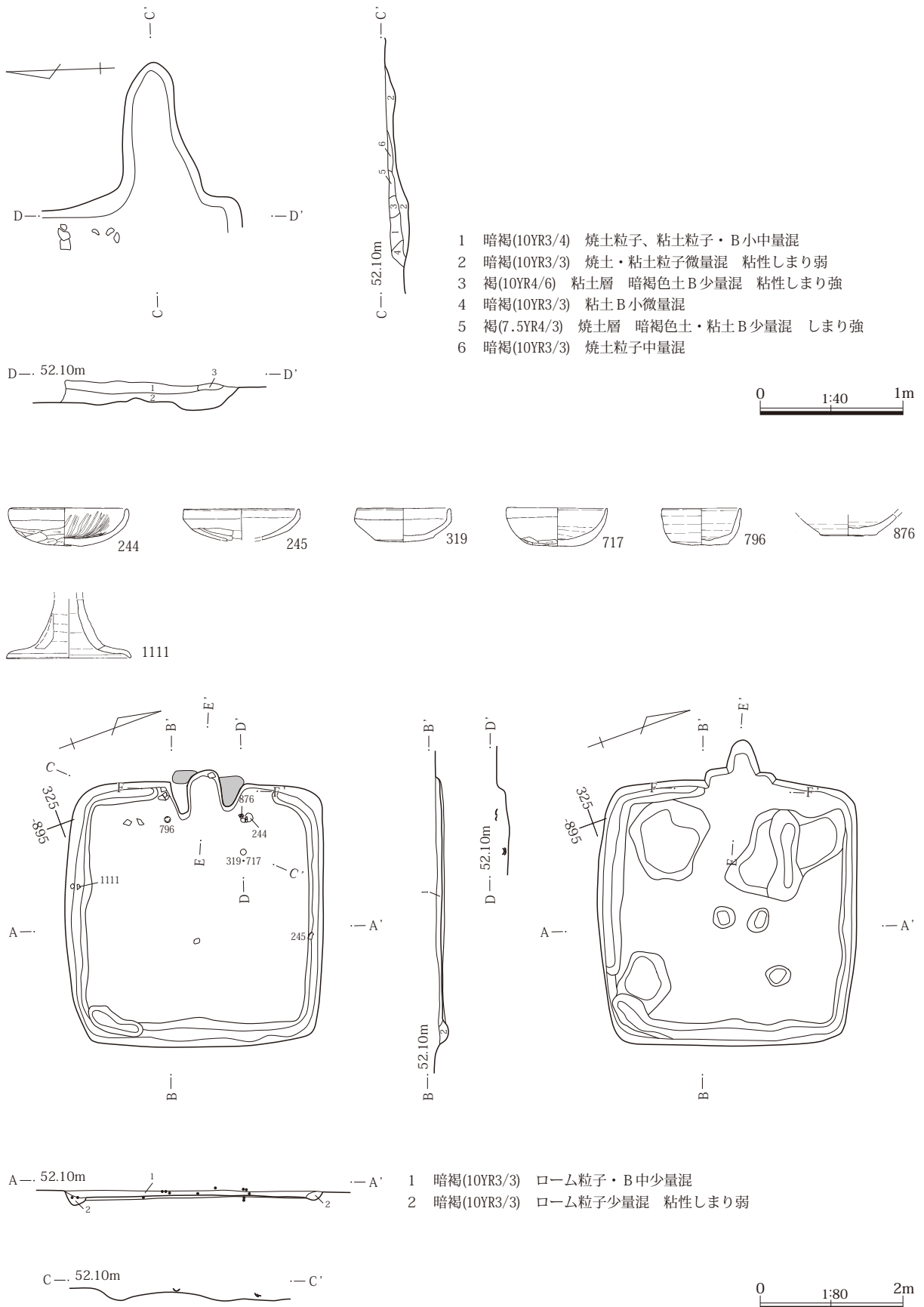
第173図 116号住居カマド 117号住居出土遺物・使用面・掘り方
