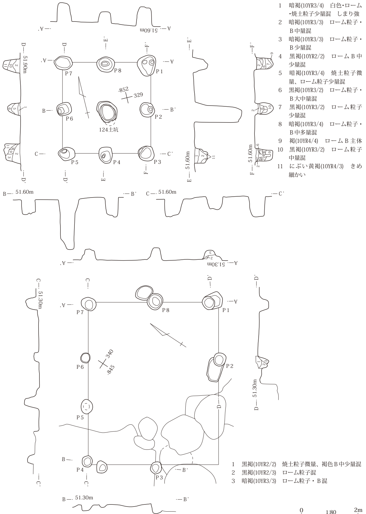
第220図 4号掘立柱建物 21号掘立柱建物
