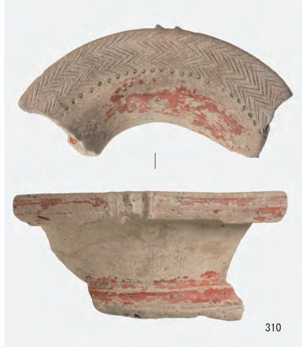
A 1 区 河道S9 南半20~40 cm (257 ~ 259 · 271 · 272 · 285 · 287 · 288 · 290), 40~60 cm (310)
