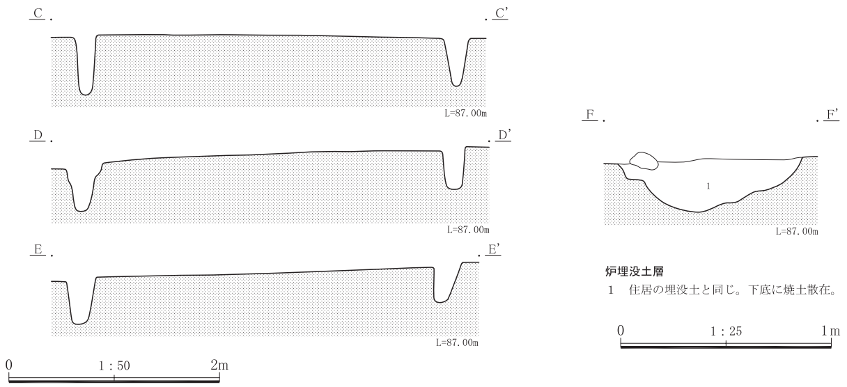
第133図 II - 2号住居断面・炉
