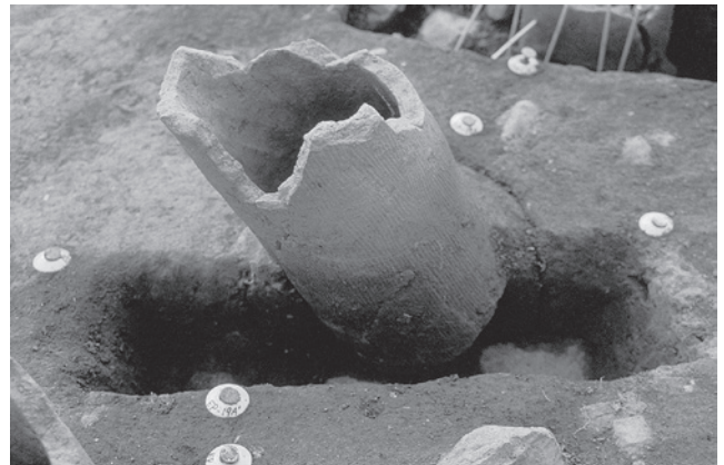
4 2号墳 埴輪列 19 掘り方断面 (東→)
