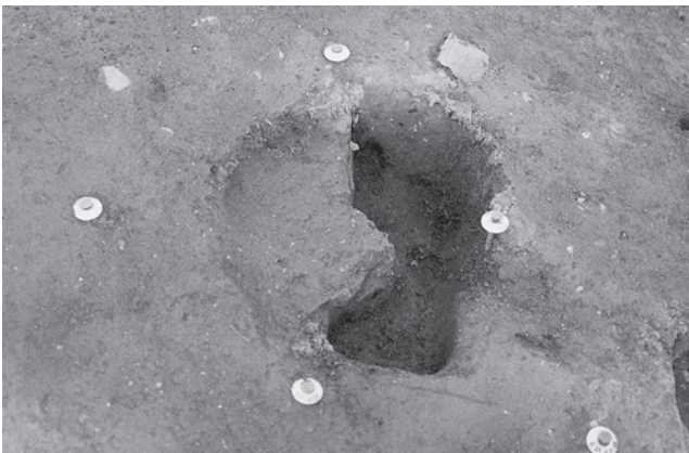
7 2号墳 埴輪列 58 掘り方 (南西→)
