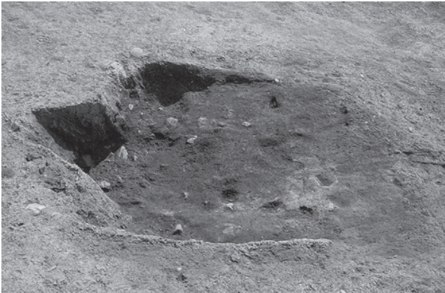
3 2号炭窯 全景 (南西→)
