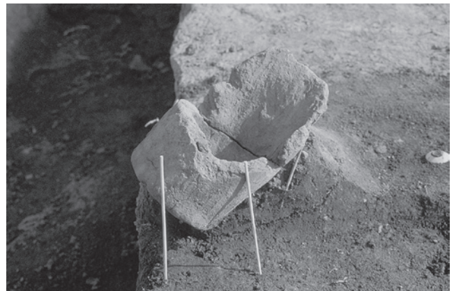
8 2号墳 埴輪列 32 掘り方断面 (北西→)
