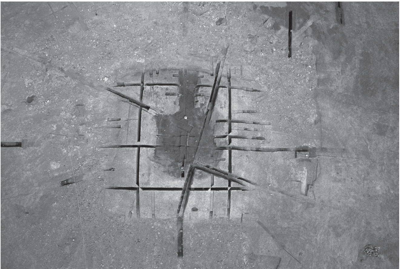
2 成塚向山1号墳 全景（構築墓壙検出時）（上が北）
