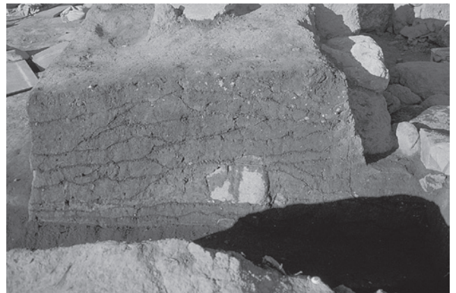
8 2号墳 墳丘盛土 断面f-f' (南→)
