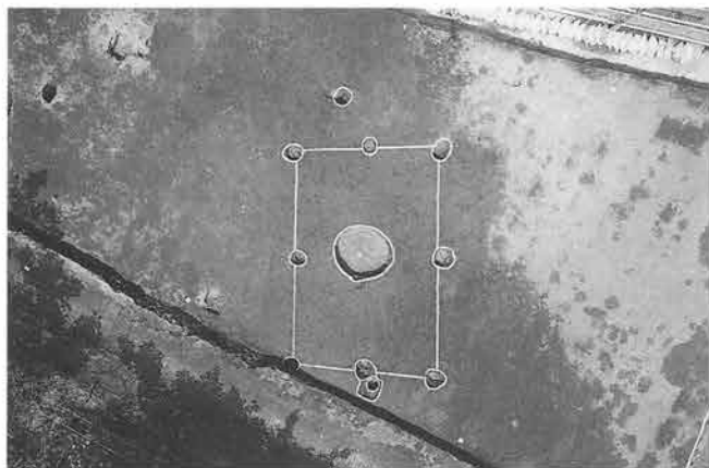
1号掘立柱建物全景（上=北）
