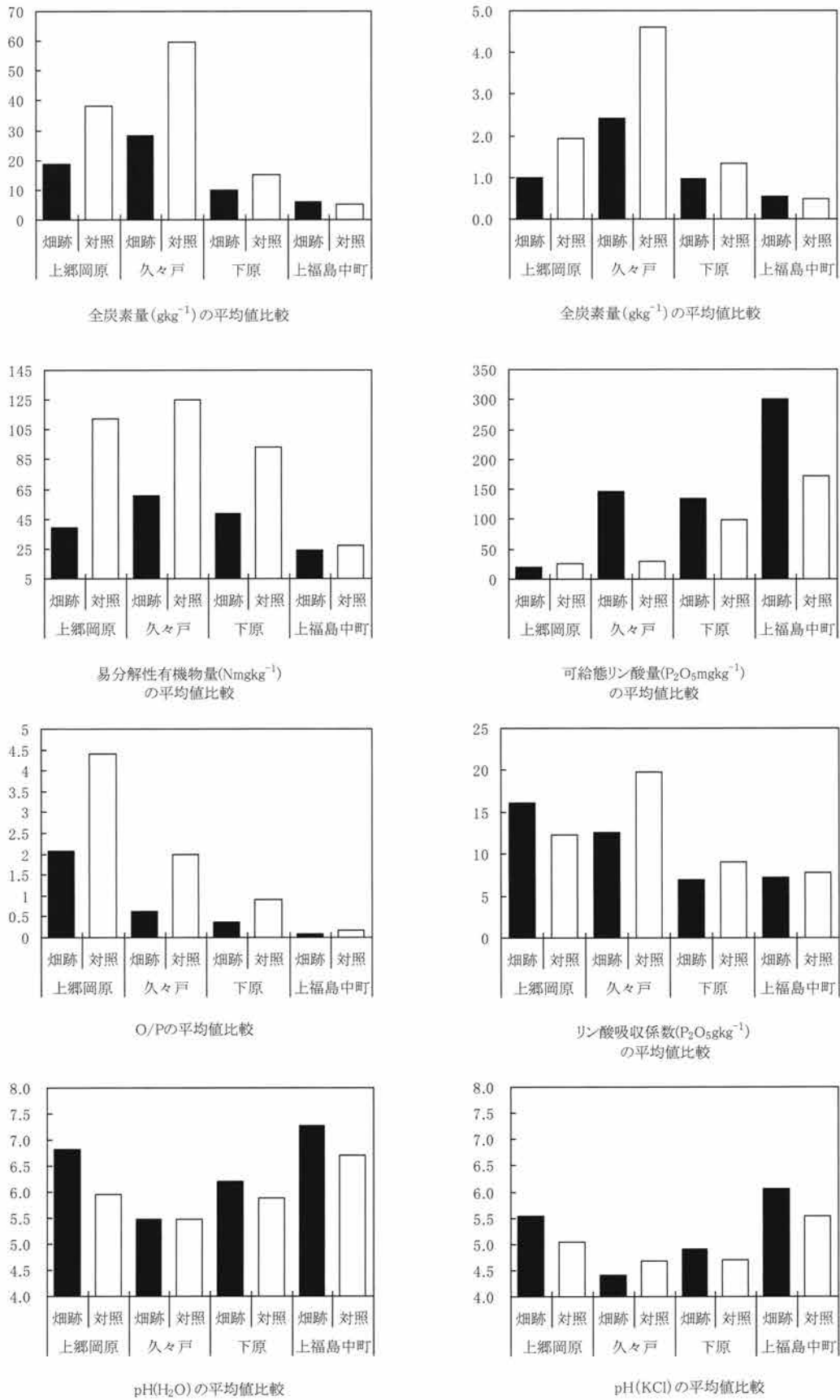
図 1 各遺跡の土壌化学性の比較
