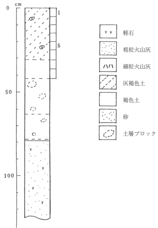
図2 B地点の土層柱状図 数字はテフラ分析の試料番号
