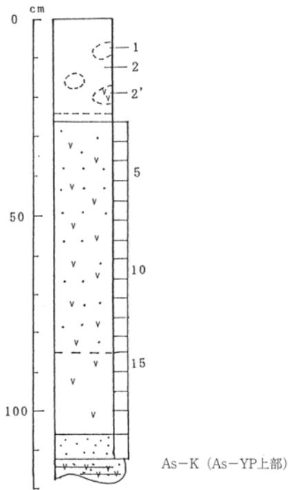
図1 A地点の土層柱状図 数字はテフラ分析の試料番号
