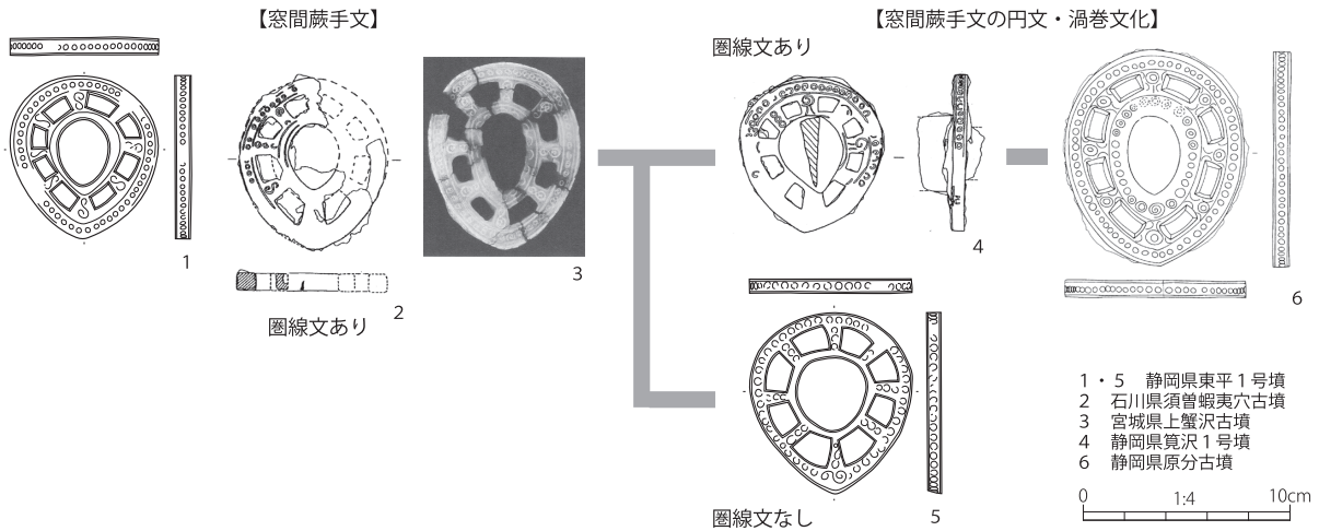
図7 寛沢1号墳出土象嵌装鏝の類例とその位置づけ（大谷 2018 に加筆）
