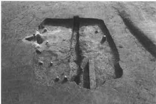
2号住居全景 南から
