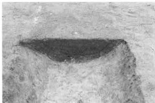
1号溝土層断面D 南から
