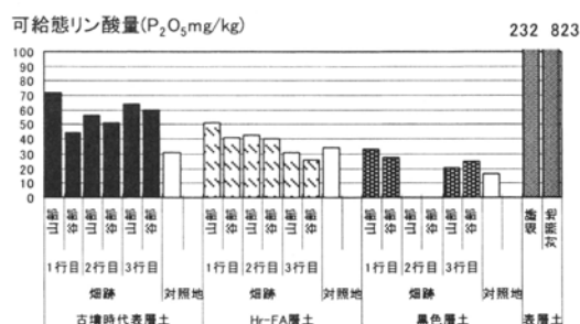
図7 供試土壌試料の可給態リン酸量
