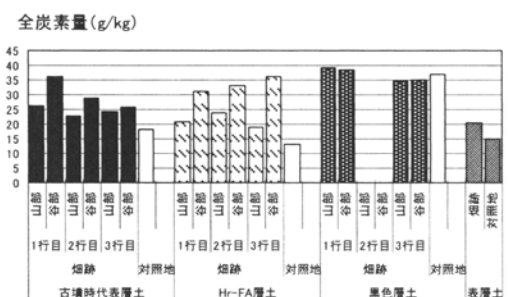
図4 供試土壌試料の全炭素量
