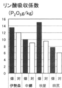
図13 古墳時代代表層土のリン酸吸収係数の平均
