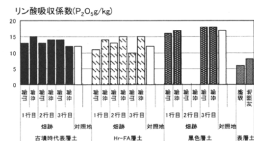
図9 供試土壌試料のリン酸吸収係数
