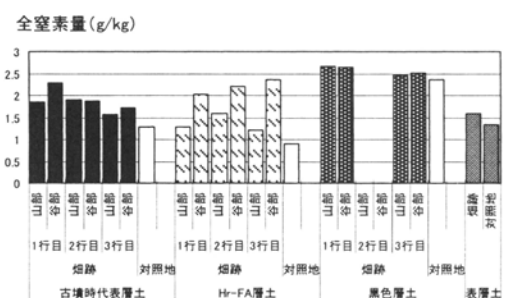
図5 供試土壌試料の全窒素量
