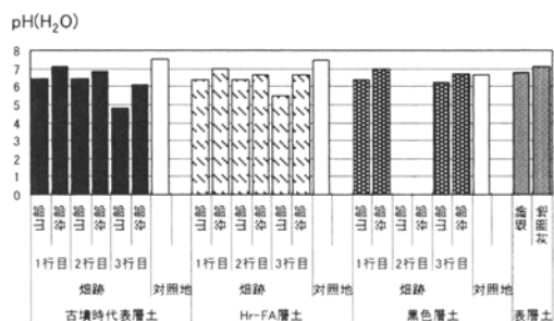
図2 供試土壌試料のpH(H 2 O)
