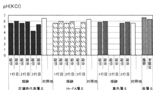
図3 供試土壌試料のpH(KCl)
