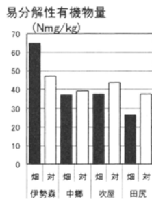
図12 古墳時代代表層土の易分解性有機物の平均
