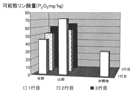
図8 古墳時代表層土の可給態リン酸量
