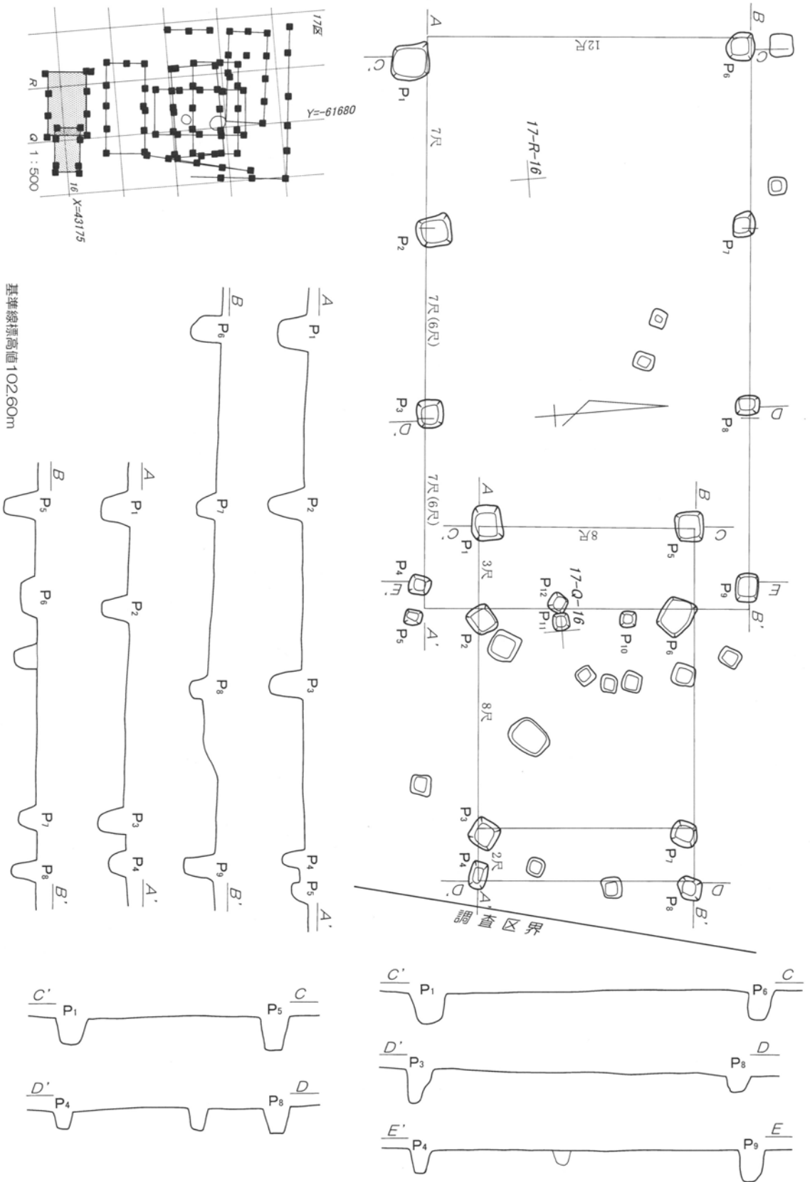
第39図 第1・7号掘立柱建物跡実測図 1 : 60
