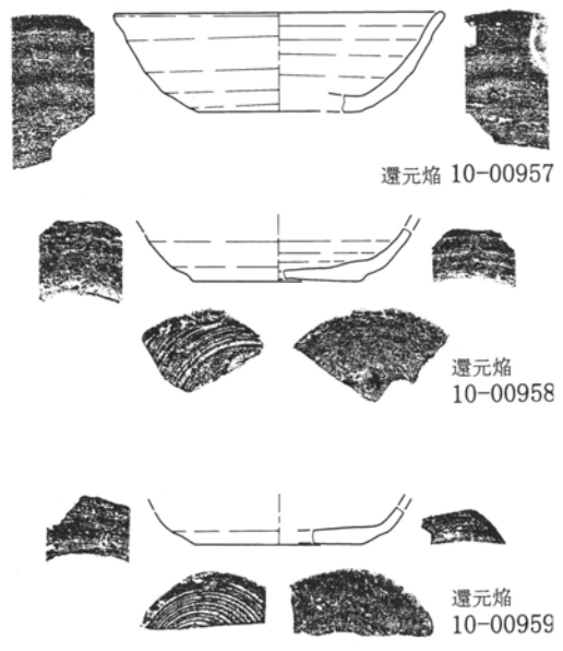
第187図 第40・59号住居跡 1 : 60・第40号住居跡出土遺物実測図 1 : 3 (1)
