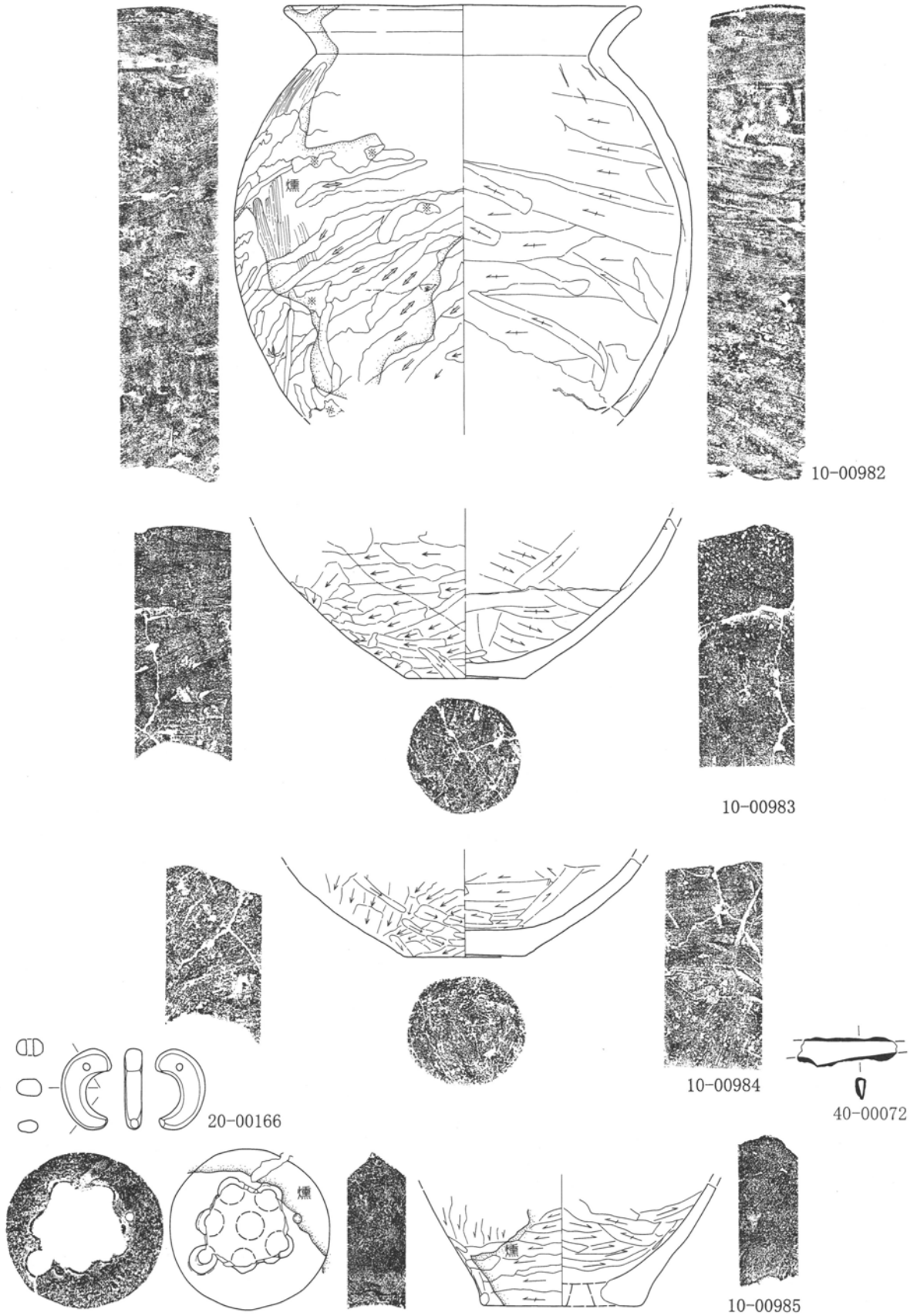
第196図 第42号住居跡出土遺物実測図1:3(5)
