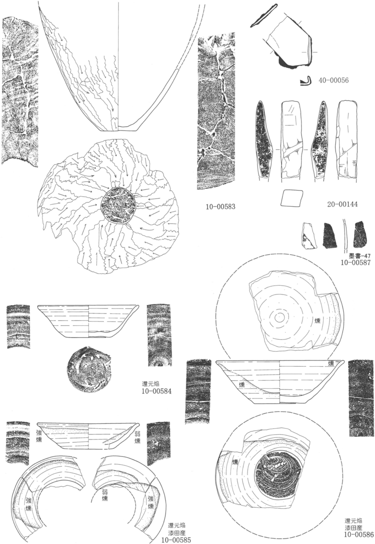
第92図 第2号住居跡出土遺物実測図1:3(2)
