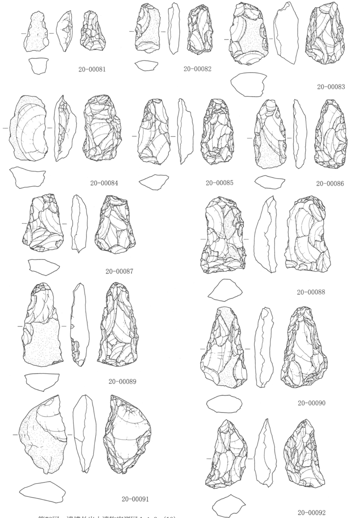
第72図 遺構外出土遺物実測図 1 : 3 (19)
