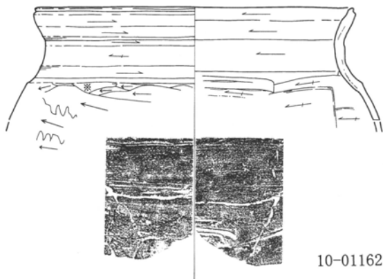
第237図 第65号住居跡 1:60・出土遺物実測図 1:3 (1)
