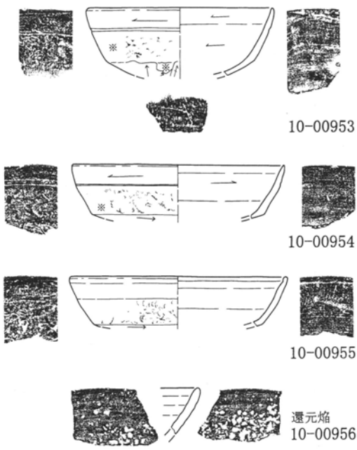
第187図 第40・59号住居跡 1 : 60・第40号住居跡出土遺物実測図 1 : 3 (1)
