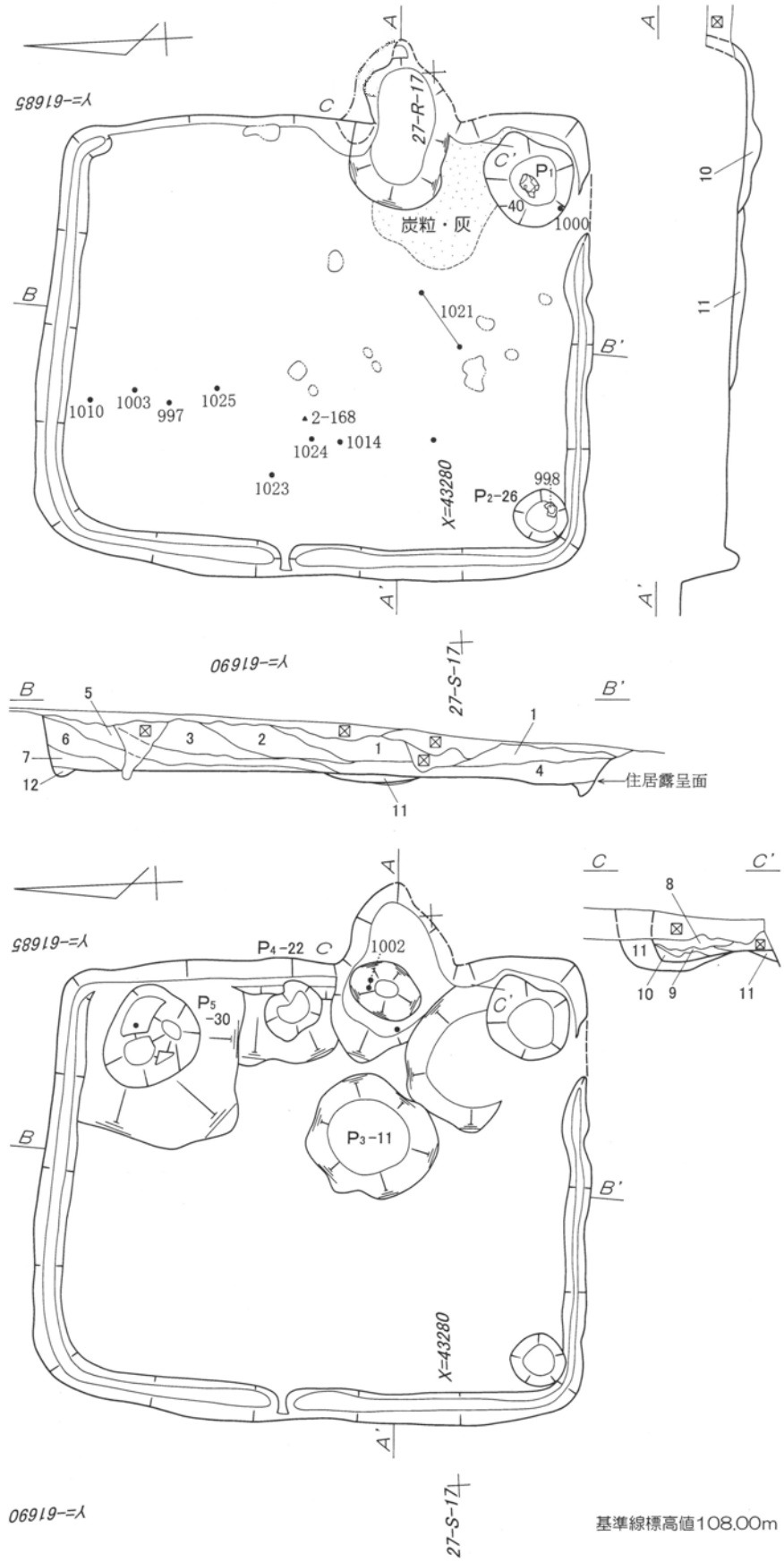
第201図 第45号住居跡実測図 1 : 60
