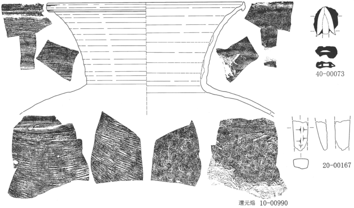
第199図 第44号住居跡出土遺物実測図 1 : 3 (2)
