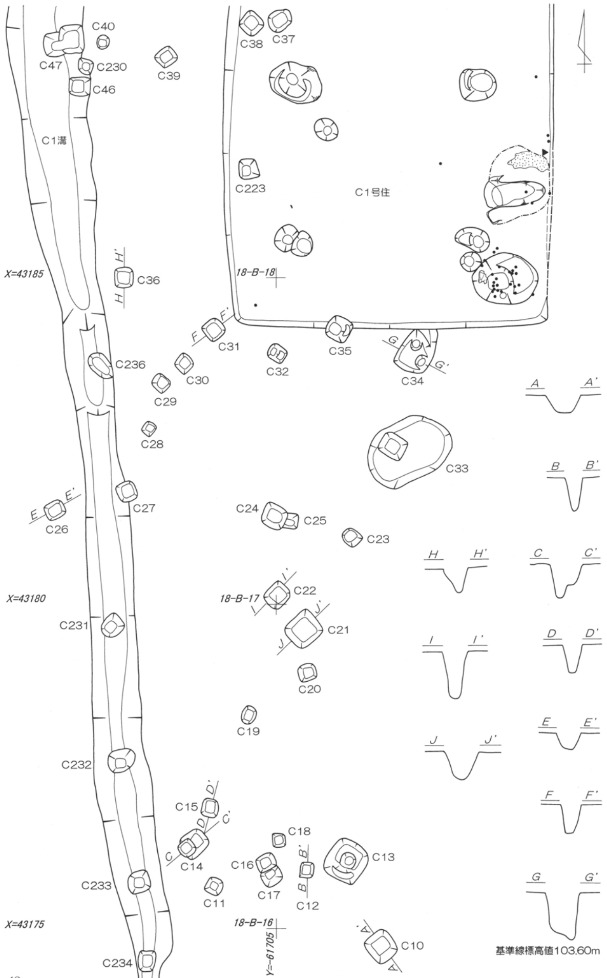
第52図 土坑実測図 1 : 60 (3)
