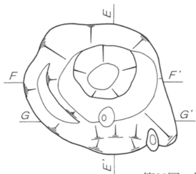
第33図 第1号住居跡 1:60・竈1:30実測図
