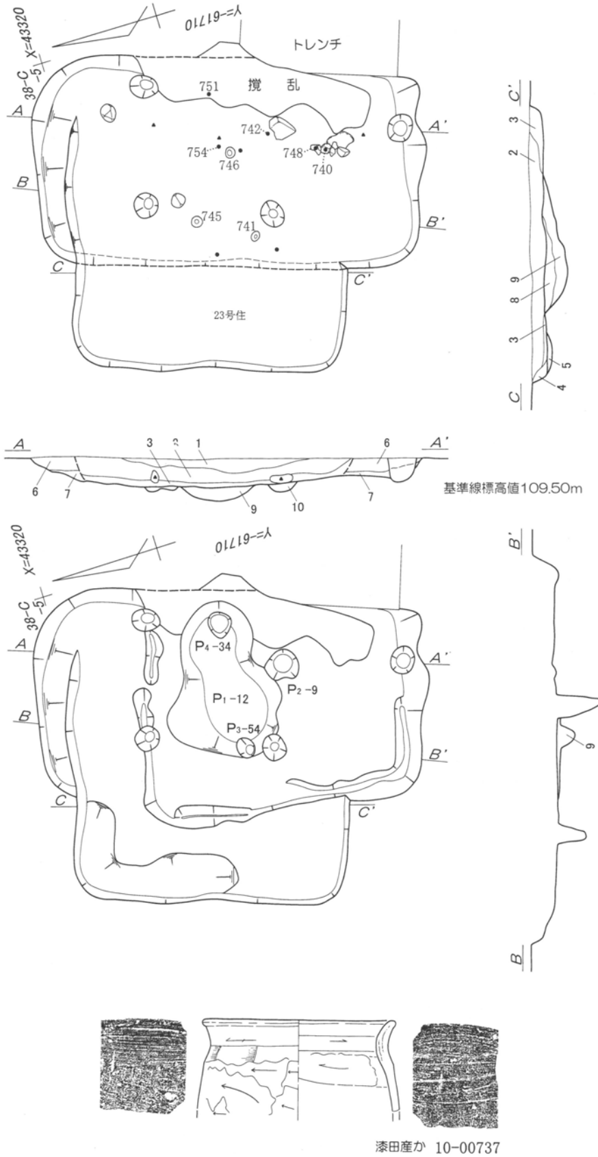
第140図 第22号住居跡 1 : 60・出土遺物実測図 1 : 3 (2)
