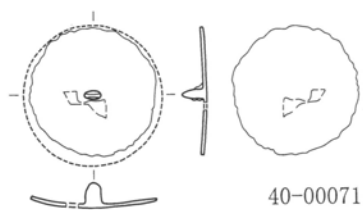
第186図 第39号住居跡出土遺物実測図 1 : 3 (3)
