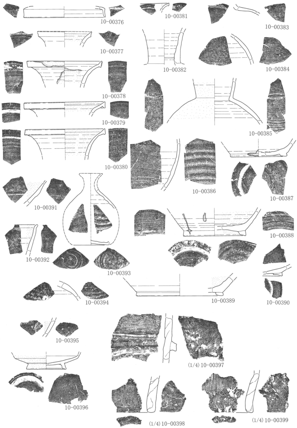
第63図 遺構外出土遺物実測図 1 : 3 · 1 : 4 (10)
