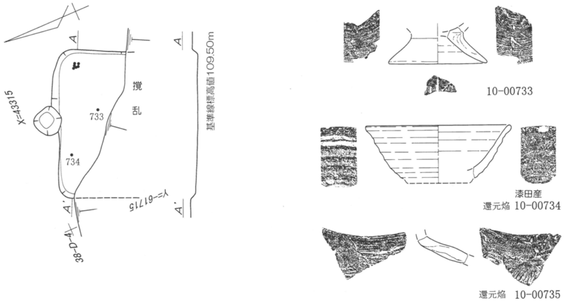
第138図 第21号住居跡 1 : 60・出土遺物実測図 1 : 3
