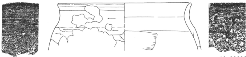
第99図 第4号住居跡1:60・出土遺物実測図1:3(1)
