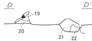
第34図 第2号住居跡 1:60・竈 1:30実測図
