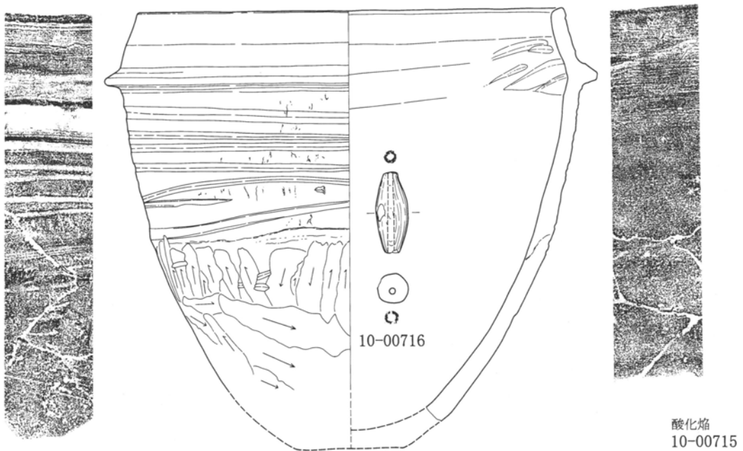
第130図 第17号住居跡出土遺物実測図 1 : 3 (4)
