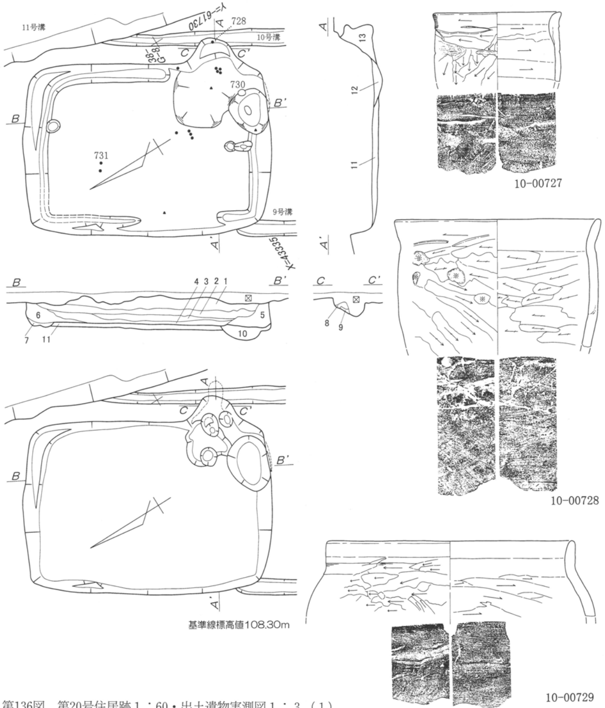
第136図 第20号住居跡 1 : 60 • 出土遺物実測図 1 : 3 (1)
