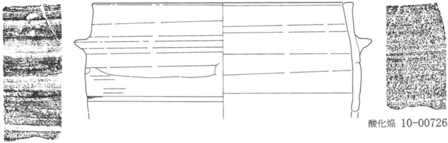
第135図 第19号住居跡出土遺物実測図 1 : 3 (3)
