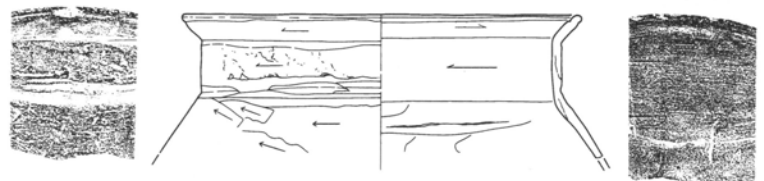
第121図 第13号住居跡 1 : 60 ・ 出土遺物実測図 1 : 3
