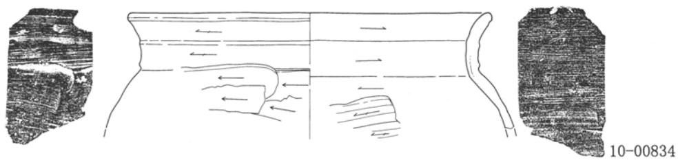
第160図 第31号住居跡出土遺物実測図1:3(1)
