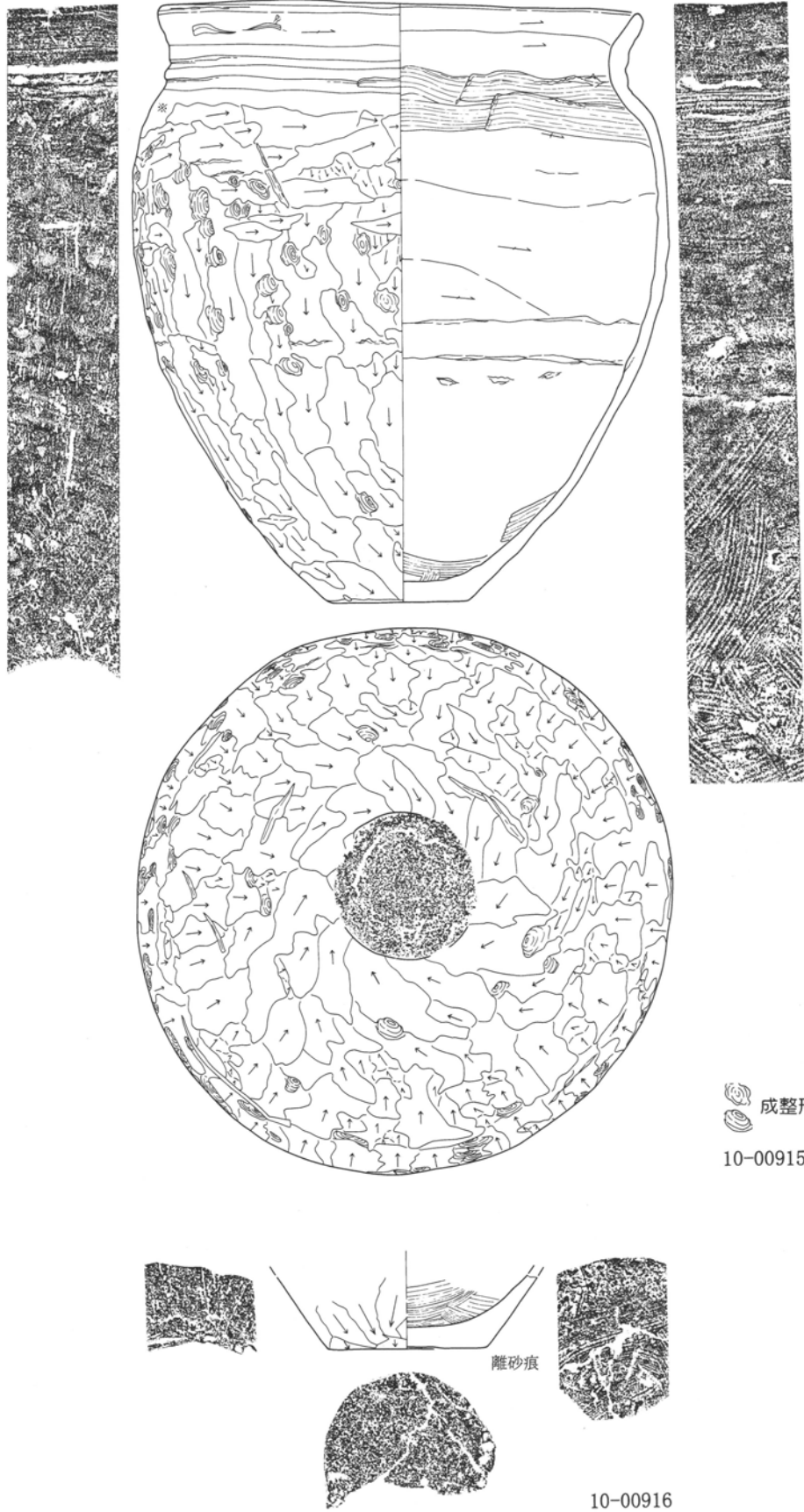
第178図 第38号住居跡出土遺物実測図 1 : 3 (3)
