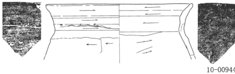
第184図 第39号住居跡出土遺物実測図 1 : 3 ( 1 )
