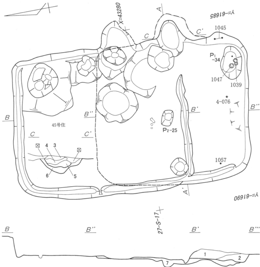
第207図 第47号住居跡実測図 1 : 60
