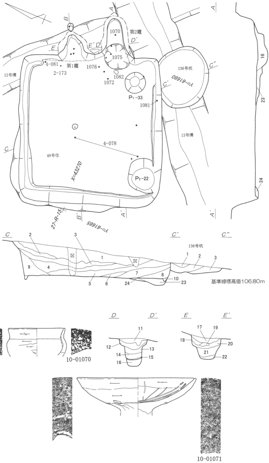
第214図 第49号住居跡 1:60・出土遺物実測図 1:3 (1)
