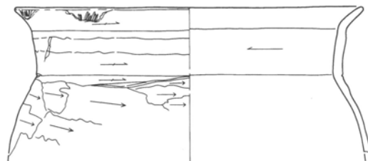
第173図 第37号住居跡出土遺物実測図 1 : 3 (1)
