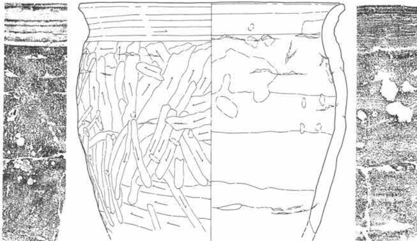
第129図 第17号住居跡竈 1:30・出土遺物実測図 1:3 (3)
