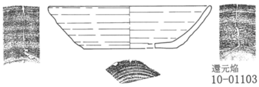
第223図 第52号住居跡 1 : 60 ・ 出土遺物実測図 1 : 3 (1)
