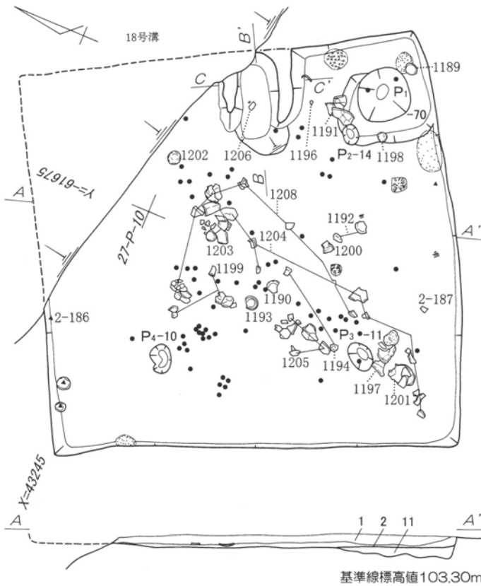
第247図 第68号住居跡 1 : 60・出土遺物実測図 1 : 3 (1)
