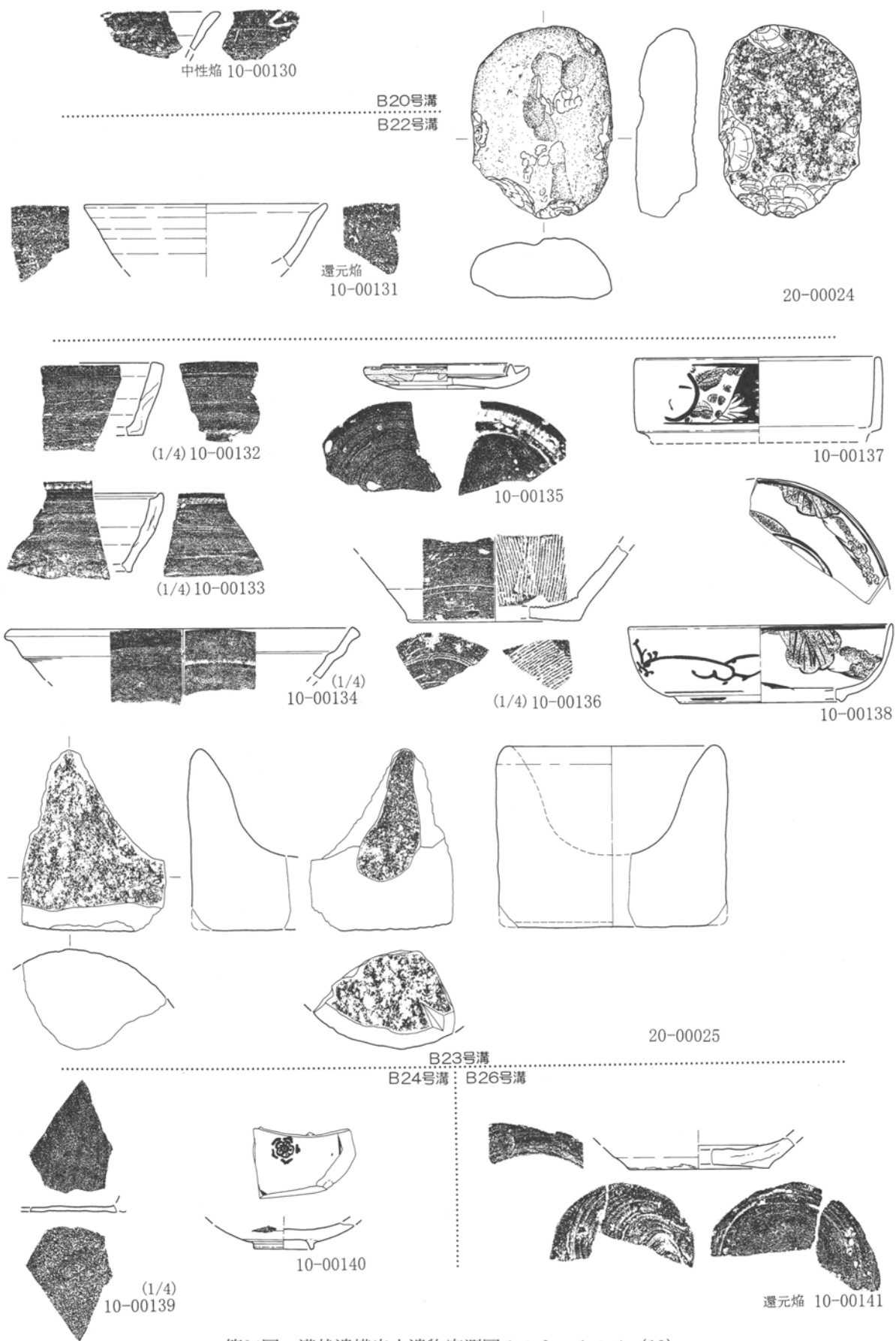
第24図 溝状遺構出土遺物実測図 1 : 3 · 1 : 4 (18)
