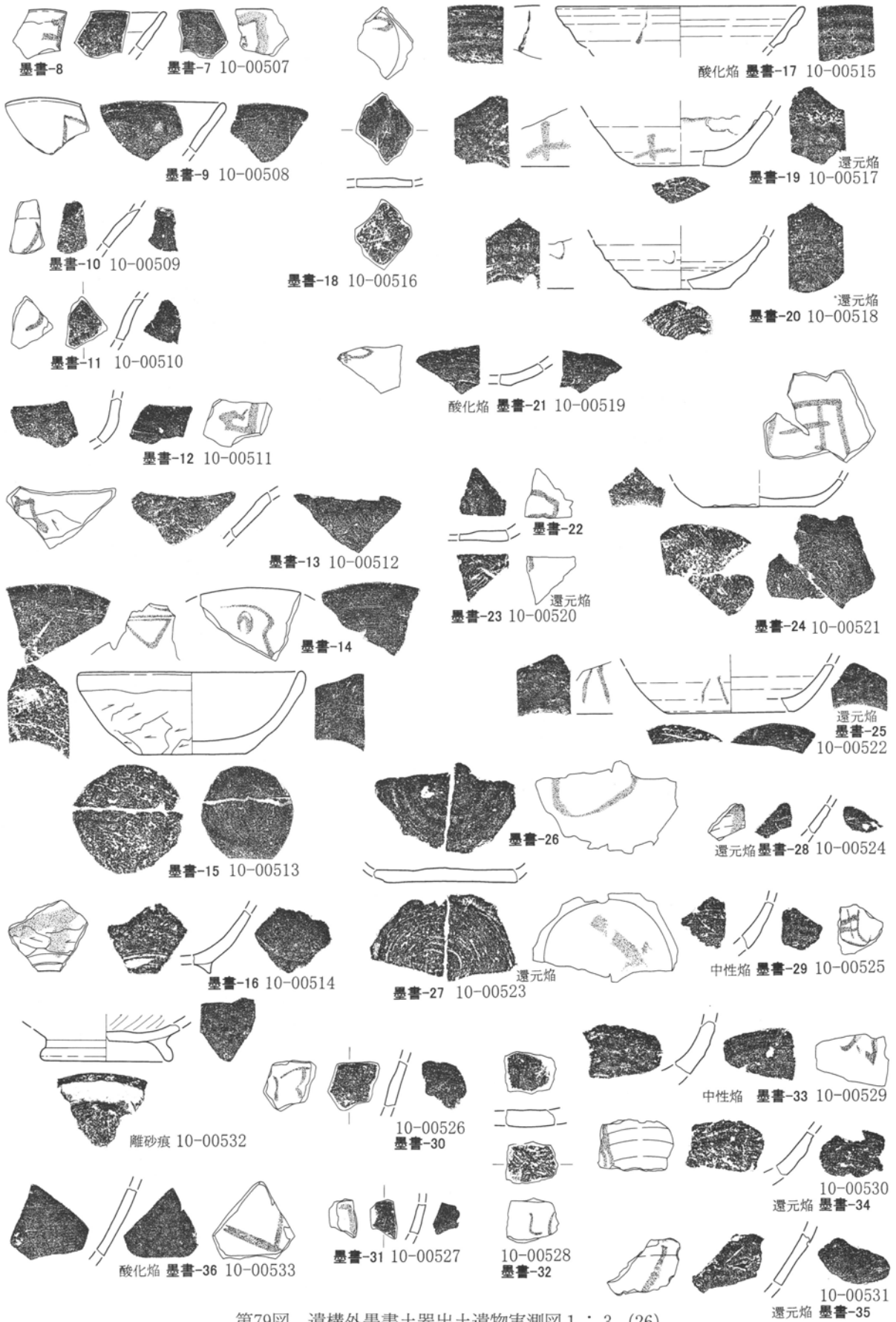
第79図 遺構外墨書土器出土遺物実測図 1 : 3 (26)
