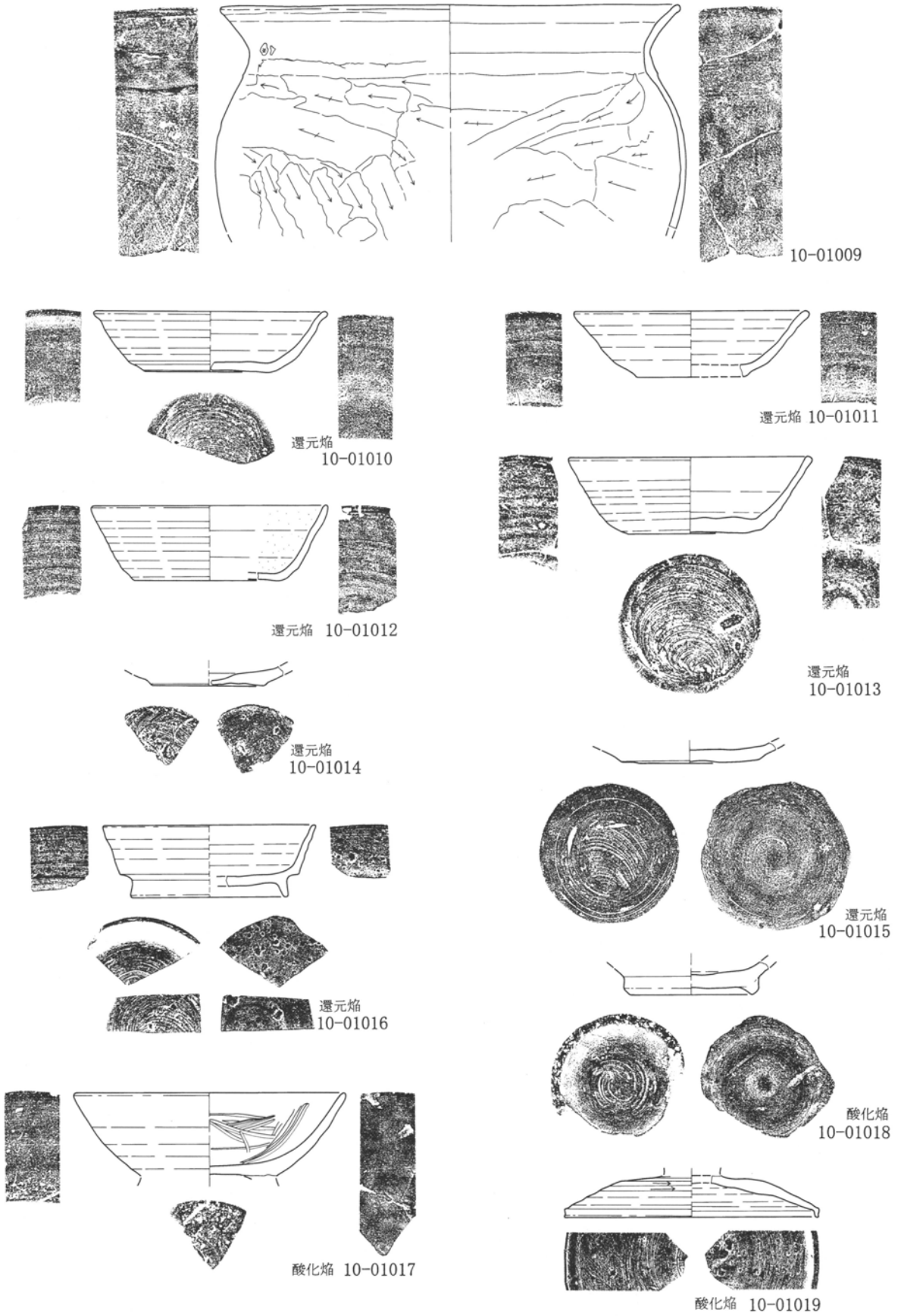
第203図 第45号住居跡出土遺物実測図 1 : 3 (2)
