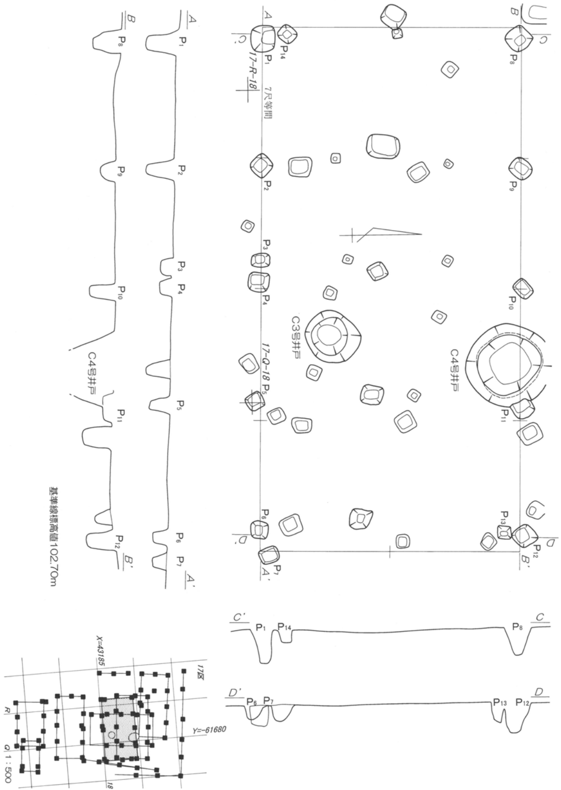
第41図 第3号掘立柱建物跡実測図 1:60
