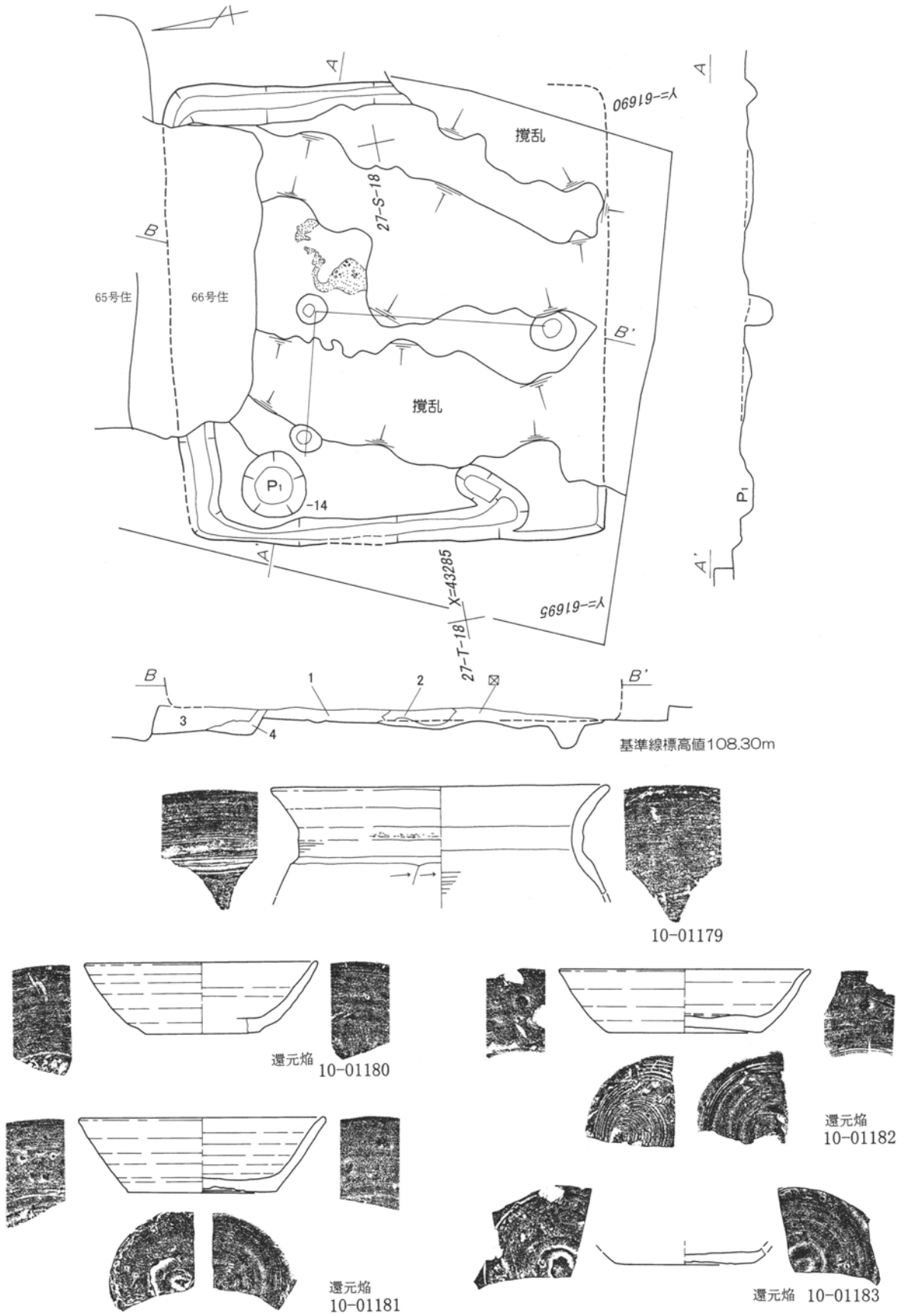
第245図 第67号住居跡 1 : 60・出土遺物実測図 1 : 3 (2)
