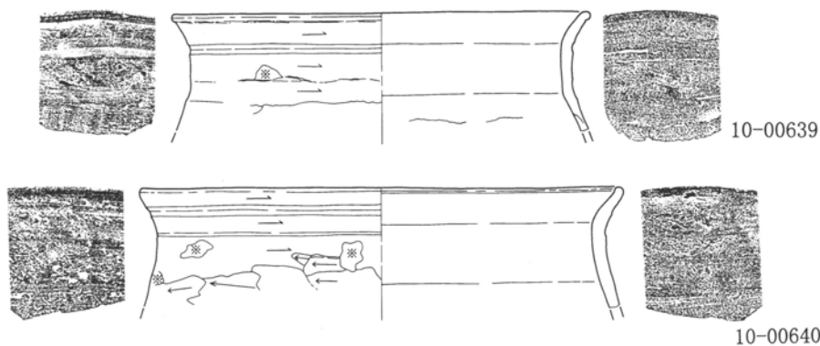
第107図 第5号住居跡出土遺物実測図 1 : 3
