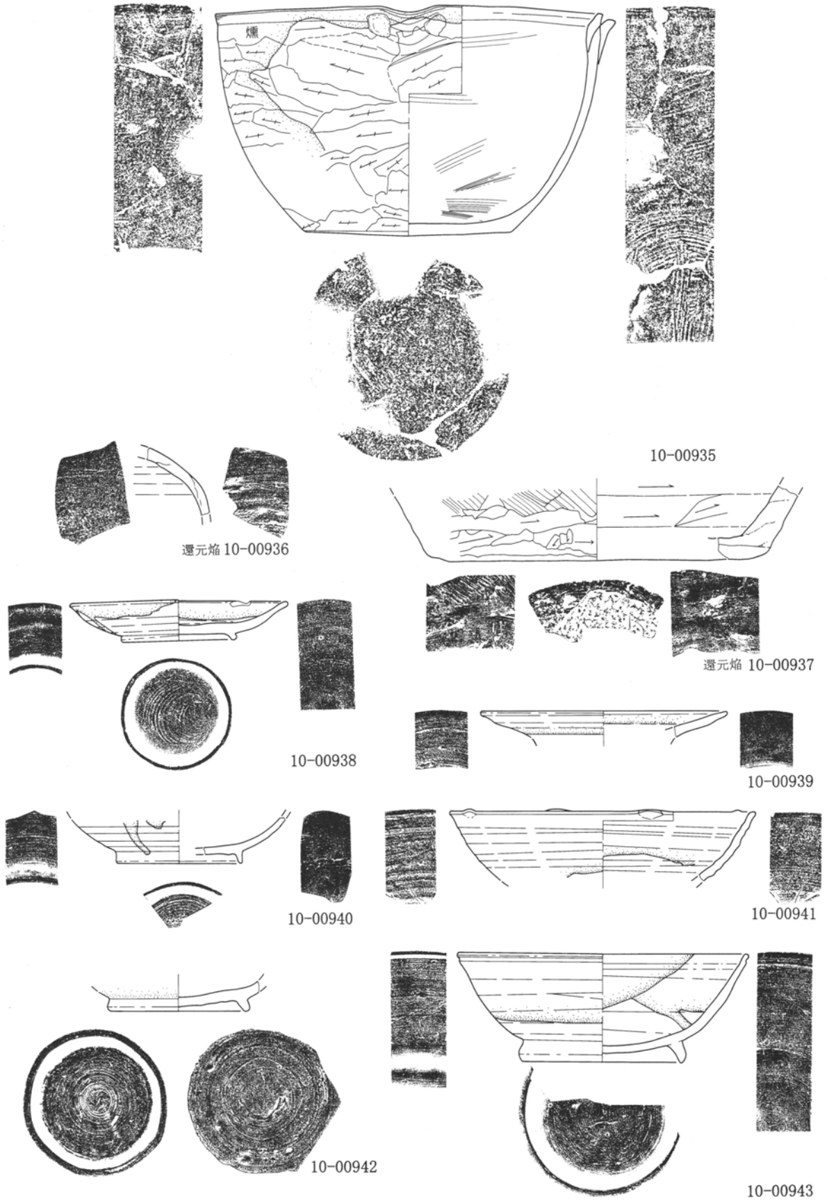
第182図 第38号住居跡出土遺物実測図 1 : 3 (7)
