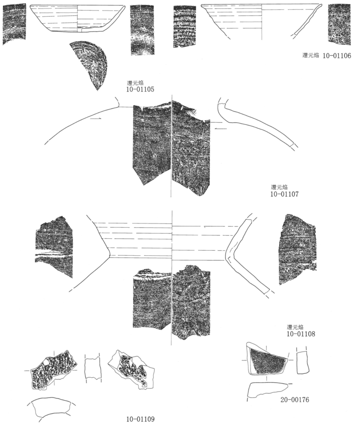
第224図 第52号住居跡出土遺物実測図 1 : 3 (2)
