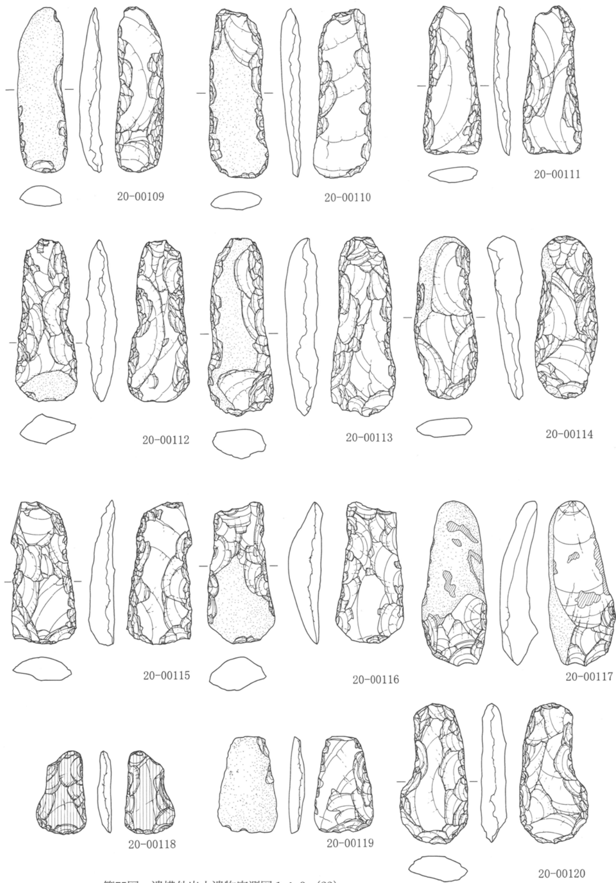
第75図 遺構外出土遺物実測図 1 : 3 (22)
