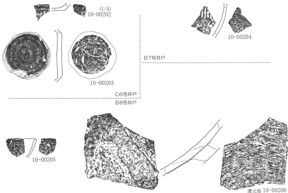
第49図 井戸跡出土遺物実測図 1 : 3 (4)
