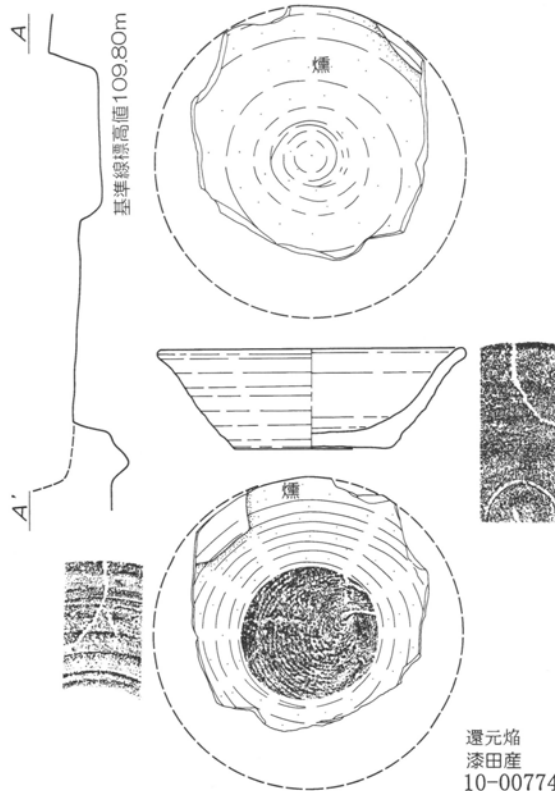
第150図 第26号住居跡 1 : 60・出土遺物実測図 1 : 3 (1)
