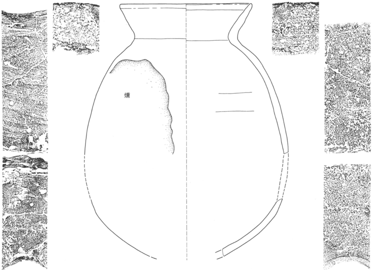
第251図 第68号住居跡出土遺物実測図 1 : 3 (5)
