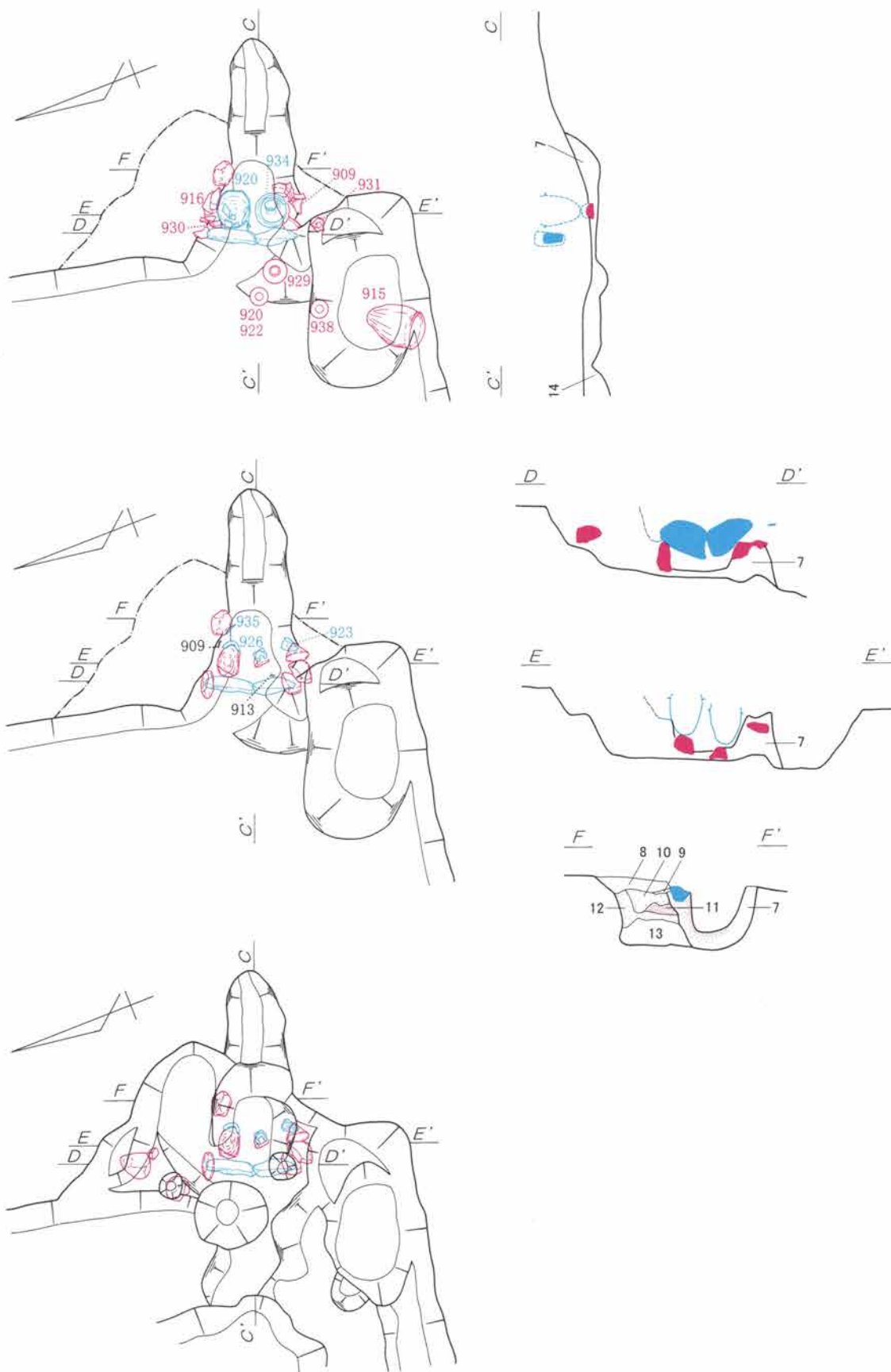
第176図 第38号住居跡電実測図 1 : 40
