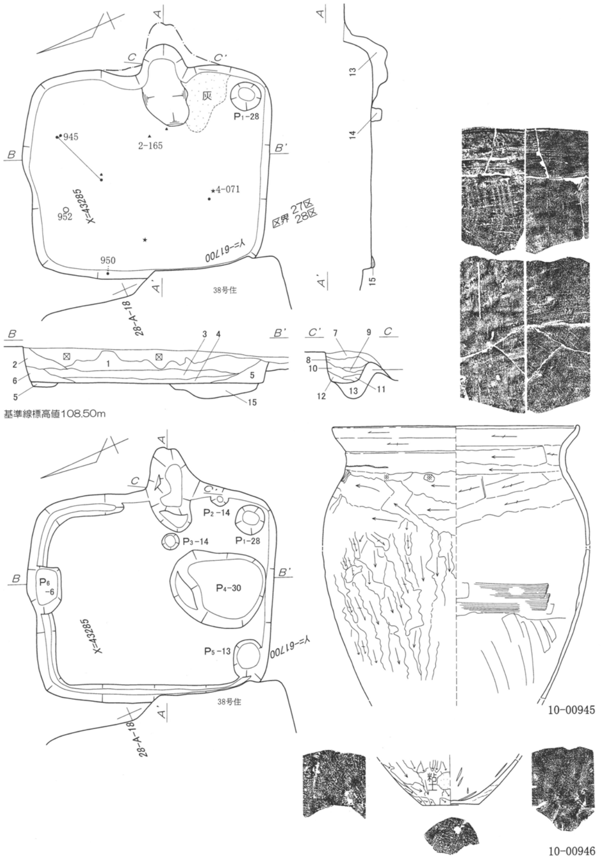
第185図 第39号住居跡 1:60・出土遺物実測図 1:3 (2)
