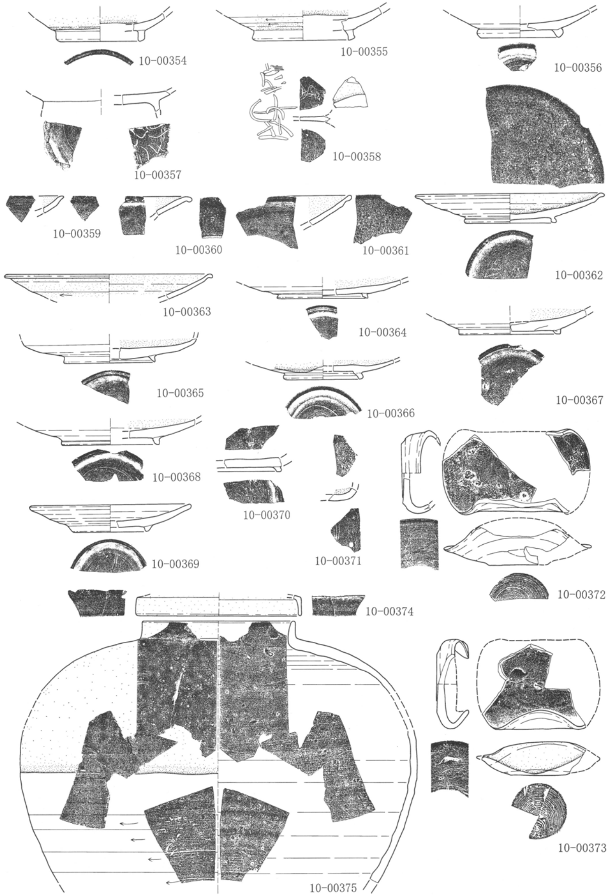
第62図 遺構外出土遺物実測図 1 : 3 (9)
