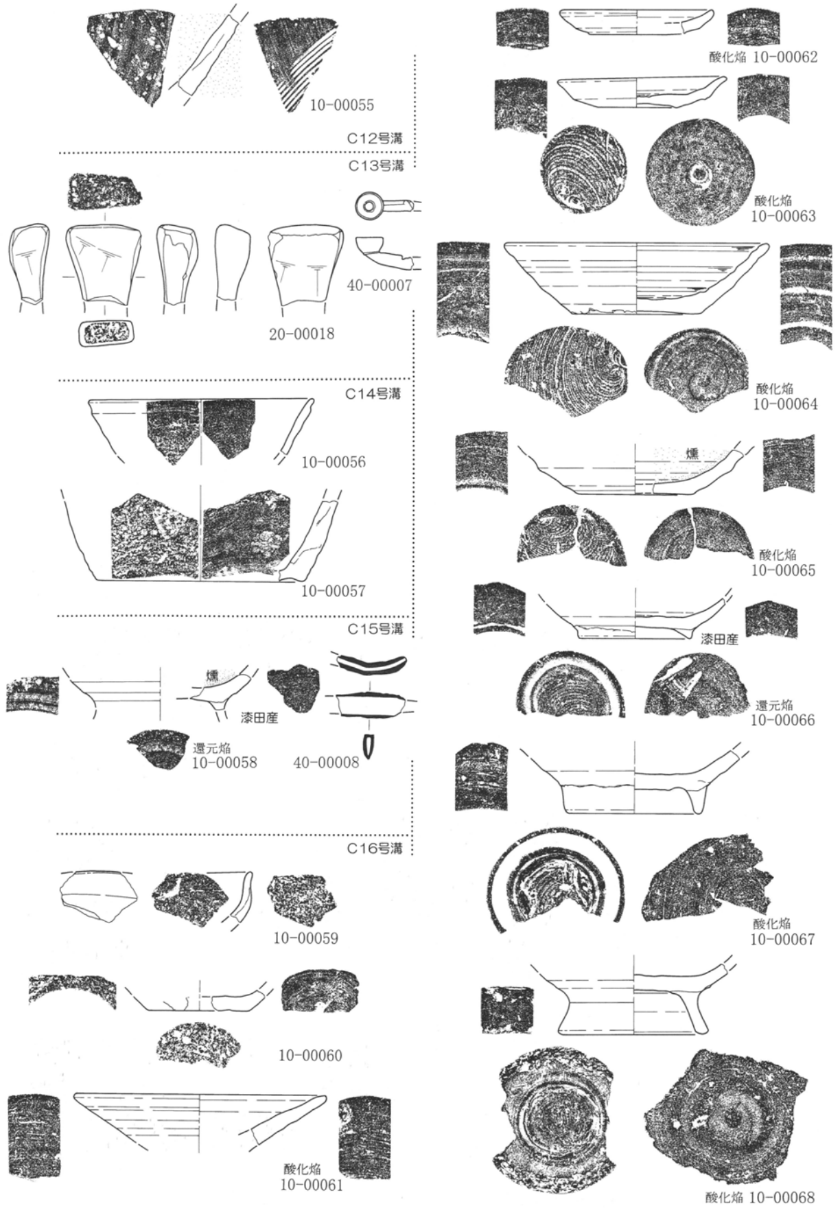
第17図 溝状遺構出土遺物実測図 1 : 3 (12)
