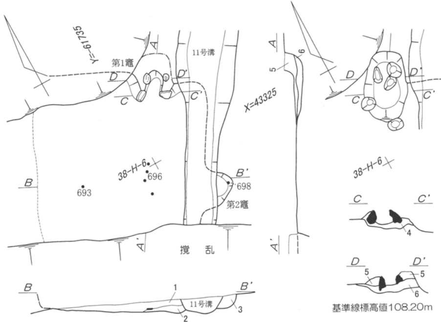
第122図 第14号住居跡 1 : 60・出土遺物実測図 1 : 3
