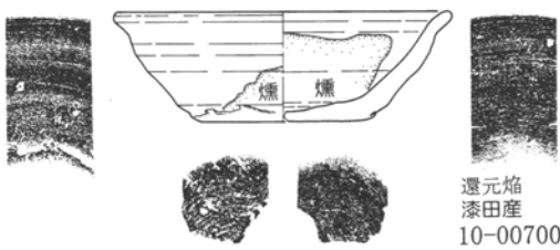
第125図 第16号住居跡 1 : 60・出土遺物実測図 1 : 3 (1)
