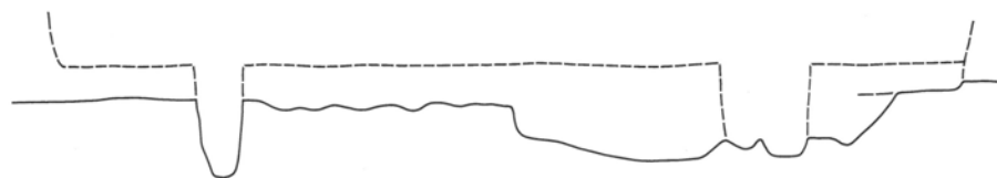
第217図 第50号住居跡実測図 1 : 60
