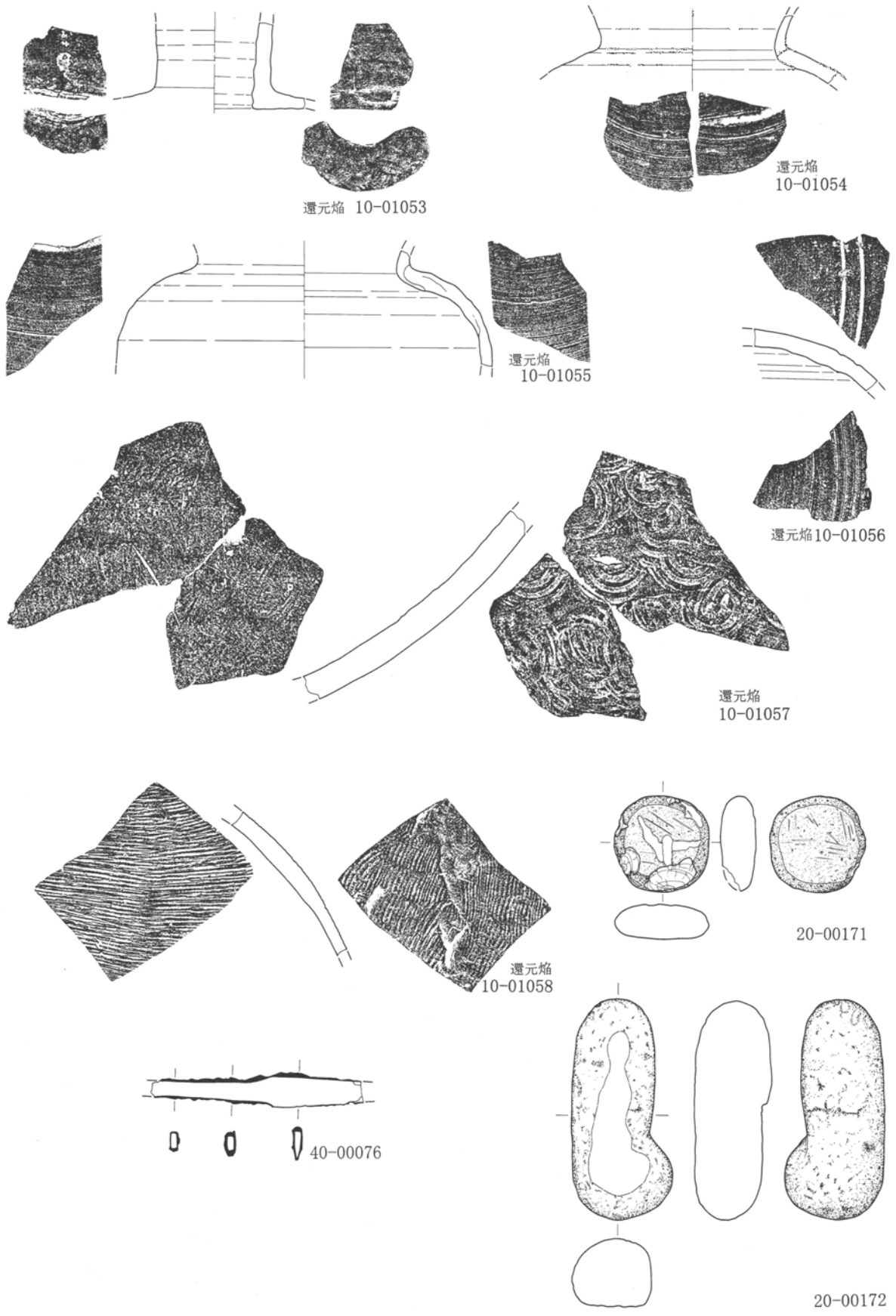
第210図 第47号住居跡出土遺物実測図 1 : 3 (3)
