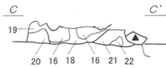
第34図 第2号住居跡 1:60・竈 1:30実測図
