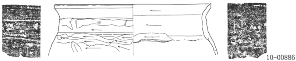
第170図 第36号住居跡出土遺物実測図1：3（2）
