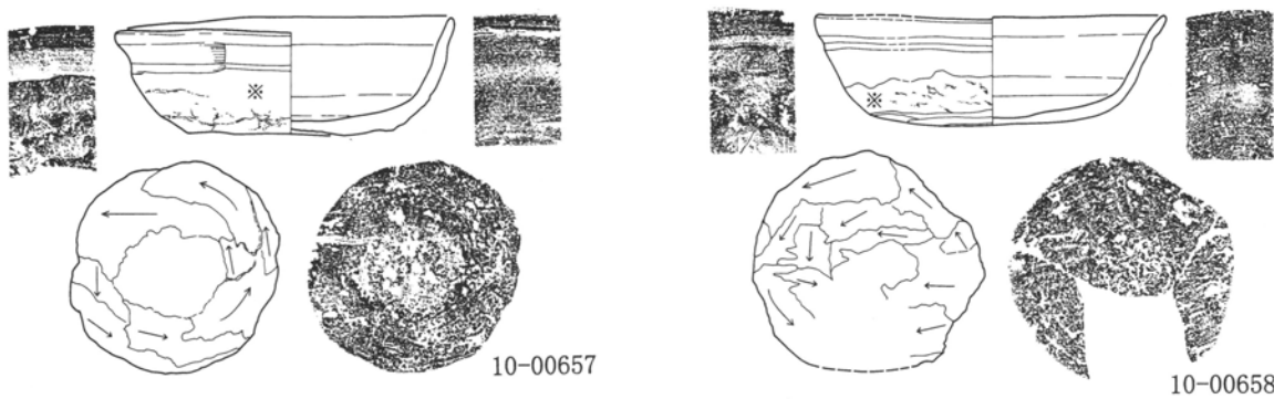
第113図 第9号住居跡 1 : 60・出土遺物実測図 1 : 3 (1)
