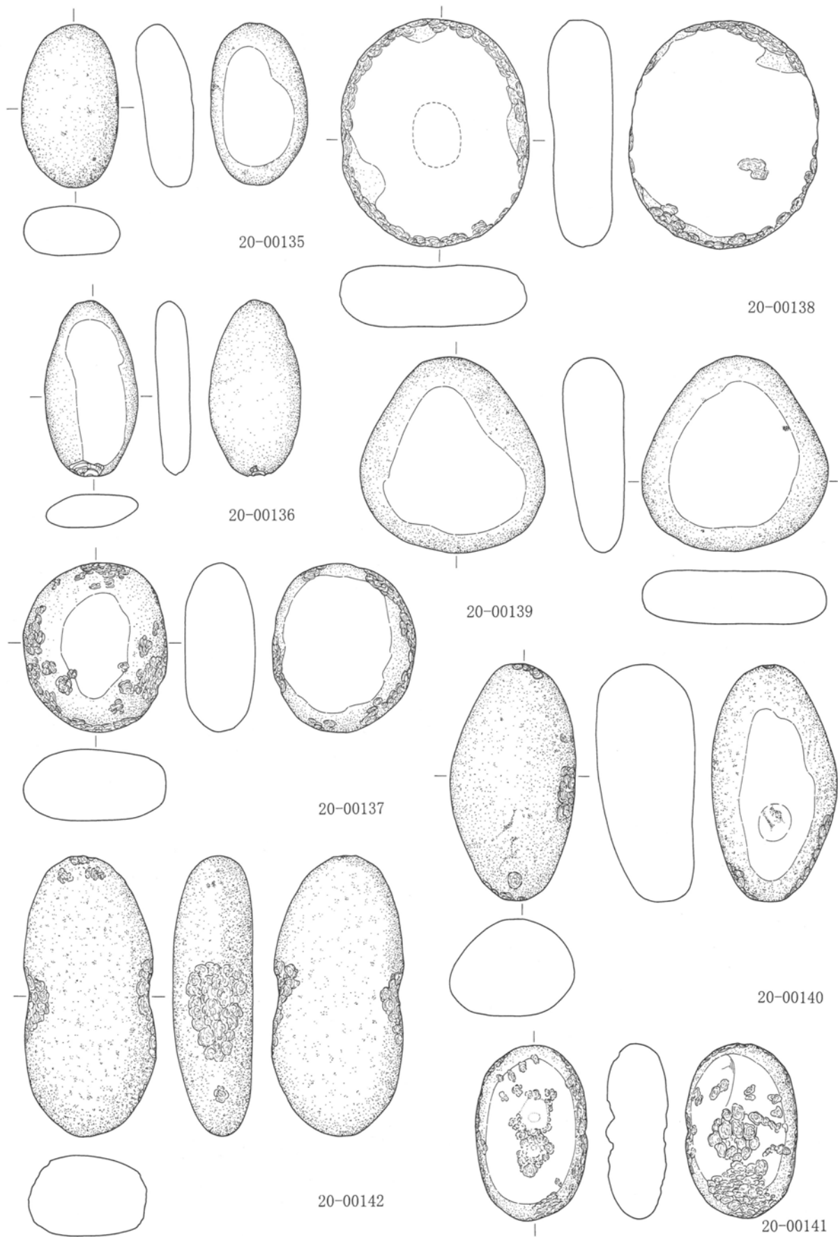
第78図 遺構外出土遺物実測図 1 : 3 (25)
