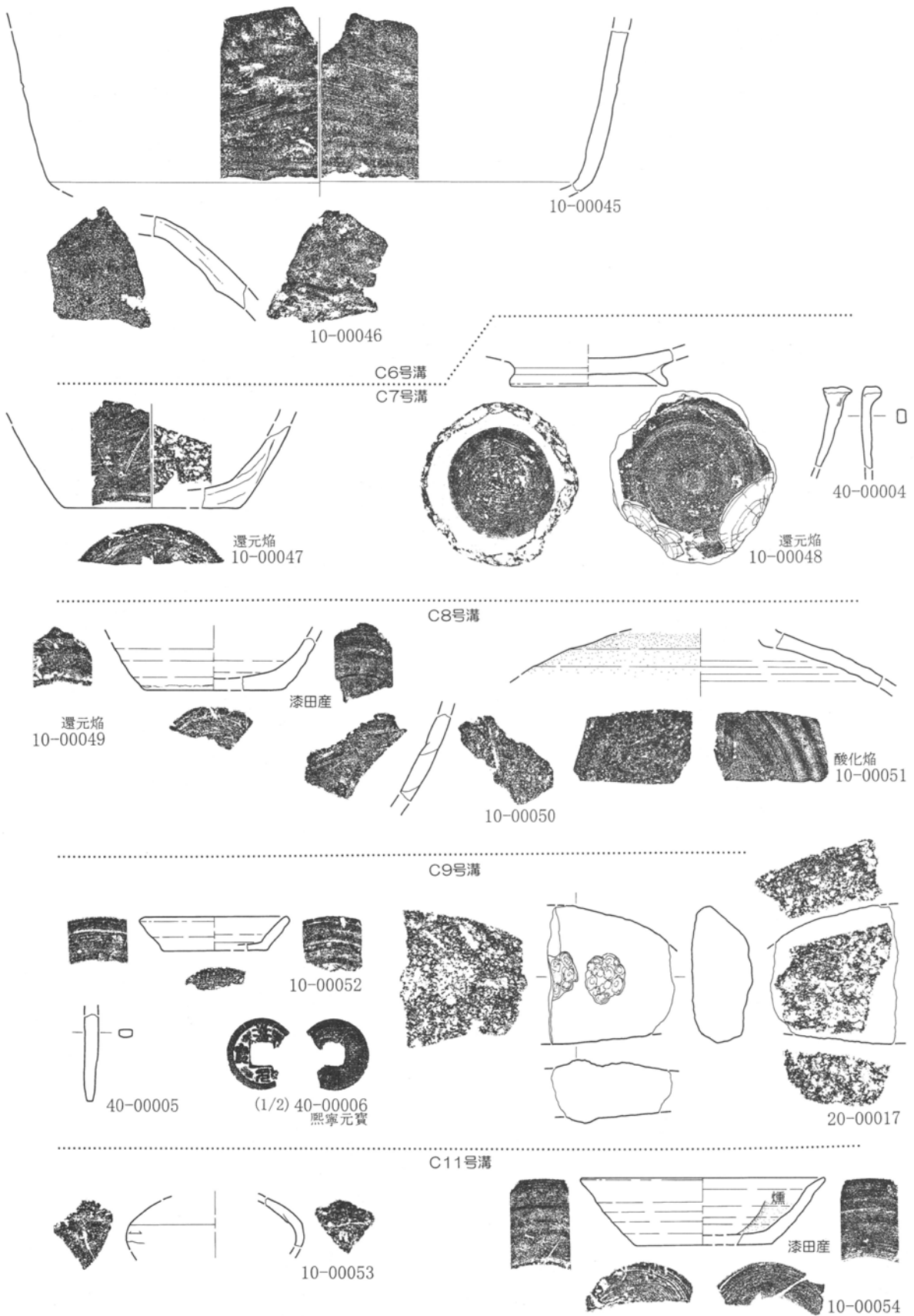
第16図 溝状遺構出土遺物実測図 1 : 2 · 1 : 3 (11)
