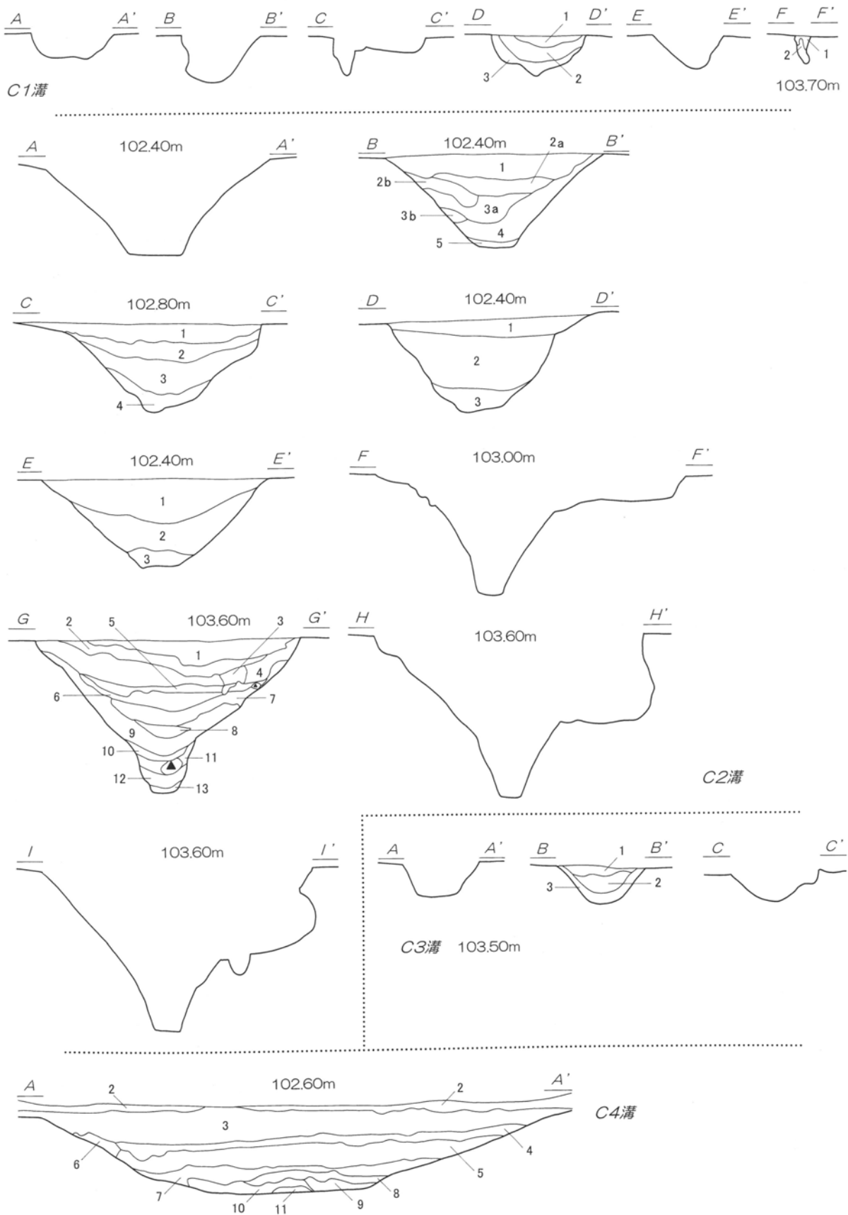
第1図 第1～4号溝状遺構土層断面図 1 : 60
