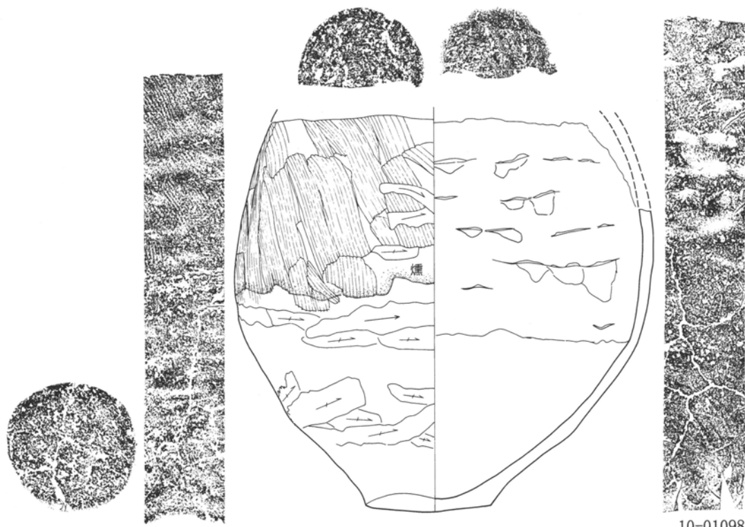
第221図 第50号住居跡出土遺物実測図 1 : 3 (3)
