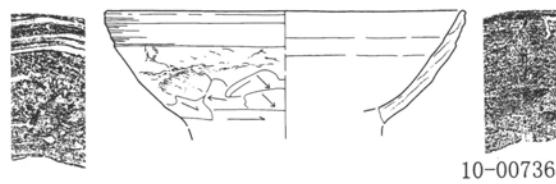
第139図 第22号住居跡出土遺物実測図 1 : 3 (1)
