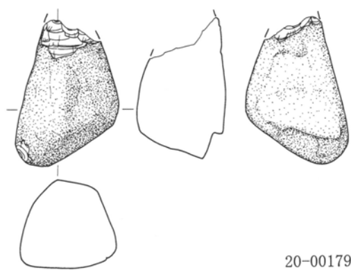
第235図 第63号住居跡 1:30・出土遺物実測図 1:3
