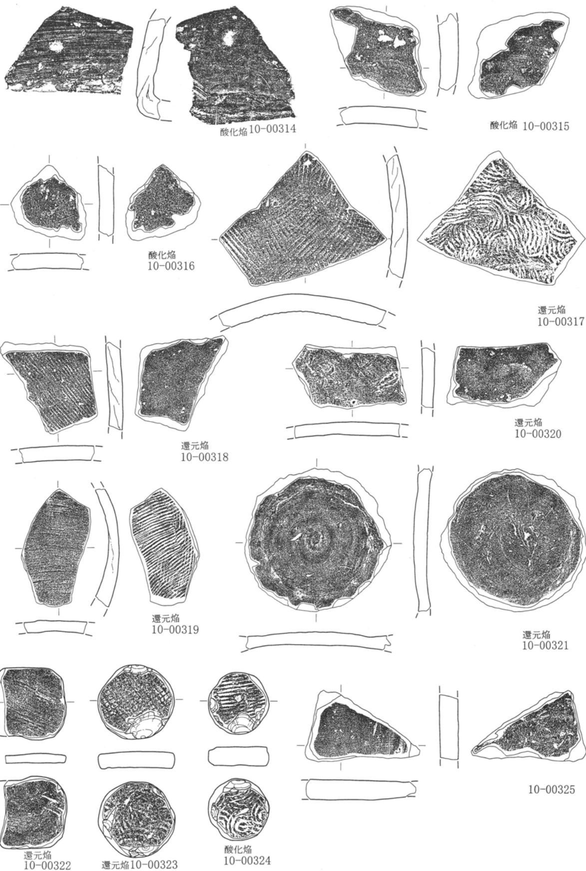
第60図 遺構外出土遺物実測図 1 : 3 ( 7 )
