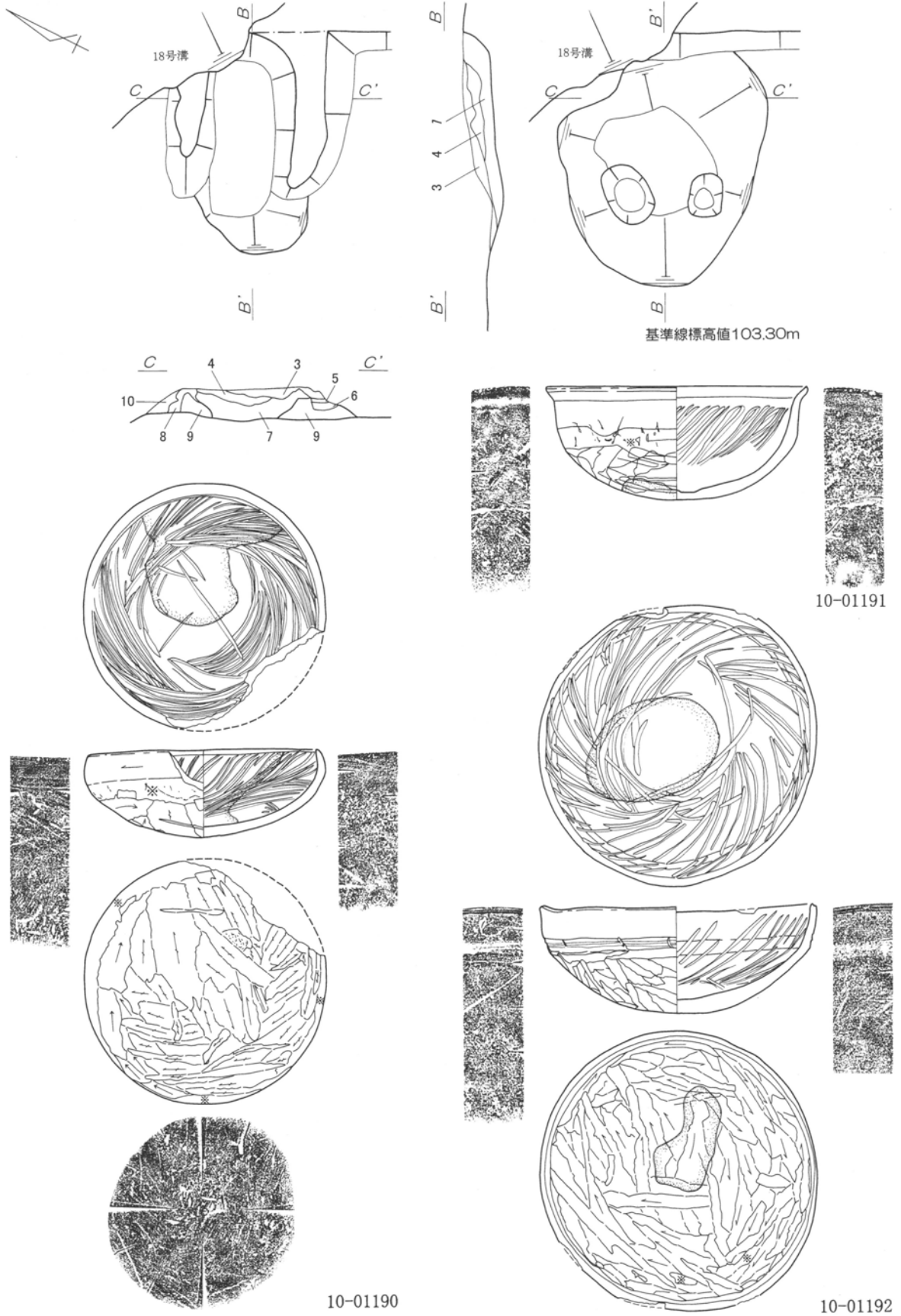
第248図 第68号住居跡竈 1 : 30 • 出土遺物実測図 1 : 3 (2)
