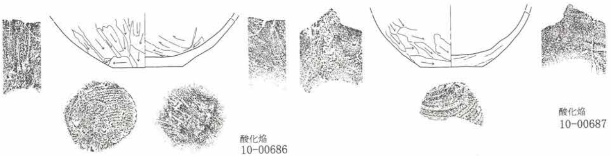
第120図 第12号住居跡竈 1:30・出土遺物実測図 1:3 (2)
