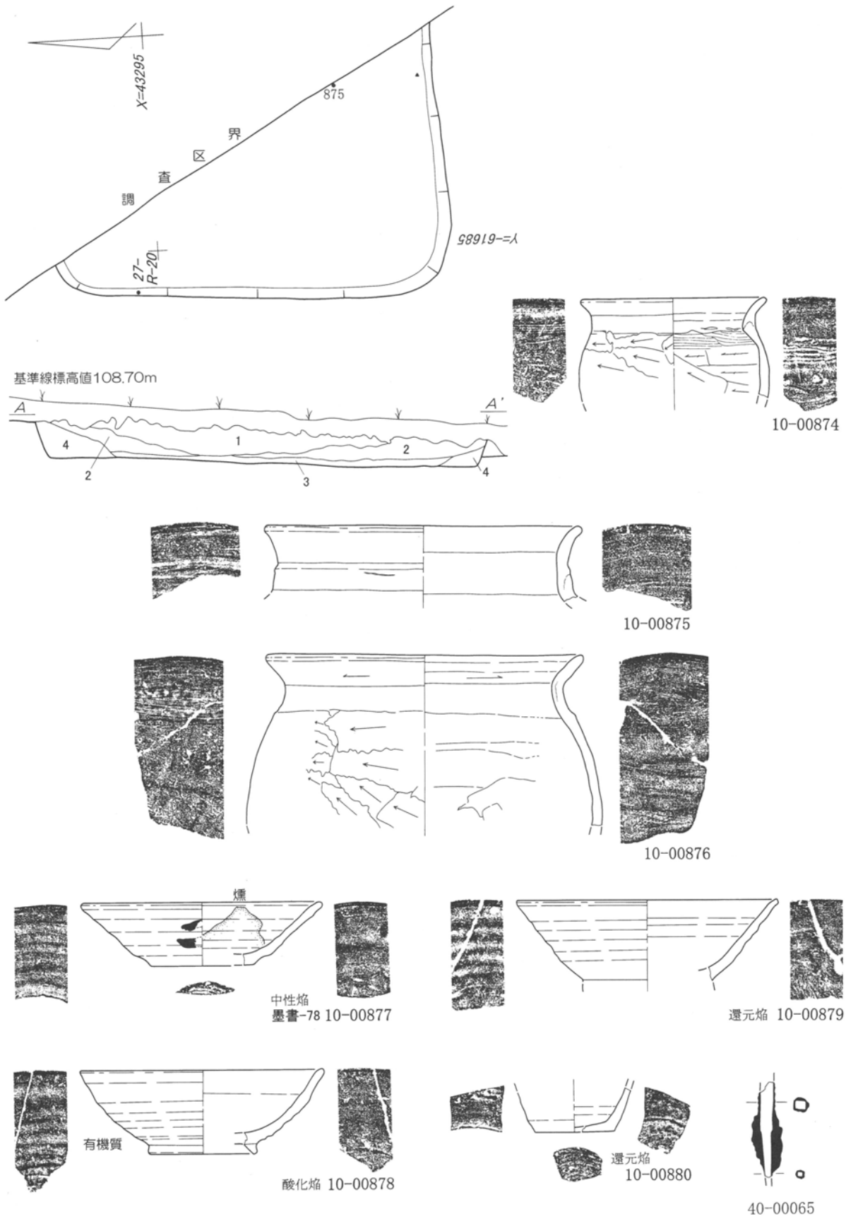
第168図 第35号住居跡 1 : 60・出土遺物実測図 1 : 3
