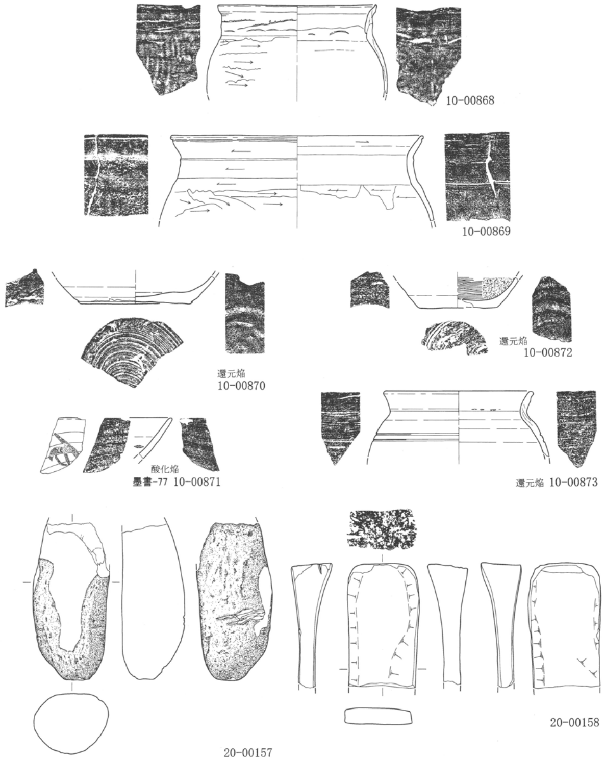
第167図 第34号住居跡出土遺物実測図 1 : 3 (3)
