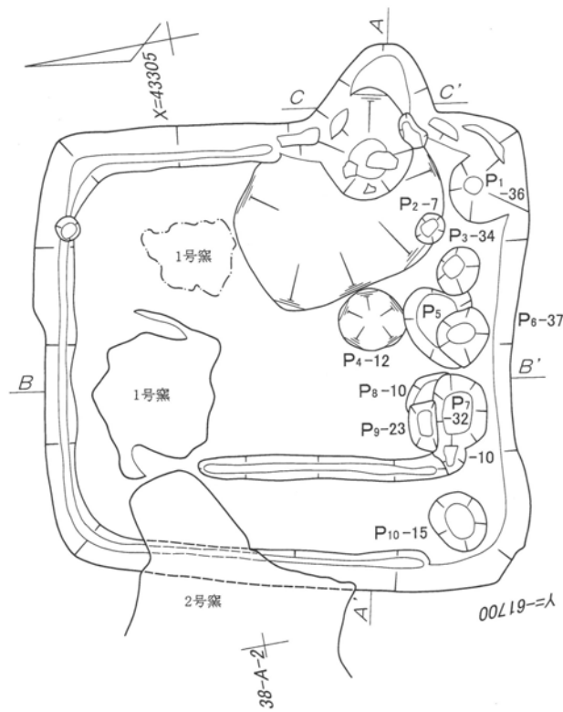
第166図 第34号住居跡 1 : 60・出土遺物実測図 1 : 3 (2)
