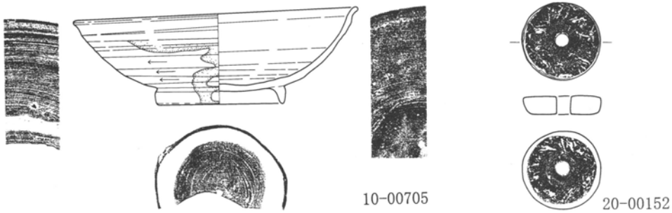
第126図 第16号住居跡出土遺物実測図 1 : 3 (2)
