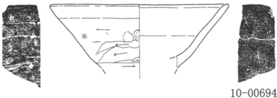
第123図 第15号住居跡 1 : 60・出土遺物実測図 1 : 3 (1)
