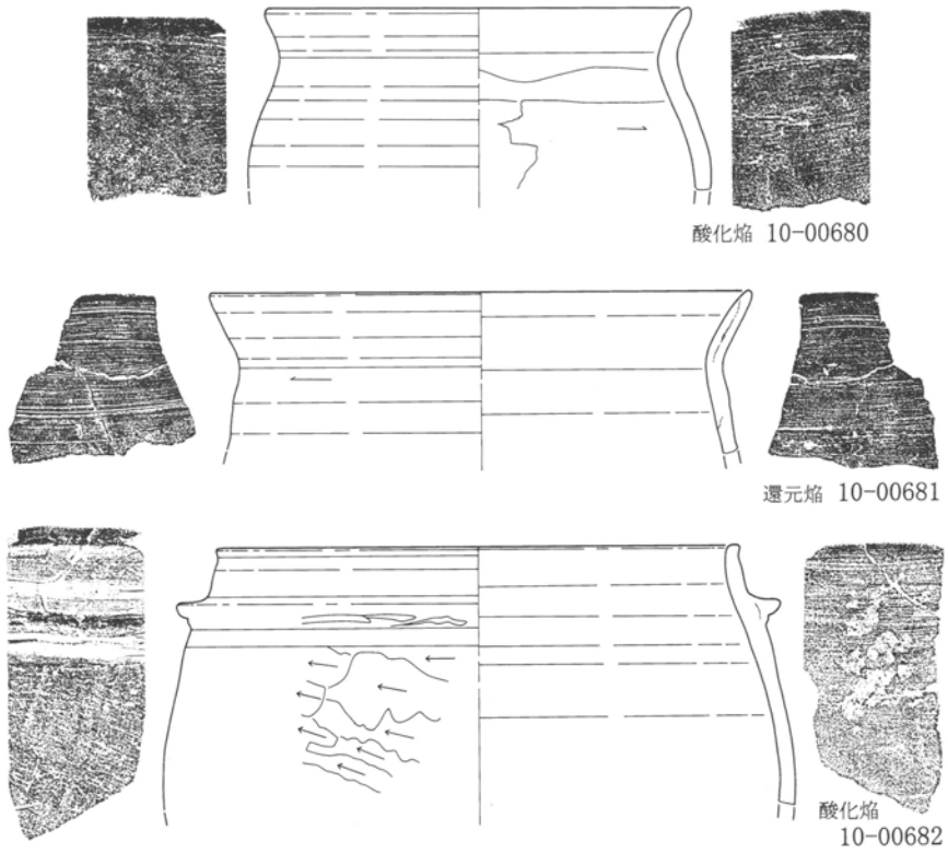
第118図 第11号住居跡出土遺物実測図 1 : 3 (3)
