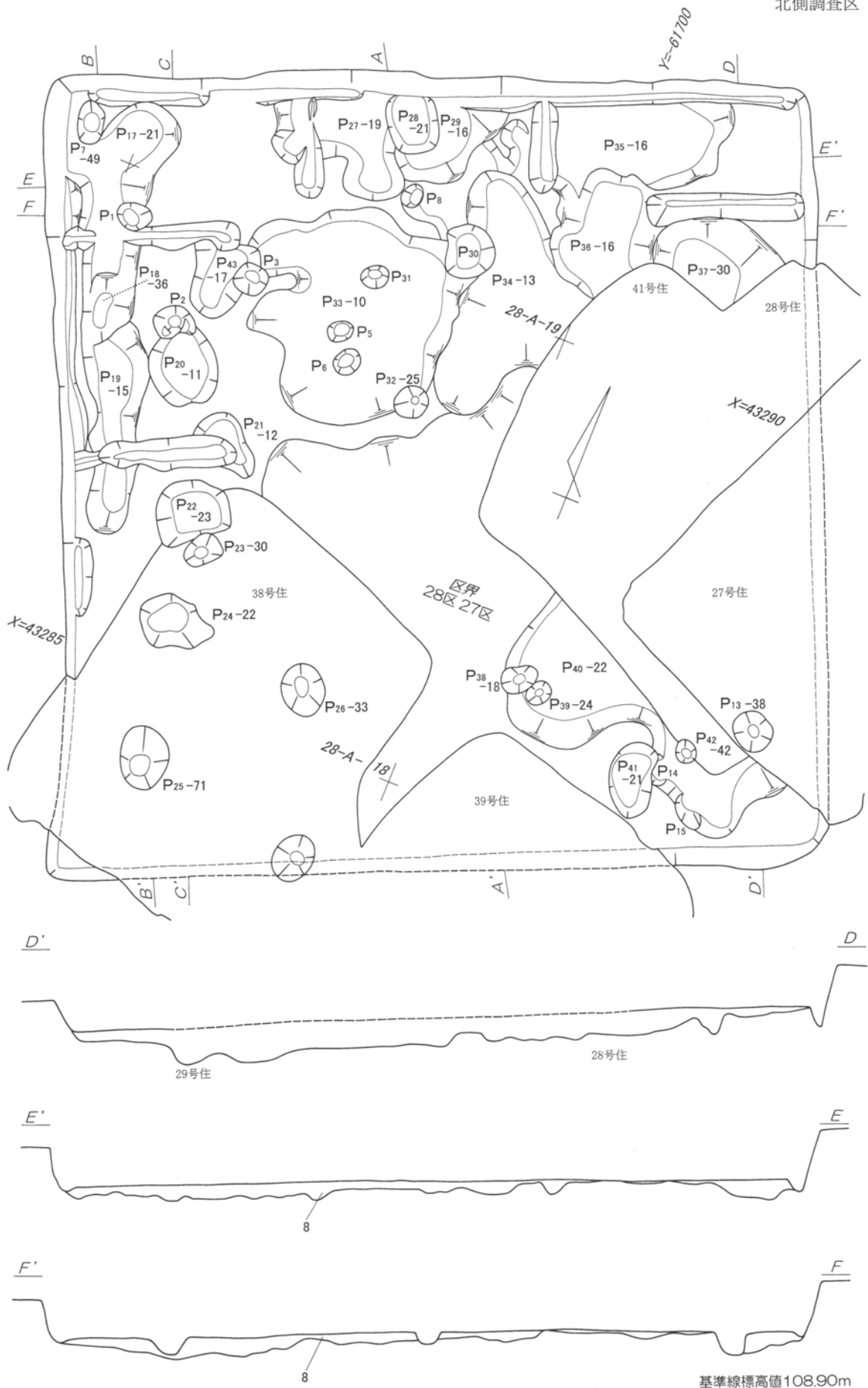
第192図 第42号住居跡掘方実測図 1 : 60
