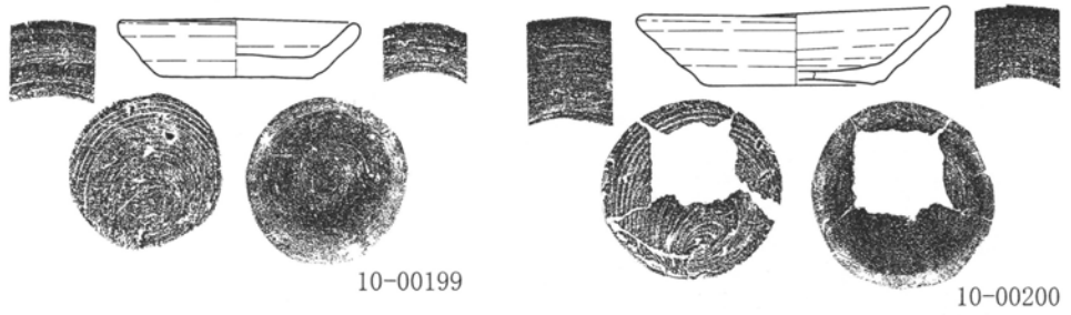
第45図 井戸跡 1 : 60 ・ 出土遺物実測図 1 : 3 ・ 1 : 4 (1)
