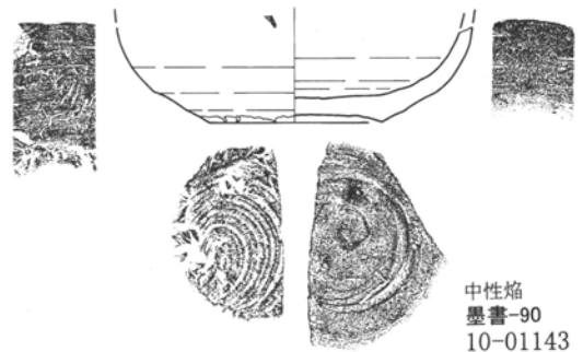
第231図 第60・61号住居跡 1 : 60・第60号住居跡出土遺物実測図 1 : 3 (1)
