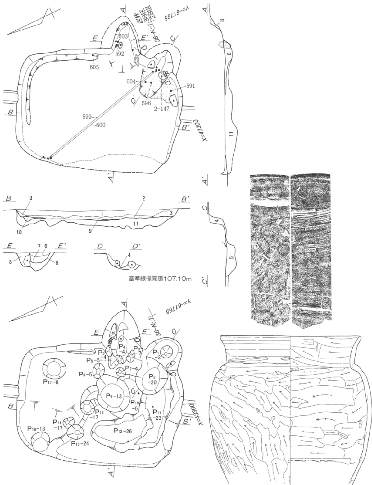
第96図 第3号住居跡 1:60・出土遺物実測図 1:3 (2)
