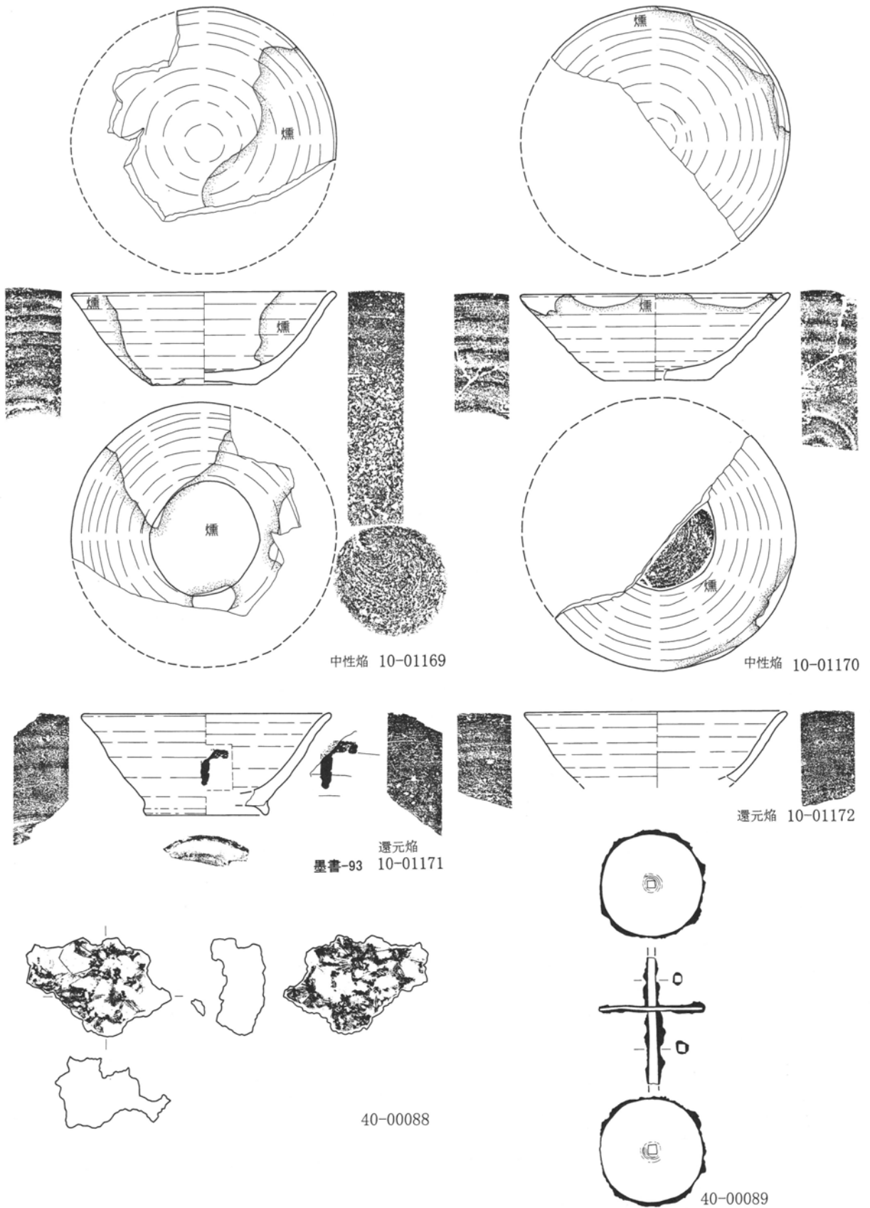
第239図 第65号住居跡出土遺物実測図 1 : 3 (3)
