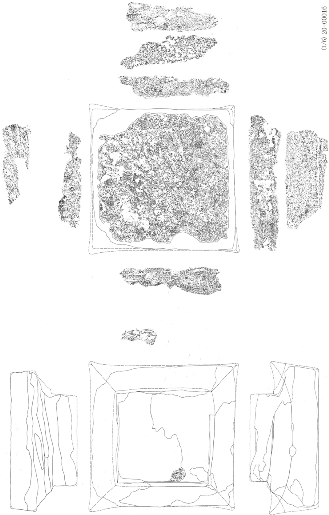
第14図 溝状遺構出土遺物実測図1：6（9）（C4溝）
