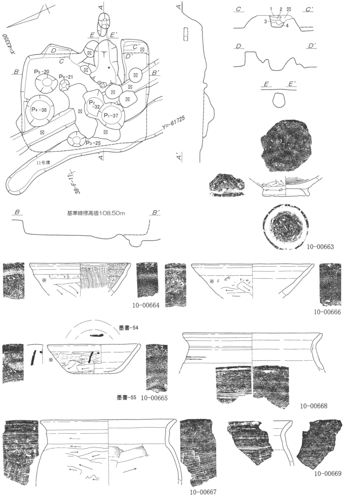
第115図 第10号住居跡 1 : 60 · 出土遺物実測図 1 : 3
