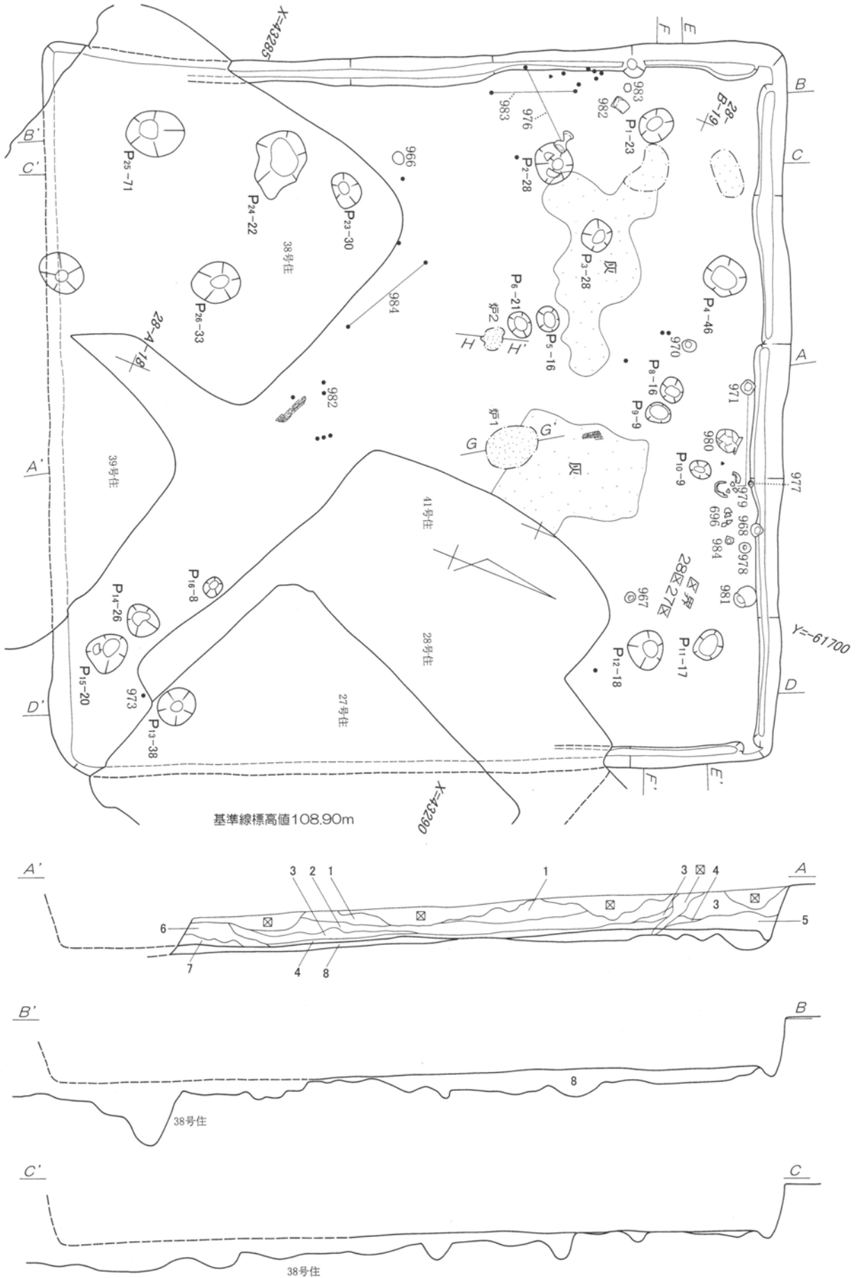
第191図 第42号住居跡実測図 1 : 60
