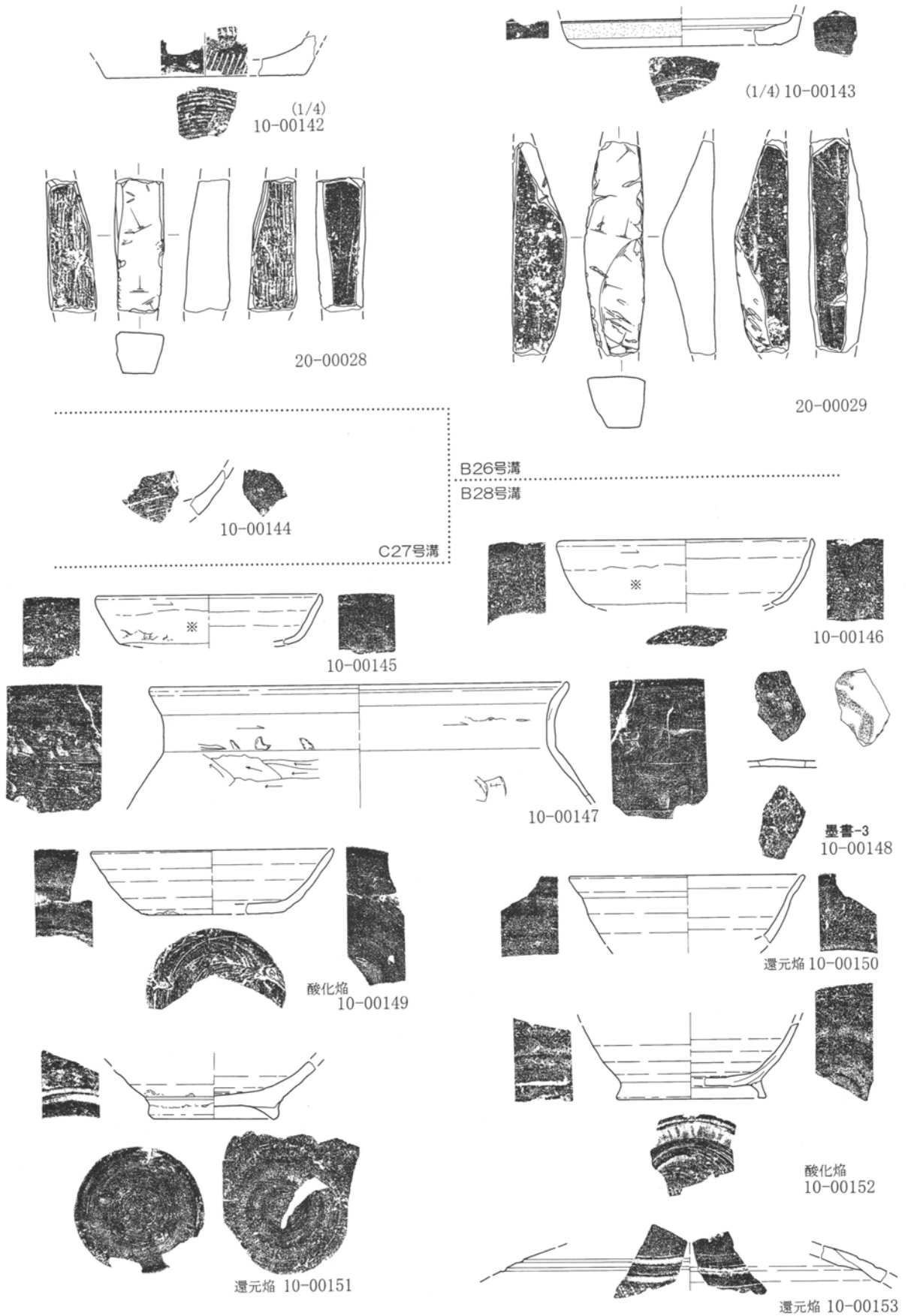
第27図 溝状遺構出土遺物実測図 1 : 3 · 1 : 4 (21)
