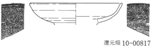
第157図 第29号住居跡 1:60・出土遺物実測図 1:3
