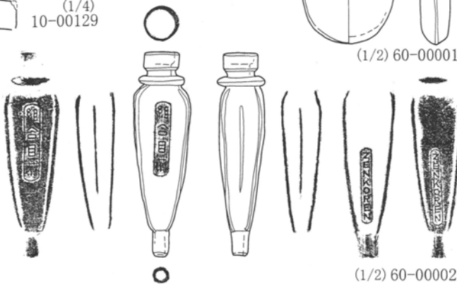
第22図 溝状遺構出土遺物実測図 1 : 2 · 1 : 3 · 1 : 4 (16)
