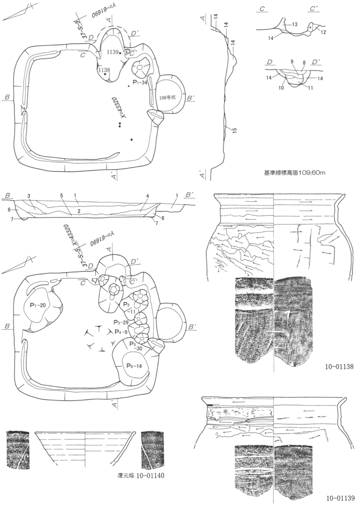
第229図 第57号住居跡 1:60・出土遺物実測図 1:3 (1)
