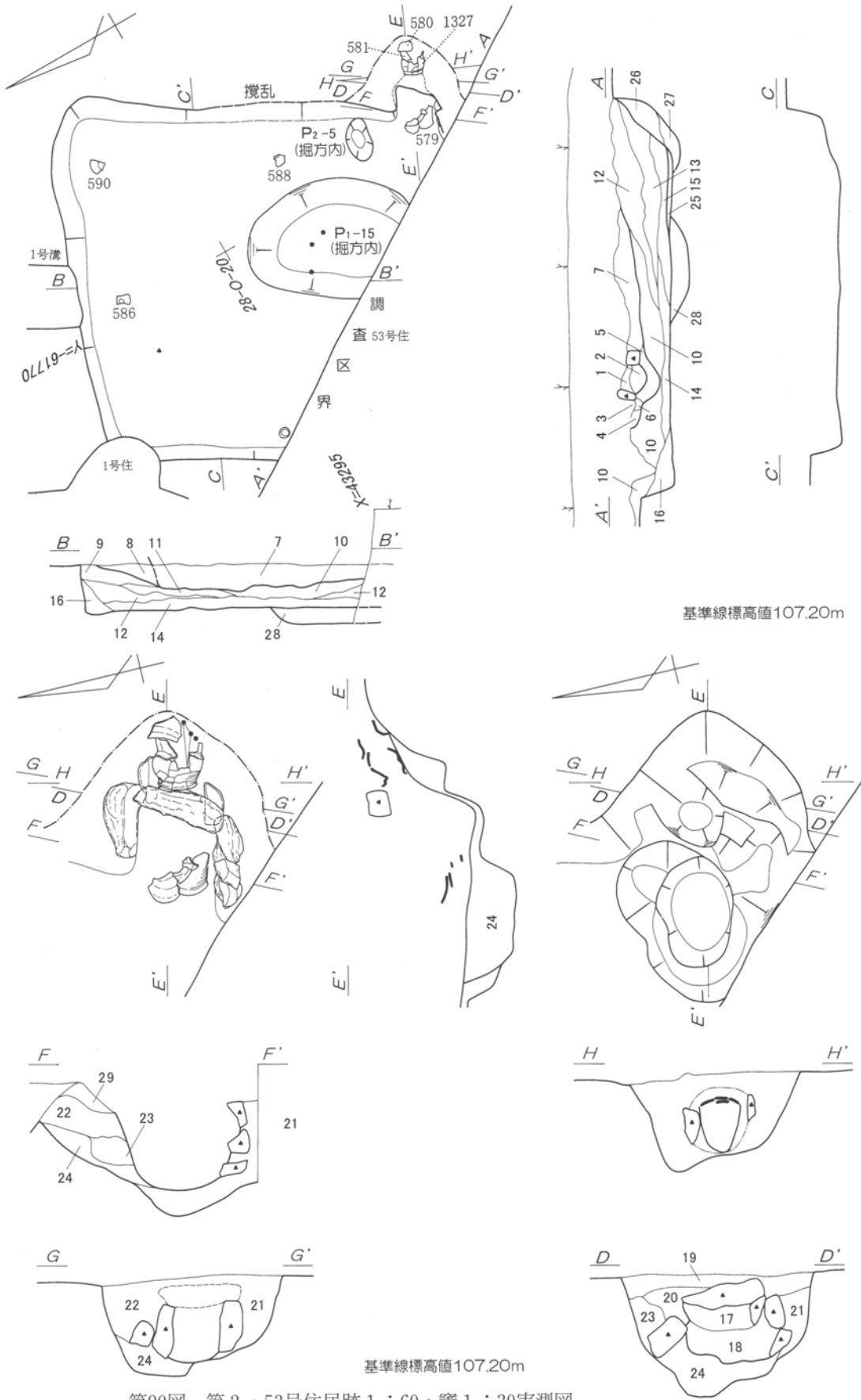
第90図 第2・53号住居跡 1:60・竈 1:30実測図
