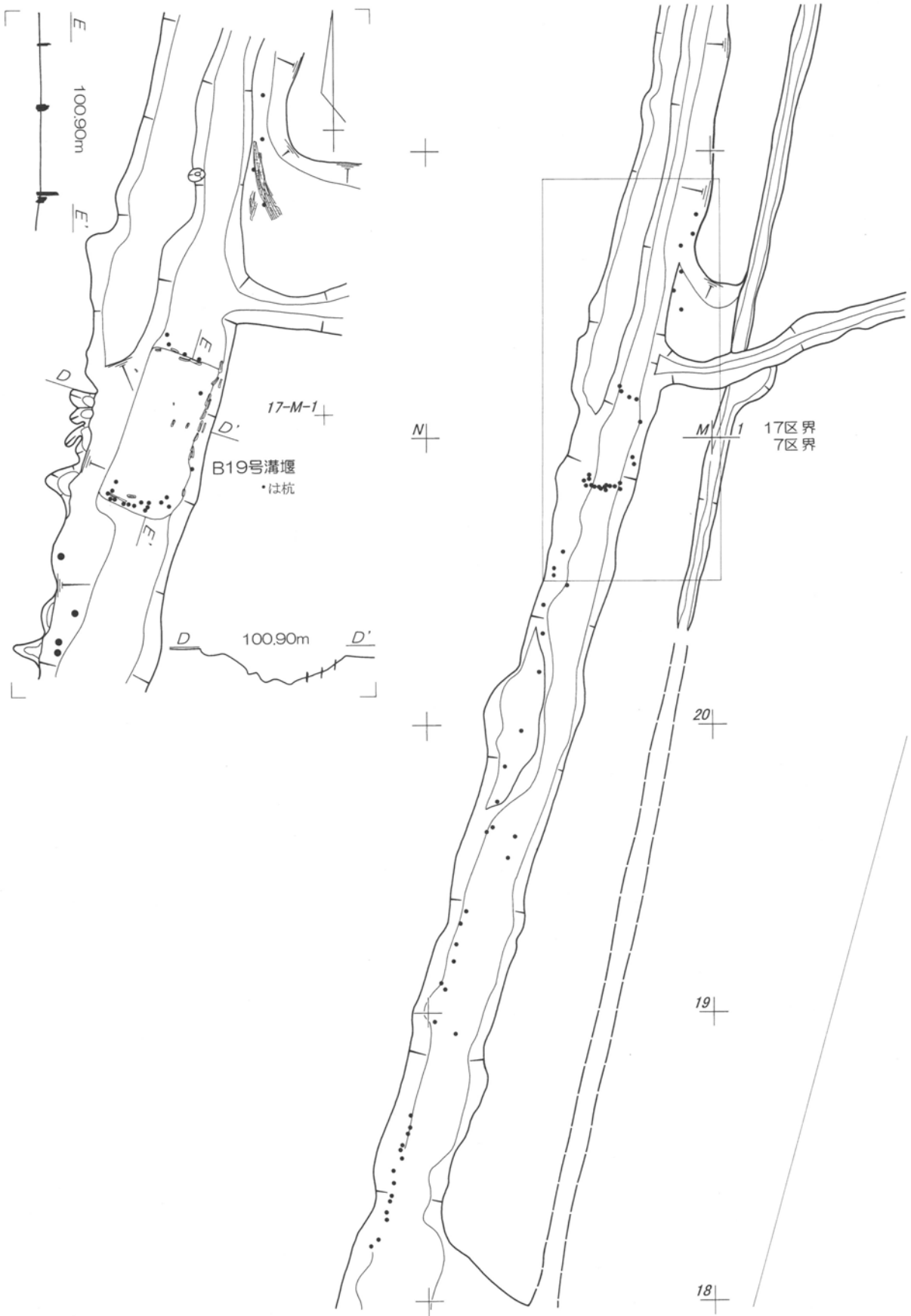
第20図 第19号溝状遺構実測図 1 : 50 · 1 : 100
