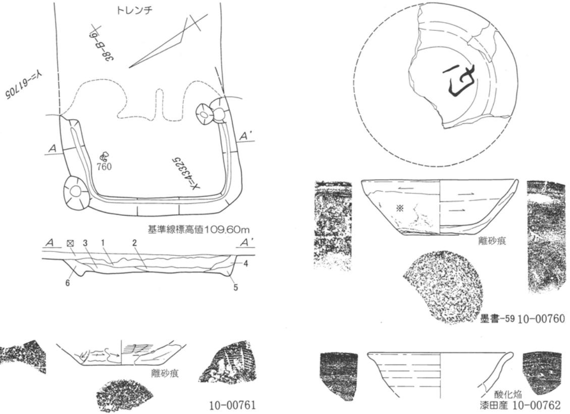
第144図 第23号住居跡出土遺物実測図 1 : 3
