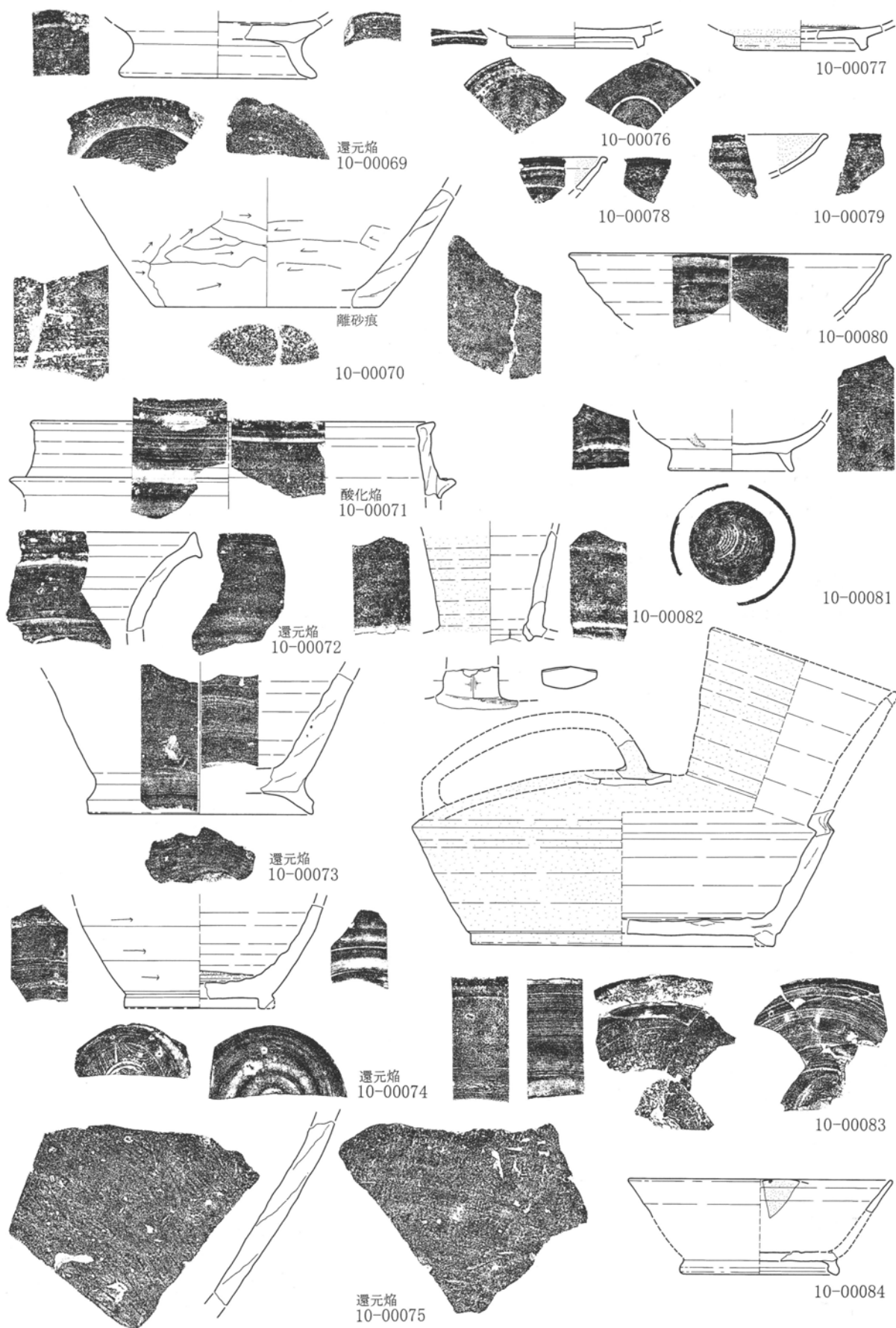
第18図 溝状遺構出土遺物実測図 1 : 3 (13) (C16溝)
