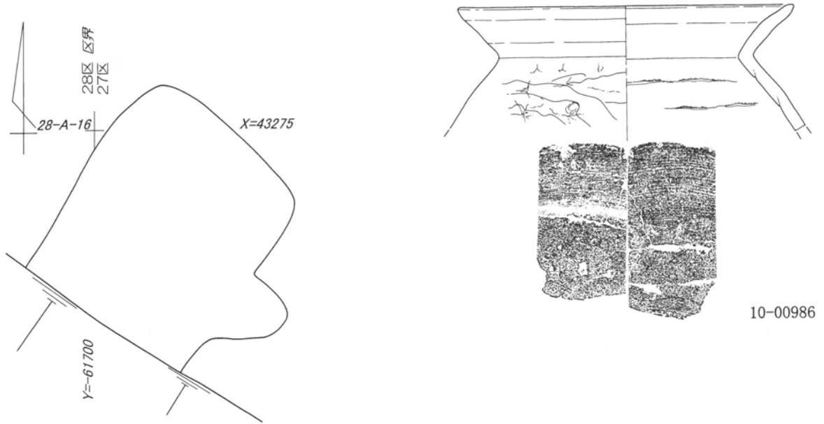
第197図 第43号住居跡 1 : 60・出土遺物実測図 1 : 3
