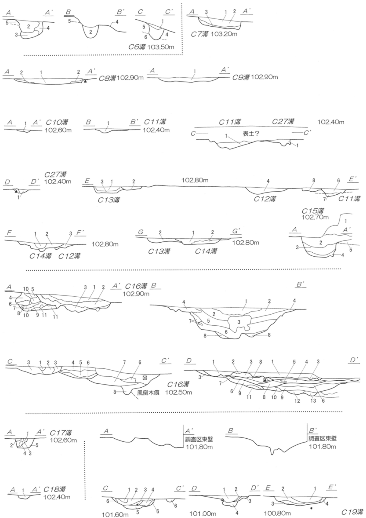
第3図 第6~19号溝状遺構土層断面図 1:60
