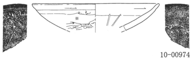
第193図 第42号住居跡出土遺物実測図 1 : 3 (2)
