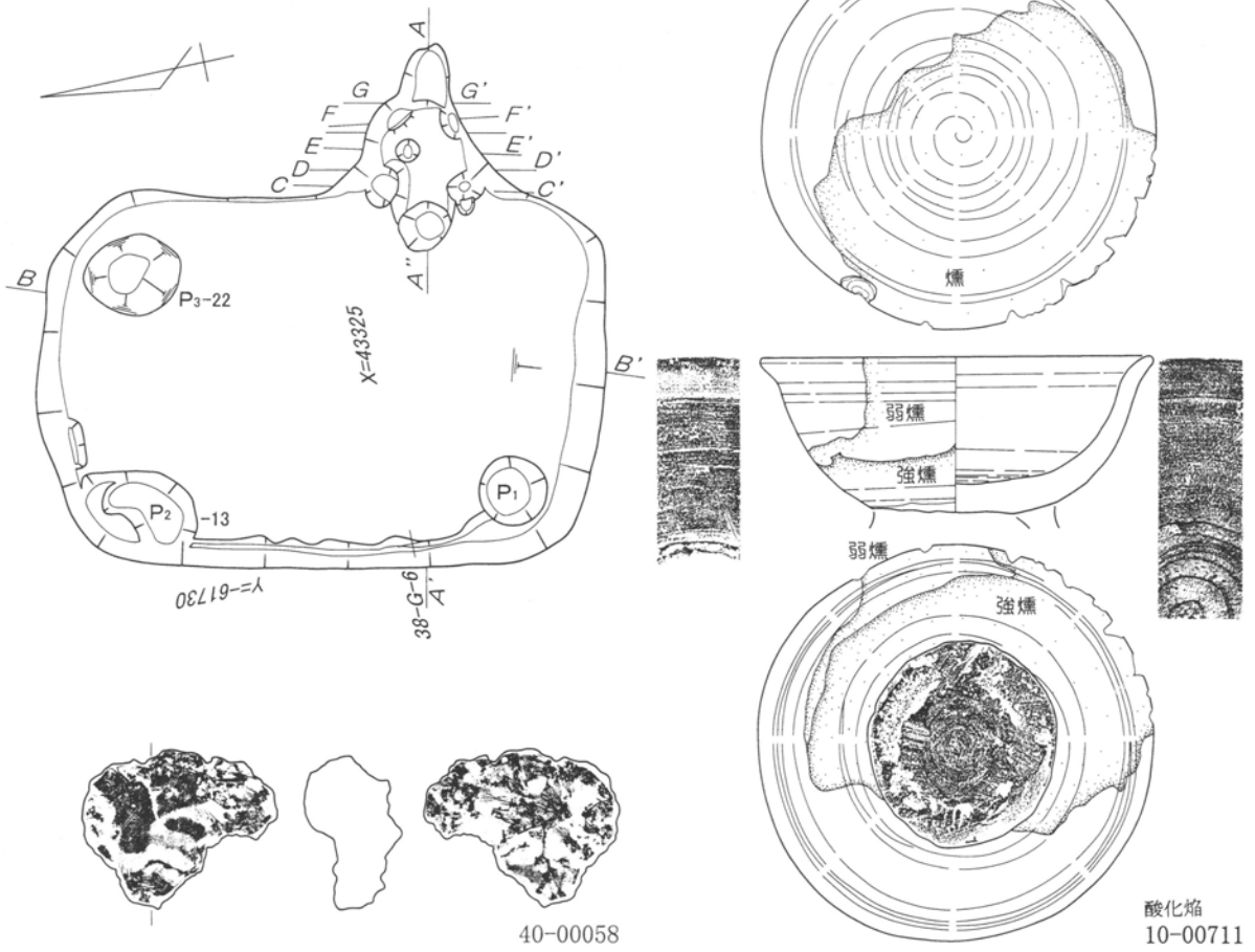
第128図 第17号住居跡 1:60・出土遺物実測図 1:3 (2)
