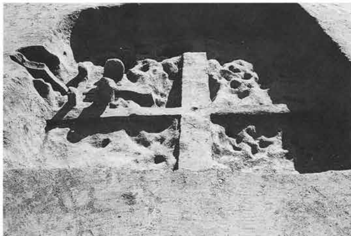
1 1区10号住居掘り方土層断面A-A' (北西から)
