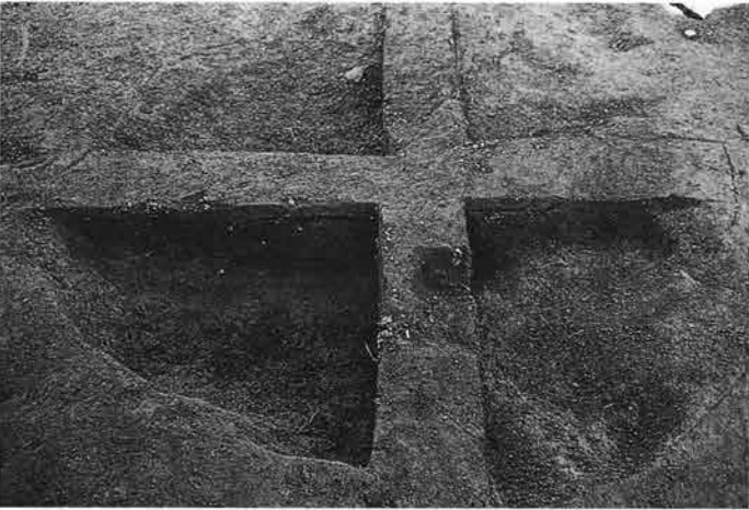
5 1区23号住居2号焼土土層断面O-O' (南東から)
