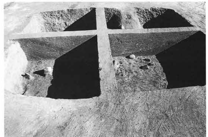
8 1区20号住居土層断面B-B' (南西から)
