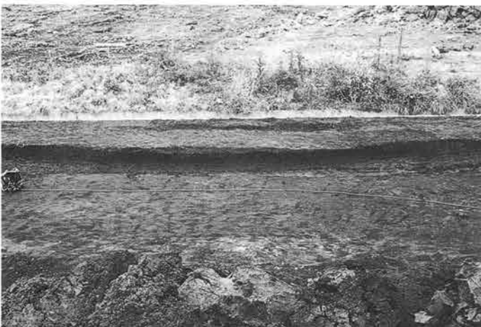
5 3区谷部横断土層断面(南から)
