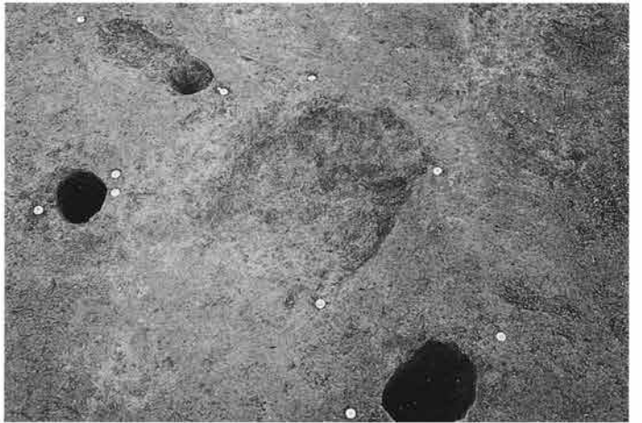
6 1区23号住居2号焼土底面全景 (南東から)
