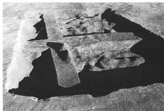
8 1区7号住居掘り方土層断面B-B' (南西から)
