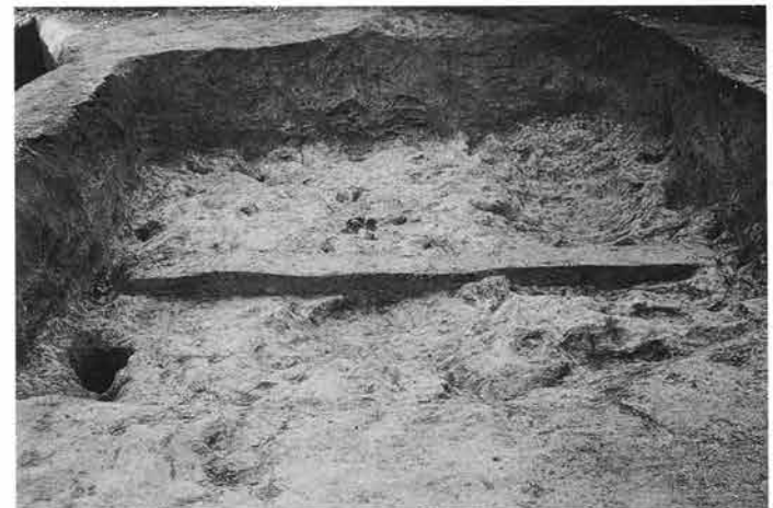
8 2区1号住居掘り方土層断面A-A' (南東から)
