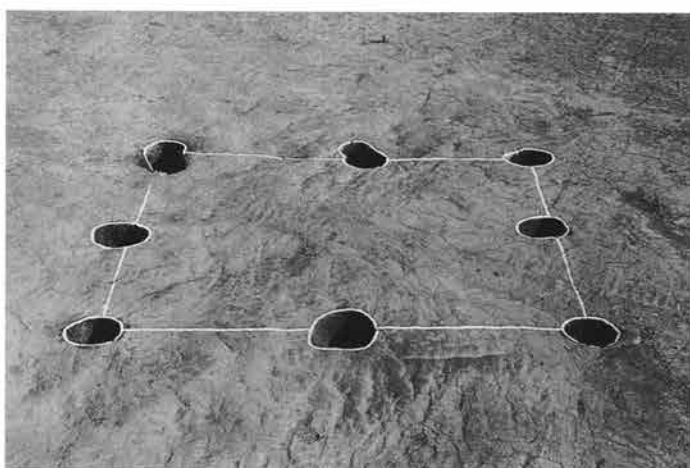
3 1区2号掘立柱建物全景 (南西から)
