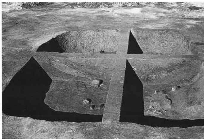
7 1区20号住居土層断面A-A' (南東から)
