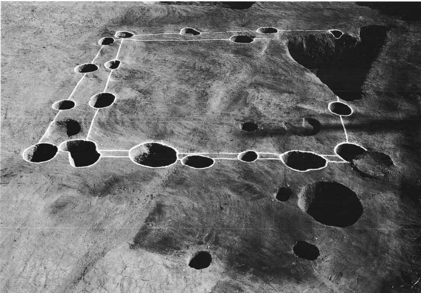
5 1区1号・3号掘立柱建物全景(南西から)
