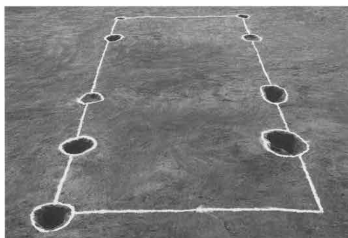
7 5号掘立柱建物 (東から)
